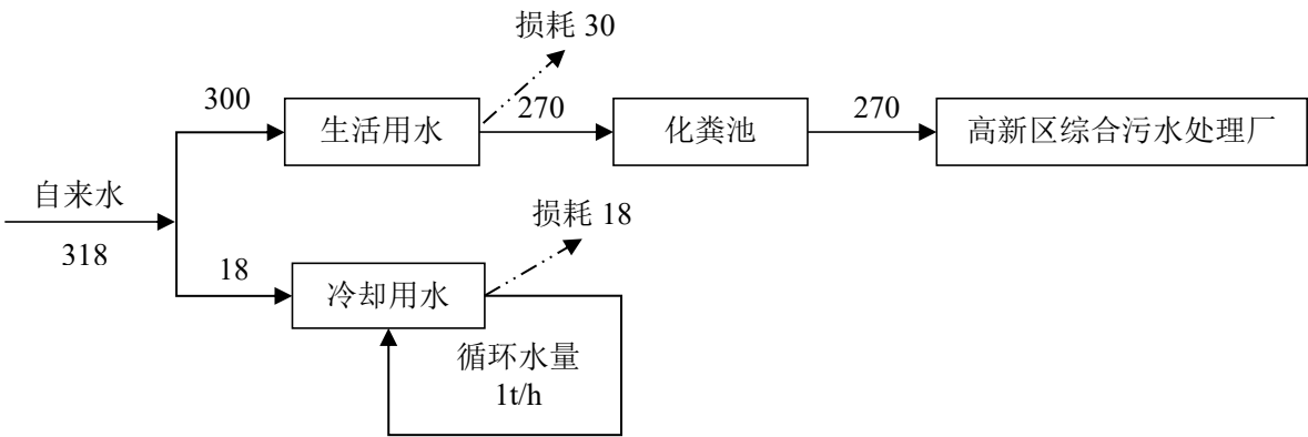
图 2-1 项目水平衡图（单位： m³/a）
