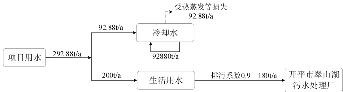
图 2-1 水平衡图
