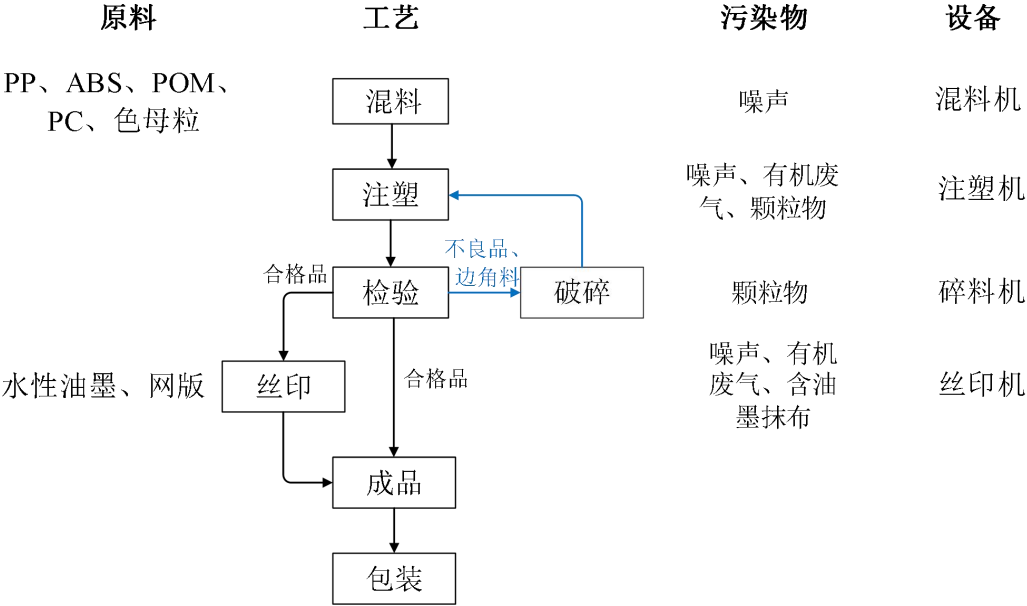
图2-2 注塑工艺流程
