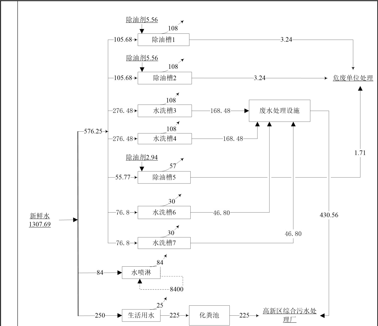
图 2-2 项目年水平衡图（单位：吨/年）
