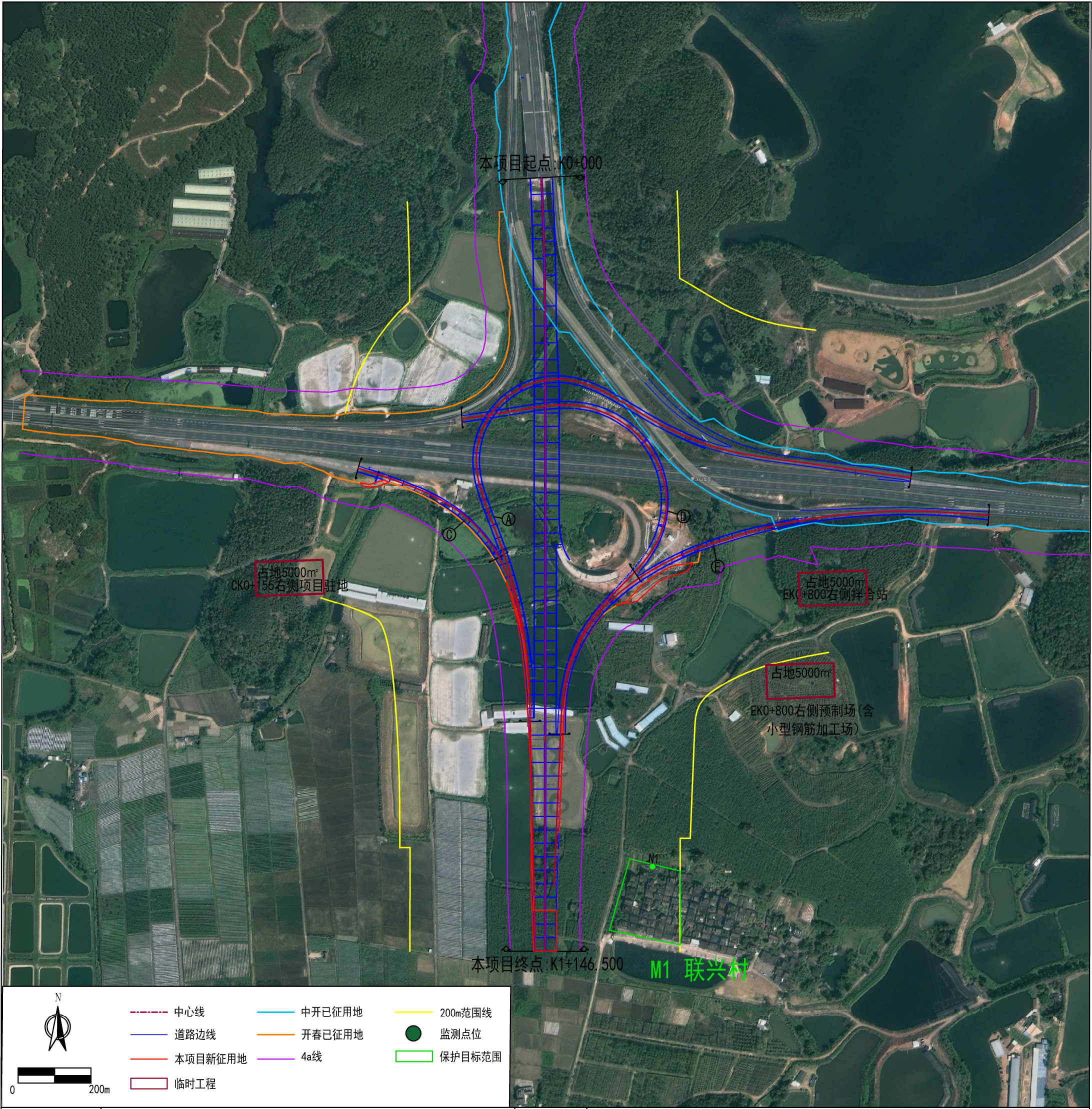
项目名称 广台高速公路开平至台山段先行工程（罗汉山枢纽互通） 图名 附图3 声环境保护目标、监测点位布置图
