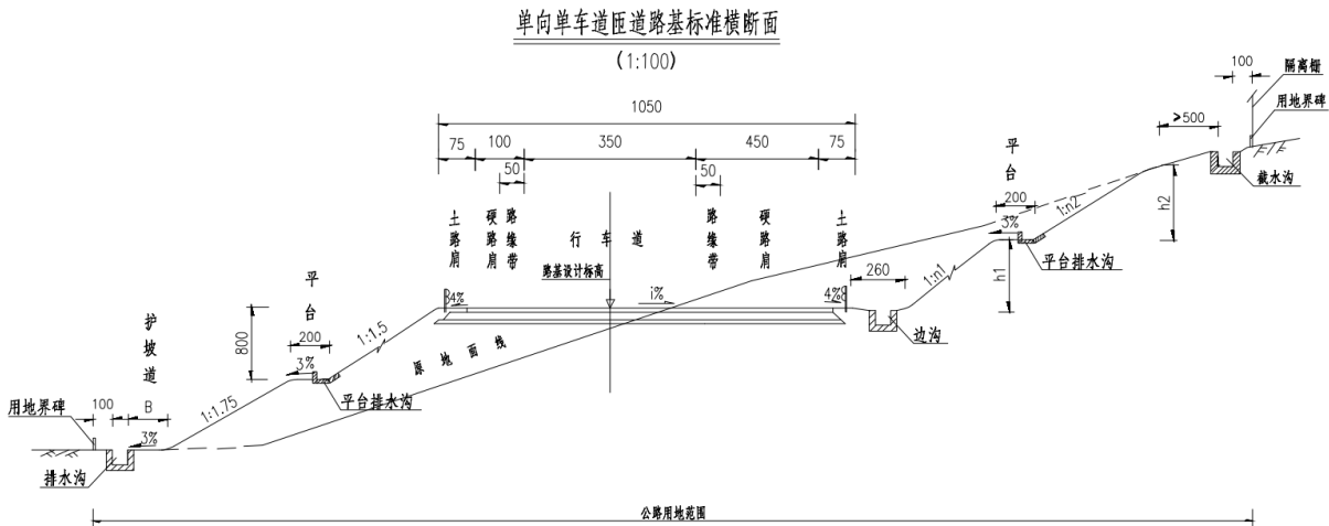
图 2.2-4 单向单车道标准横断面（C 匝道）
