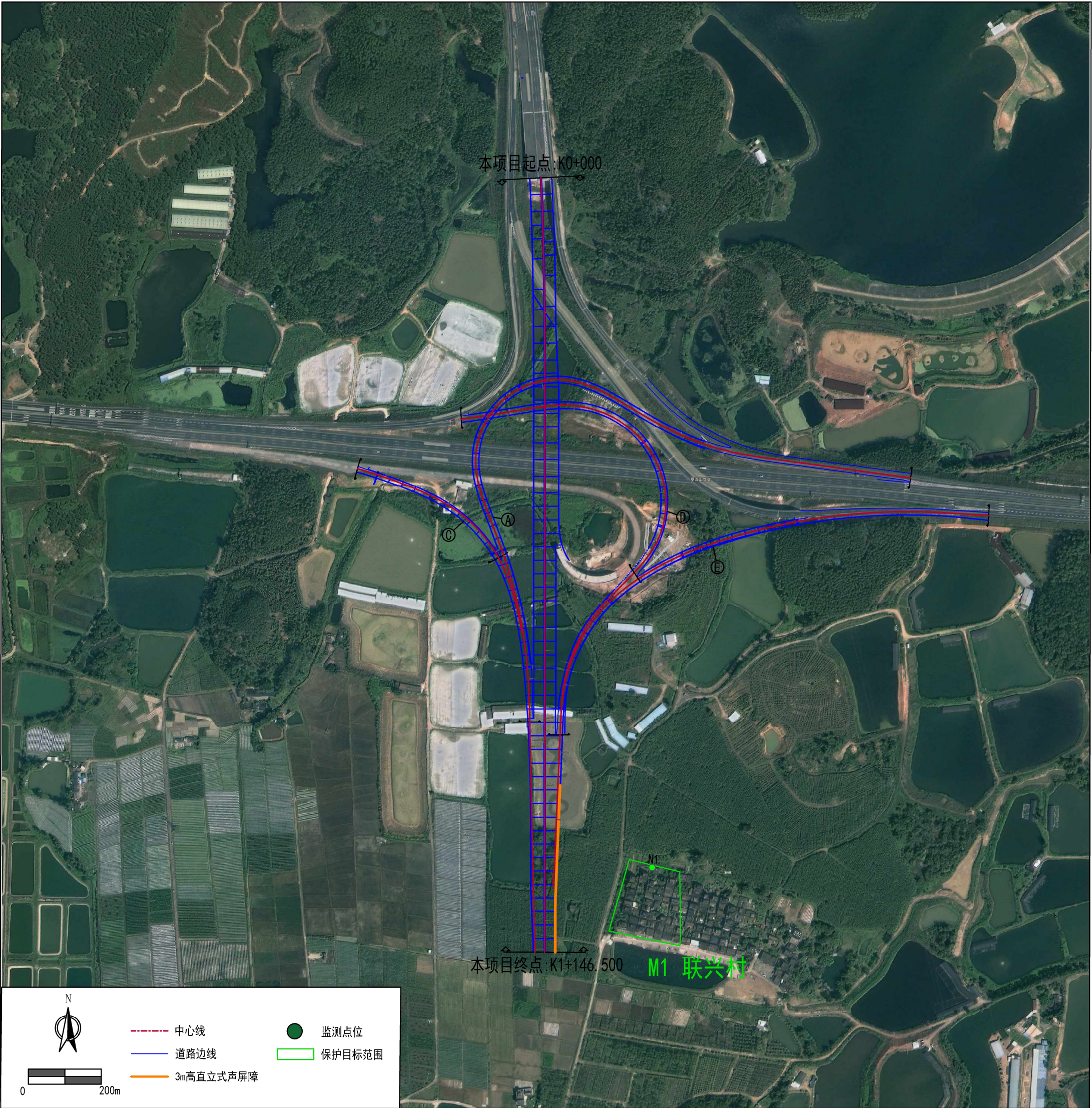
项目名称 广台高速公路开平至台山段先行工程（罗汉山枢纽互通） 图名 附图4 噪声污染防治措施平面布置图
