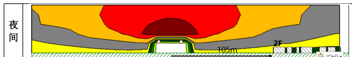
图 4.1-8 本项目运营中期垂直声场情况
