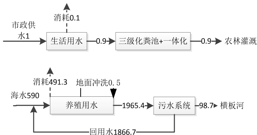
图 4-1 水平衡图 (t/d)
