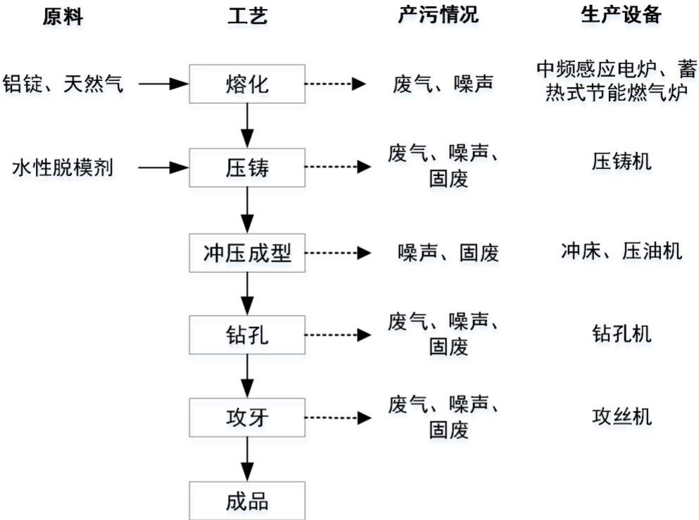
图 2-2 生产工艺及产污节点图
