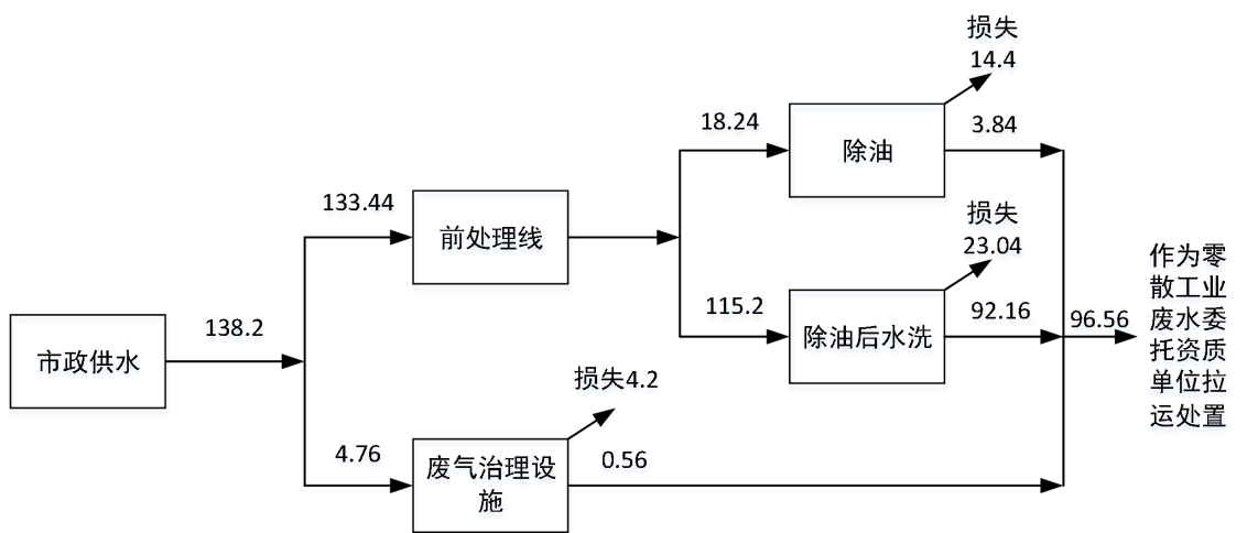
图 2-1 本项目水平衡图 (单位: m³)
