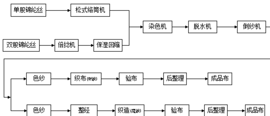
图 2-4 色布生产工艺
