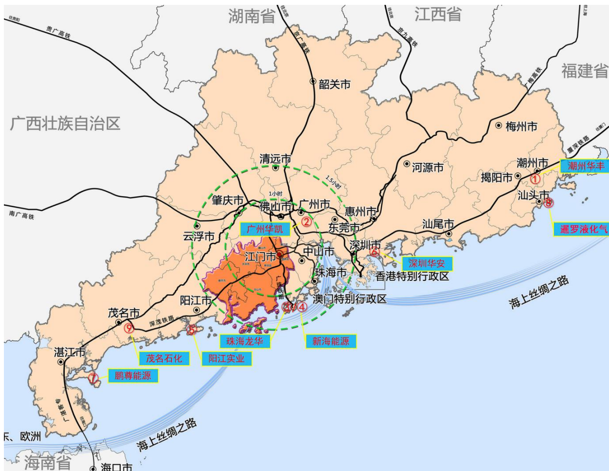
图 9 广东省液化石油气储库分布图（序号与上表对应）
