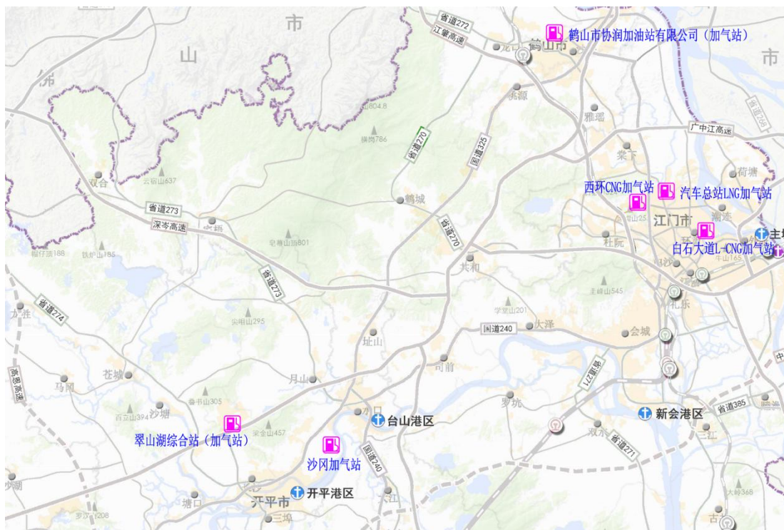
图 5 天然气汽车加气站现状分布图
