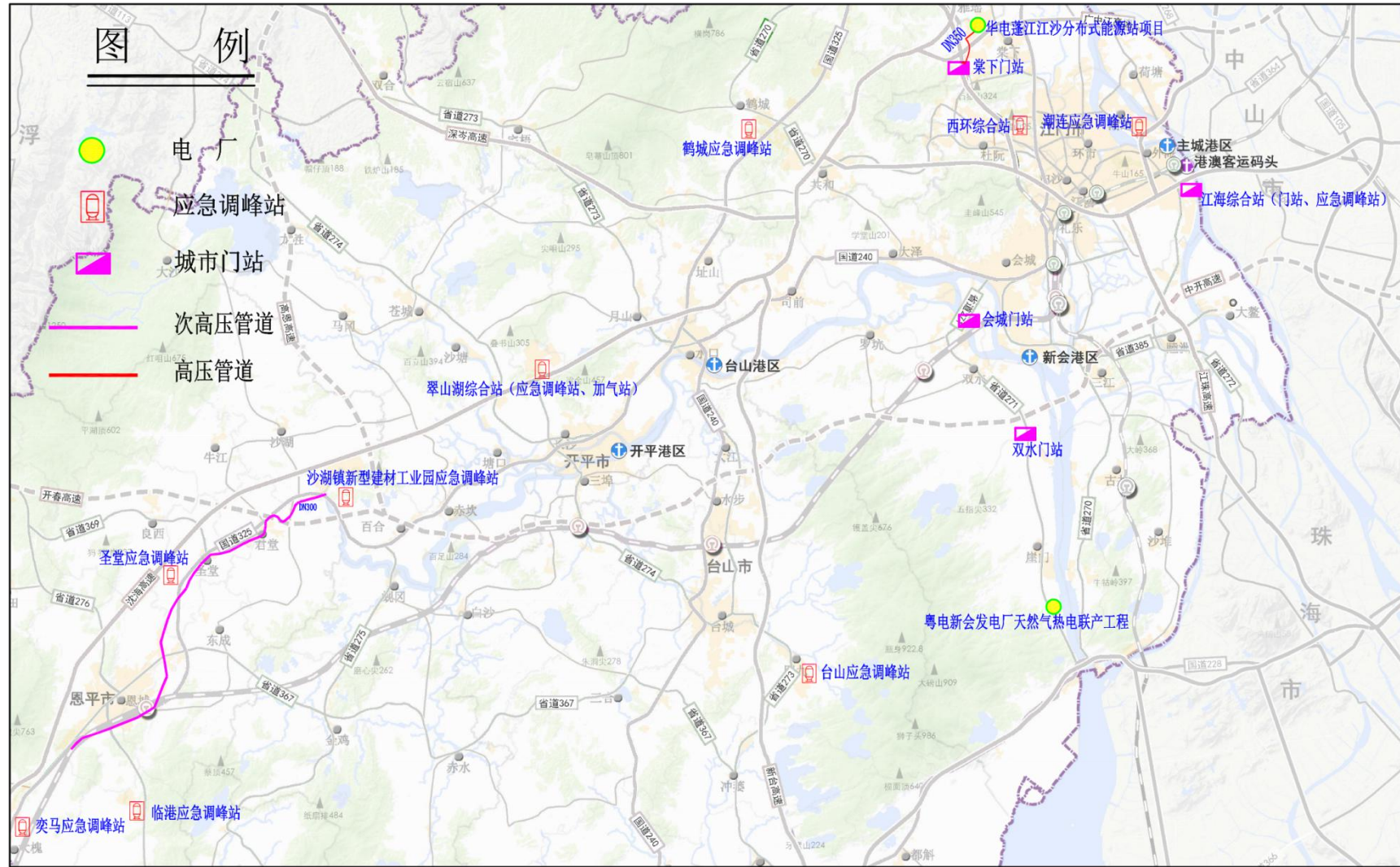
图 4 现状天然气场站、管线设施分布图
