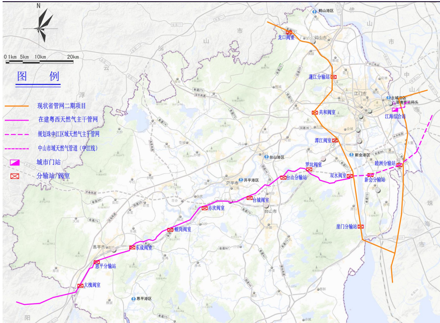
图 11 天然气气源规划图
