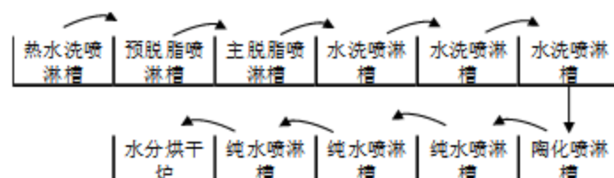
图 3.4-4 车架、五金配件喷粉线前处理工艺流程图
