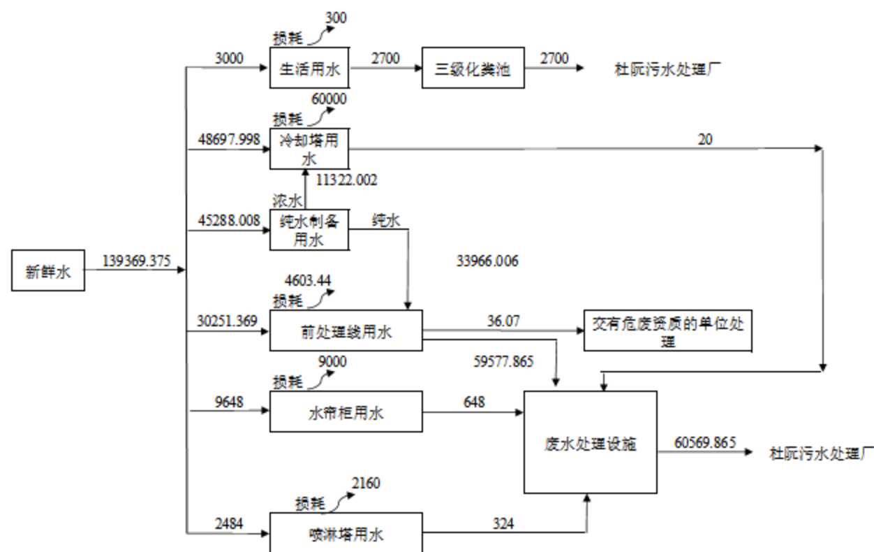
图 3.6-1 现有项目水平衡图 (t/a)
