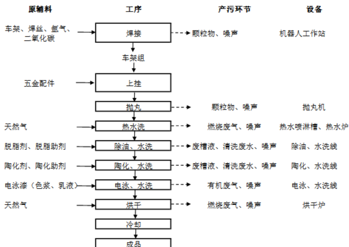
图 3.4-1 车架、五金配件电泳线工艺流程图
