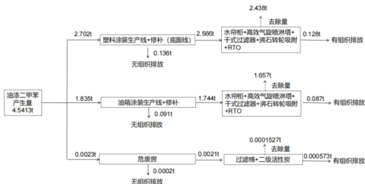
图 4.9-6 扩建项目二甲苯平衡分析图 (t/a)
