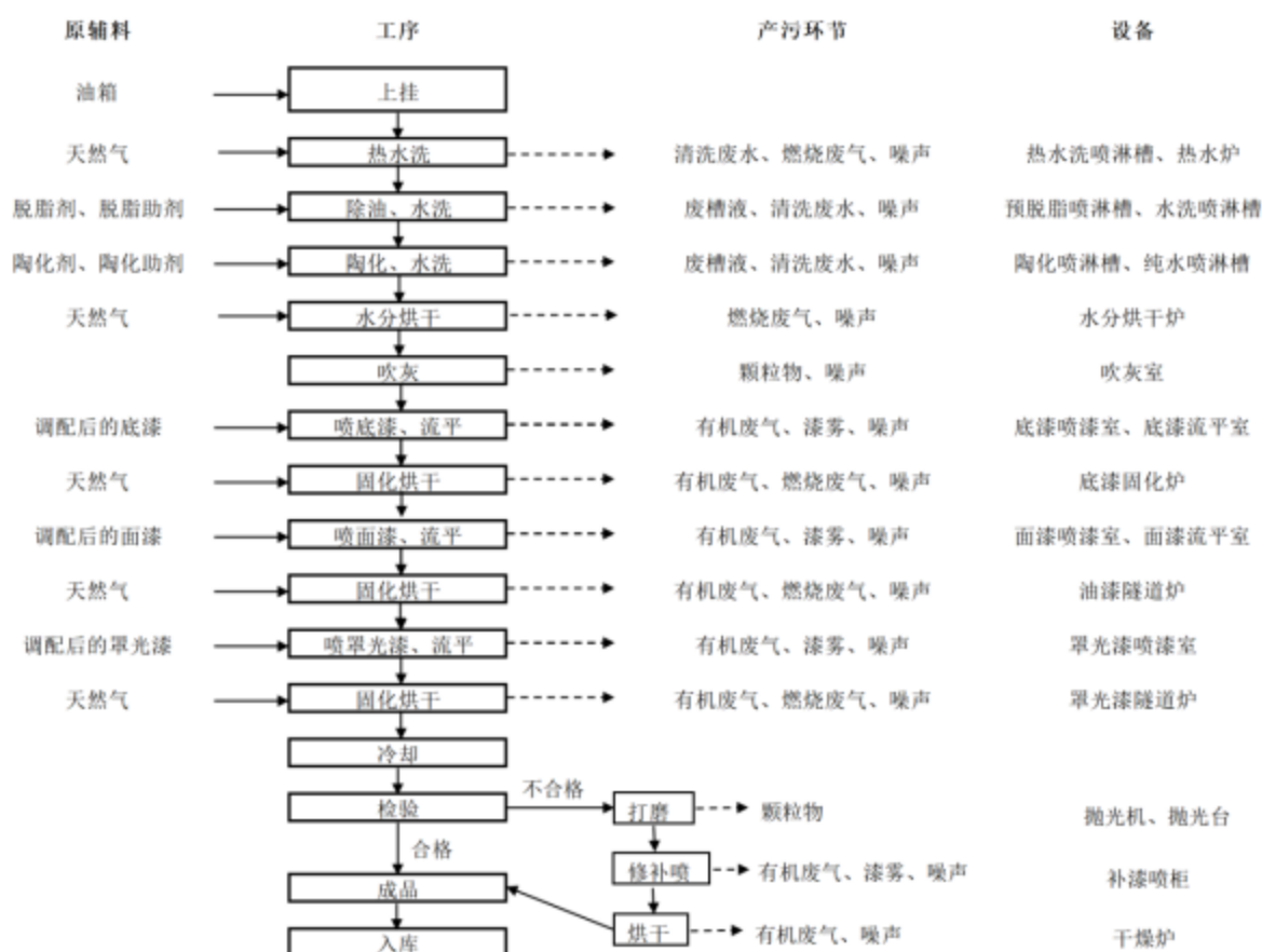
图 4.8-3 油箱生产线工艺流程图
