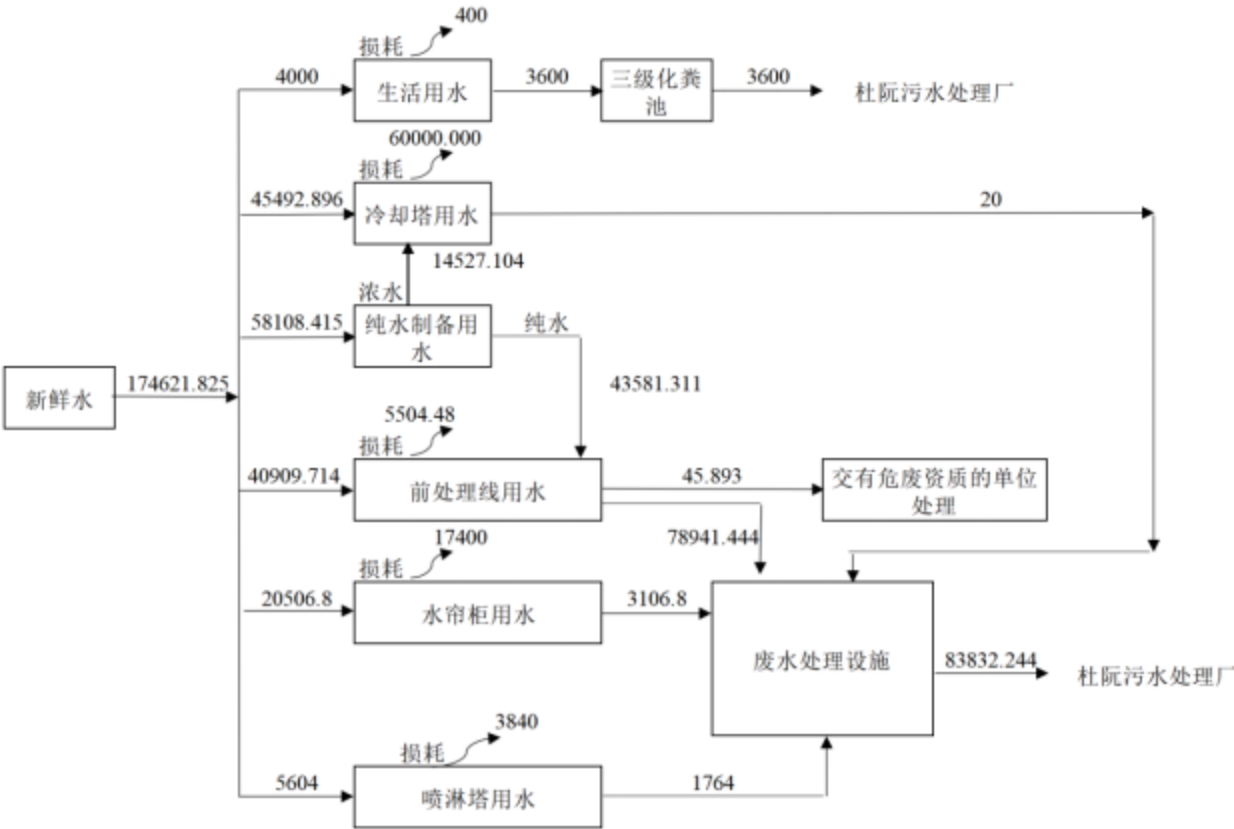
图 4.9-2 扩建后项目水平衡图 (t/a)
