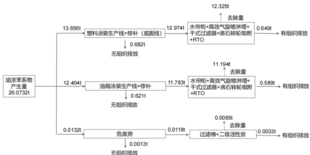
图 4.9-7 扩建项目苯系物平衡分析图 (t/a)
