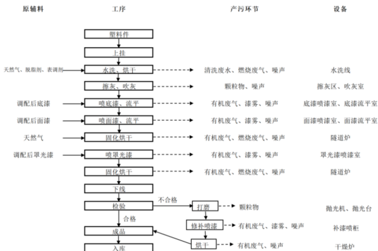
图 4.8-1 塑料件涂装工艺流程
