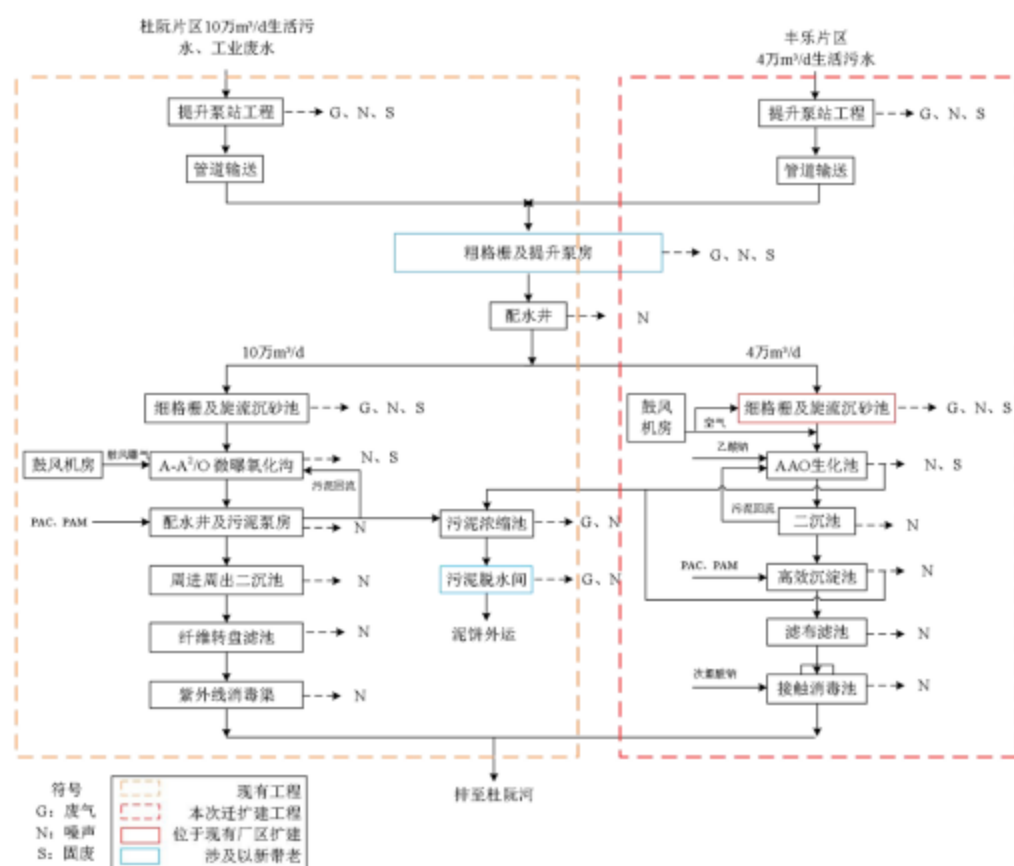
图 9.3-3 杜阮污水厂工艺流程图
