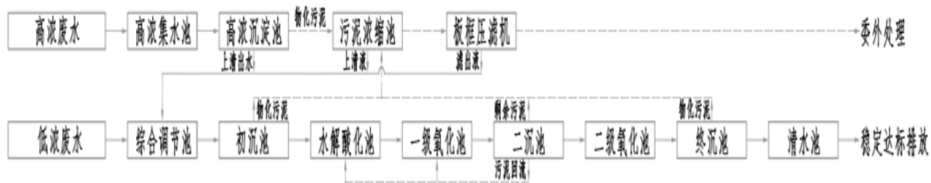
图 9.3-1 废水处理工艺流程图
