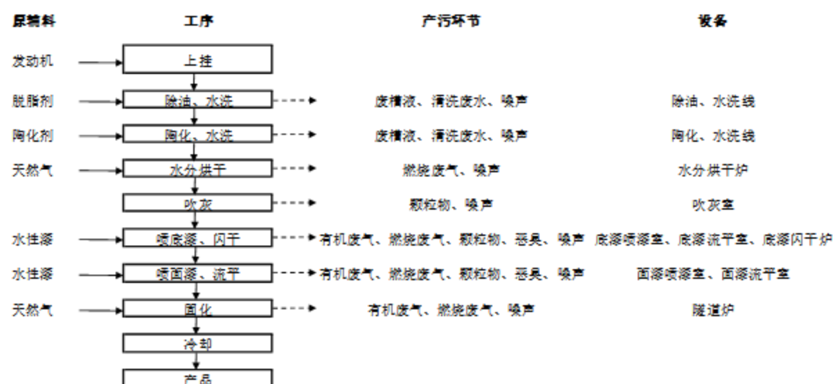
图 3.4-5 发动机八件套喷漆线工艺流程图
