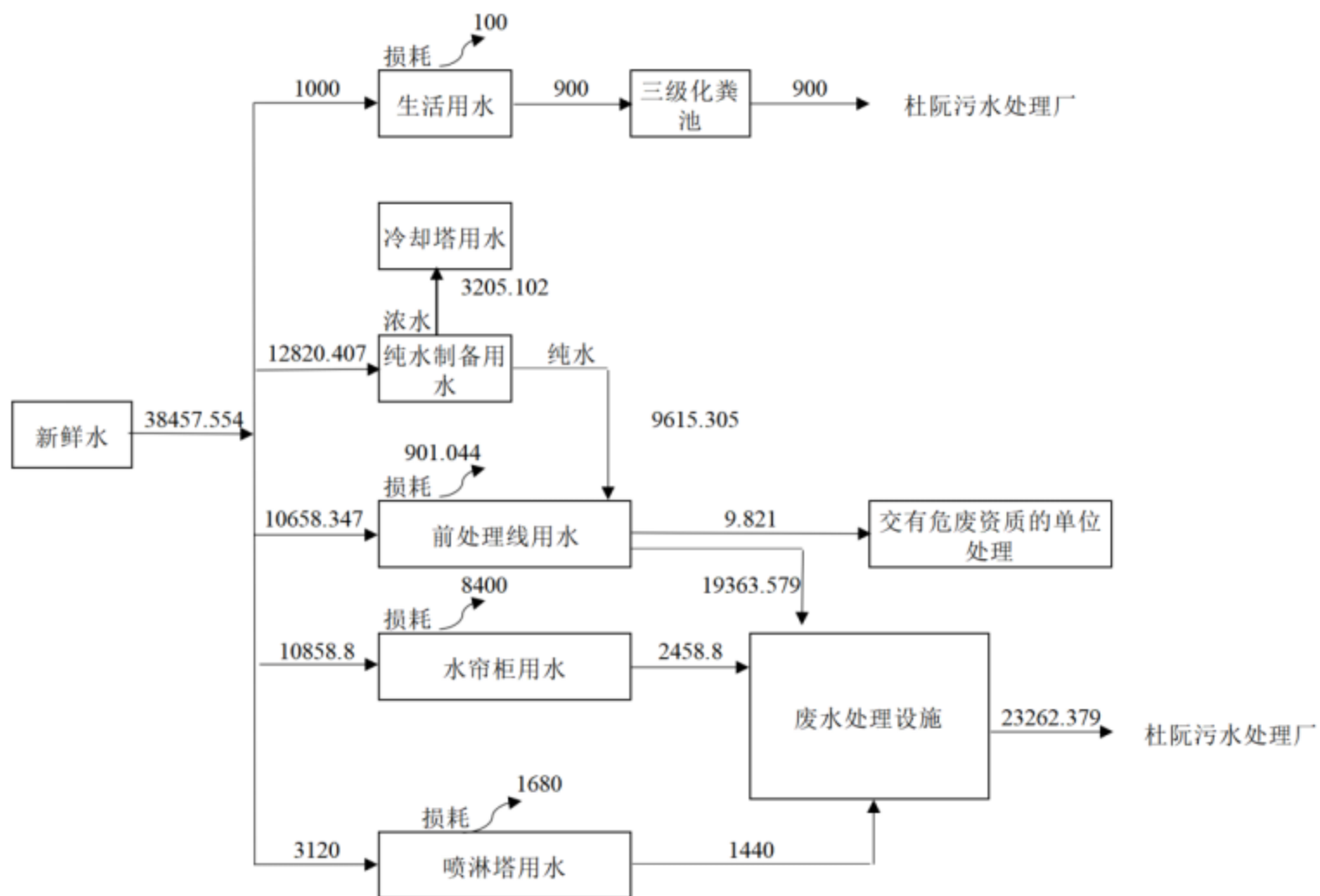
图 4.9-1 扩建项目水平衡图 (t/a)
