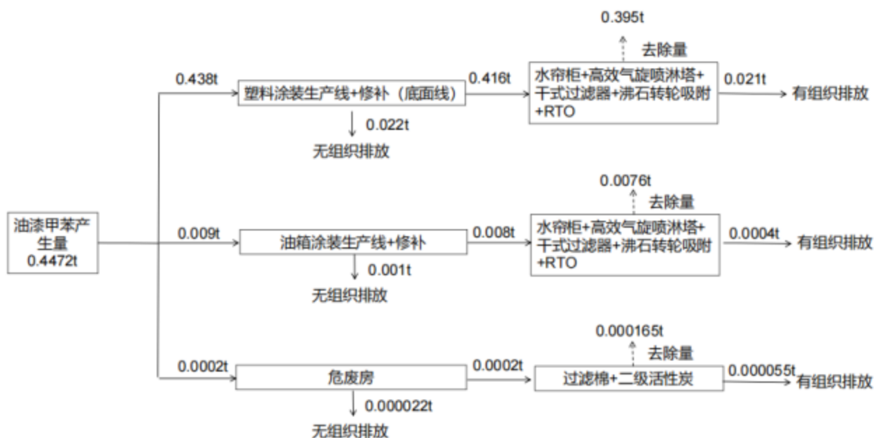
图 4.9-5 扩建项目甲苯平衡分析图 (t/a)
