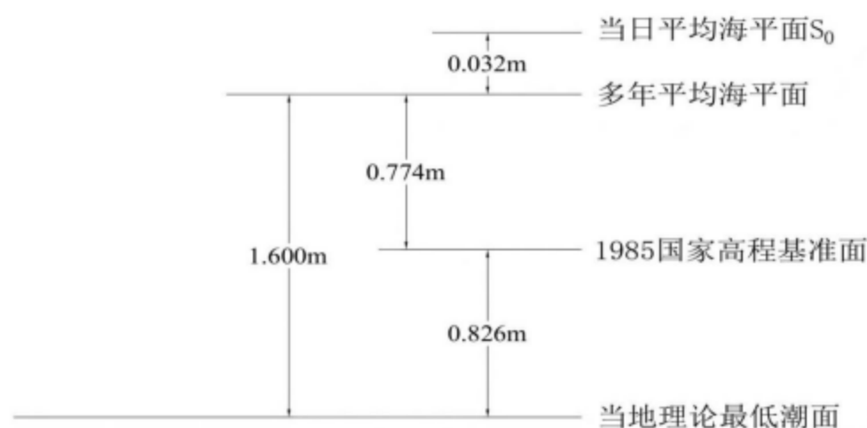
图 5.1.2-1b 基面换算关系示意图（川岛海域）
