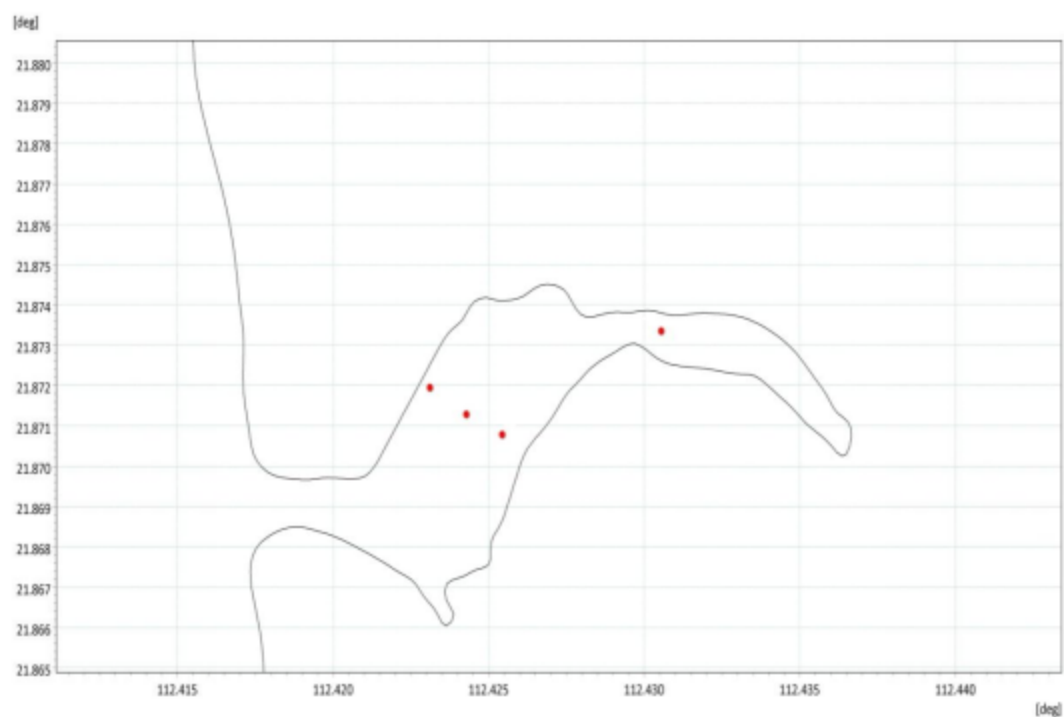
图 7.3.1-2 横山渔港典型工况源强分布图
