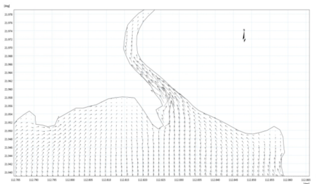
图 7.1.4-7 广海渔港（烽火角港区）附近海域现状涨急流场图
