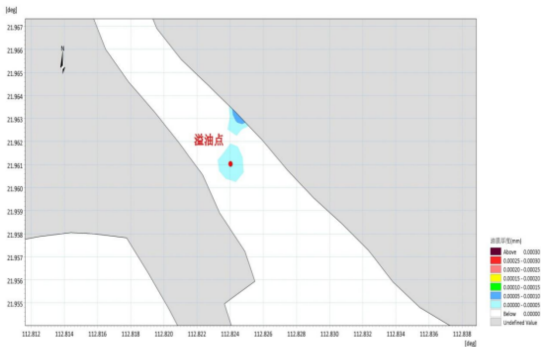
图 8.5.3-8 S 风向、13.8m/s 大潮落初发生溢油 72 小时油膜扫海范围图
