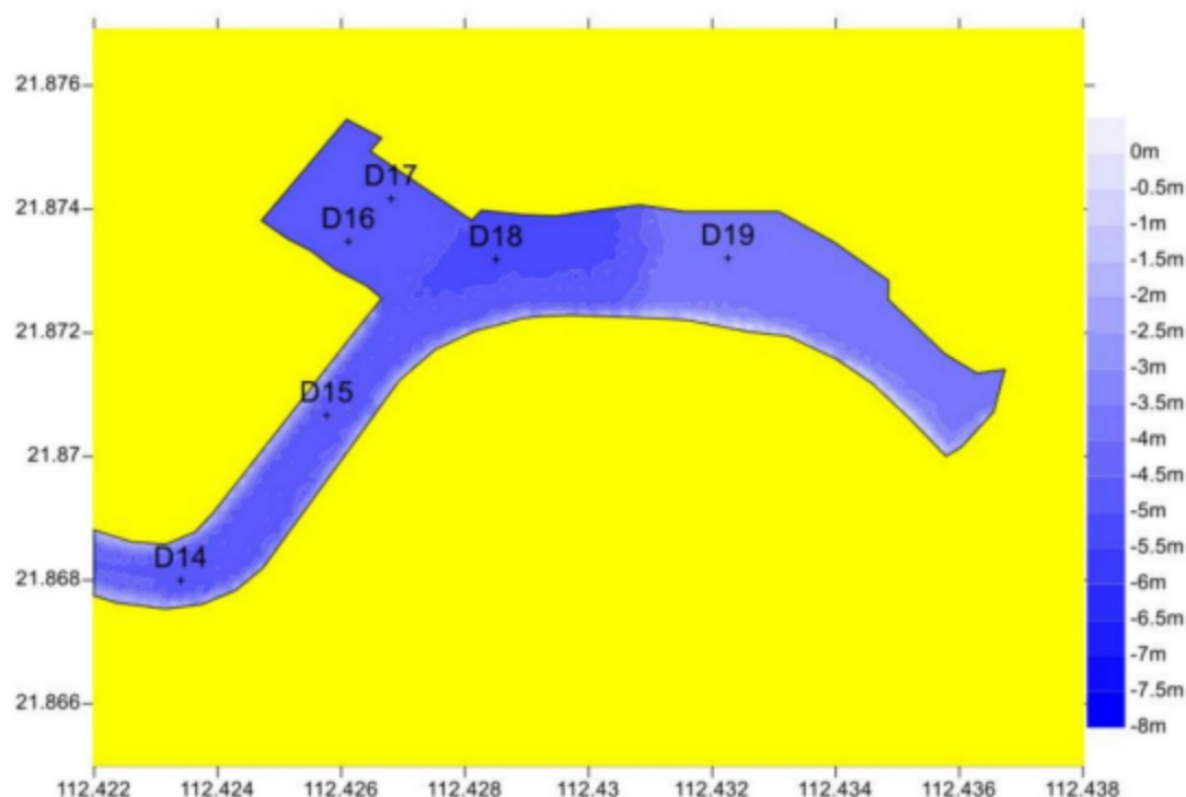
图 5.1.4-9 横山涌内港池和航道疏浚后水深及回淤代表点示意图
