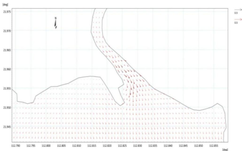
图 7.1.4-12 广海渔港（烽火角港区）工程前后海域落急流场对比图
