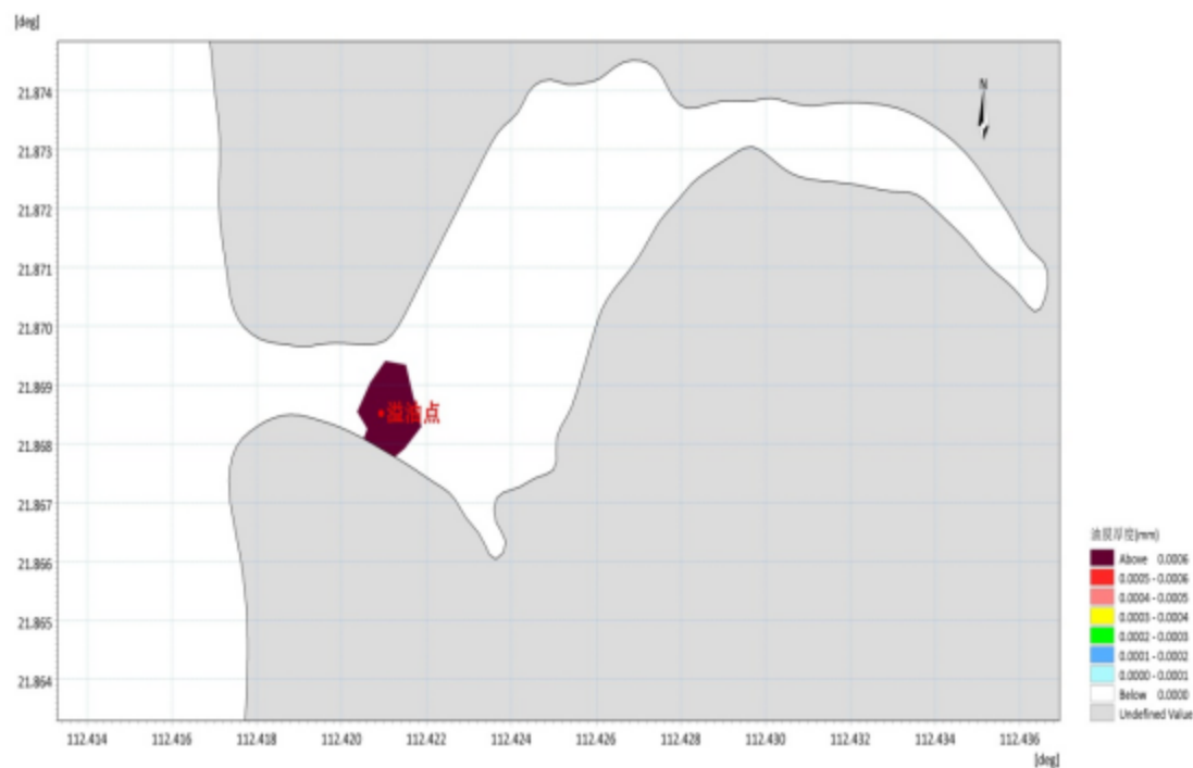
图 8.5.2-6 N 风向、13.8m/s 大潮落初发生溢油 72 小时油膜扫海范围图
