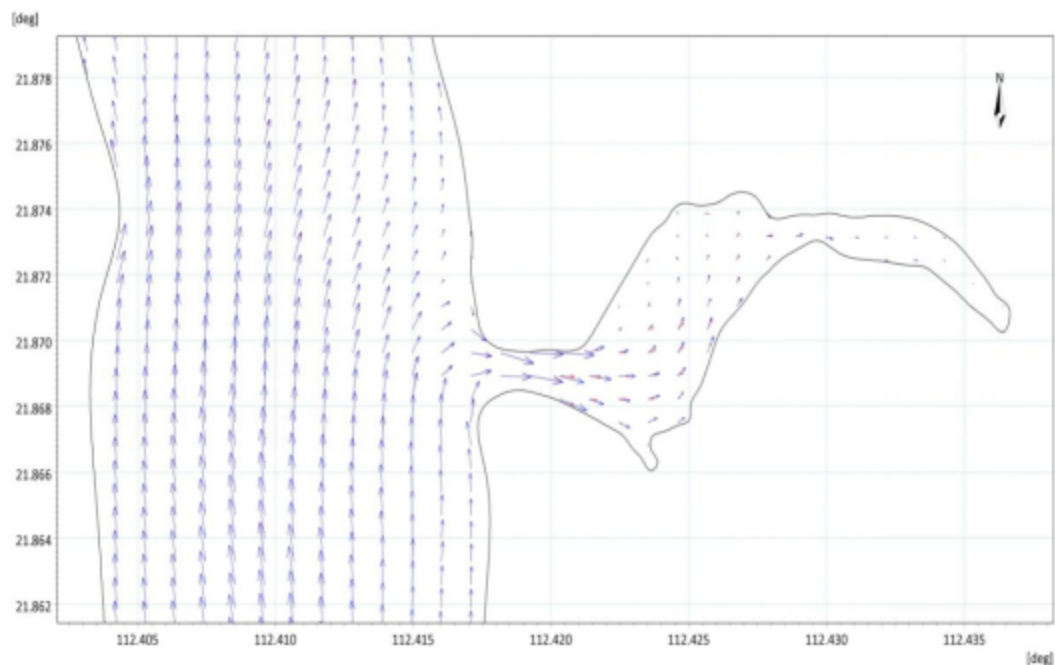
图 7.1.4-5 横山渔港工程海域涨急流场对比
