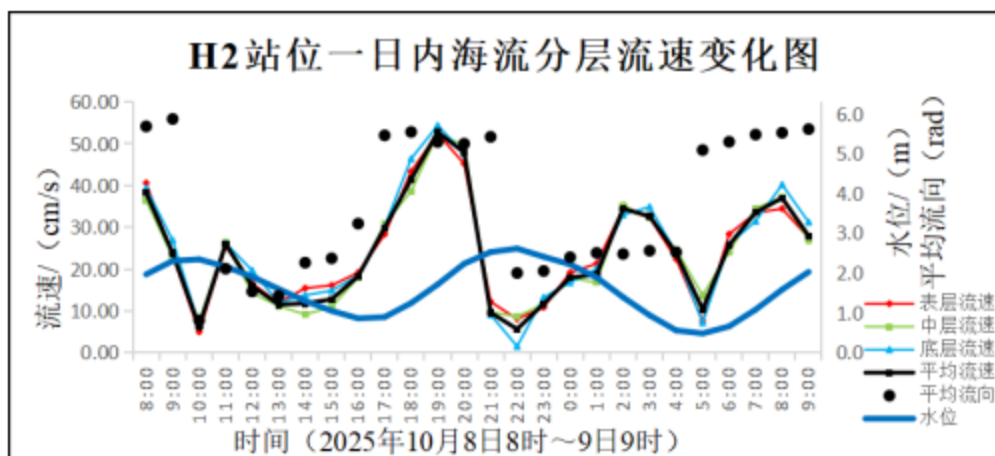
图 6.1.2-11 H2 站位海流分层流速变化图
