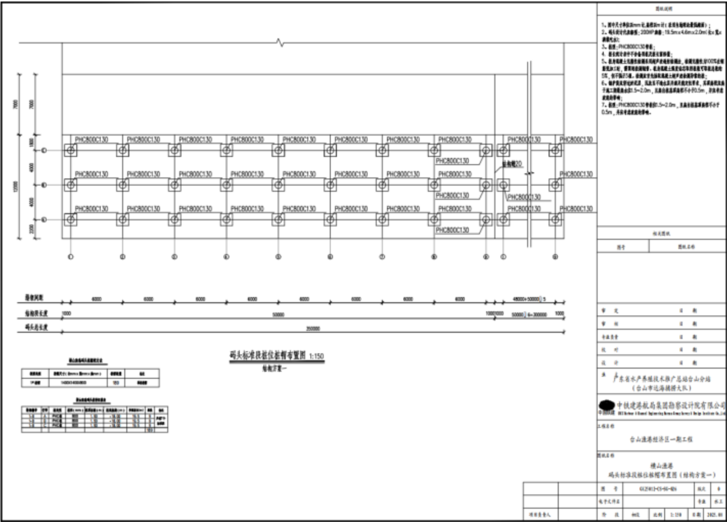
图 3.4.1-3 码头桩位布置图
