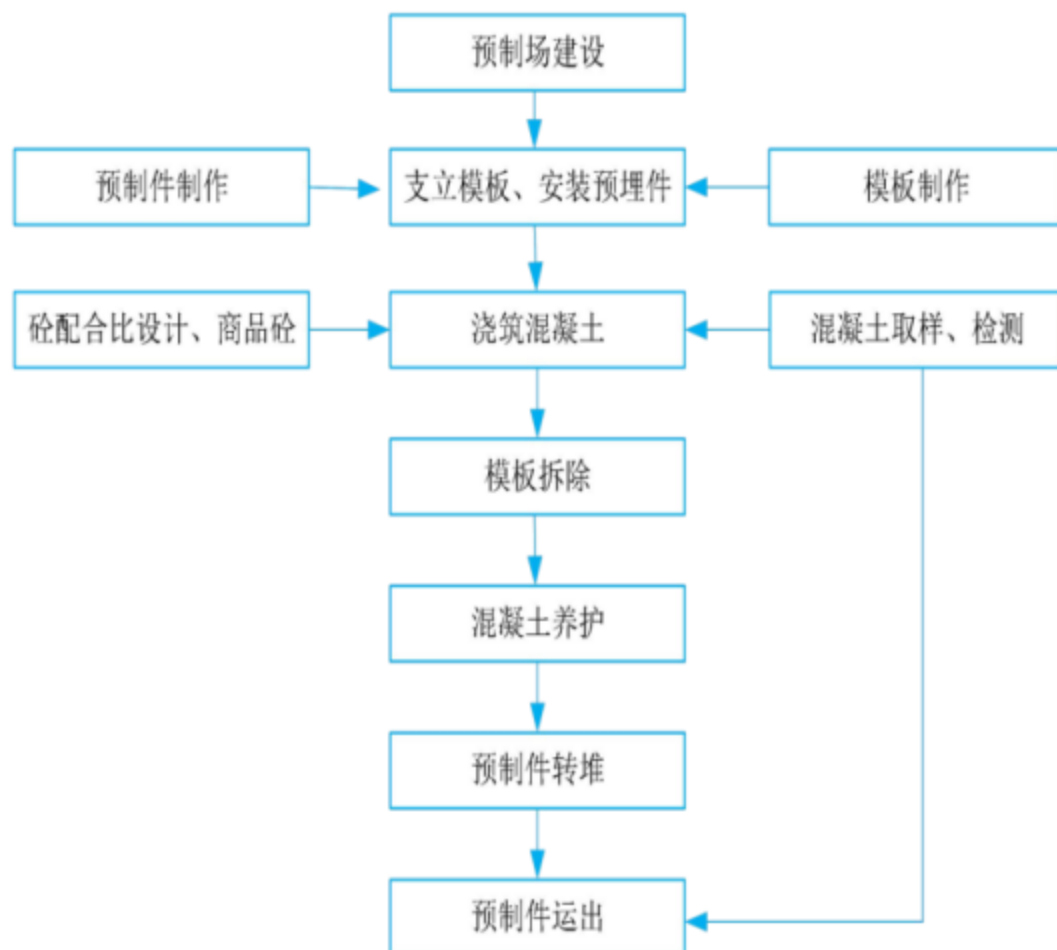
图 3.11.2-3 构件预制工艺流程图
