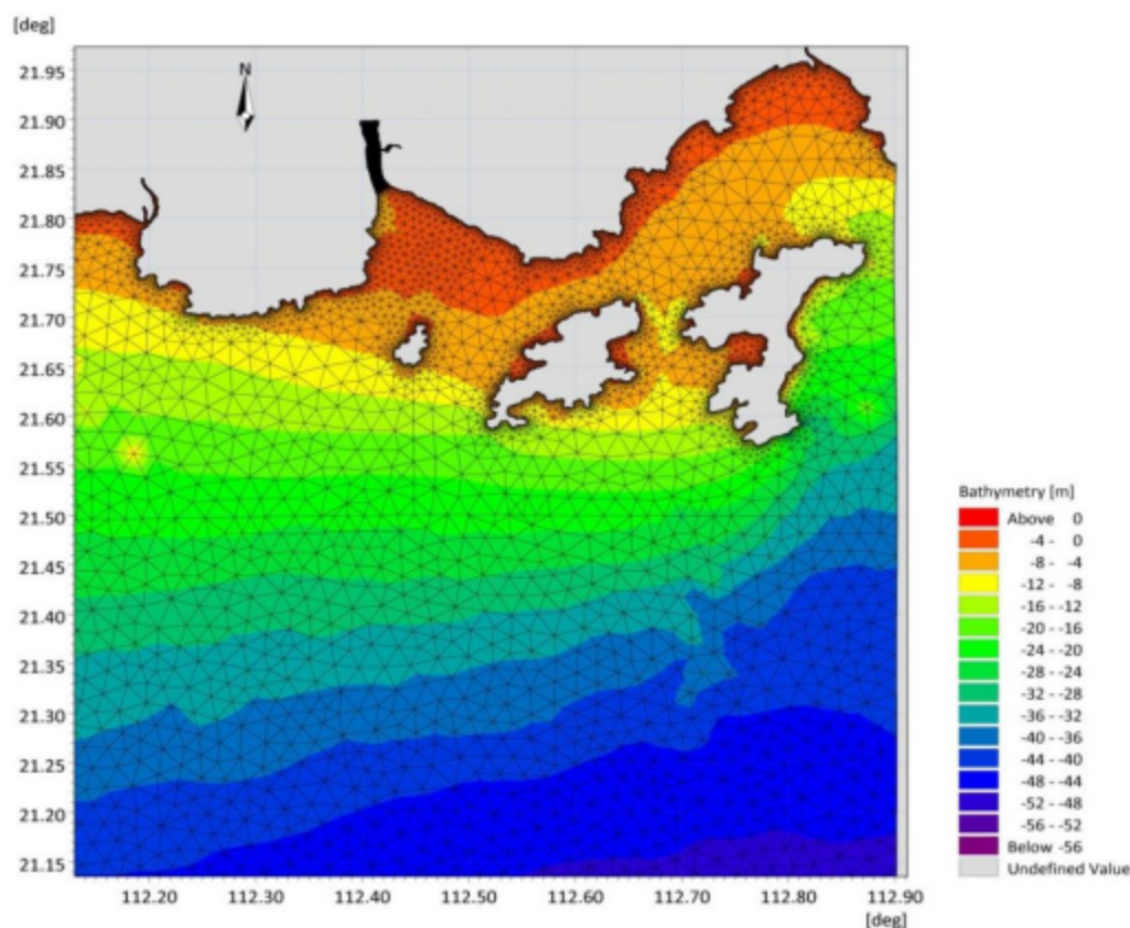
图 7.1.2-1 横山渔港大范围模型计算范围和网格剖分示意图
