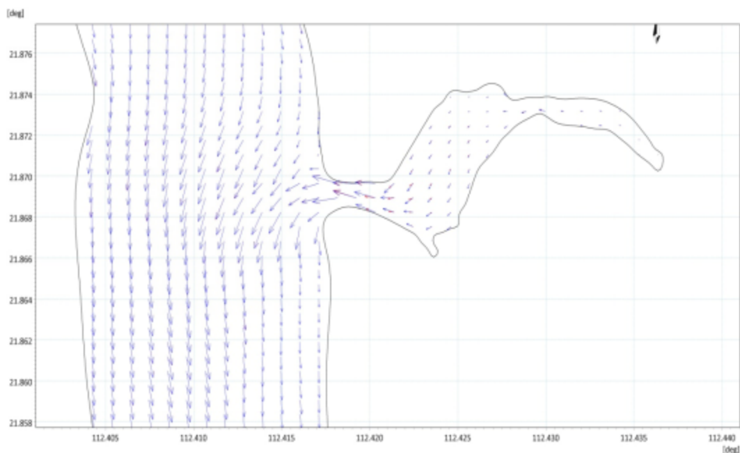
图 7.1.4-6 横山渔港工程海域落急流场对比（蓝色为工前，红色为工后）
