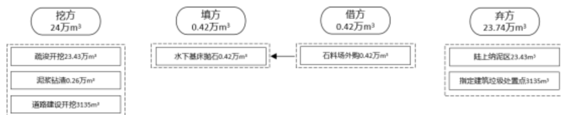
图 3.11.5-2 项目广海渔港（烽火角港区）土石方平衡图
