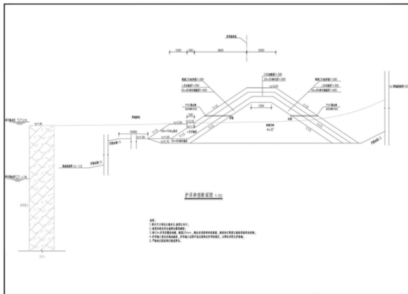
图 3.4.3-1 南侧护岸典型断面图
