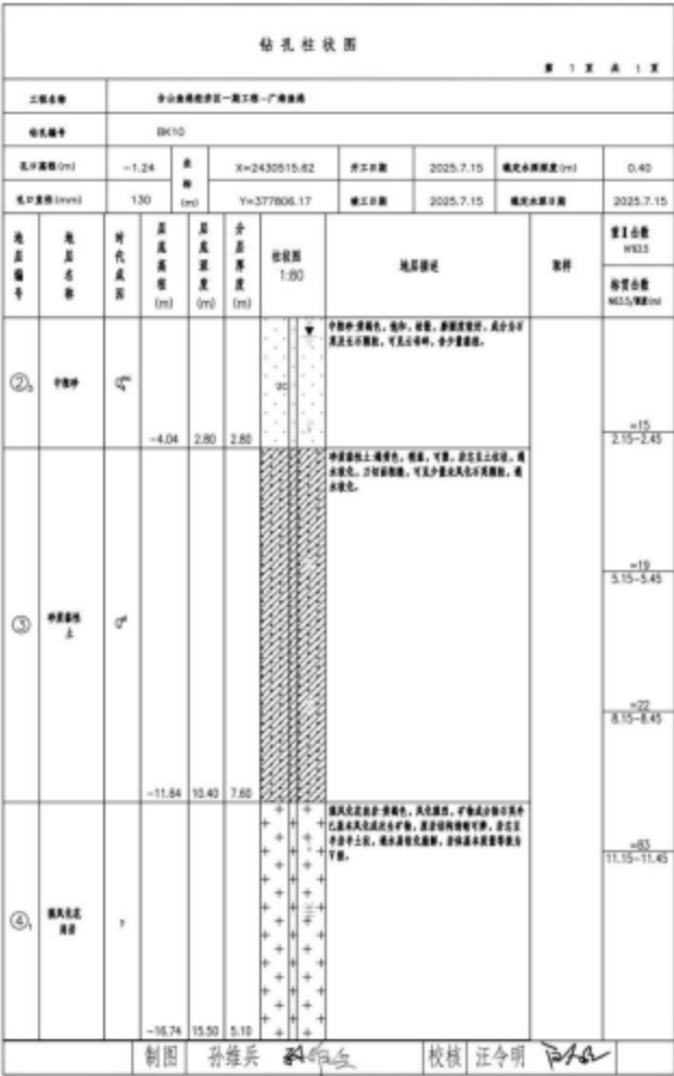
图 5.1.4-8b 广海渔港(烽火角港区)钻孔柱状图
