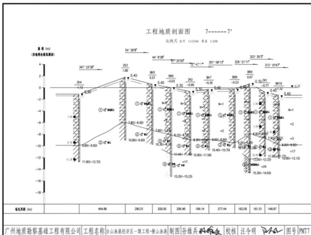
图 5.1.4-4e 工程地质剖面图
