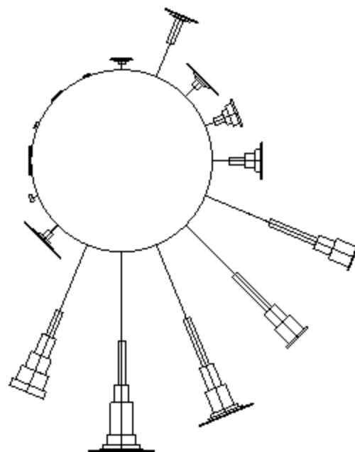
图 6.1.1-4 临时站年 H_{1/10} 波高玫瑰图
