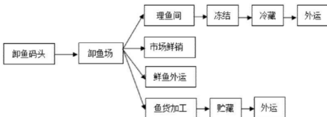
图 3.10-3 鱼货生产工艺流程图
