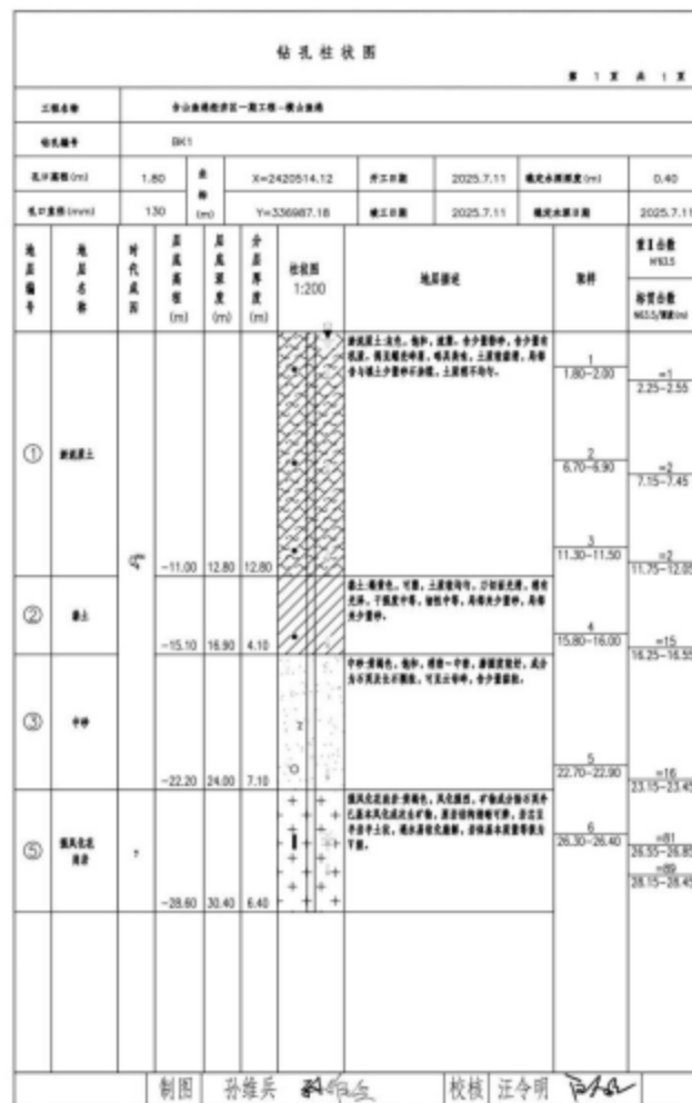
图 5.1.4-5a 项目横山渔港钻孔柱状图
