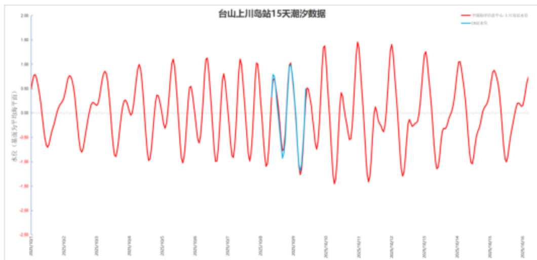
图 6.1.2-3 C4 潮位观测点与台山上川岛站潮位验证图
