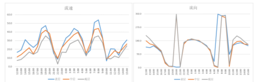
图 6.1.1-3d 海流矢量时间变化序列图 (S4 站)
