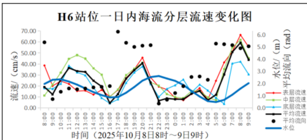
图 6.1.2-15 H6 站位海流分层流速变化图
