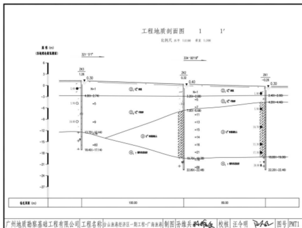
图 5.1.4-7a 工程地质剖面图
