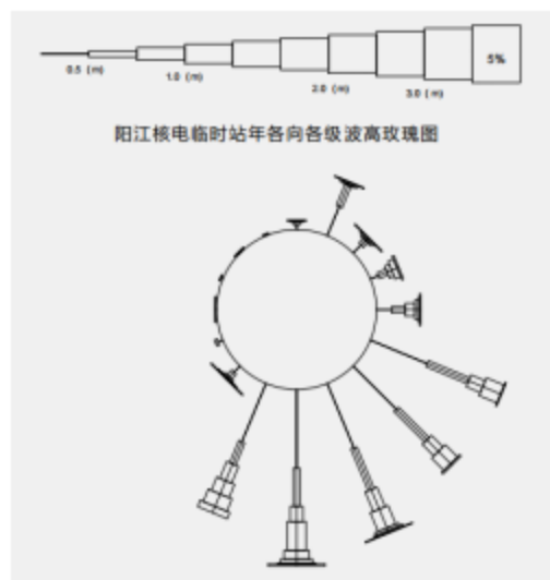
图 5.1.2-2 阳江核电临时站年 H_{1/10} 波高玫瑰图
