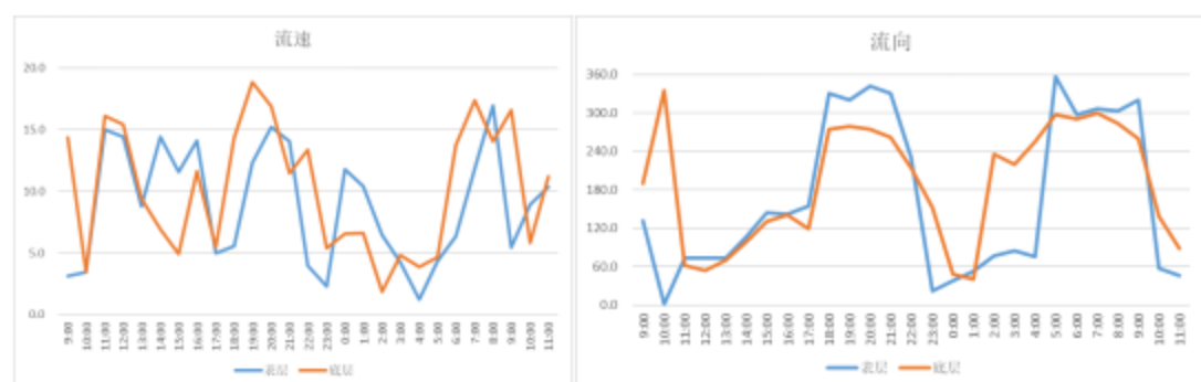
图 6.1.1-3f 海流矢量时间变化序列图 (S6 站)
