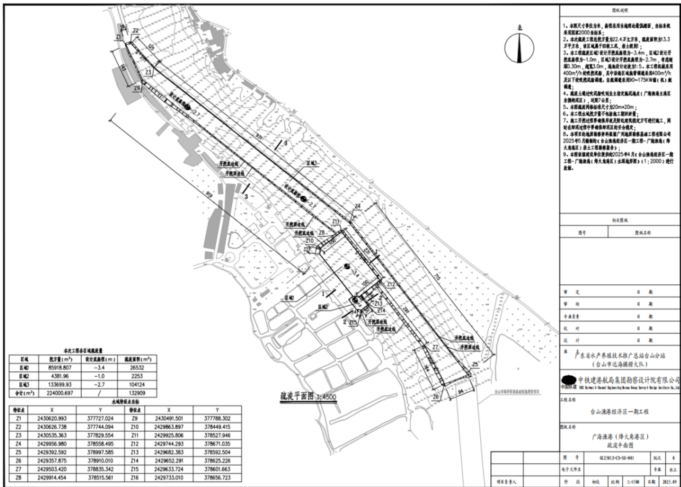
图 3.5.2-1 项目疏浚平面图
