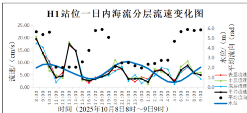
图 6.1.2-10 H1 站位海流分层流速变化图
