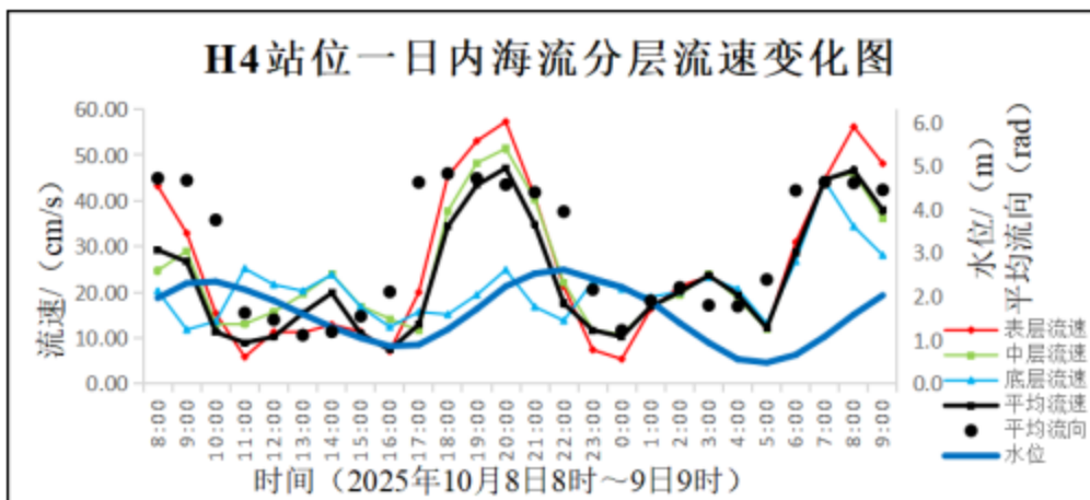
图 6.1.2-13 H4 站位海流分层流速变化图
