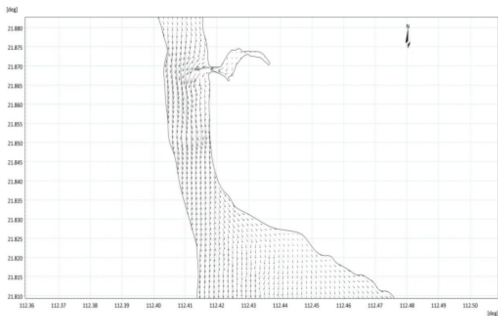
图 7.1.4-2 横山渔港工程前落急时刻流场图
