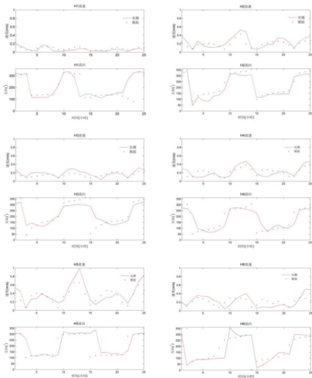
图 7.1.3-6 广海渔港（烽火角港区）流速流向验证图
