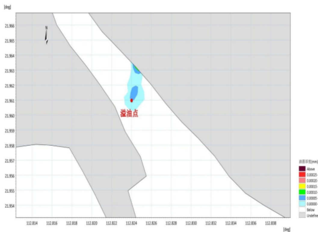
图 8.5.3-5 S 风向、2m/s 大潮涨初发生溢油 72 小时油膜扫海范围图
