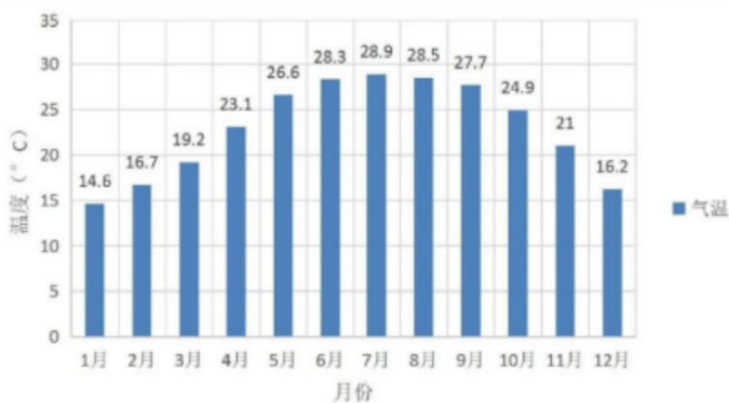
图 5.1.1-1 台山市月平均气温
