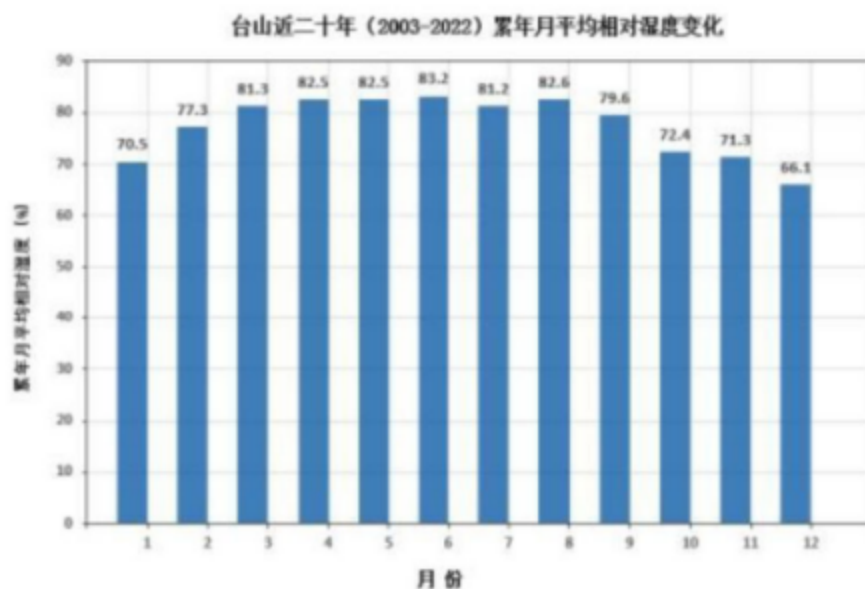
图 5.1.1-3 台山累年月平均相对湿度
