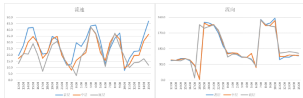
图 6.1.1-3b 海流矢量时间变化序列图 (S2 站)
