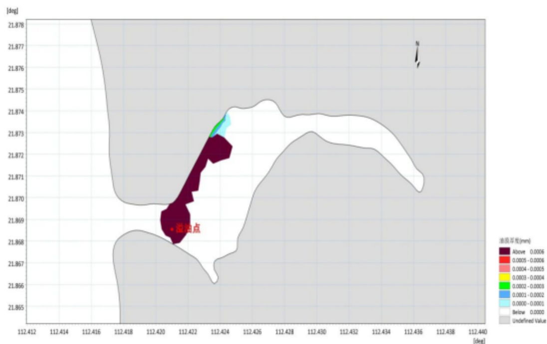
图 8.5.2--8 S 风向、13.8m/s 大潮落初发生溢油 72 小时油膜扫海范围图
