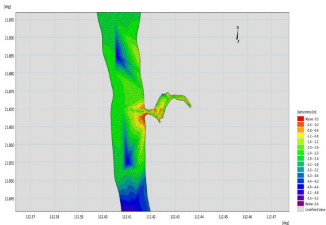
图 7.1.3-3 横山渔港工程区域计算网格和地形
