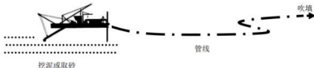
图 3.11.2-1 绞吸式挖泥船作业示意图
