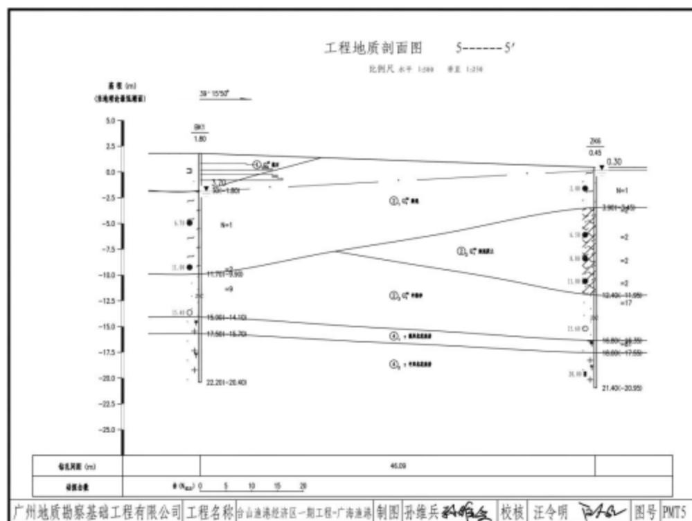
图 5.1.4-7e 工程地质剖面图
