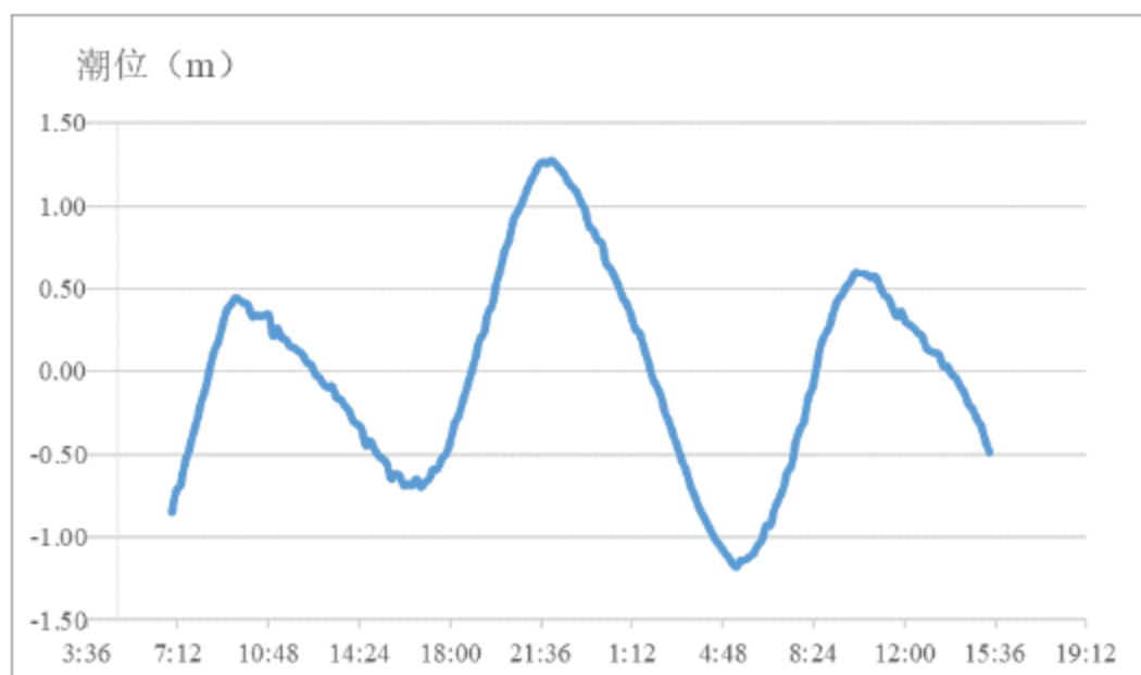
图 6.1.1-2 T1 站潮位过程曲线 (2021 年 3 月 13 日~3 月 14 日)
