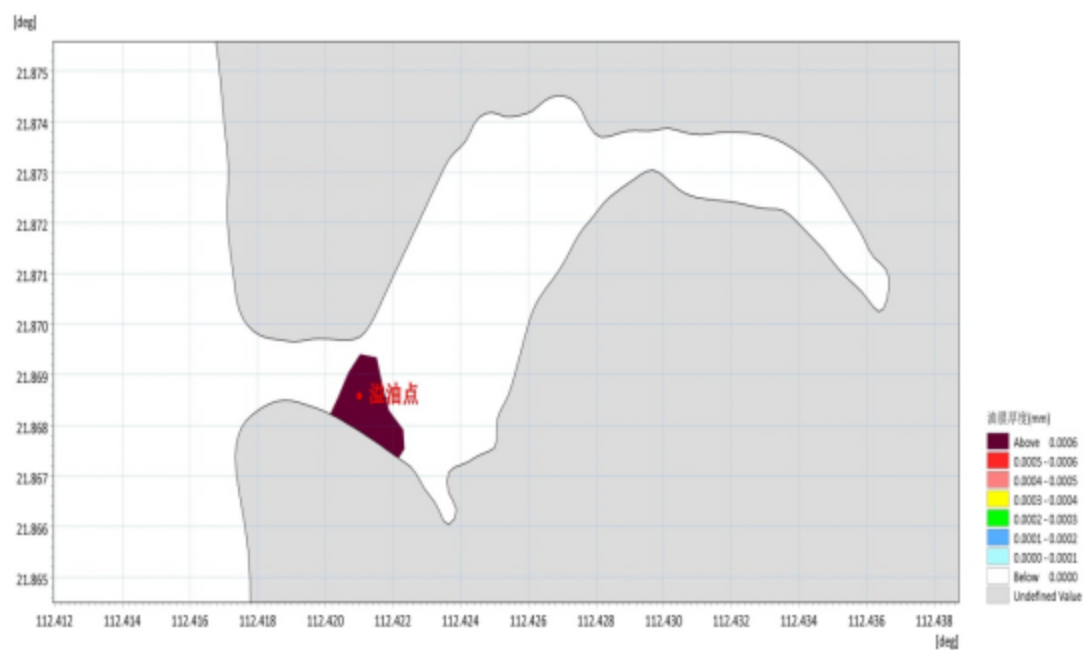
图 8.5.2-3 N 风向、2.7m/s 大潮涨初发生溢油 72 小时油膜扫海范围图
