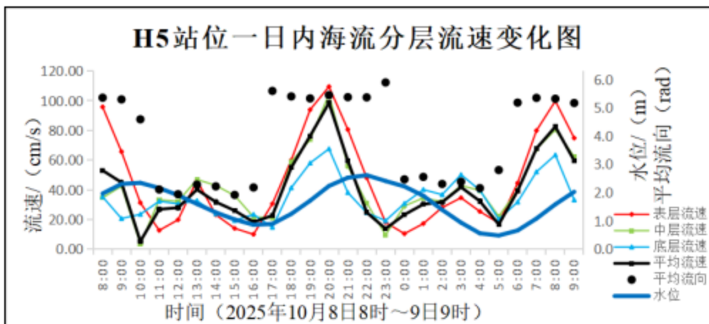
图 6.1.2-14 H5 站位海流分层流速变化图
