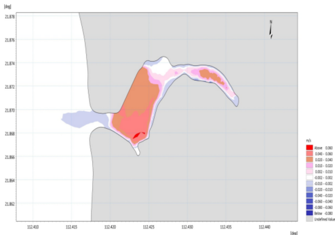
图 7.2.2-1 横山渔港工程区附近海床年冲淤变化平面分布图
