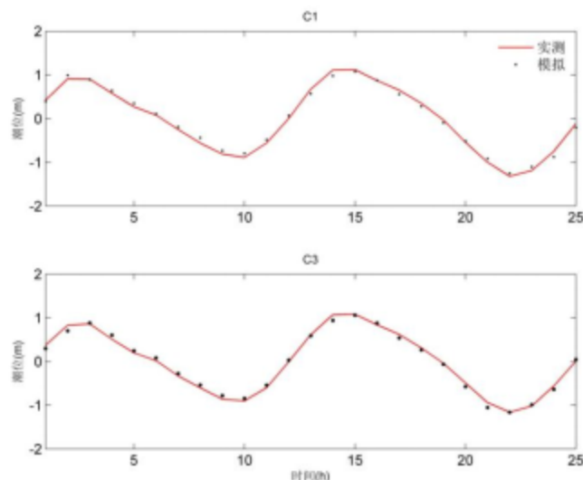
图 7.1.3-5 广海渔港（烽火角港区）潮位验证曲线（2025 年 10 月 8 日~9 日）
