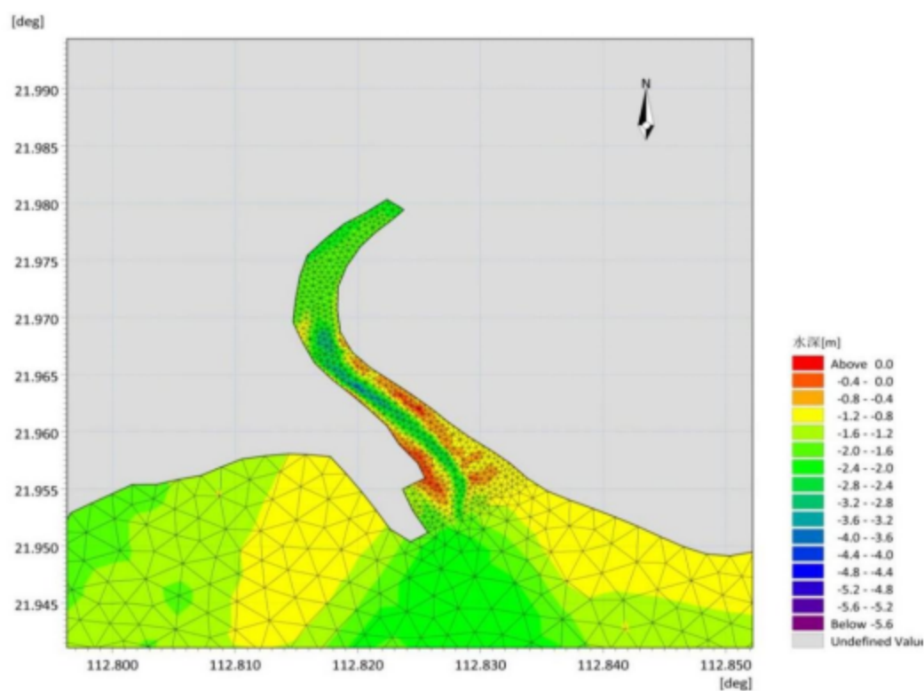
图 7.1.2-4 广海渔港（烽火角港区）项目海域网格剖分示意图
