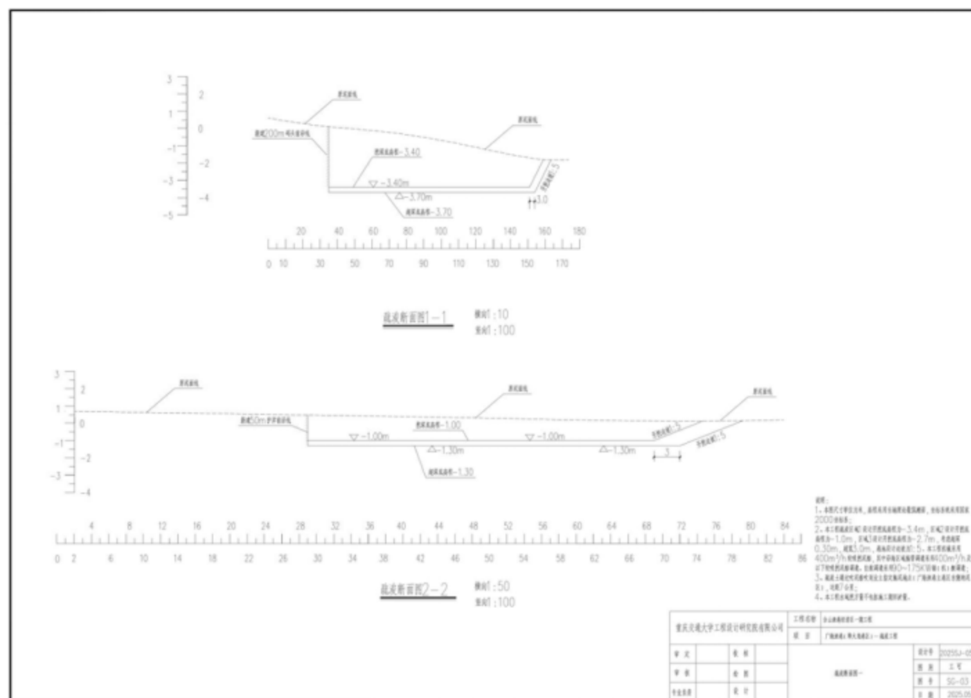
图 3.5.2-3 疏浚断面图一
