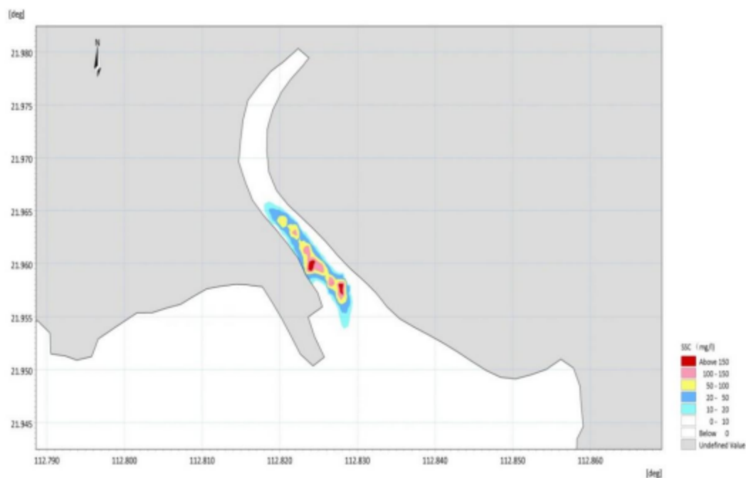
图 7.3.1-11 码头、护岸以及疏浚同时施工增量悬浮泥沙最大浓度平面分布
