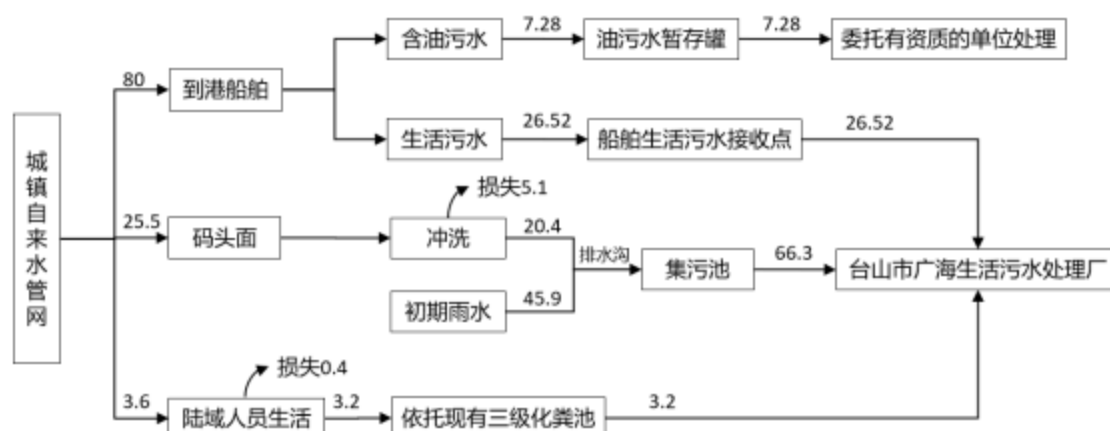
图 3.8.3-2 项目广海渔港（烽火角港区）水平衡图（单位： \text{m}^3/\text{d} ，初期雨水为 \text{m}^3/\text{次} ）
