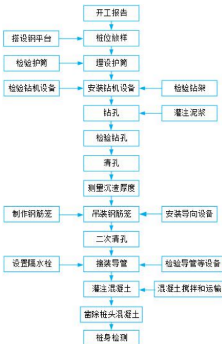
图 3.11.2-2 灌注桩施工工艺流程图
