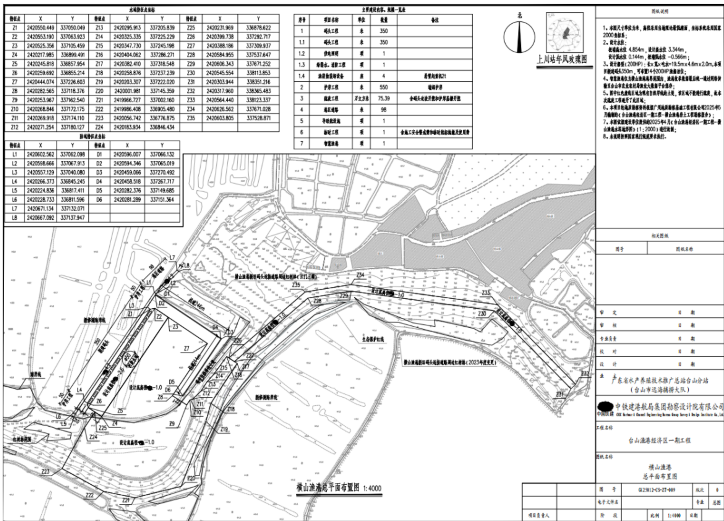
图 3.5.1-1 项目疏浚平面图
