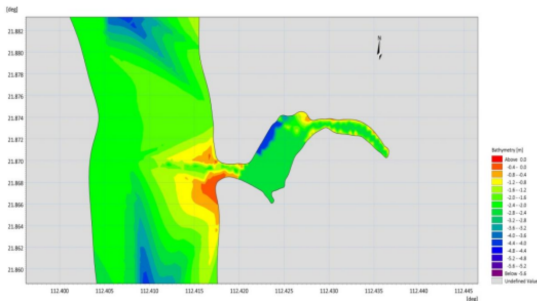
图 7.1.4-3 横山渔港工程区域工后地形图
