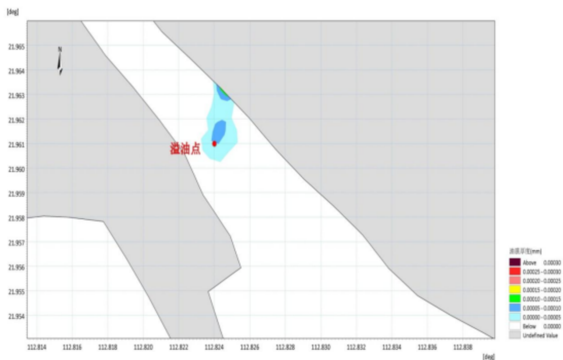
图 8.5.3-3 N 风向、2.7m/s 大潮涨初发生溢油 72 小时油膜扫海范围图
