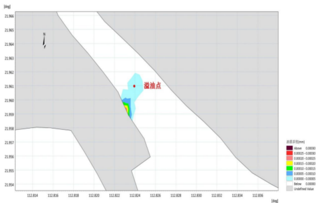
图 8.5.3-7 N 风向、2.7m/s 大潮落初发生溢油 72 小时油膜扫海范围图
