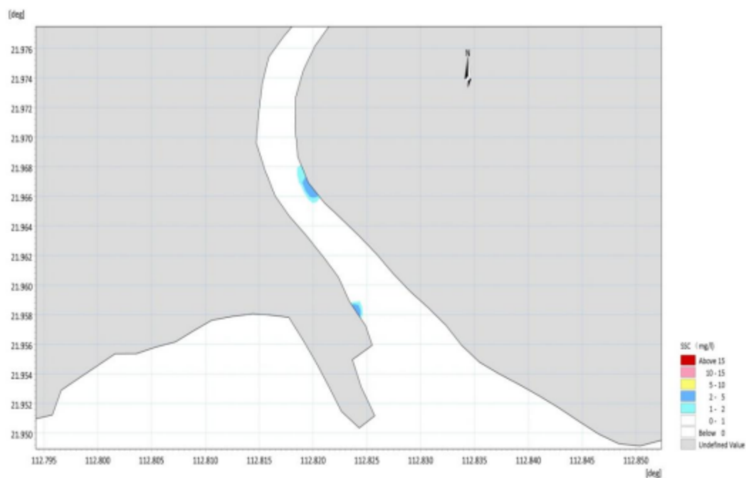
图 7.3.1-9 护岸单独施工增量悬浮泥沙最大浓度平面分布
