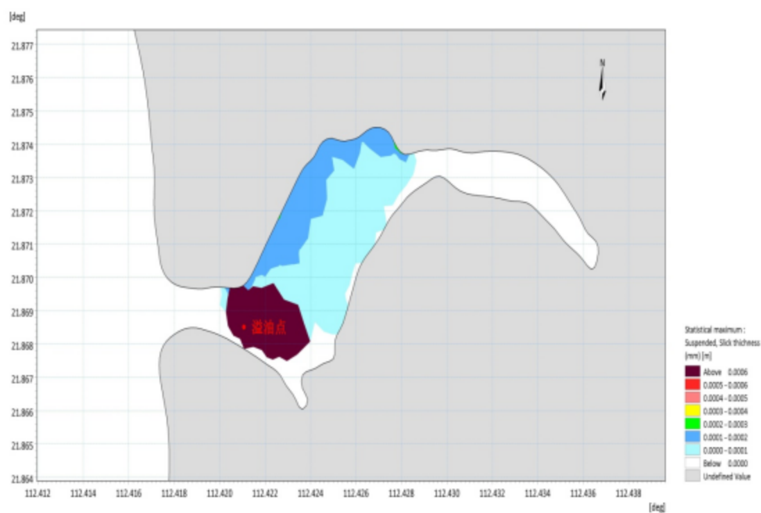
图 8.5.2-5 S 风向、2.7m/s 大潮涨初发生溢油 72 小时油膜扫海范围图
