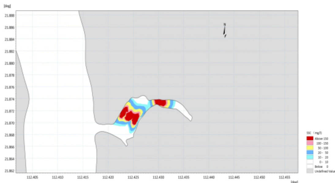
图 7.3.1-7 护岸单独施工增量悬浮泥沙最大浓度平面分布
