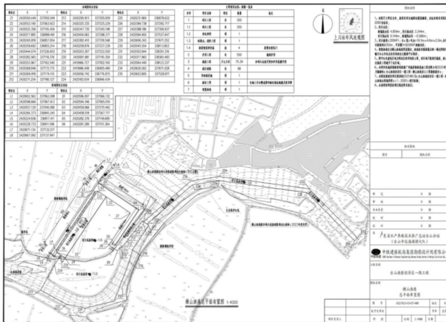
图 3.3.2-1 项目横山渔港总平面布置图
