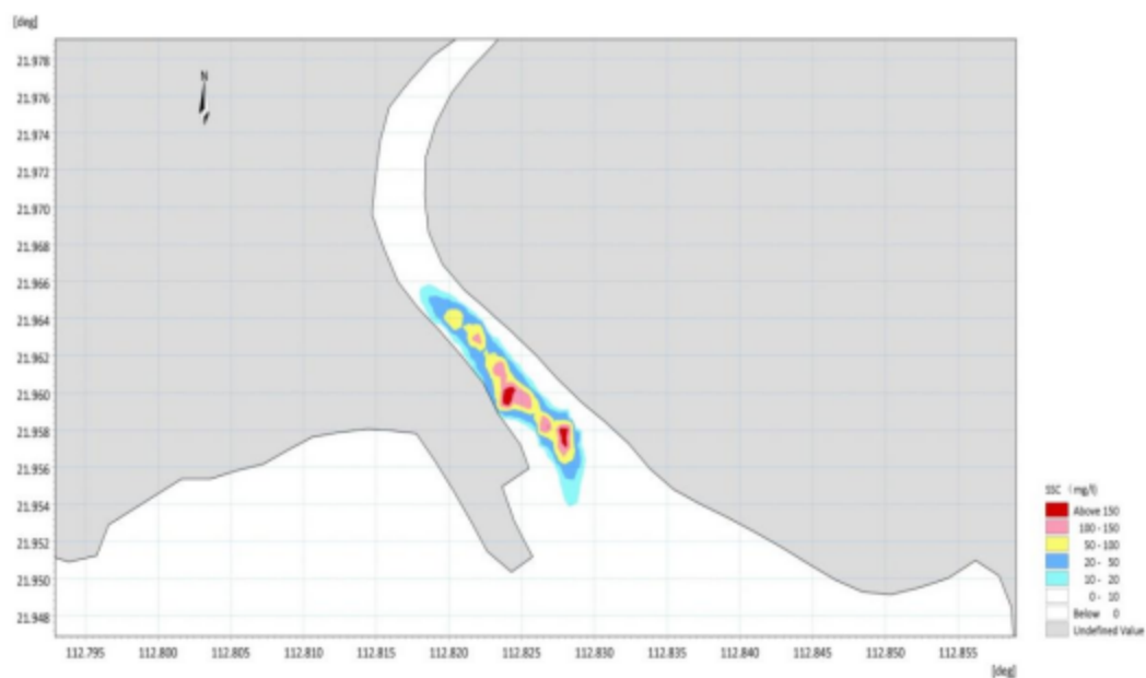
图 7.3.1-10 港池、航道疏浚单独施工增量悬浮泥沙最大浓度平面分布
