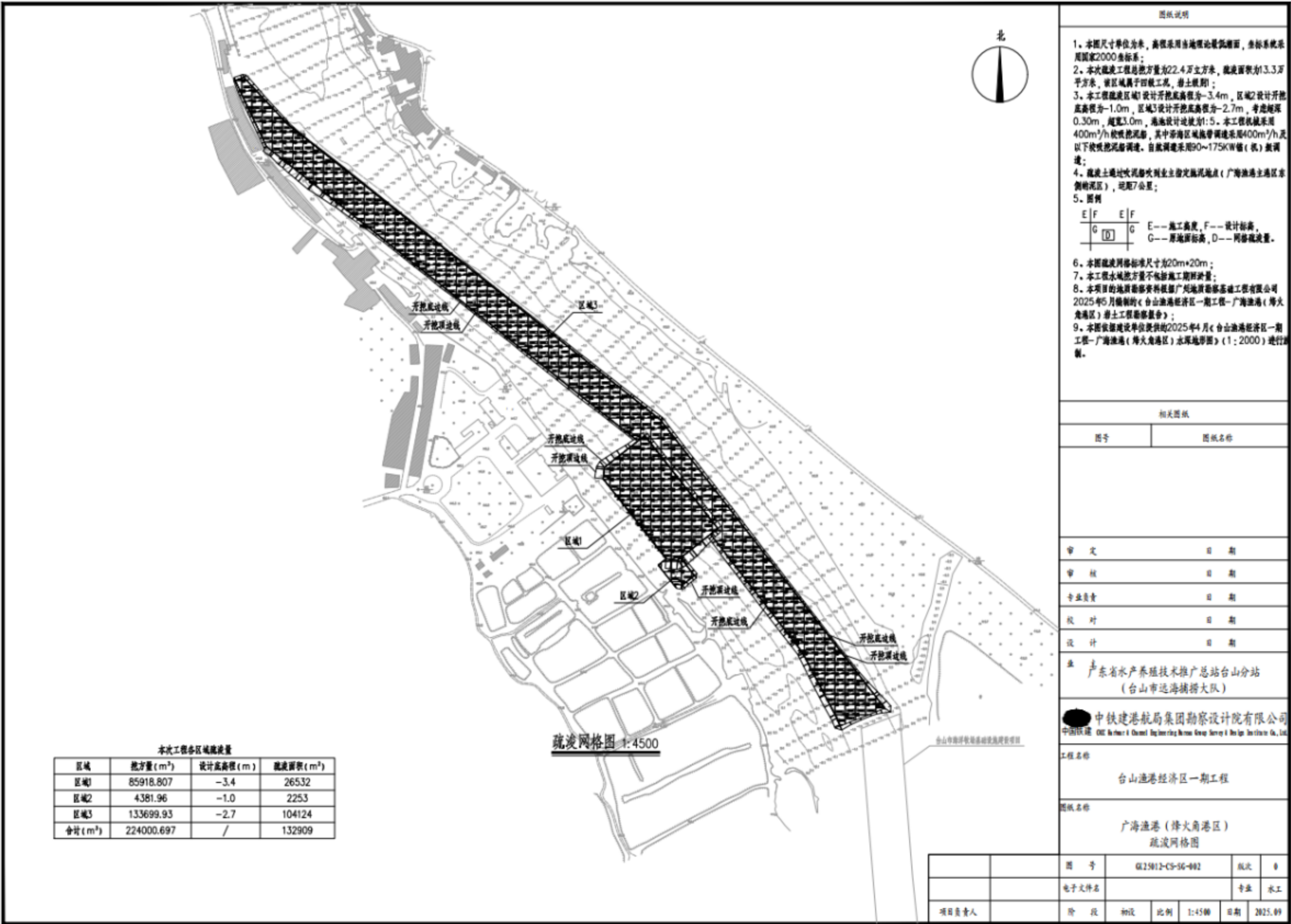
图 3.5.2-2 项目疏浚网格图
