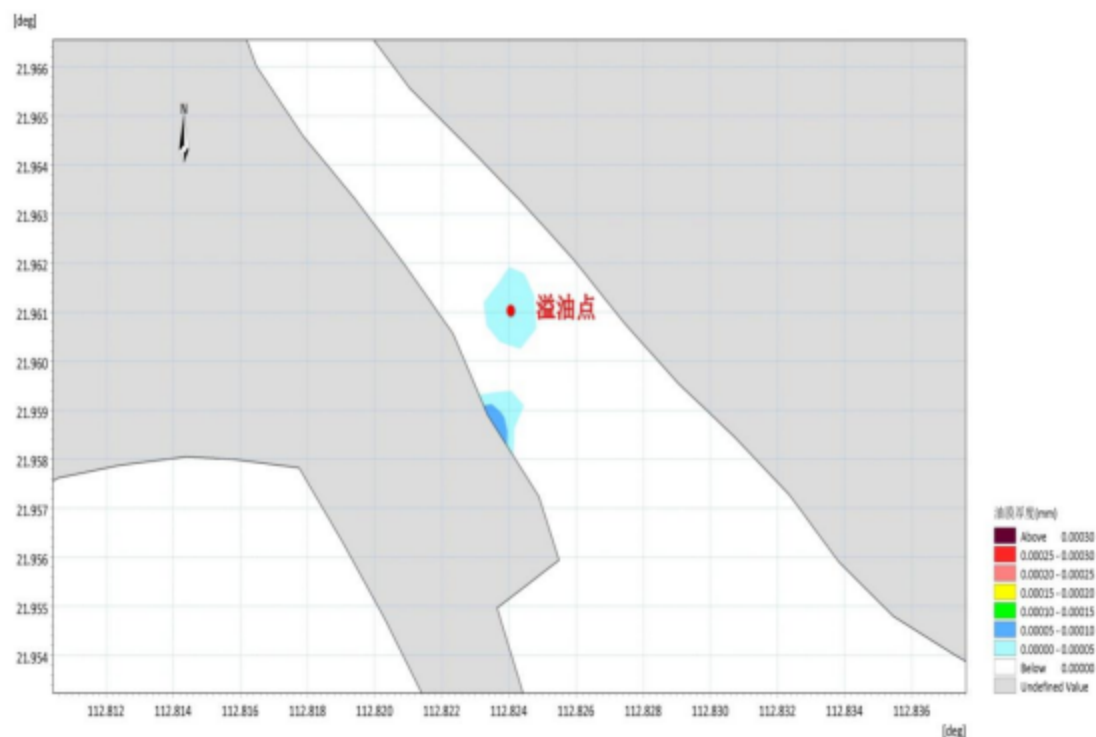
图 8.5.3-6 N 风向、13.8m/s 大潮落初发生溢油 72 小时油膜扫海范围图
