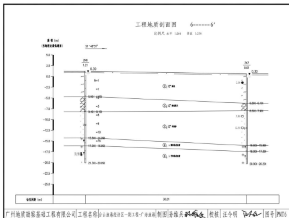
图 5.1.4-7f 工程地质剖面图
