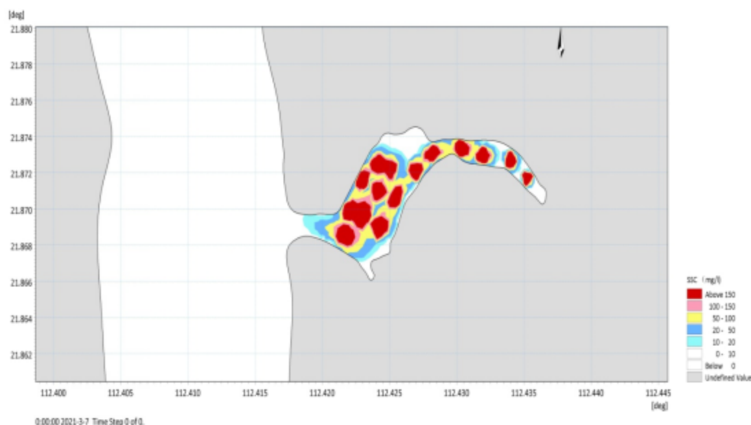
图 7.3.1-6 码头单独施工增量悬浮泥沙最大浓度平面分布
