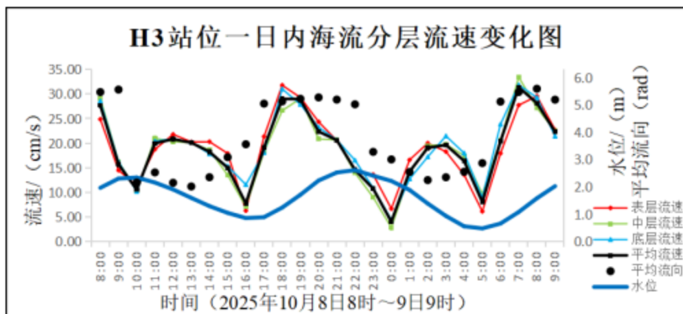
图 6.1.2-12 H3 站位海流分层流速变化图
