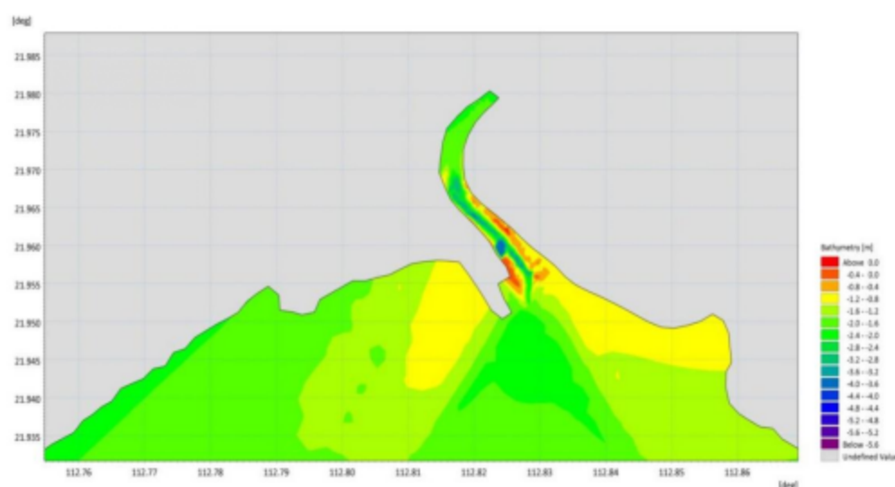
图 7.1.4-9 广海渔港（烽火角港区）工程区域工程后地形图
