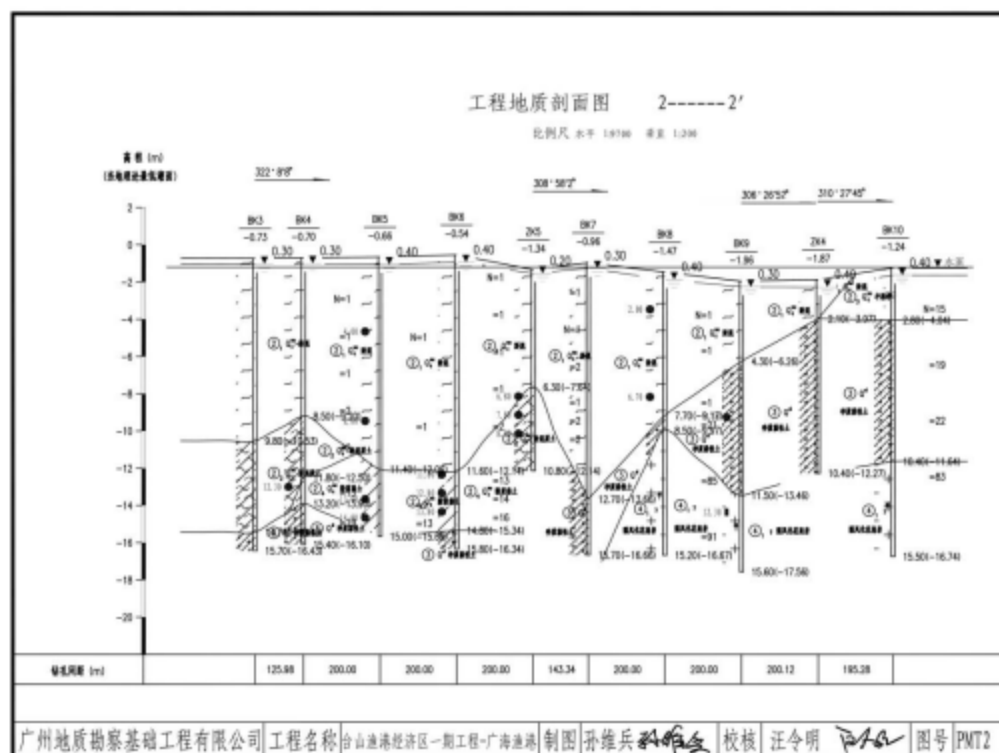
图 5.1.4-7b 工程地质剖面图
