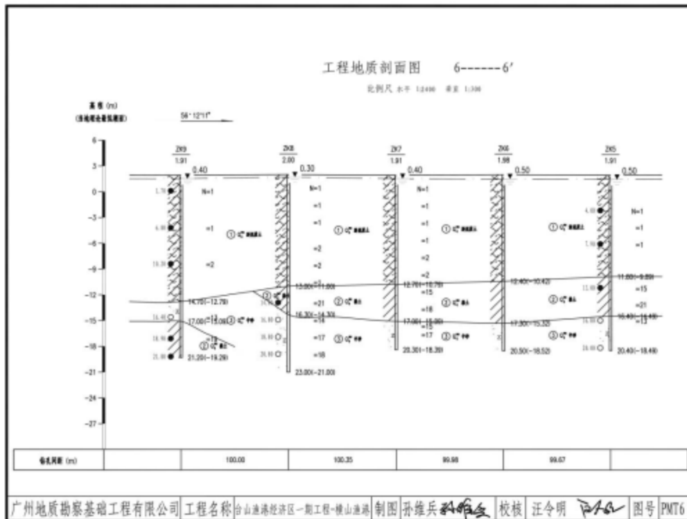
图 5.1.4-4d 工程地质剖面图
