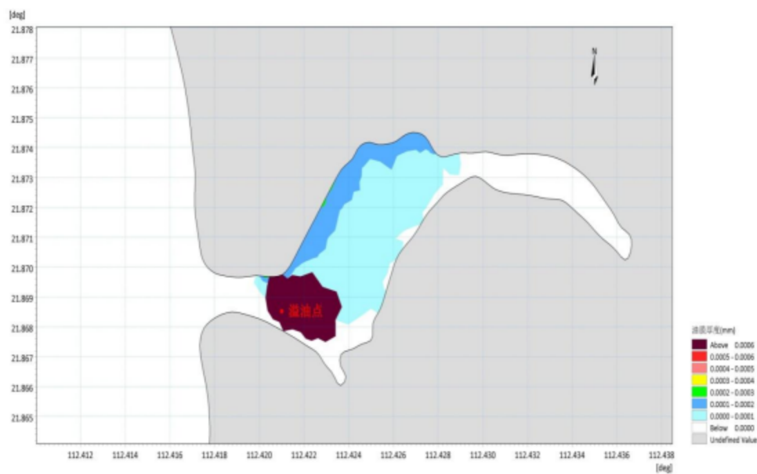
图 8.5.2-9 S 风向、2m/s 大潮落初发生溢油 72 小时油膜扫海范围图
