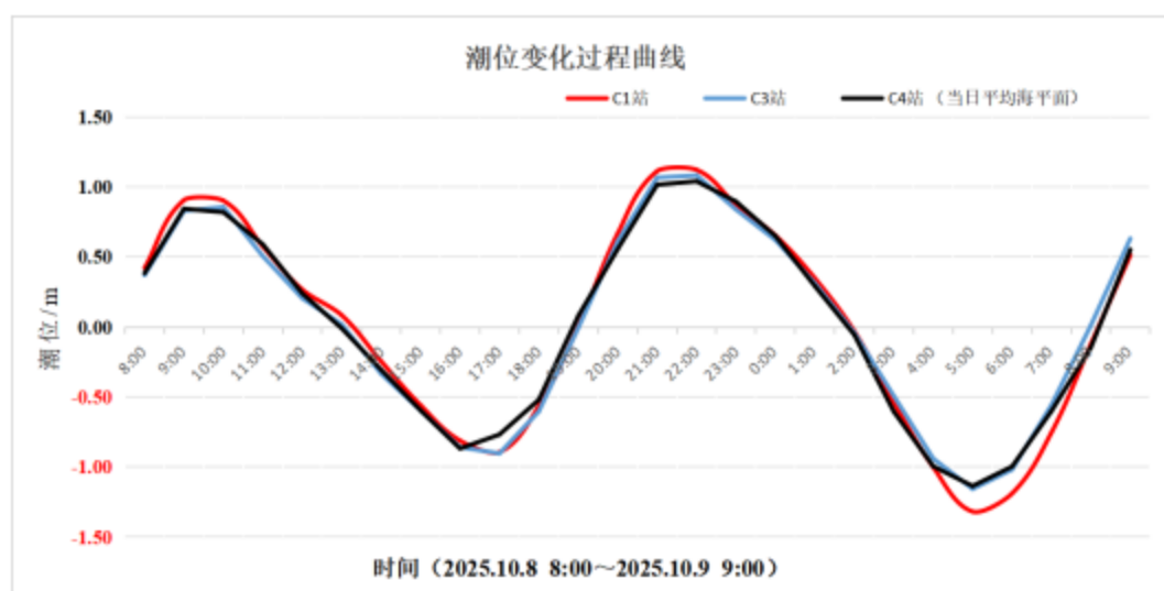
图 6.1.2-2 C1、C3、C4 站位一日内潮位过程曲线图
