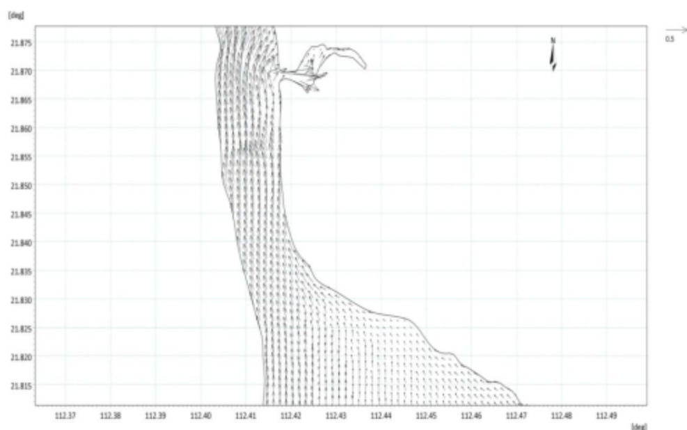
图 7.1.4-1 横山渔港工程前涨急时刻流场图
