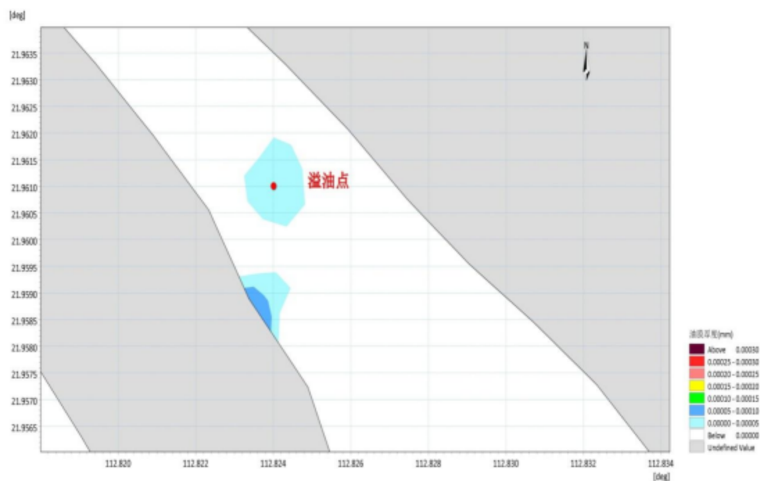
图 8.5.3-2 N 风向、13.8m/s 大潮涨初发生溢油 72 小时油膜扫海范围图
