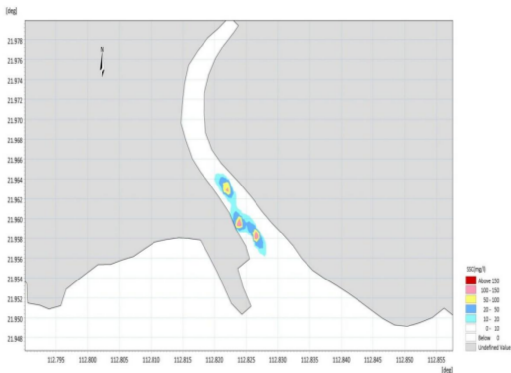
图 7.3.1-12 港池、航道疏浚施工典型工况增量悬浮泥沙最大浓度平面分布
