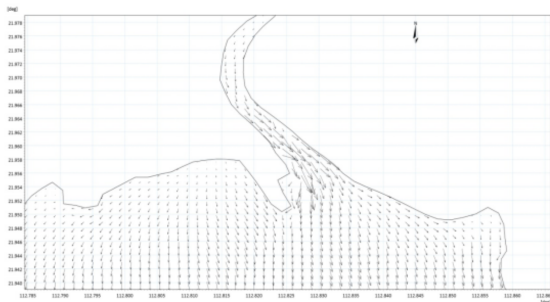
图 7.1.4-8 广海渔港（烽火角港区）附近海域现状落急流场图
