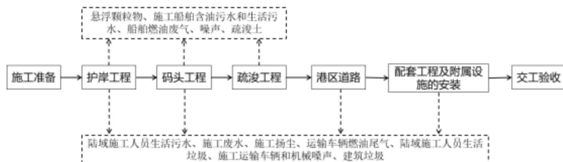
图 4.1.1-1 项目横山渔港施工过程主要产污环节示意图
