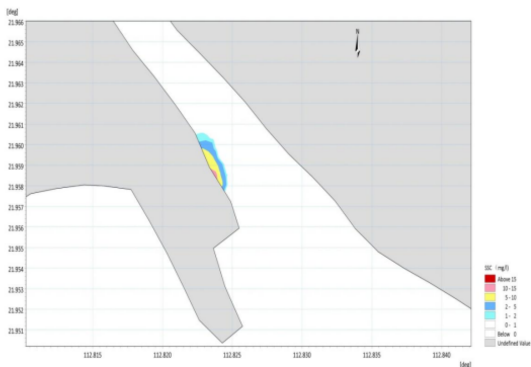
图 7.3.1-8 码头单独施工增量悬浮泥沙最大浓度平面分布
