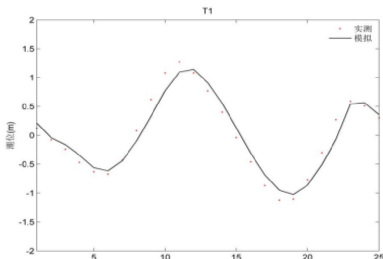
图 7.1.3-3 横山渔港潮位验证曲线（2021 年 3 月 13 日~14 日）
