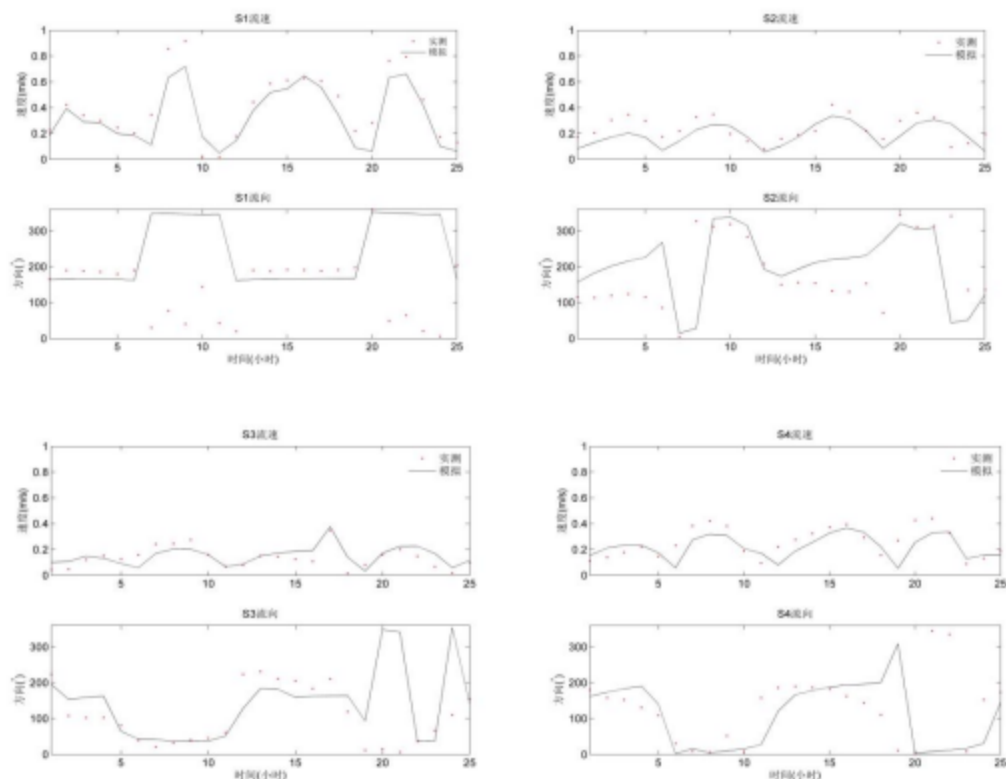
图 7.1.3-4 横山渔港流速流向验证图（—表示模拟值，·表示实测值）
