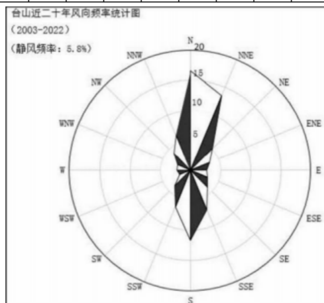
图 5.1.1-2 台山气象站风向玫瑰图
