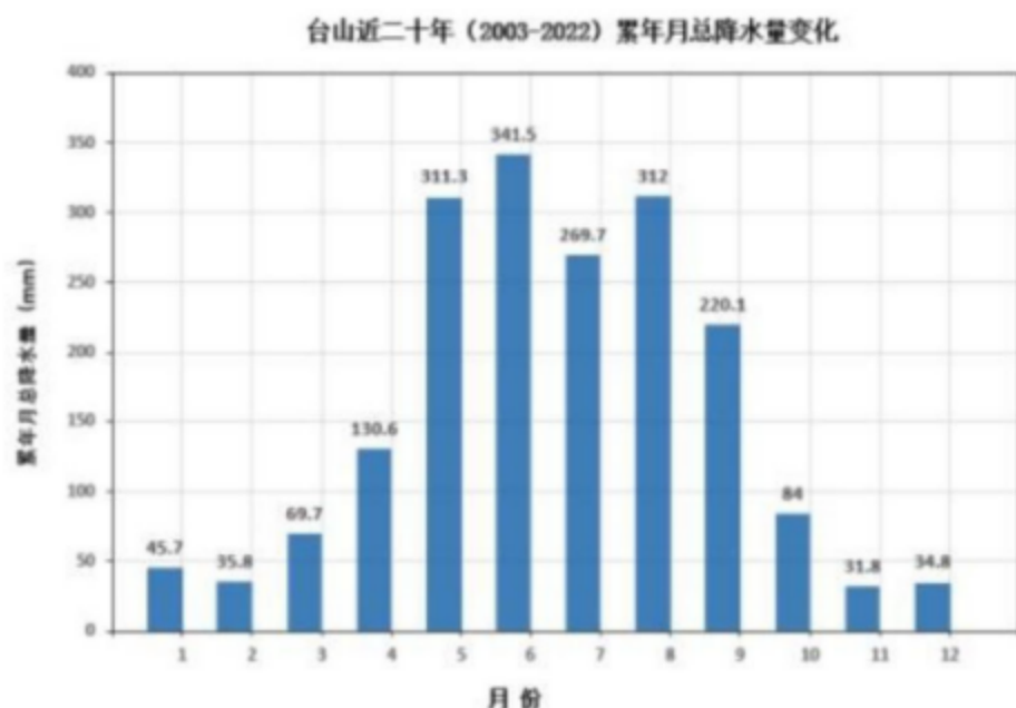
图 5.1.1-2 台山累年月总降水量
