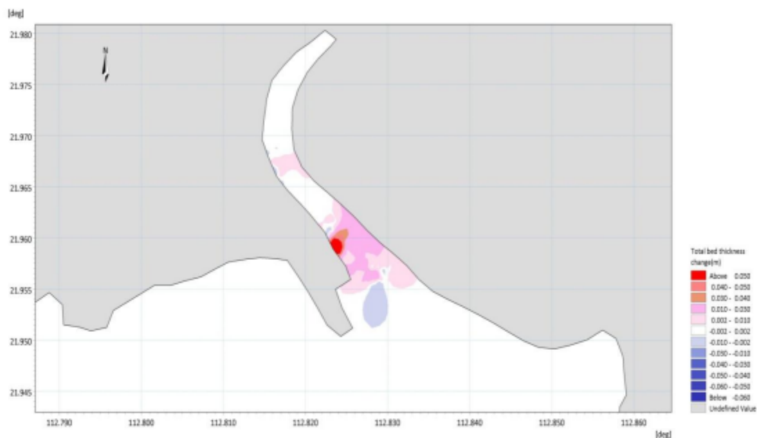
图 7.2.2-2 广海渔港（烽火角港区）工程区附近海床年冲淤变化平面分布图
