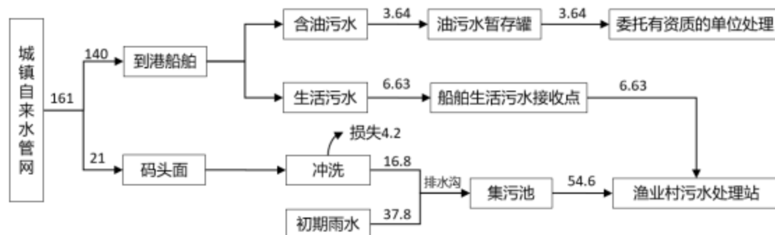
图 3.8.3-1 项目横山渔港水平衡图（单位： \text{m}^3/\text{d} ，初期雨水为 \text{m}^3/\text{次} ）
