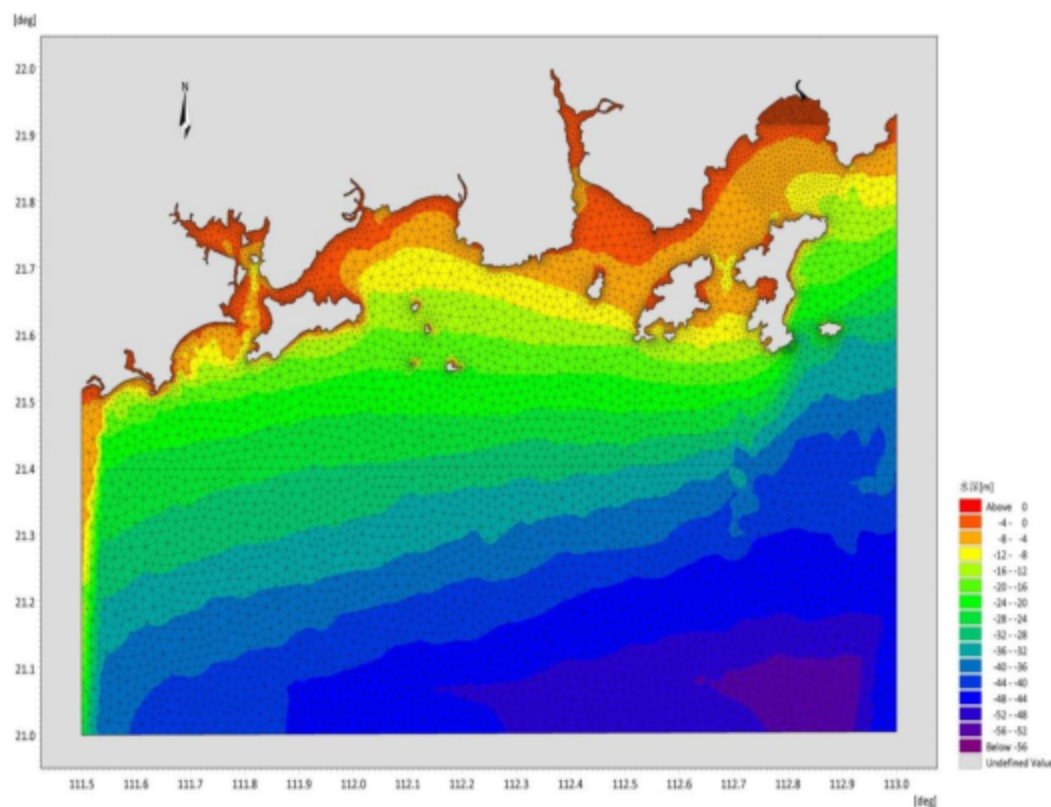
图 7.1.2-2 广海渔港（烽火角港区）大范围模型计算范围和网格剖分示意图
