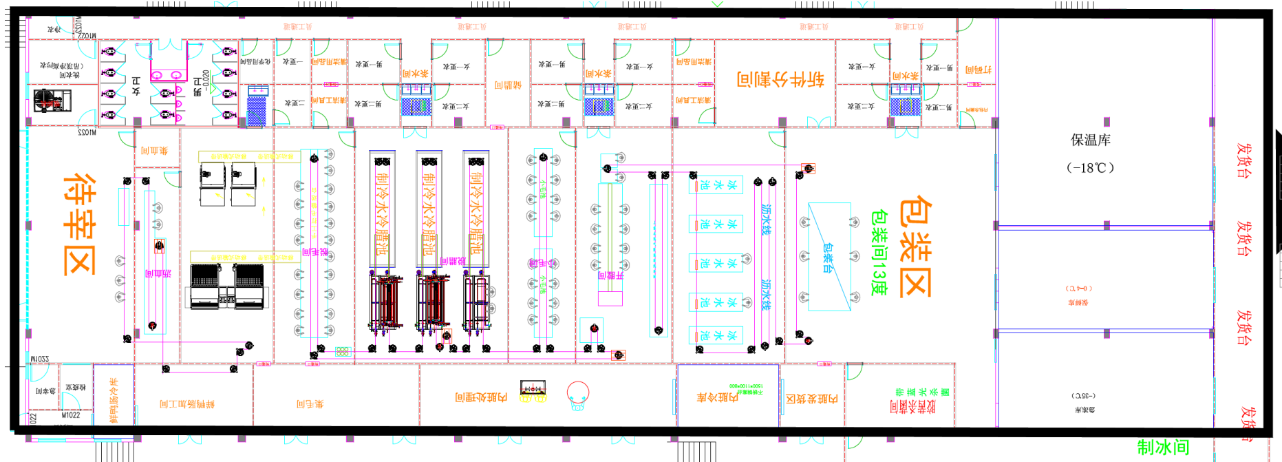
图 3.2-3 项目屠宰车间 1 之一、二、三分区首层平面布局图（局部放大）
