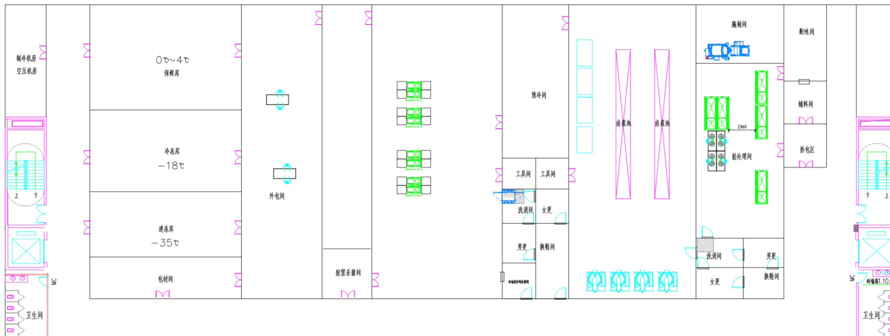
图 3.2-7 熟食车间 1 二层平面布置图
