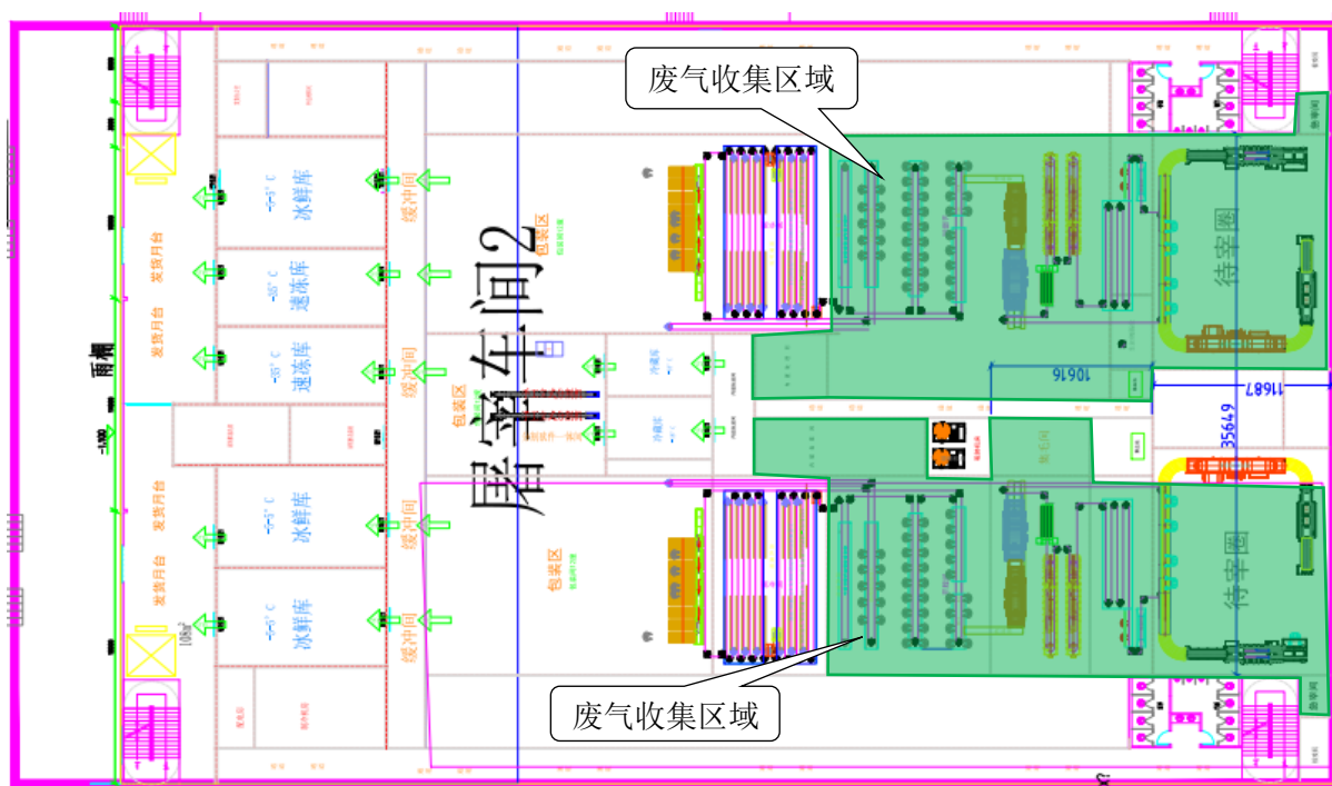
图 3.6-3 屠宰车间 2 废气收集区域示意图
