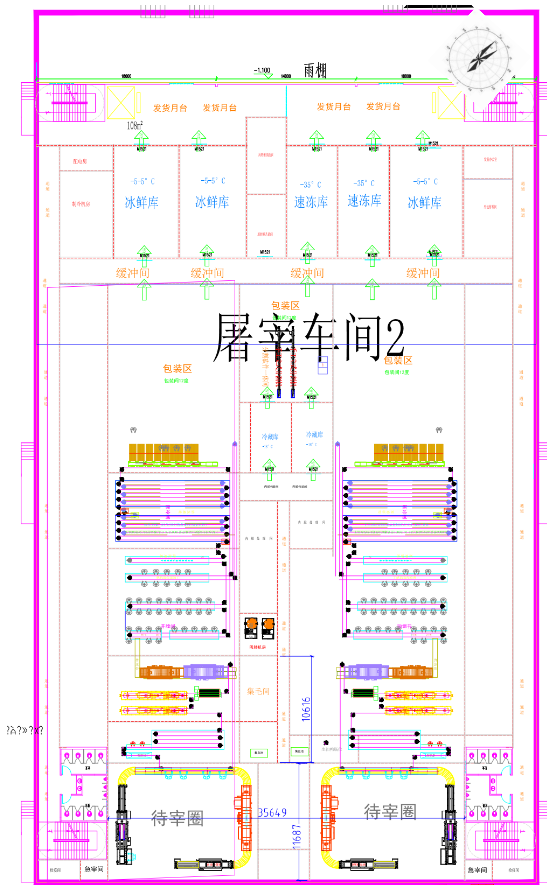
图 3.2-4 屠宰车间 2 首层平面布置图
