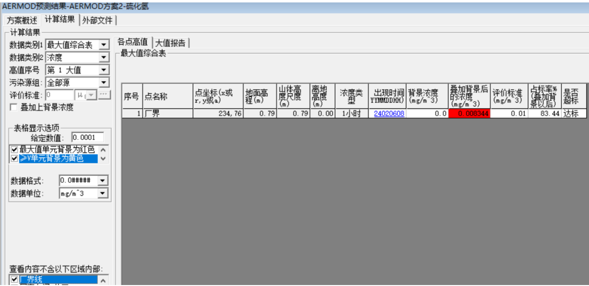
图5.2-8厂界氨气浓度预测结果
