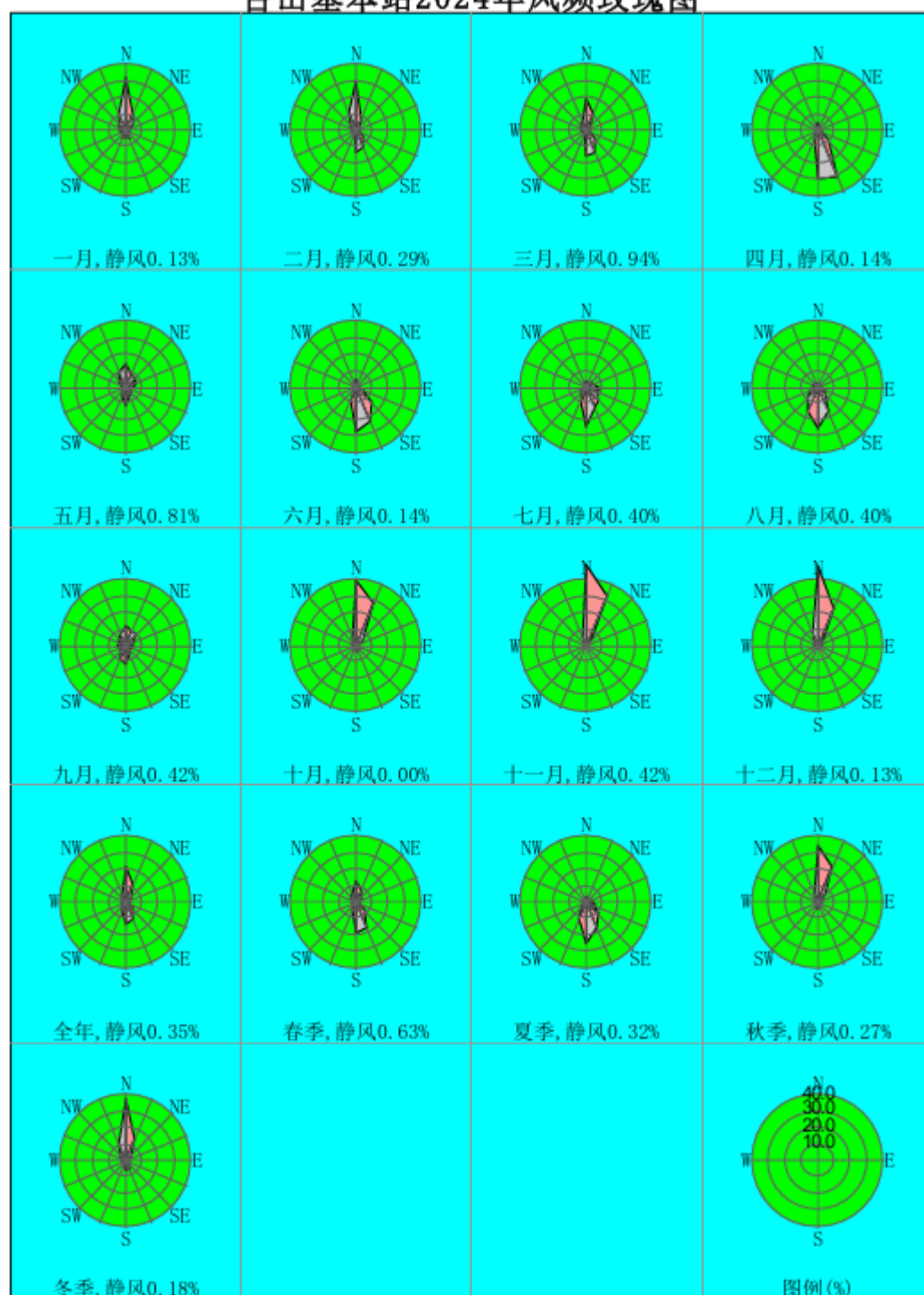
图 5.2-5 台山市 2024 年地面风向玫瑰图
