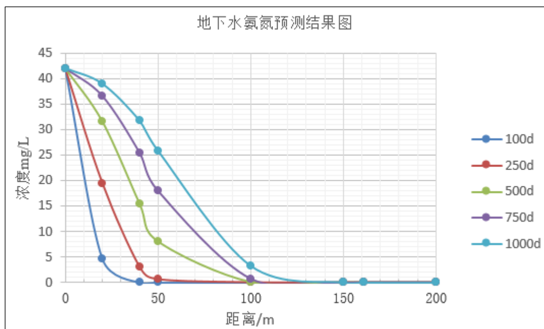
图 5.4-3 地下水氨氮预测结果图
