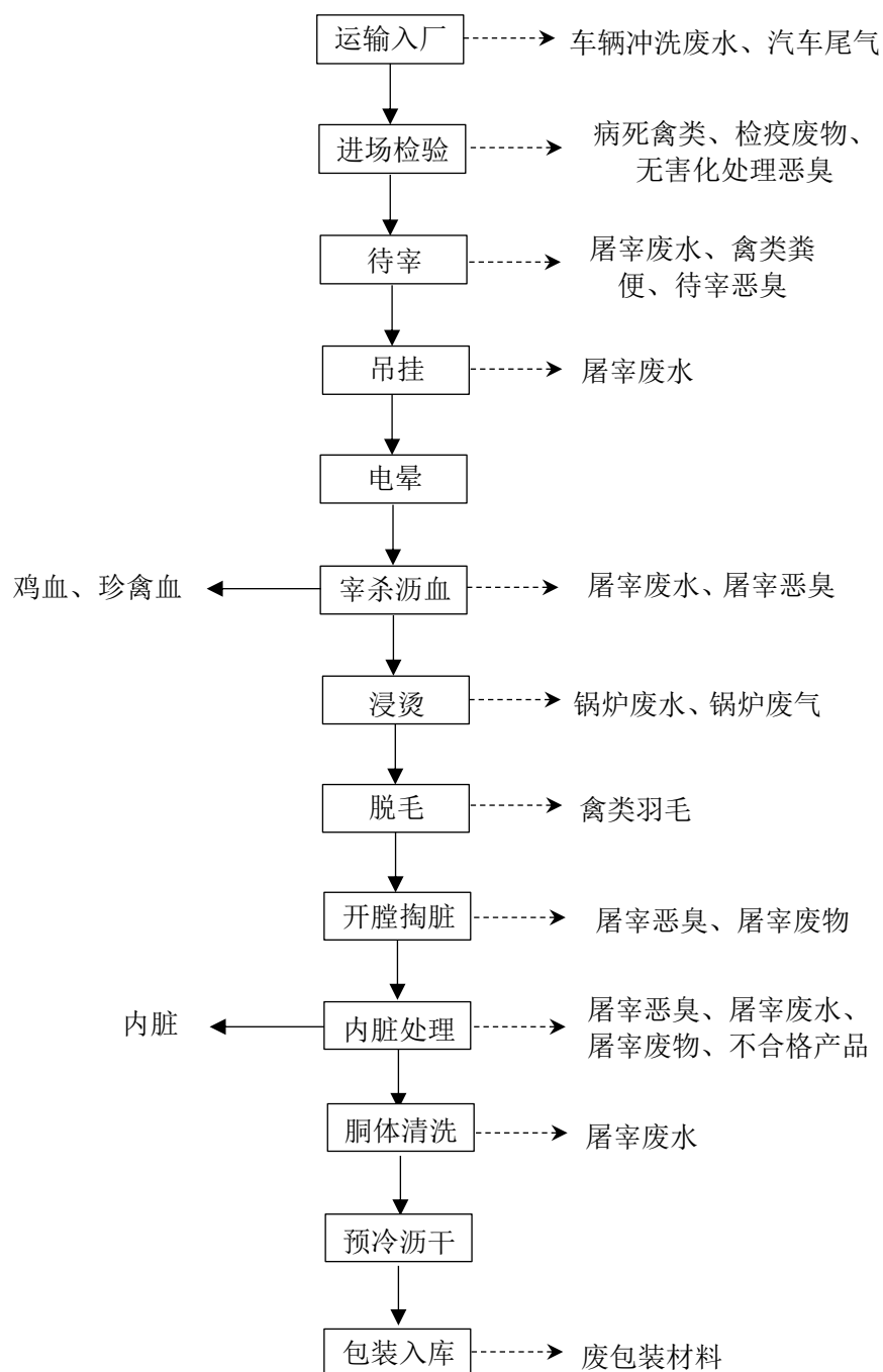
图 3.3-1 鸡、珍禽（鸽、鹌鹑、鹌鹑）屠宰加工生产工艺流程及产污节点图
