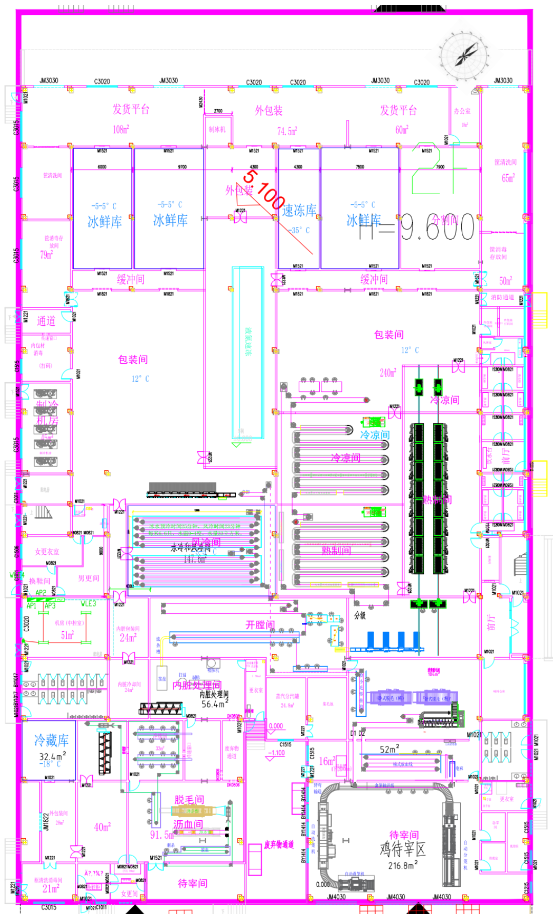
图 3.2-6 屠宰车间 4 首层平面布置图
