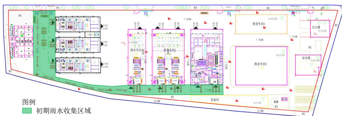
图 3.6-1 初期雨水收集区域示意图
