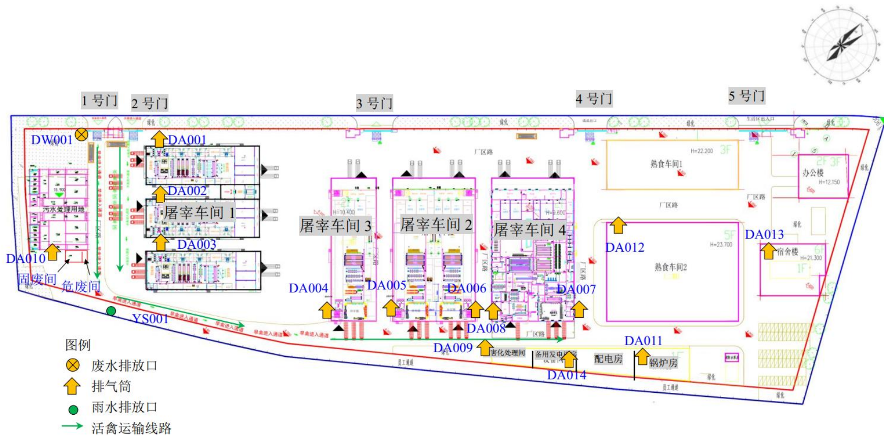
图 3.2-1 本项目总平面布置图
