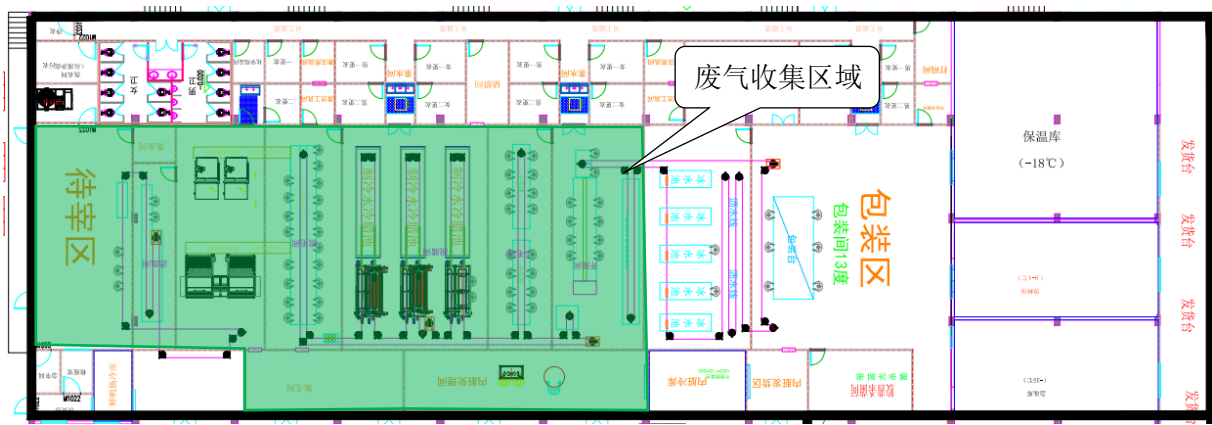
图 3.6-2 屠宰车间 1 分区一~三中典型车间废气收集区域示意图
