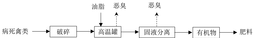
图 3.3-5 无害化处理机工艺流程及产污节点图
