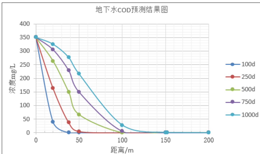
图 5.4-2 地下水 COD Mn 预测结果图
