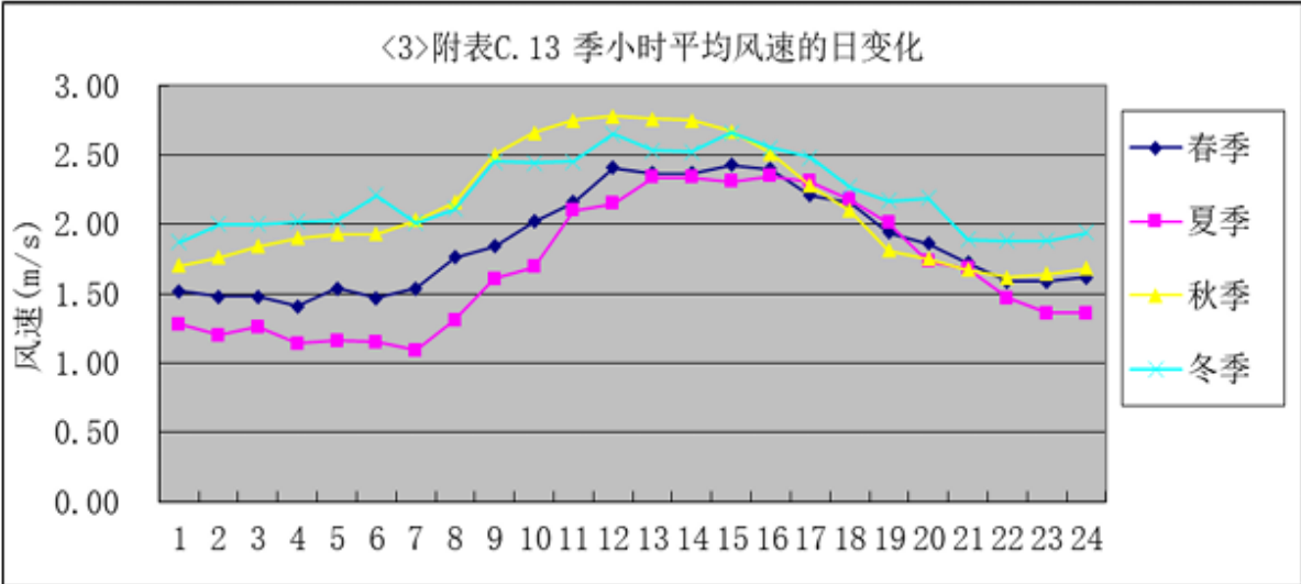
图 5.2-4 台山市 2023 年季小时平均风速的变化图
