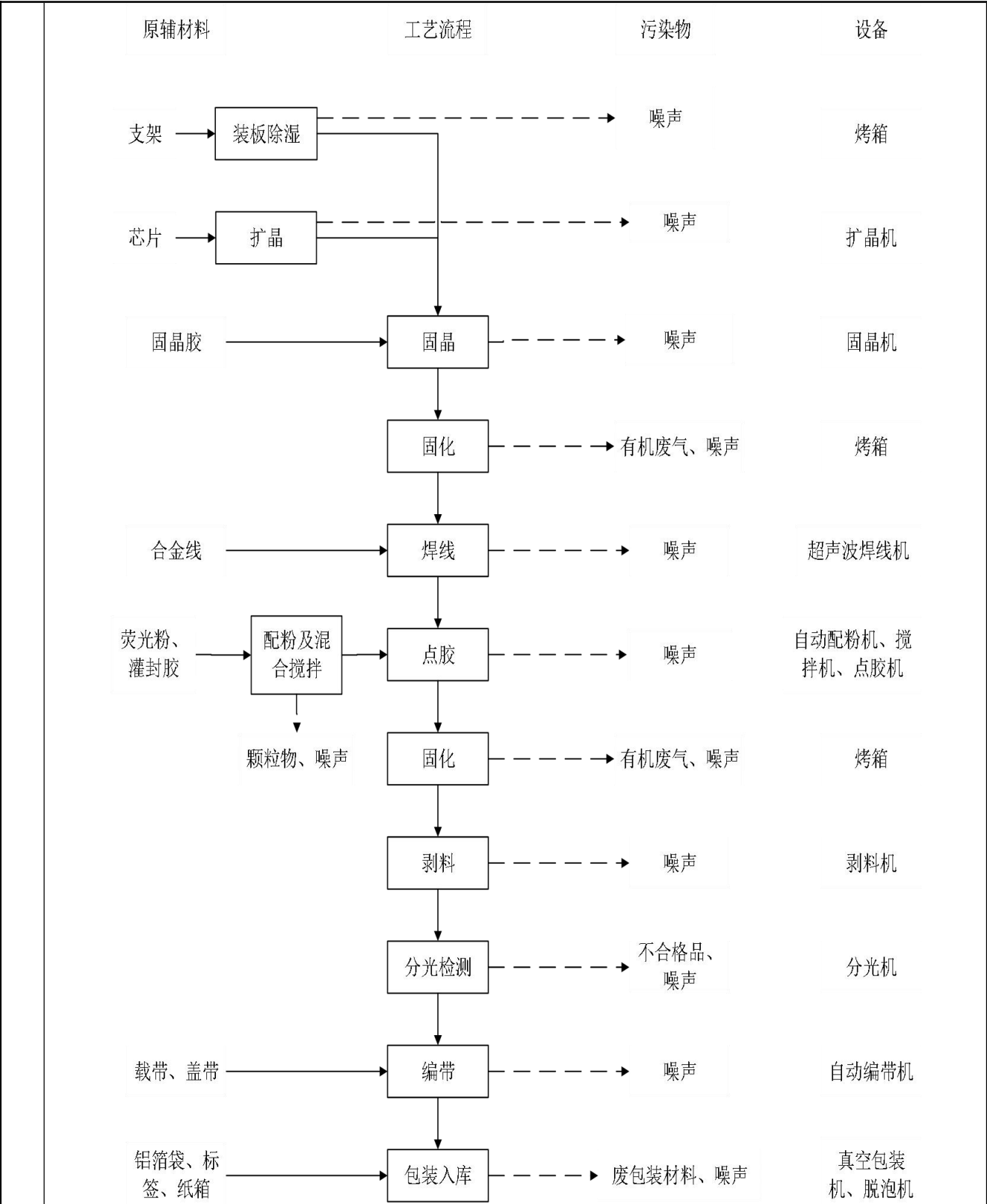
图 2-2 LED 灯珠生产工艺流程及产污环节图
