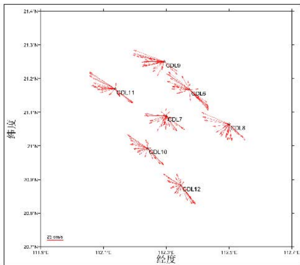
图 5.1.4-1f 冬季底层海流平面分布矢量图
