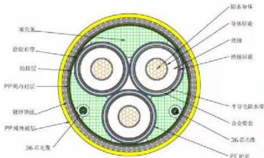
图 3.4-2 海底电缆结构型式图
