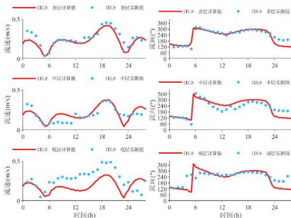
图 6.1.1-13 CDL9 站流速、流向验证（冬季）（2023 年 12 月 13 日 1:00~14 日 3:00）
