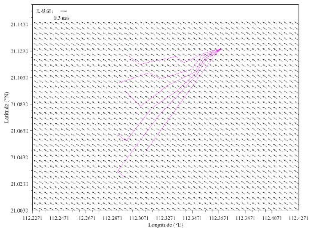
图 6.1.2-1b 工程前工程海域冬季大潮涨急流场（中层）
