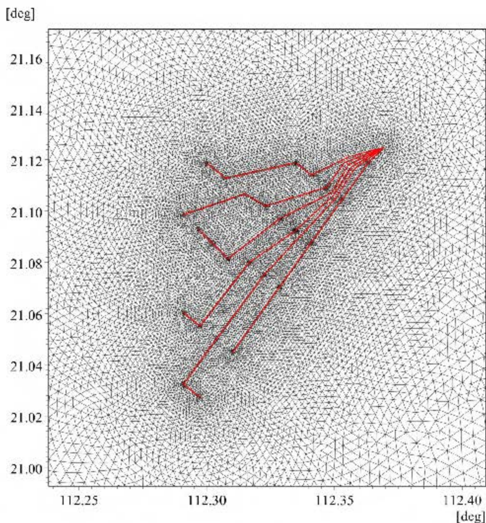
图 6.1.1-2 项目附近海域网格加密
