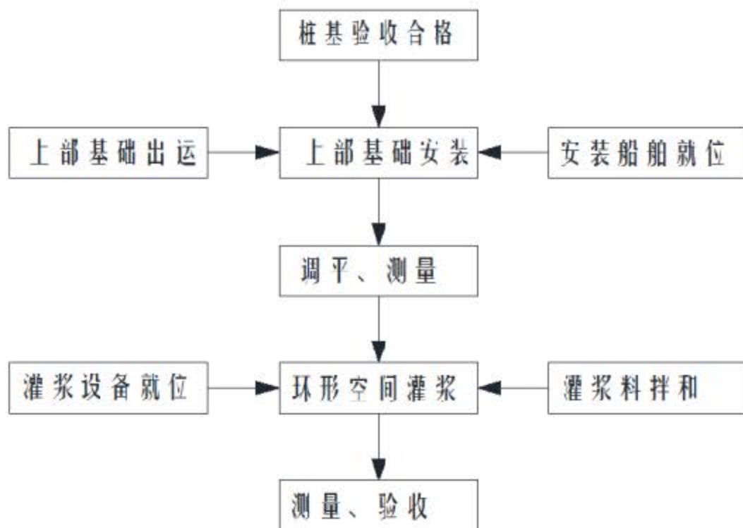
图 3.5.1-4 上部基础结构施工工艺流程图
