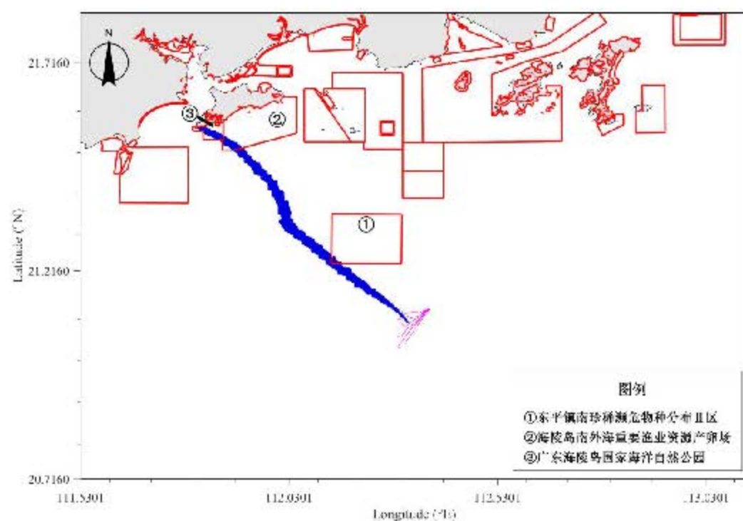
图 7.3.2-4 工况 3 溢油扫海范围 (48 时)
