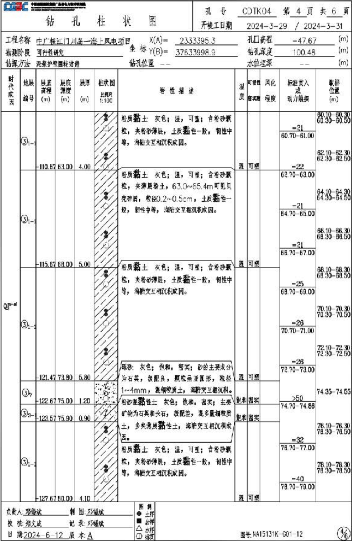
图 5.2.2-3d 钻孔柱状图 (CDTK04)
