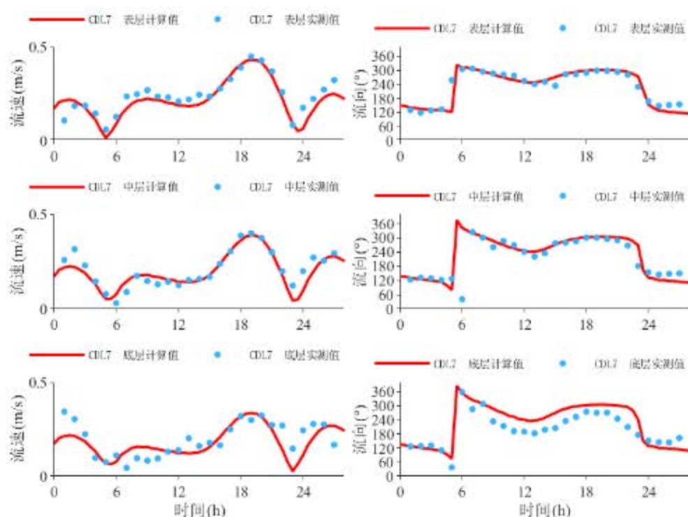
图 6.1.1-11 CDL7 站流速、流向验证 (冬季) (2023 年 12 月 13 日 1:00~14 日 3:00)
