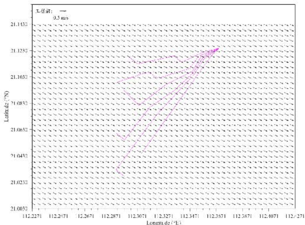
图 6.1.2-2c 工程前工程海域冬季大潮落急流场（底层）
