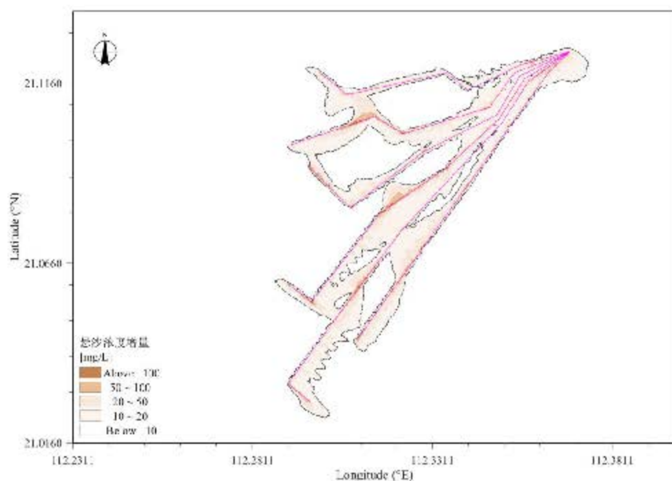
图 6.3.1-5 海缆施工产生悬沙增量包络线图（次底层）
