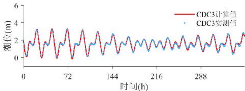
图 6.1.1-6 CDC3 站潮位验证曲线
