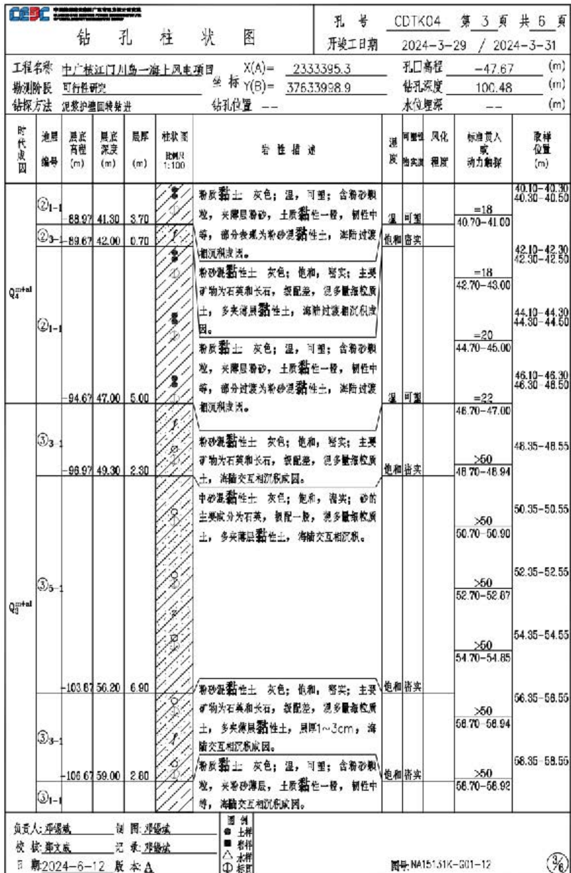
图 5.2.2-3c 钻孔柱状图 (CDTK04)
