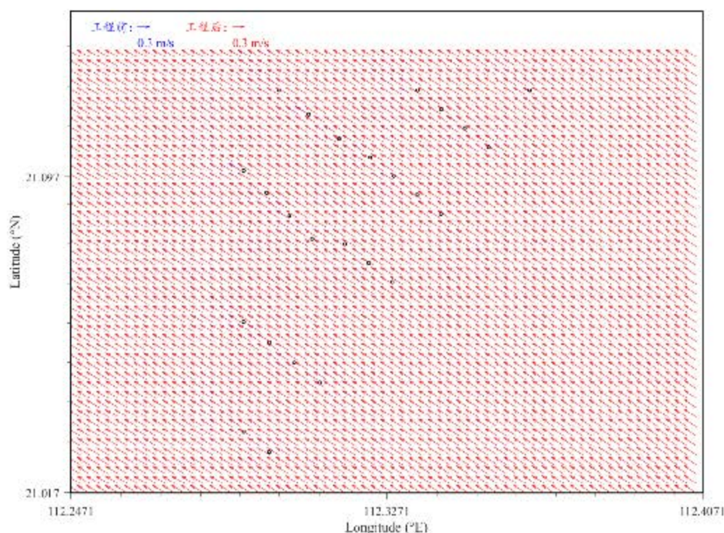
图 6.1.2-4 工程前后大潮涨急流场对比图 (中层)
