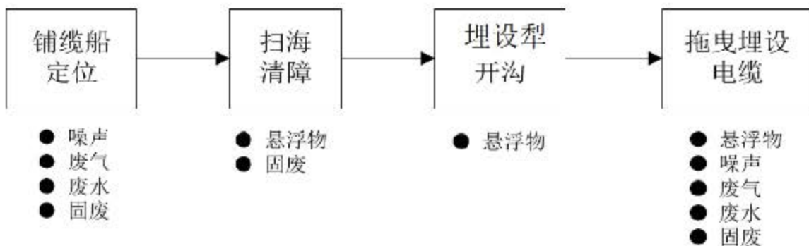
图 3.8.1-2 海底电缆主要施工工序与产污环节
