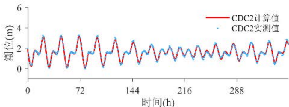
图 6.1.1-5 CDC2 站潮位验证曲线
