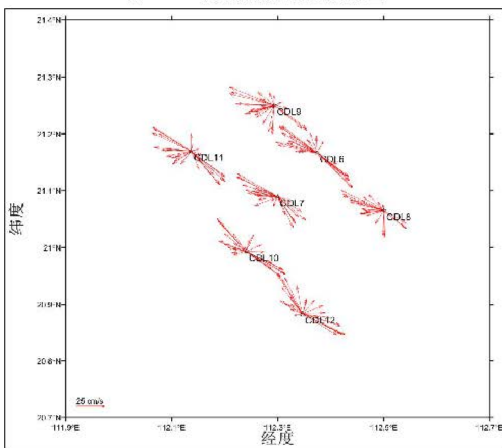
图 5.1.4-1b 冬季 0.2H 层海流平面分布矢量图
