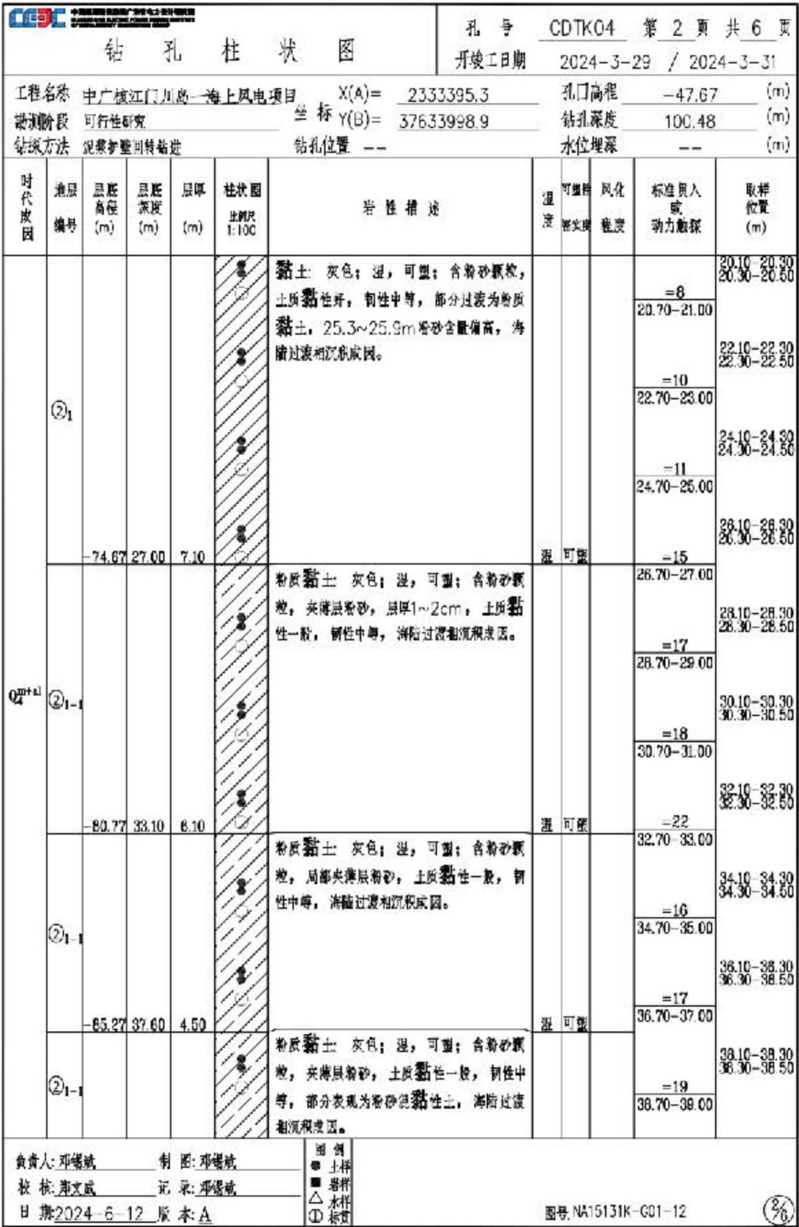
图 5.2.2-3b 钻孔柱状图 (CDTK04)
