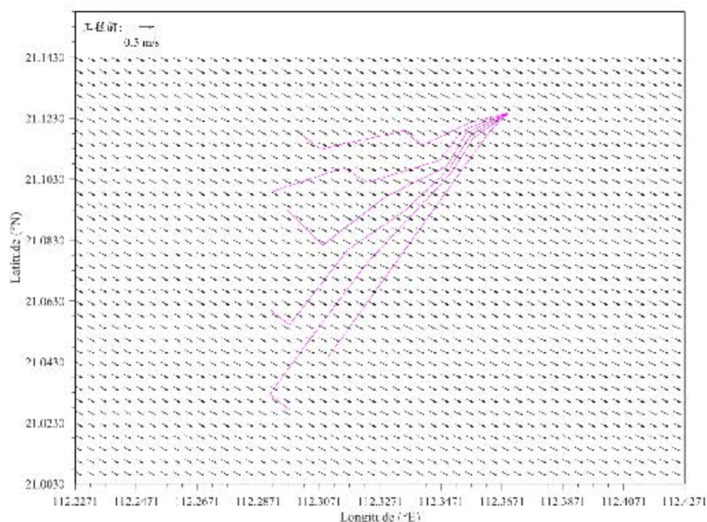
图 6.1.2-2a 工程前工程海域冬季大潮落急流场（表层）
