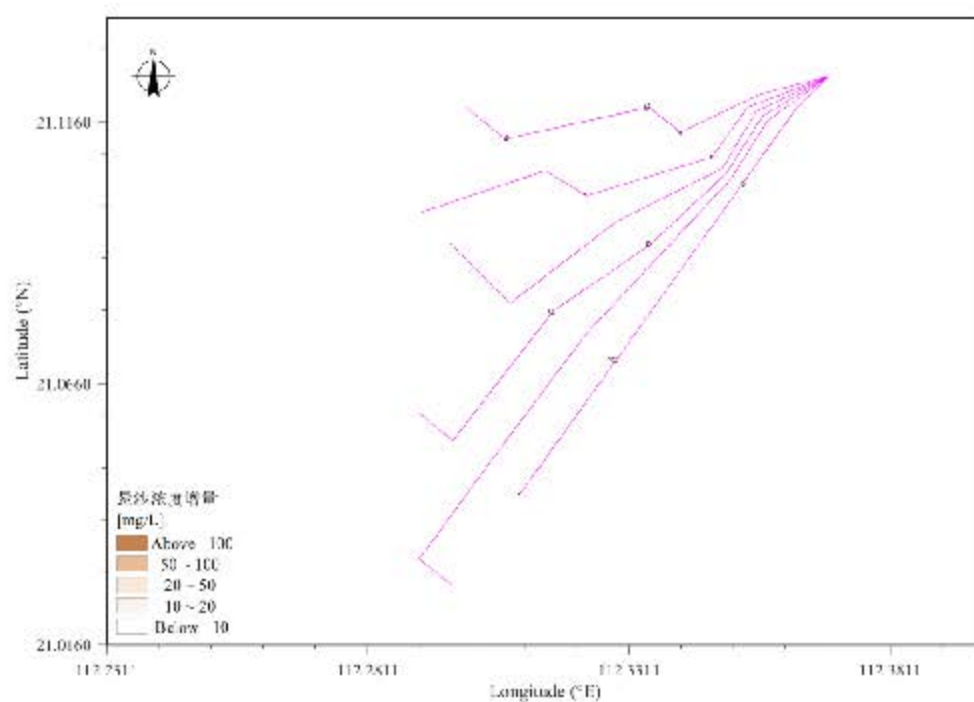
图 6.3.1-11 辅助桩拆除施工产生悬沙增量包络线图（次底层）
