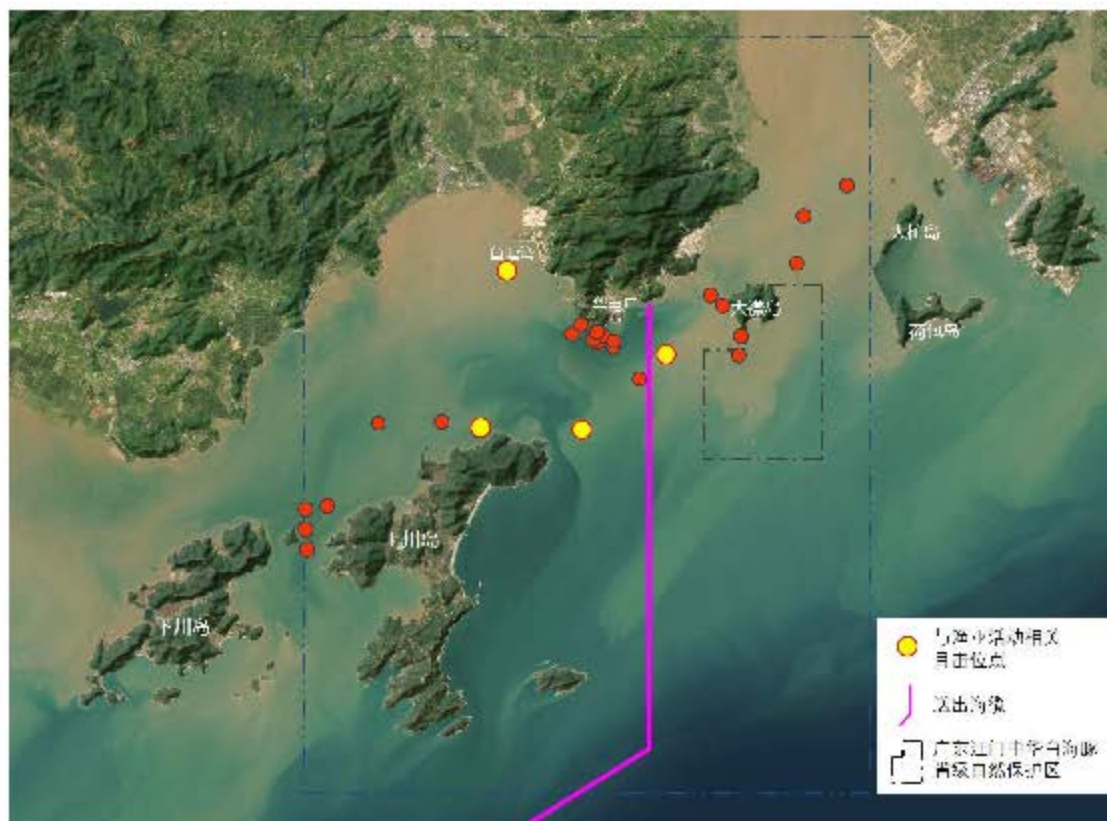
图 5.11.6-3 江门川岛风电项目海域与渔业活动关联的中华白海豚目击分布
