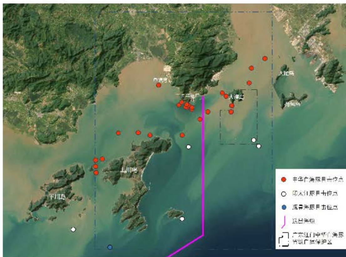
图 5.11.2-1 近岸监测区中华白海豚目击分布
