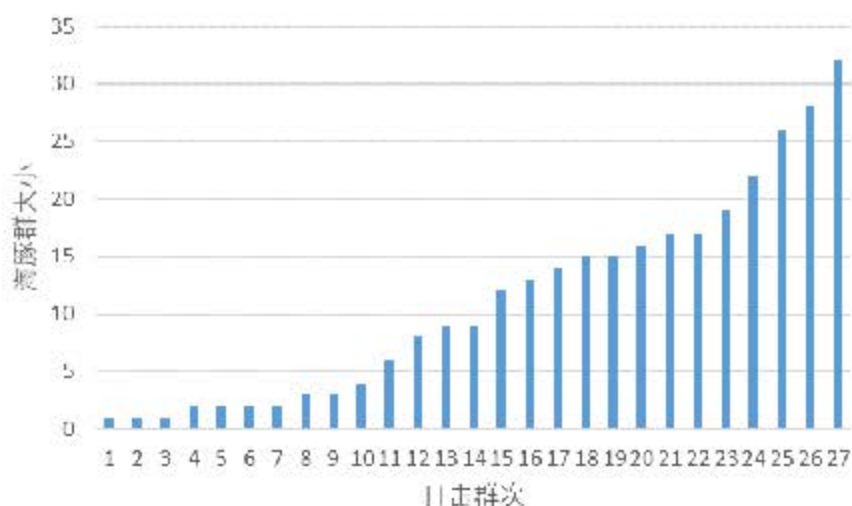
图 5.11.4-2 中华白海豚群大小频次分布
