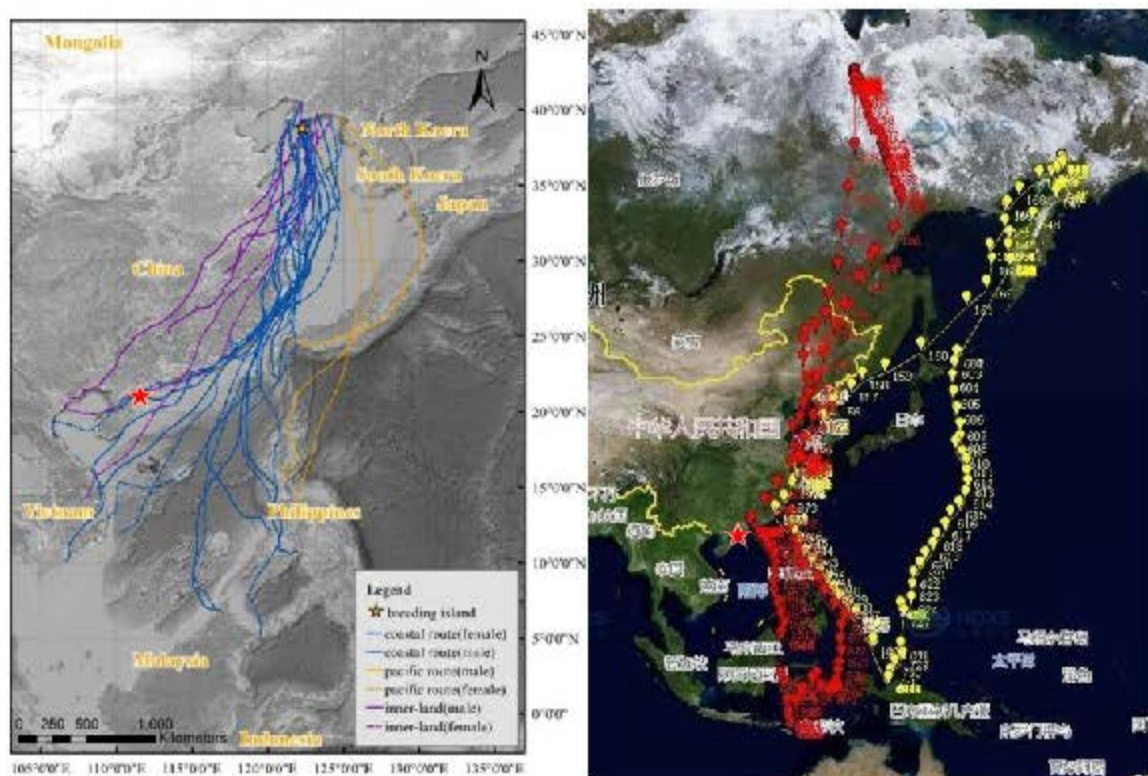
图 5.8.6-2 不同类群鸟类迁徙路线（上：环颈鸬；下左：黄嘴白鹭；下右：中杓鸬，星型符号为项目场址）
