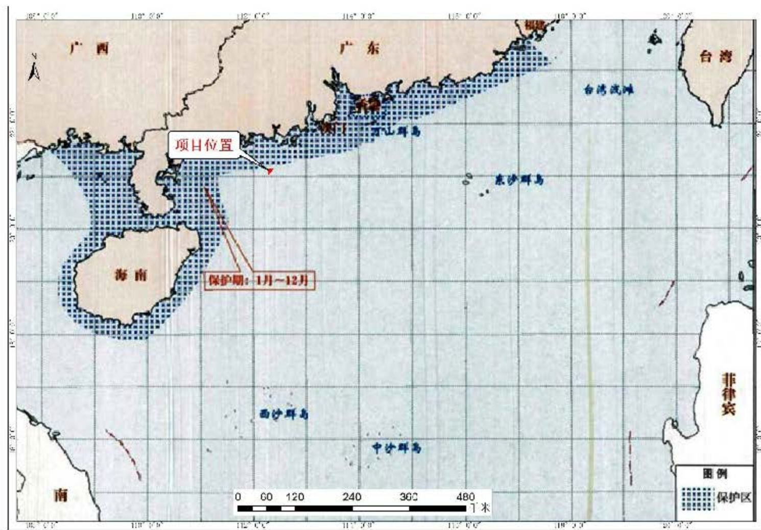
图 4.2.9-3 南海北部幼鱼繁育场保护区范围示意图
