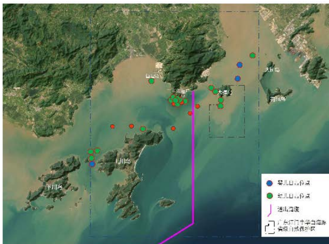
图 5.11.5-2 江门川岛风电项目海域中华白海豚幼豚目击分布
