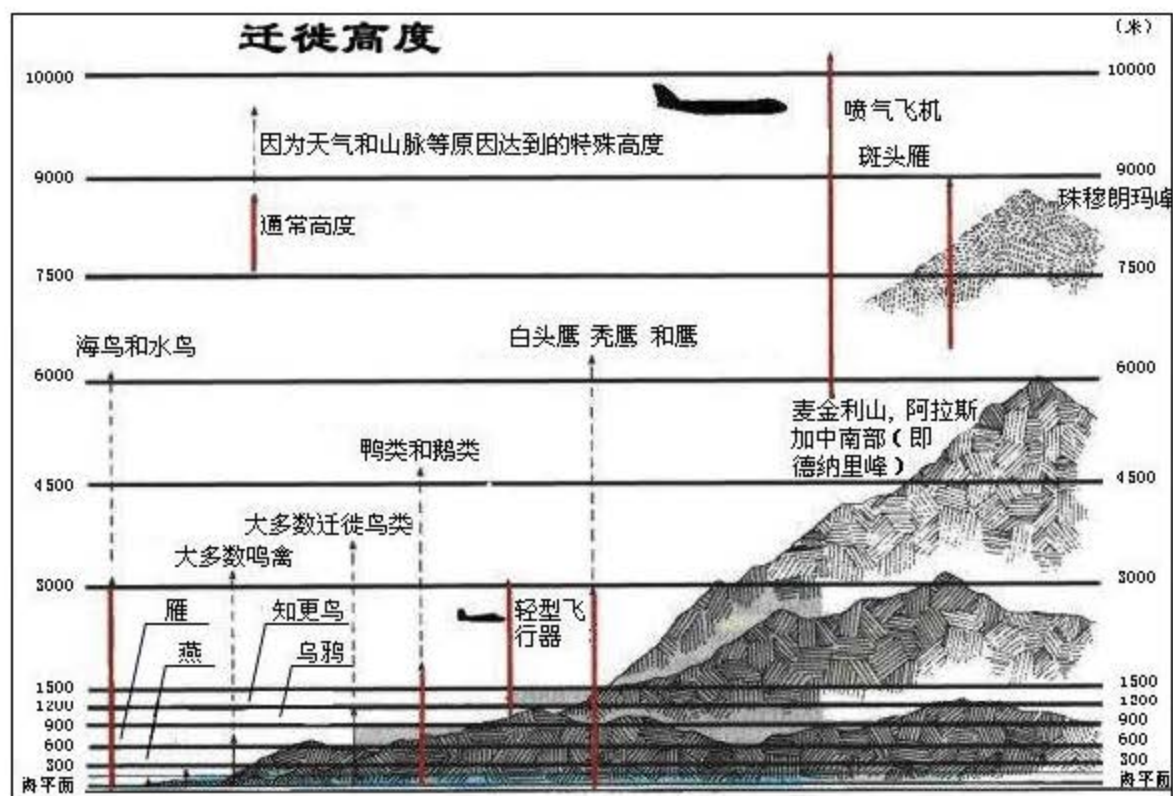
图 5.8.6-3 不同鸟类类群的飞行高度示意图
