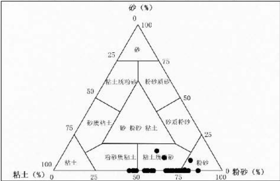
图 5.1.8-2 冬季悬沙所有样品谢帕德三角图分布（N=28）
