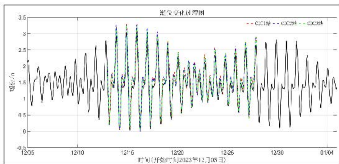
图 5.1.3-2b 冬季高栏岛站潮位过程曲线
