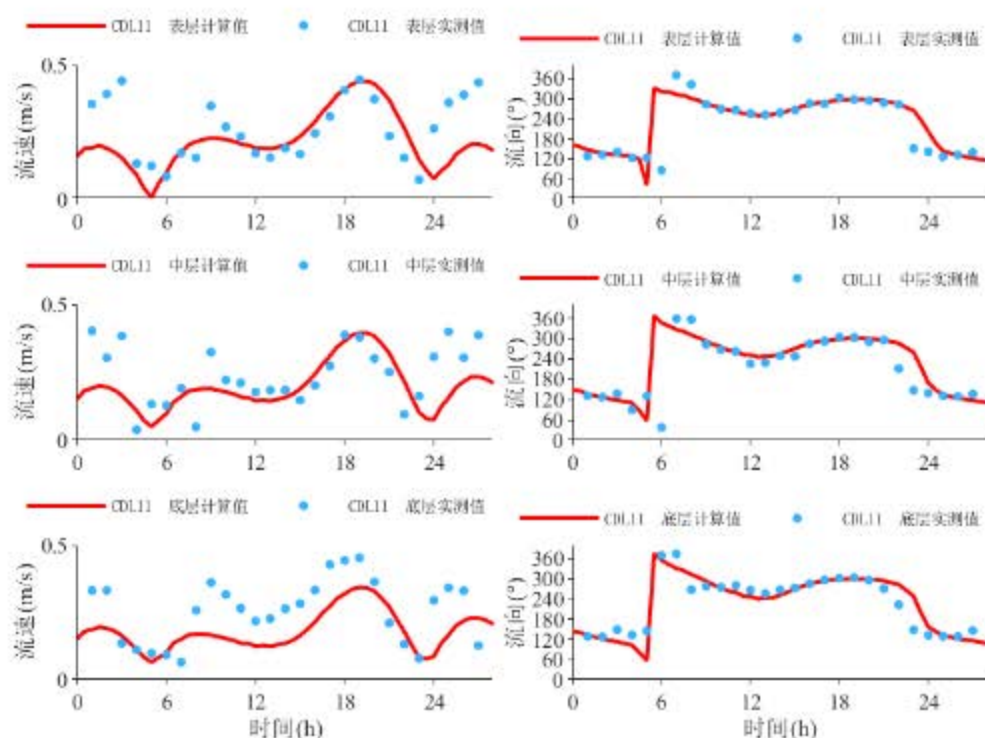
图 6.1.1-15 CDL11 站流速、流向验证 (冬季) (2023 年 12 月 13 日 1:00~14 日 3:00)
