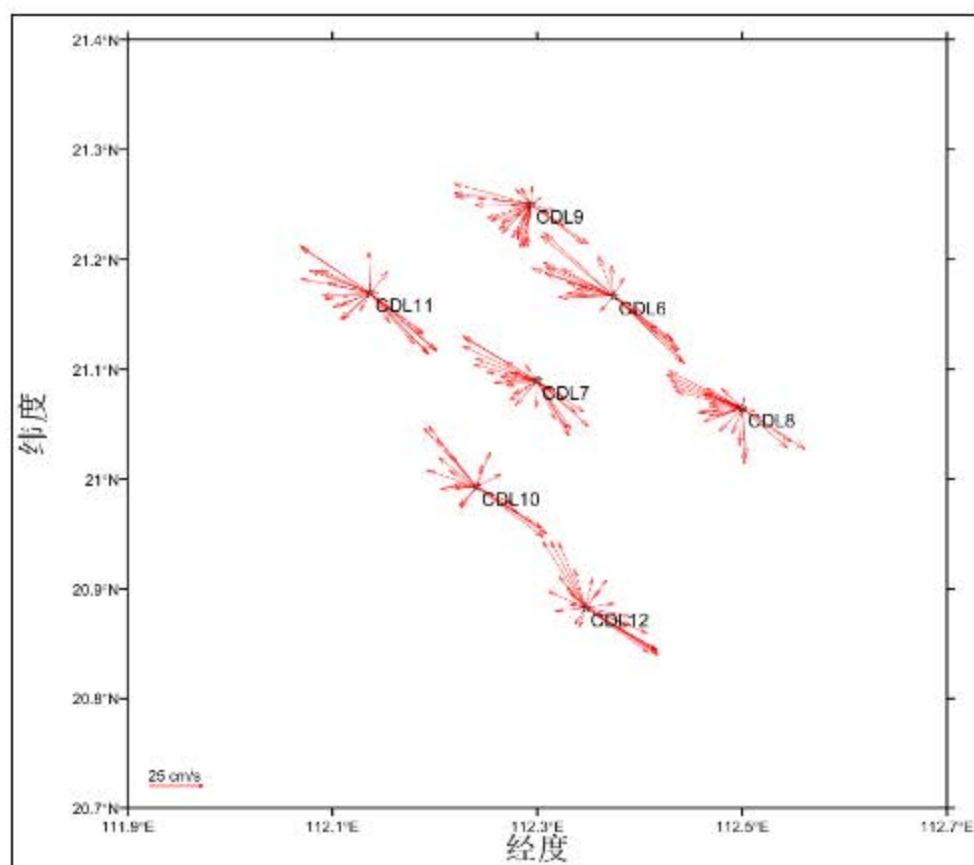
图 5.1.4-1c 冬季 0.4H 层海流平面分布矢量图
