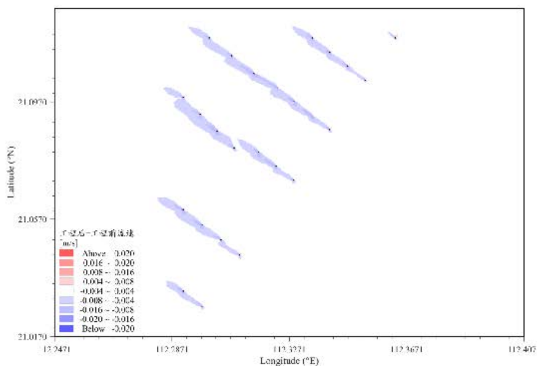
图 6.1.2-8 工程后-工程前涨急流速变化等值线图（中层）
