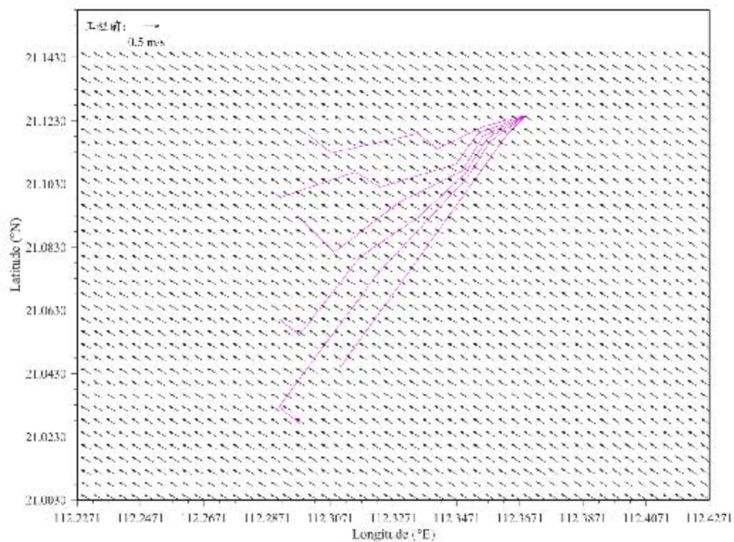
图 6.1.2-1c 工程前工程海域冬季大潮涨急流场（底层）
