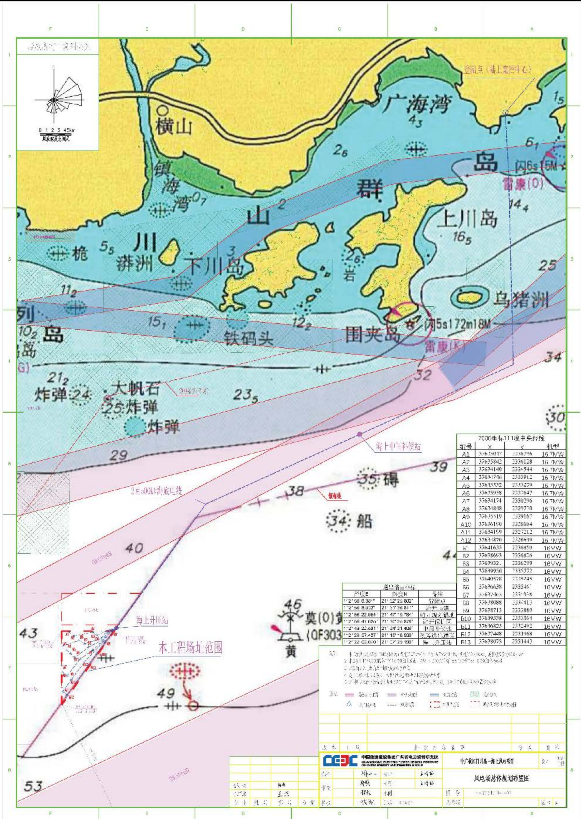
图 3.3-1 项目总平面布置图
