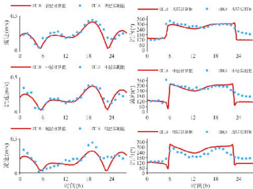
图 6.1.1-12 CDL8 站流速、流向验证 (冬季) (2023 年 12 月 13 日 1:00~14 日 3:00)
