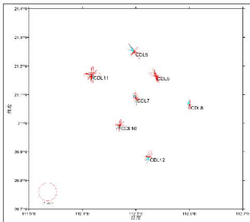
图 5.15-1d 冬季各站各层 S 2 分潮椭圆图
