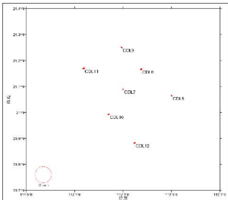
图 5.1.5-1f 冬季各站各层 MS 4 分潮椭圆图
