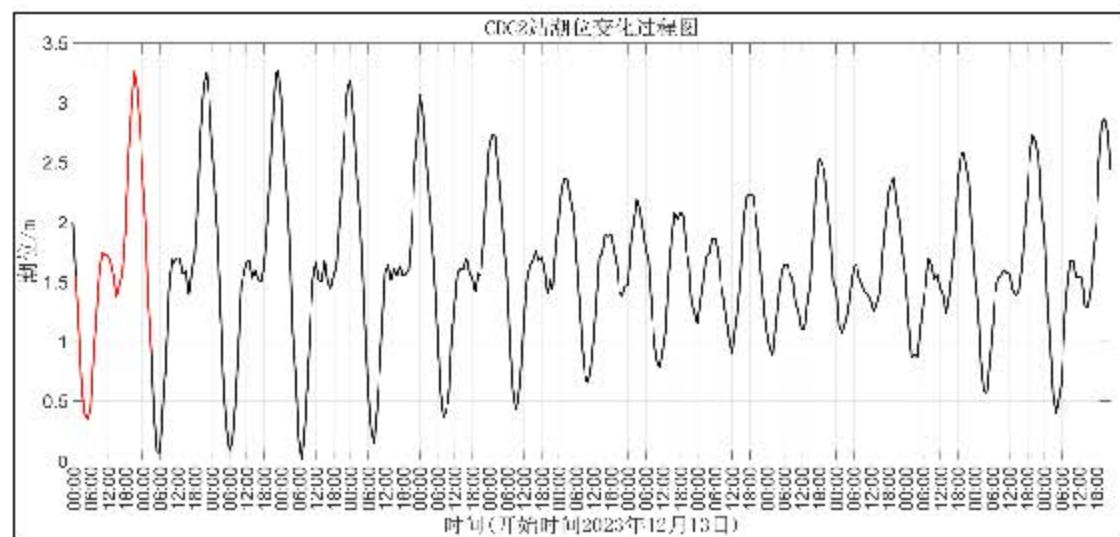
图 5.1.3-1b 冬季 CDC2 站潮位过程曲线
