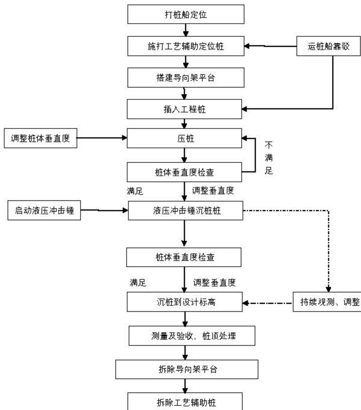
图 3.5.1-1 常规钢管桩沉桩施工工艺图
