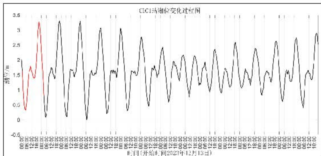
图 5.1.3-1a 冬季 CDC1 站潮位过程曲线
