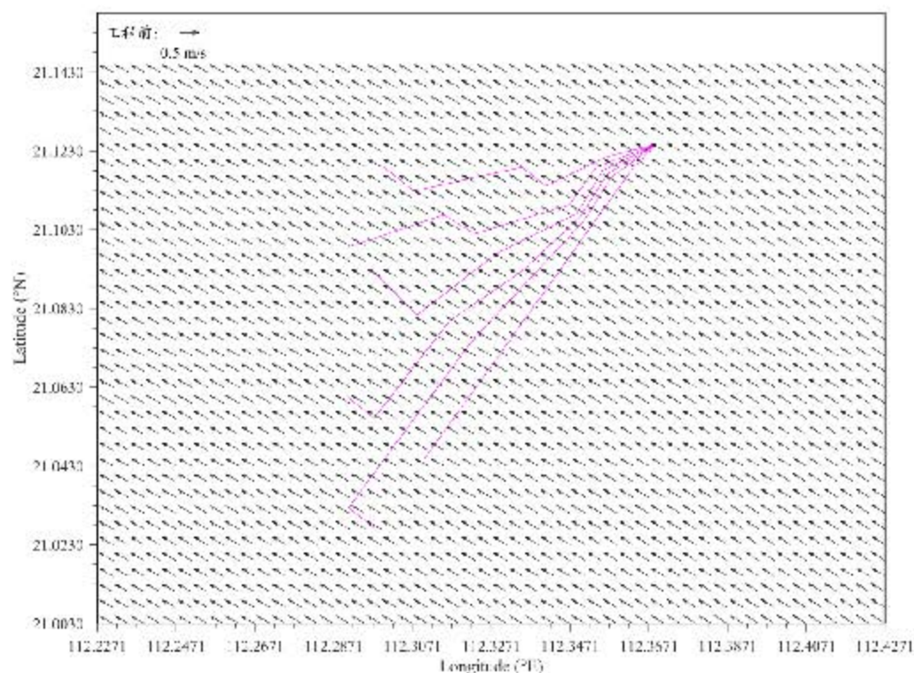
图 6.1.2-1a 工程前工程海域冬季大潮涨急流场（表层）
