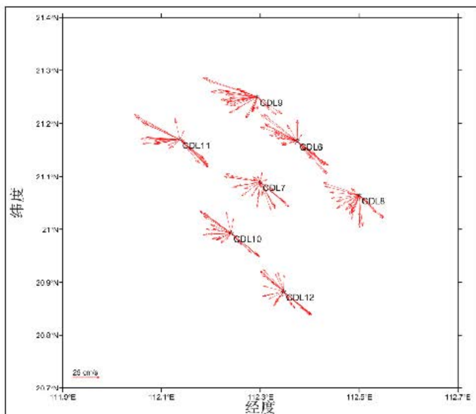
图 5.1.4-1e 冬季 0.8H 层海流平面分布矢量图
