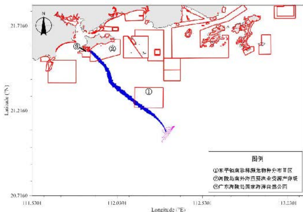
图 7.3.2-5 工况 4 溢油扫海范围 (48 时)
