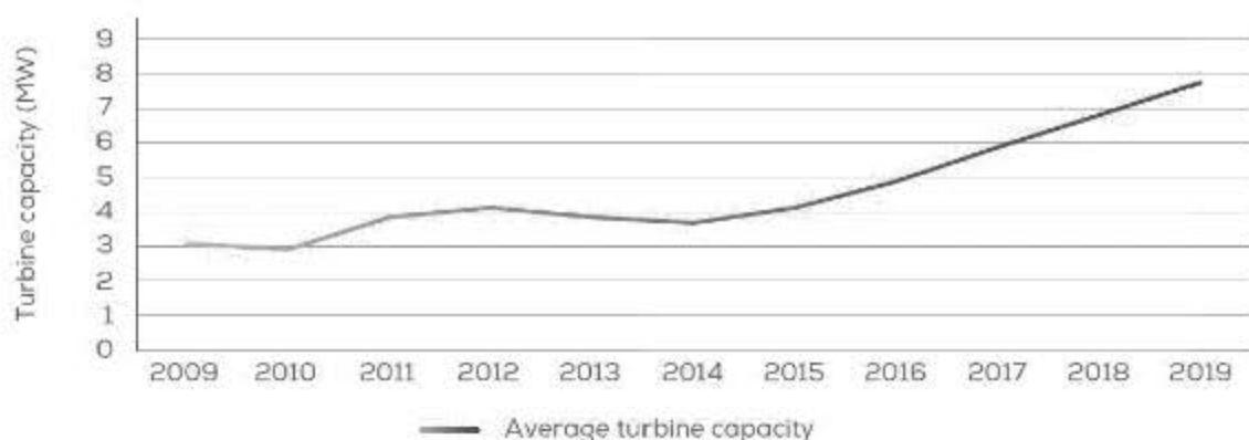
图 3.12.2-1 欧洲海上风电机组历年平均单机容量
