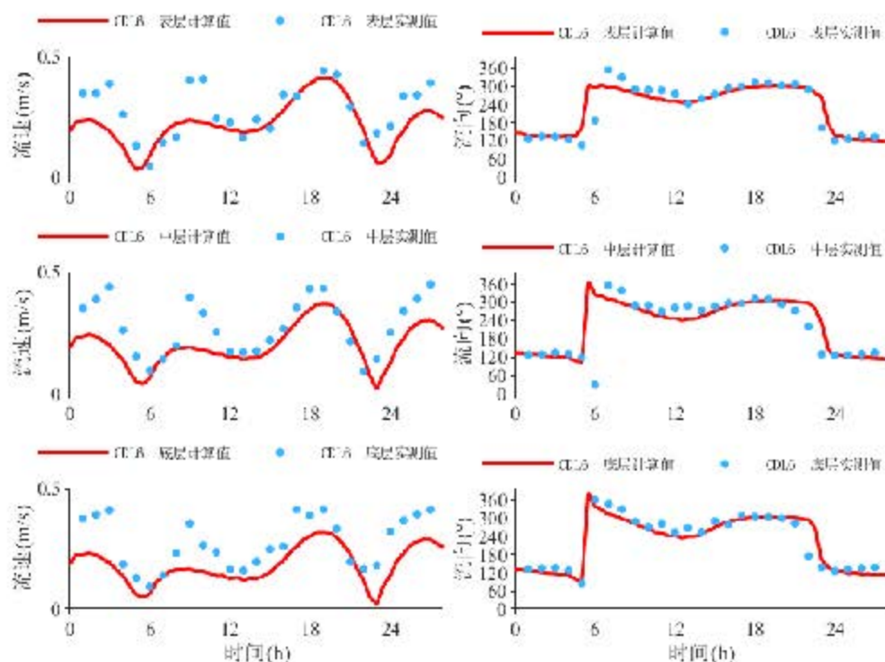
图 6.1.1-10 CDL6 站流速、流向验证（冬季）（2023 年 12 月 13 日 1:00~14 日 3:00）
