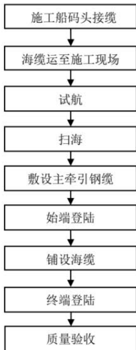
图 3.5.1-6 海缆敷设施工工艺
