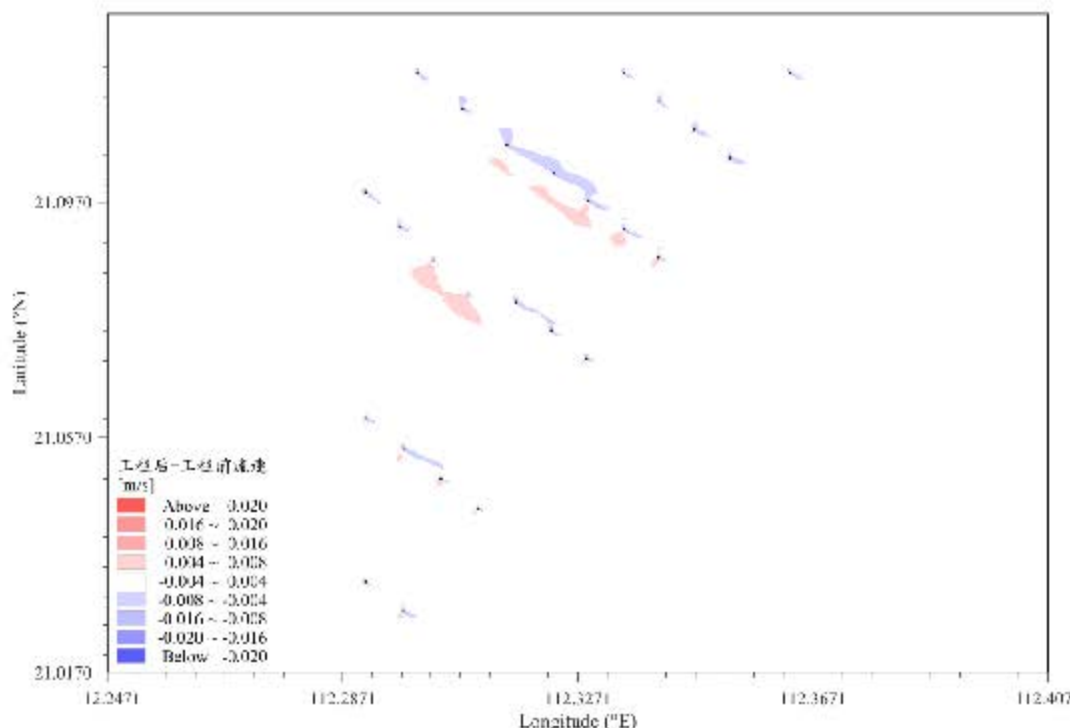
图 6.1.2-9 工程后-工程前落急流速变化等值线图（中层）
