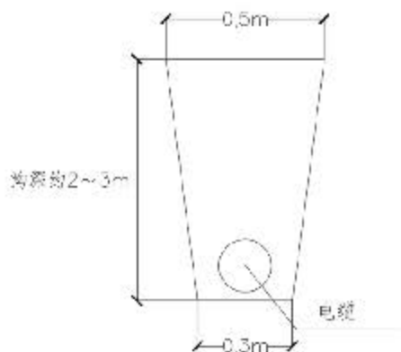
图 3.5.1-9 电缆沟剖面图
