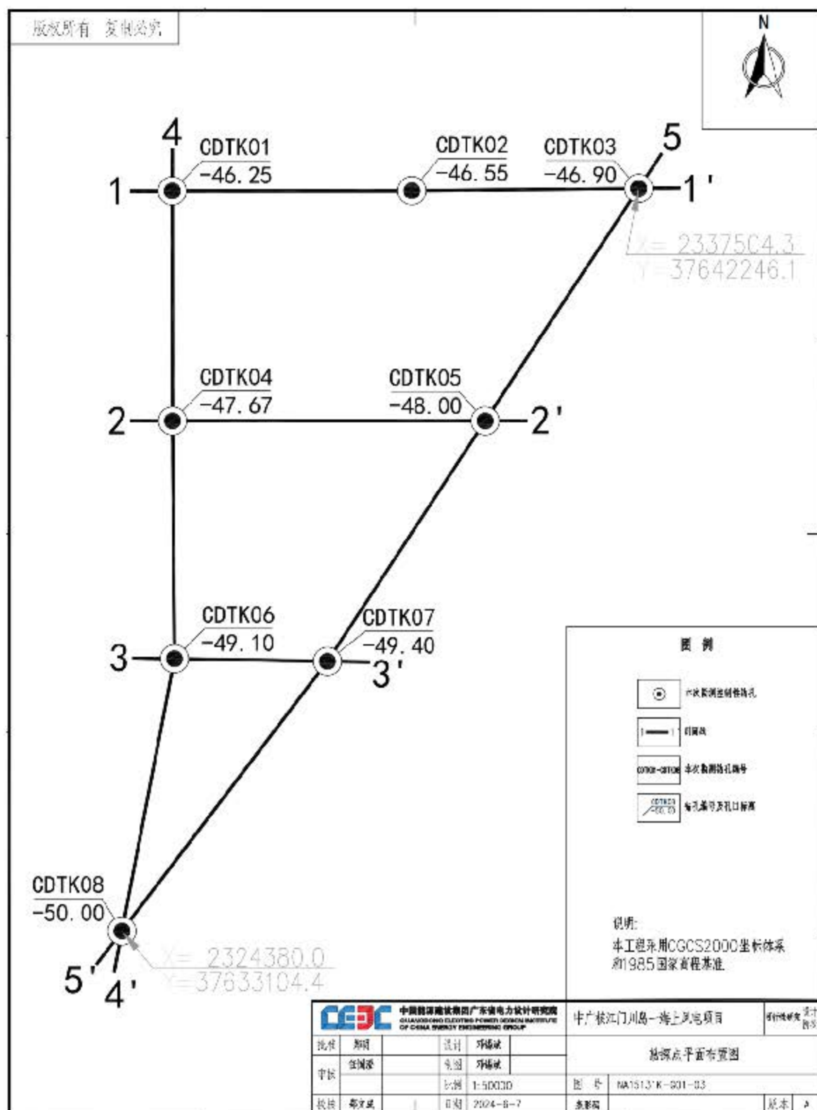
图 5.2.2-1 钻孔平面布置图
