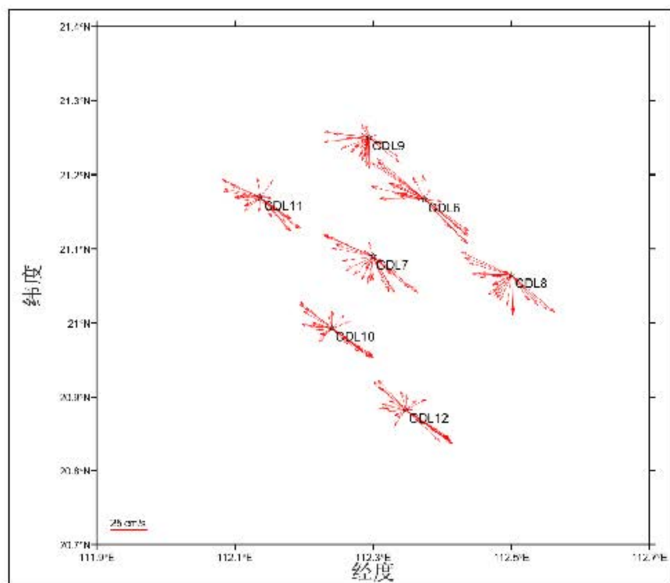
图 5.1.4-1d 冬季 0.6H 层海流平面分布矢量图
