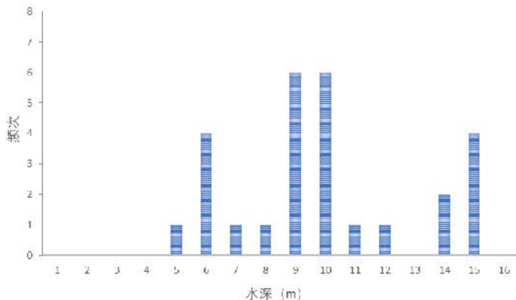
图 5.11.2-2 江门川岛海上风电海域中华白海豚目击位置水深与发现频次关系
