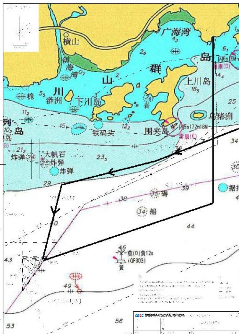
图 3.5.1-10 海上运输线路示意图
