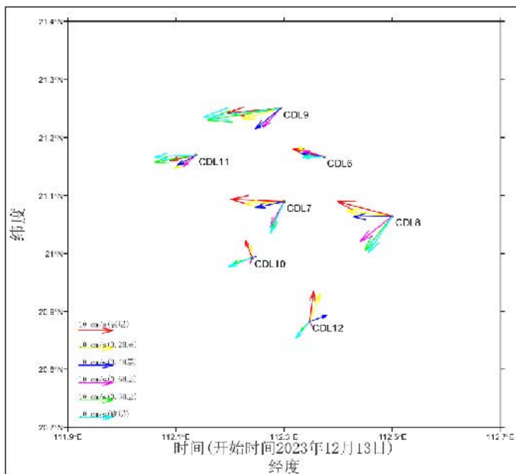
图 5.1.6-1 冬季观测期各站余流图
