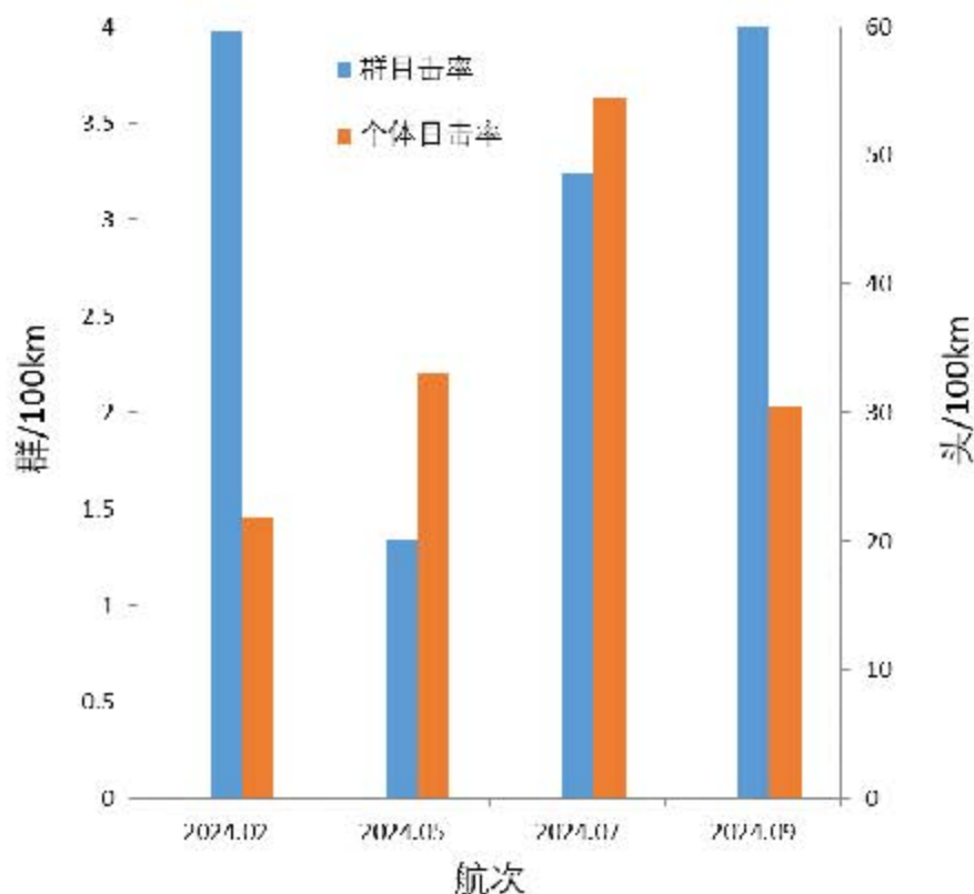
图 5.11.3-1 江门川岛风电项目海域各航次中华白海豚目击率
