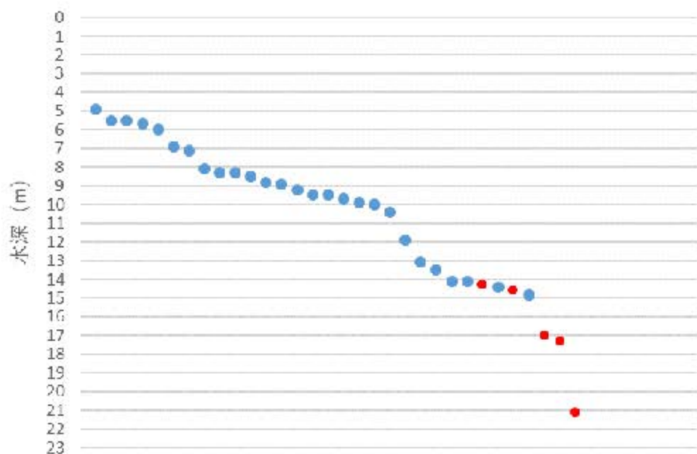
图 5.11.2-3 江门川岛海上风电海域（近岸区）中华白海豚与印太江豚目击位置水深对比示意图
