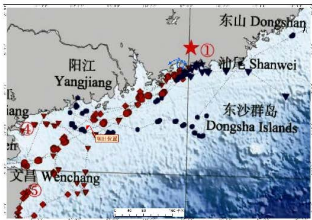
图 4.2.8-36 只幼年绿海龟的洄游路线
