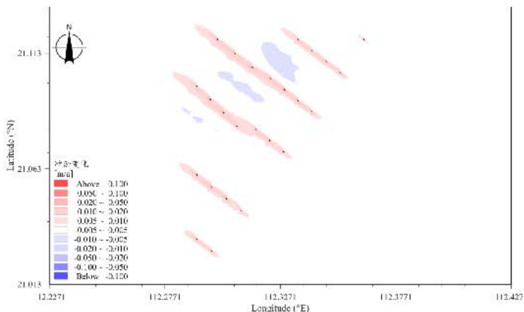
图 6.2-1 工程实施后附近海域年冲刷变化图
