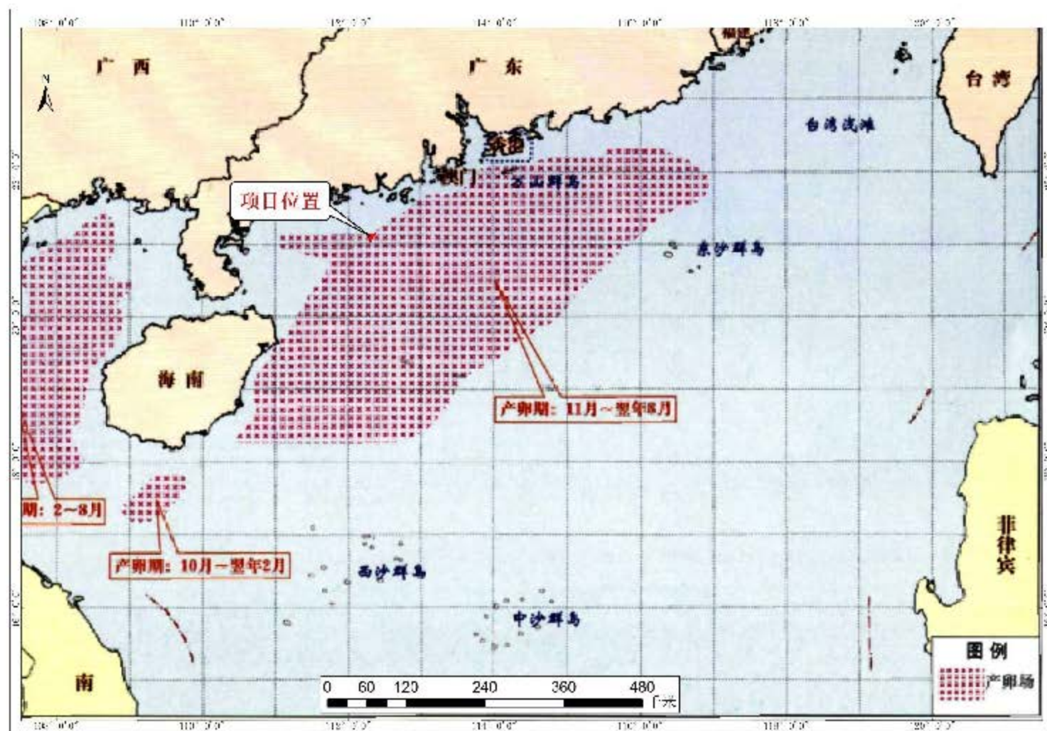
图 4.2.9-2 南海底层、近底层鱼类产卵场示意图
