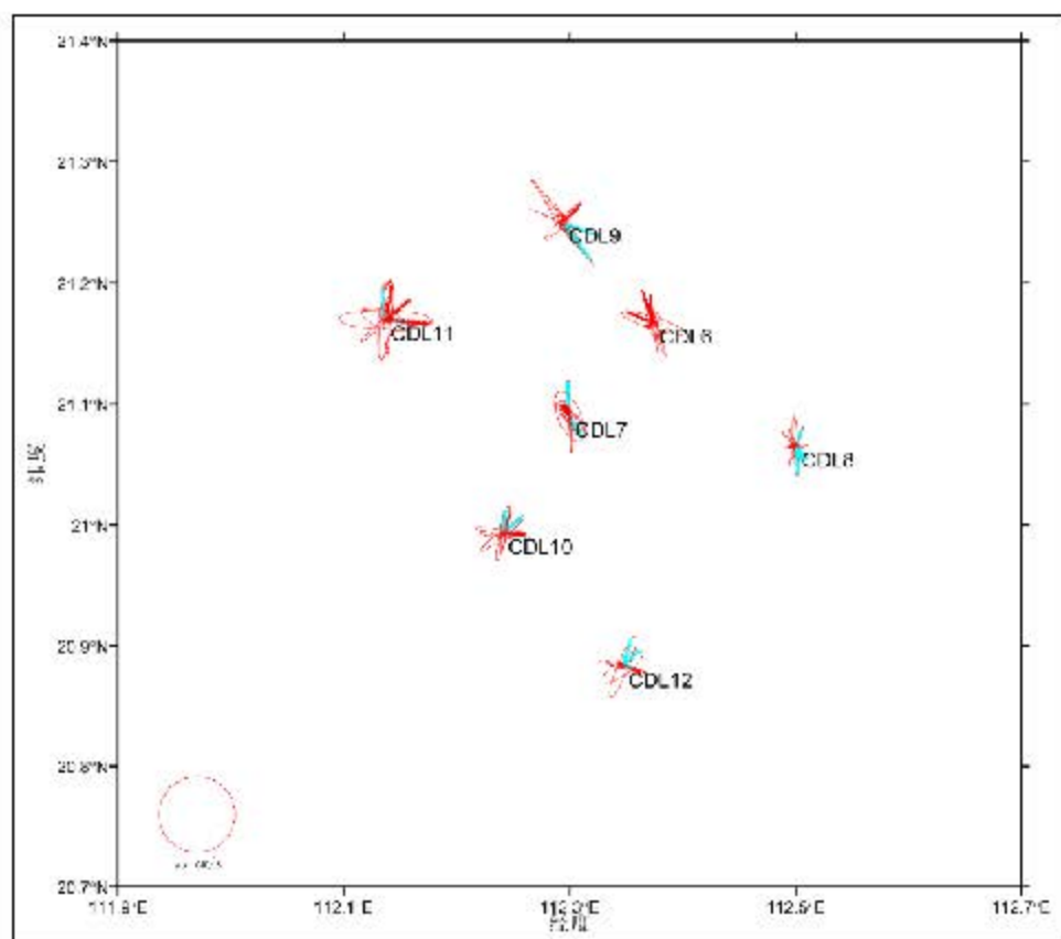
图 5.1.5-1c 冬季各站各层 M 2 分潮椭圆图
