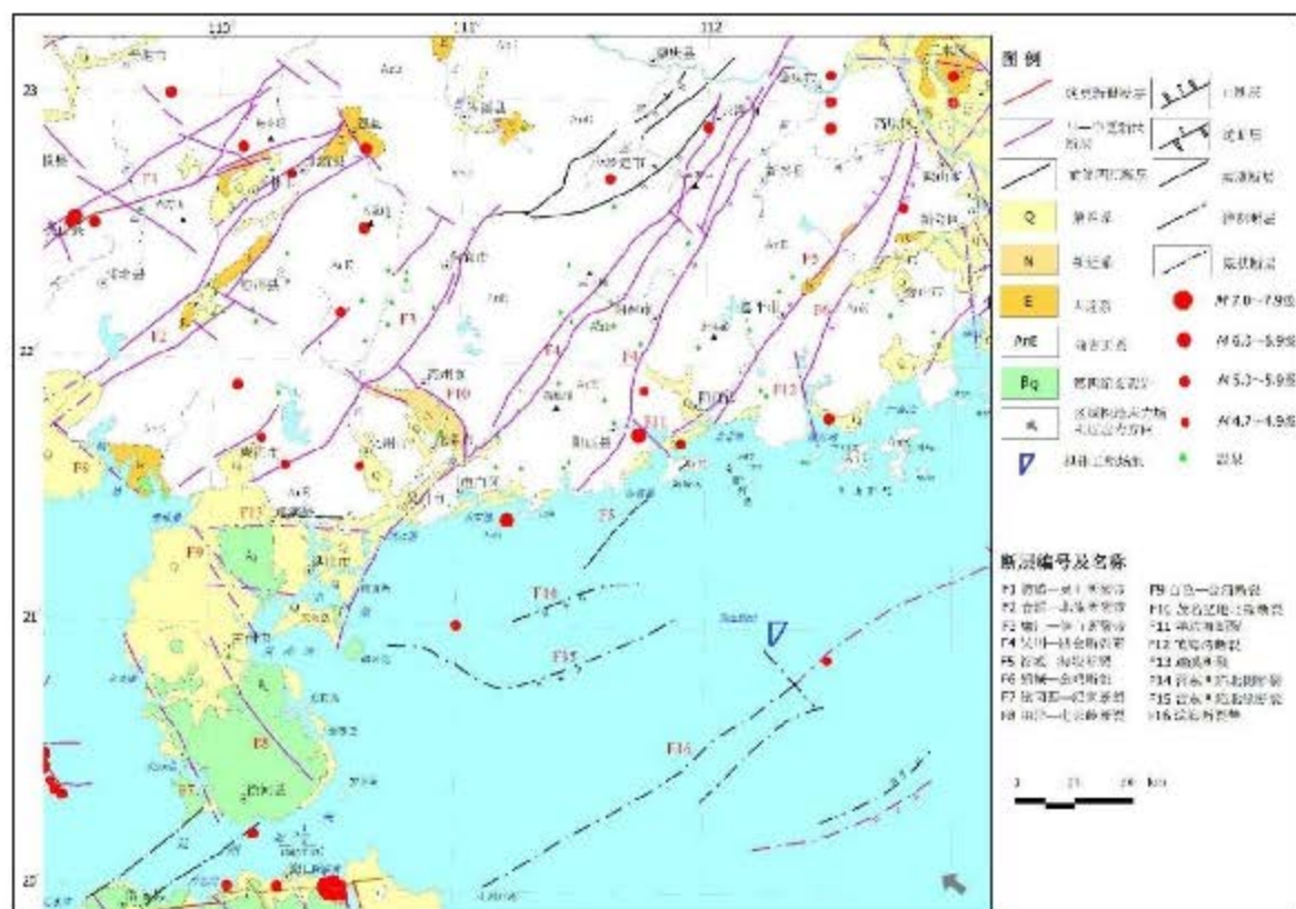
图 4.1.3-1 区域地质构造图（M≥4.7，1507~2020 年）
