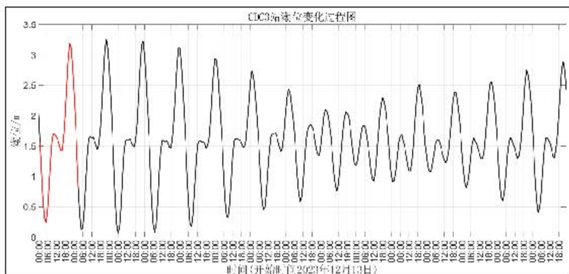
图 5.1.3-1c 冬季 CDC3 站潮位过程曲线
