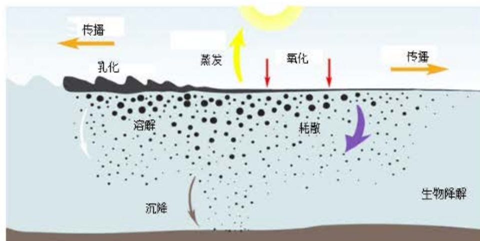
图 7.3.2-1 溢油风化过程示意图
