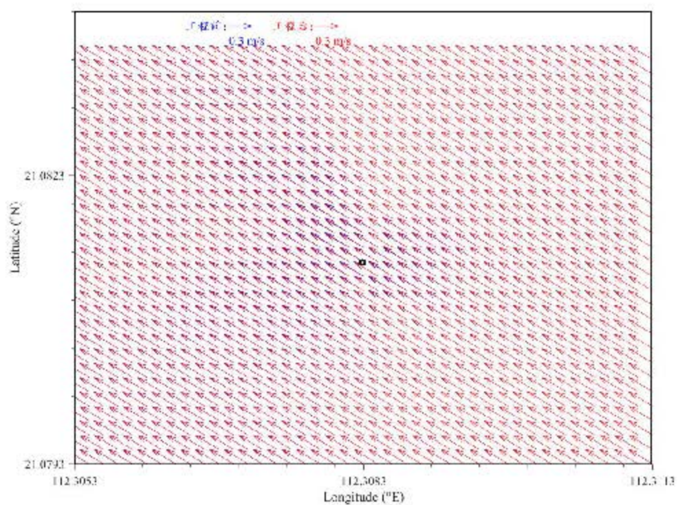
图 6.1.2-6 工程前后大潮涨急流场对比图（中层局部放大）
