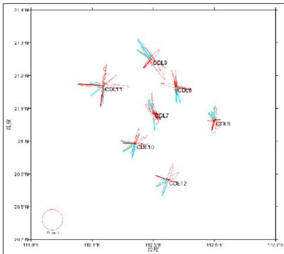
图 5.1.5-1a 冬季各站各层 O_1 分潮椭圆图
