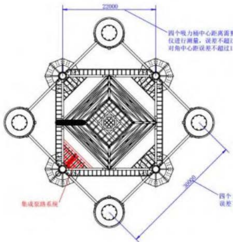
图 3.5.1-3 定位架平面布置示意图
