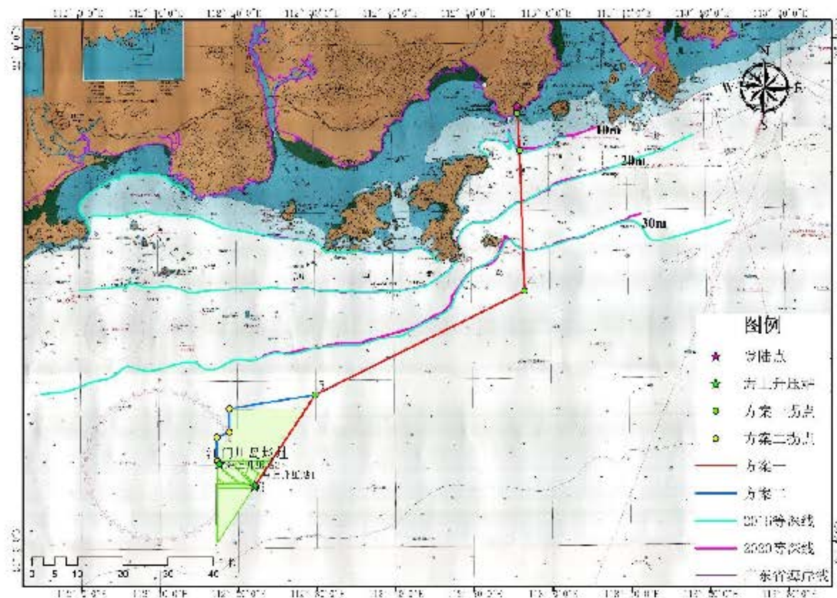
图 5.2.6-1 2016~2020 年海床等深线变化图
