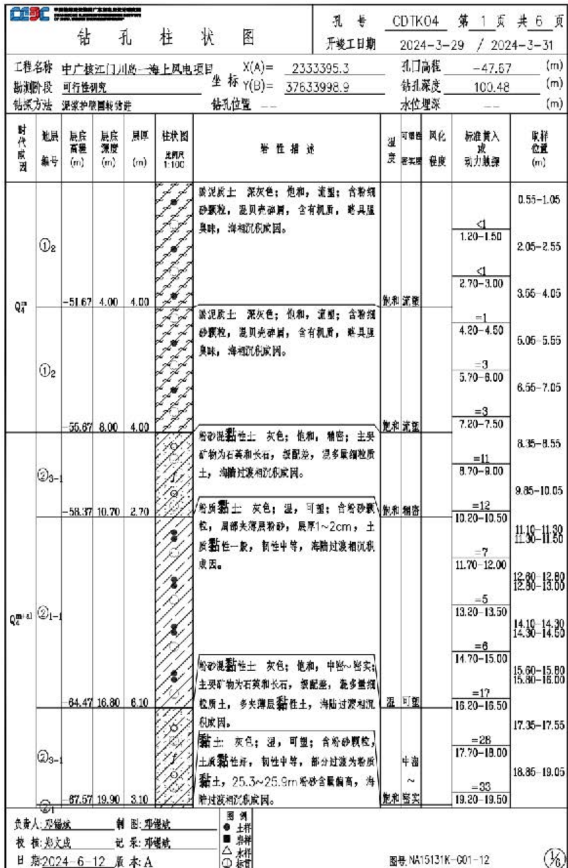
图 5.2.2-3a 钻孔柱状图 (CDTK04)
