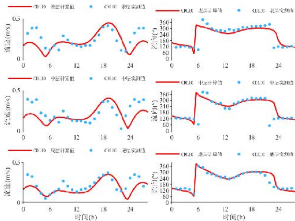
图 6.1.1-14 CDL10 站流速、流向验证（冬季）（2023 年 12 月 13 日 1:00~14 日 3:00）
