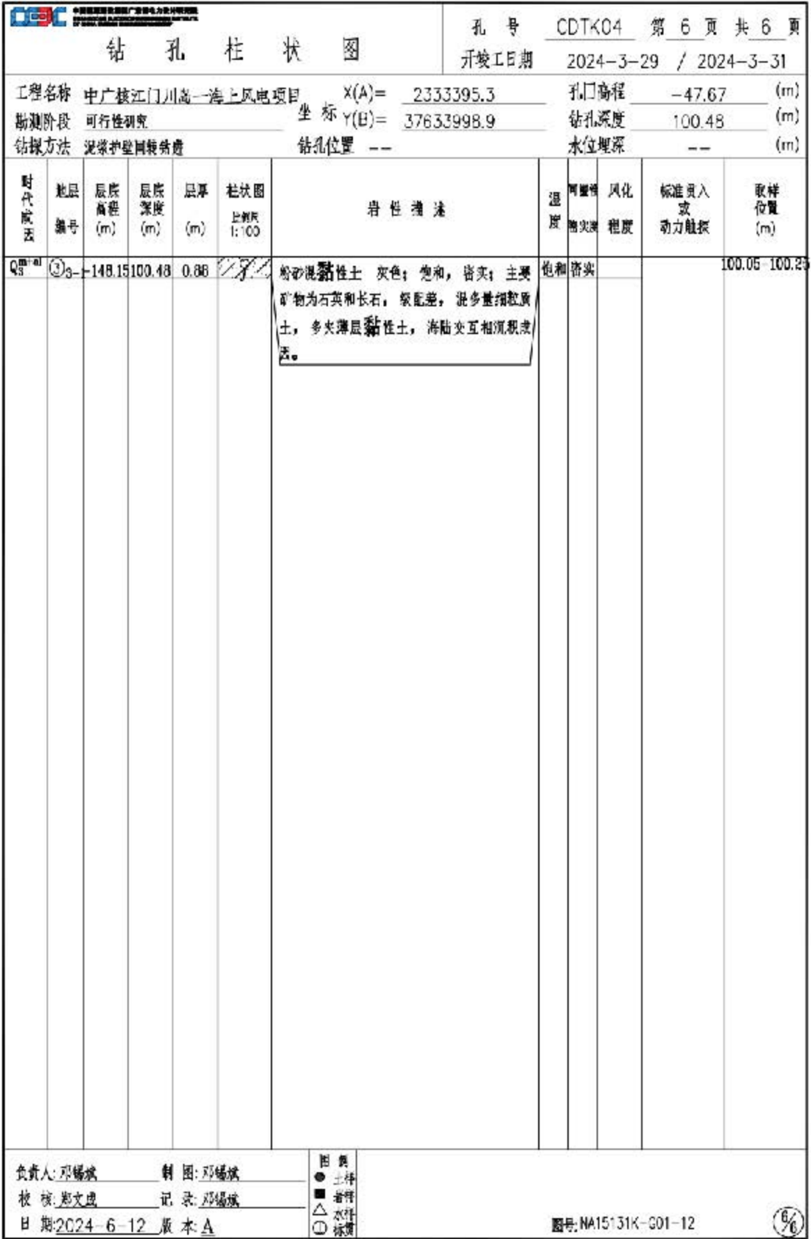
图 5.2.2-3f 钻孔柱状图 (CDTK04)
