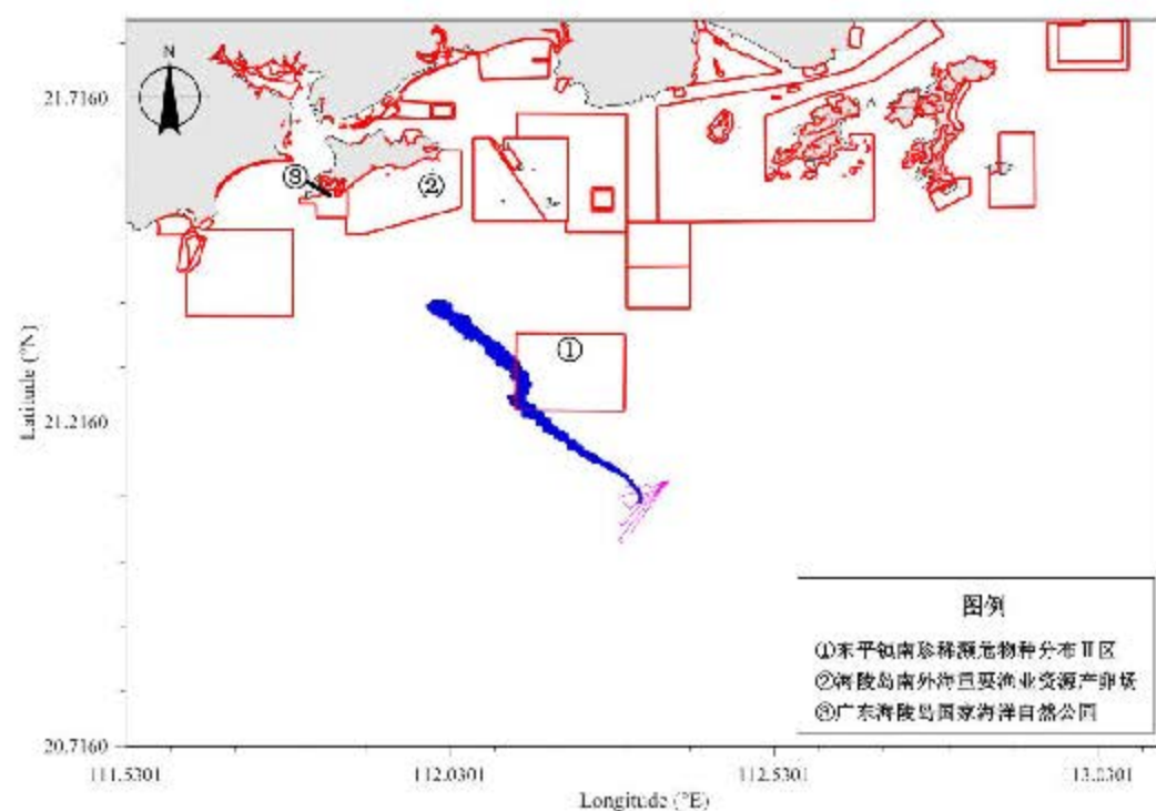
图 7.3.2-3 工况 2 溢油扫海范围 (48 时)
