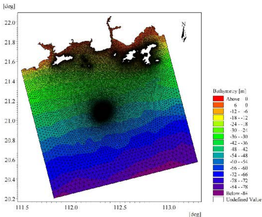
图 6.1.1-1 模型计算范围
