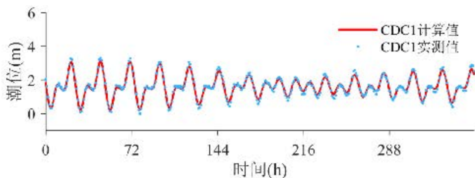
图 6.1.1-4 CDC1 站潮位验证曲线
