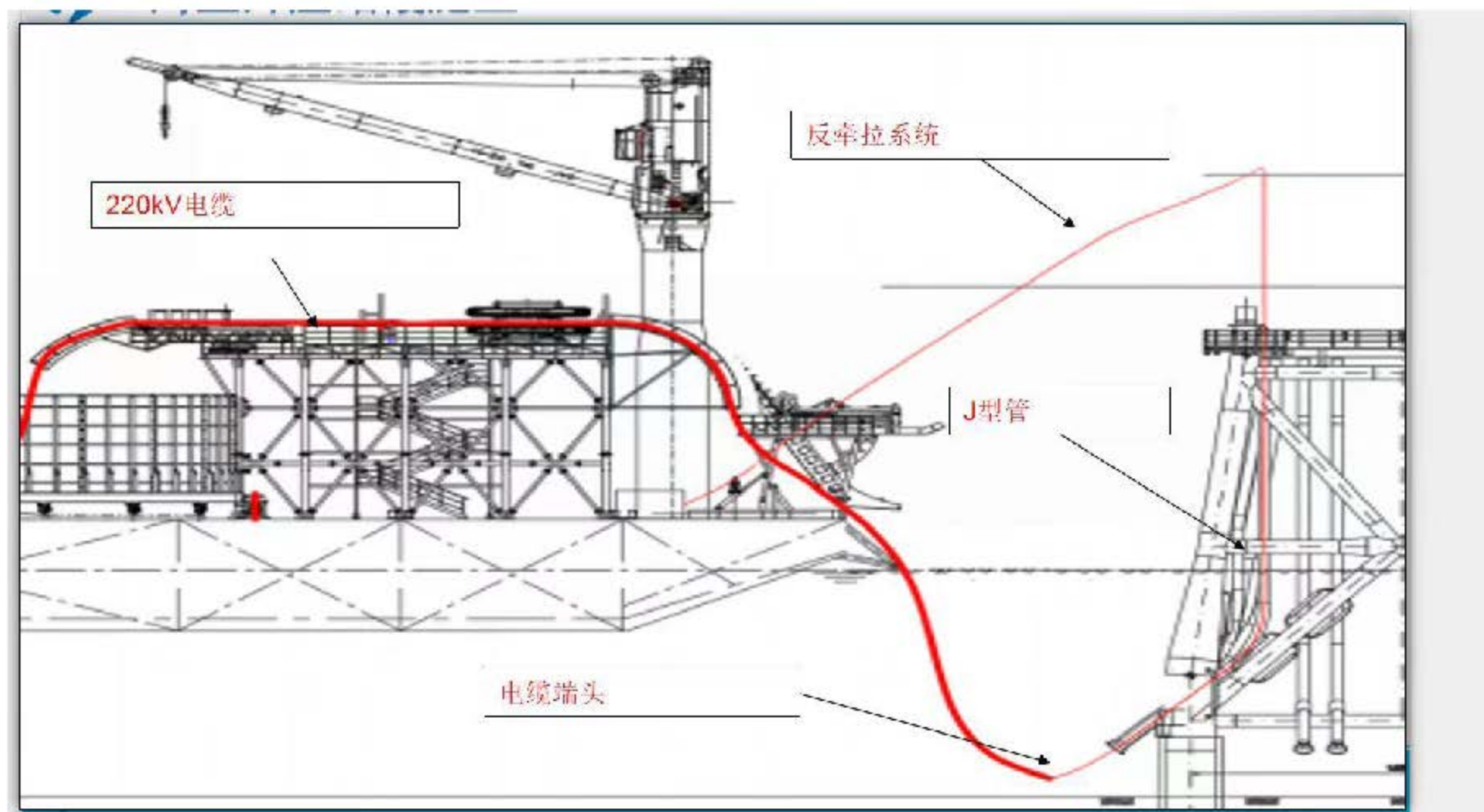
图 3.5.1-7 “J” 管式设计工艺图件
