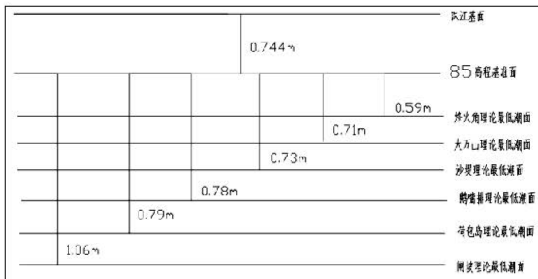
图 4.1.2-1 基面关系图
