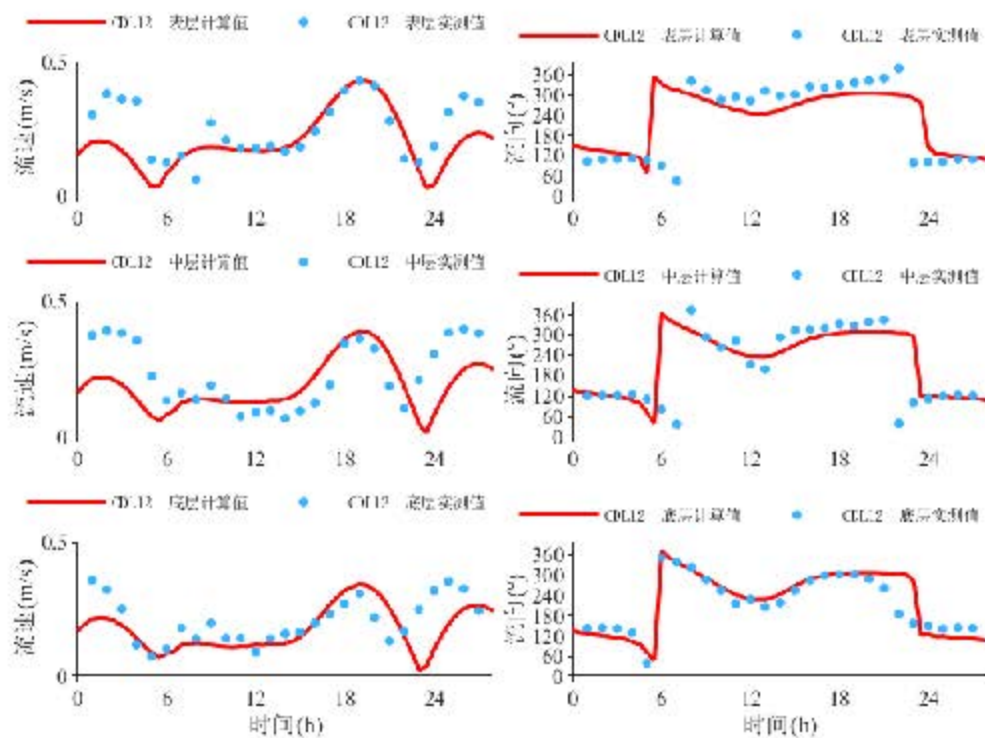
图 6.1.1-16 CDL12 站流速、流向验证 (冬季) (2023 年 12 月 13 日 1:00~14 日 3:00)
