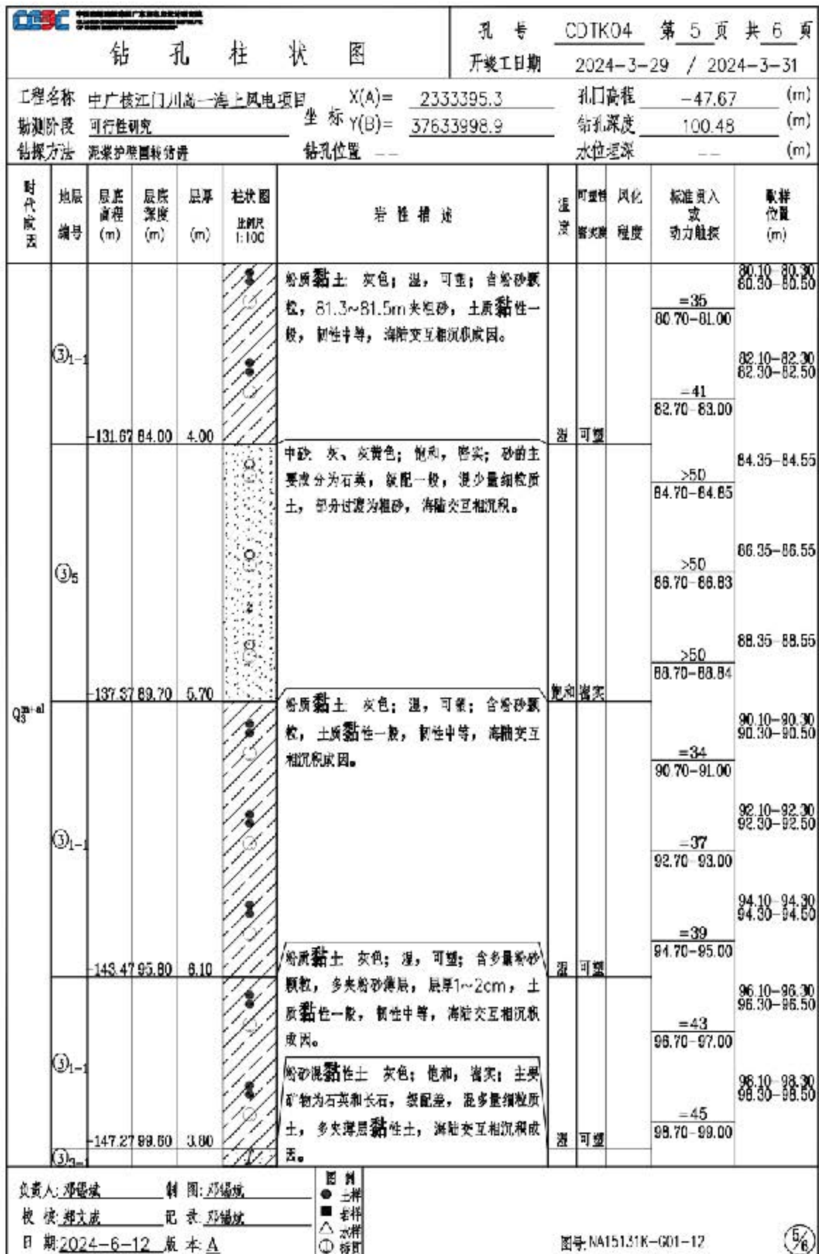
图 5.2.2-3e 钻孔柱状图 (CDTK04)
