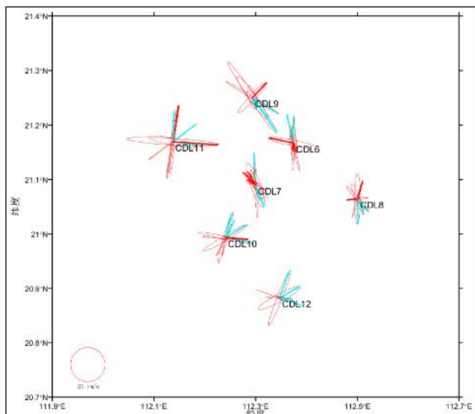
图 5.1.5-1b 冬季各站各层 K 1 分潮椭圆图
