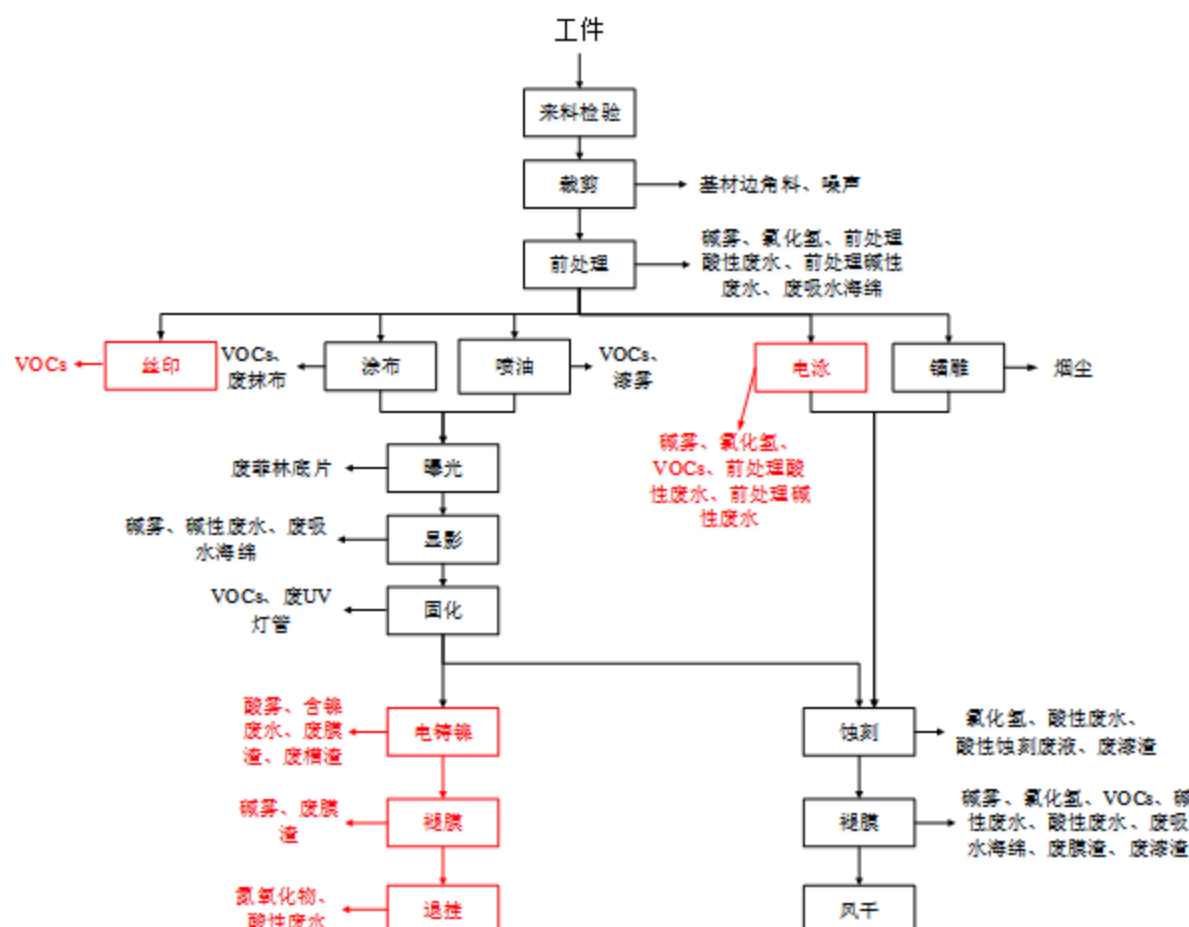
图 3.2-1 现有项目工艺流程及产污环节图（红色中丝印和电泳委外，电铸取消）
