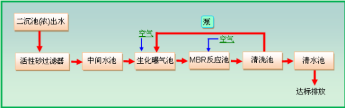
图 9.1-10 MBR 膜生物反应器系统处理工艺
