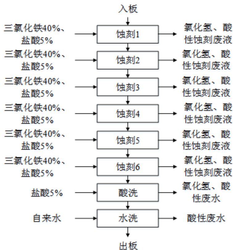
图 3.2-4 两条蚀刻线工艺流程及产污节点示意图
