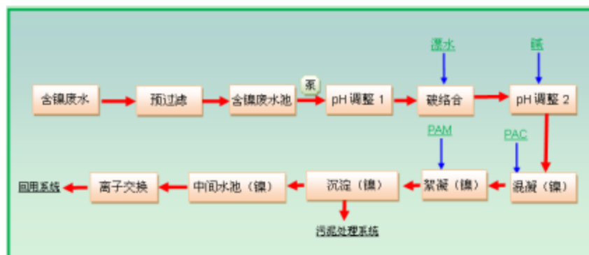
图 9.1-6 含镍废水系统处理工艺
