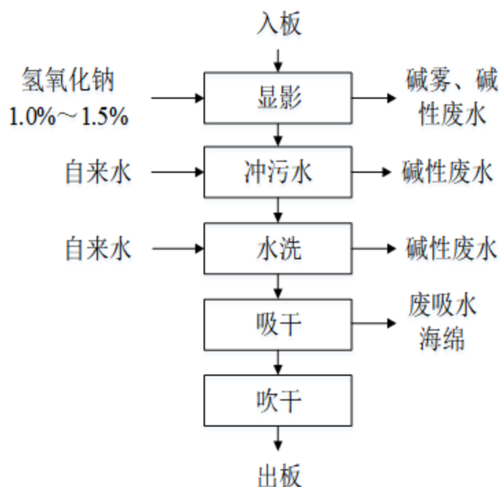
图 3.2-3 显影工艺流程及产污节点示意图
