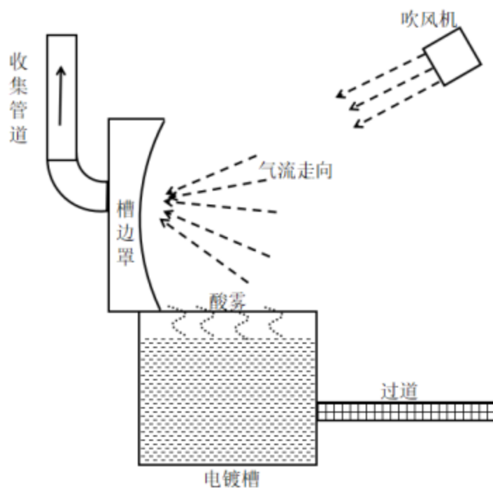
图 4.5-2 侧边吹气+槽边罩收集示意图
