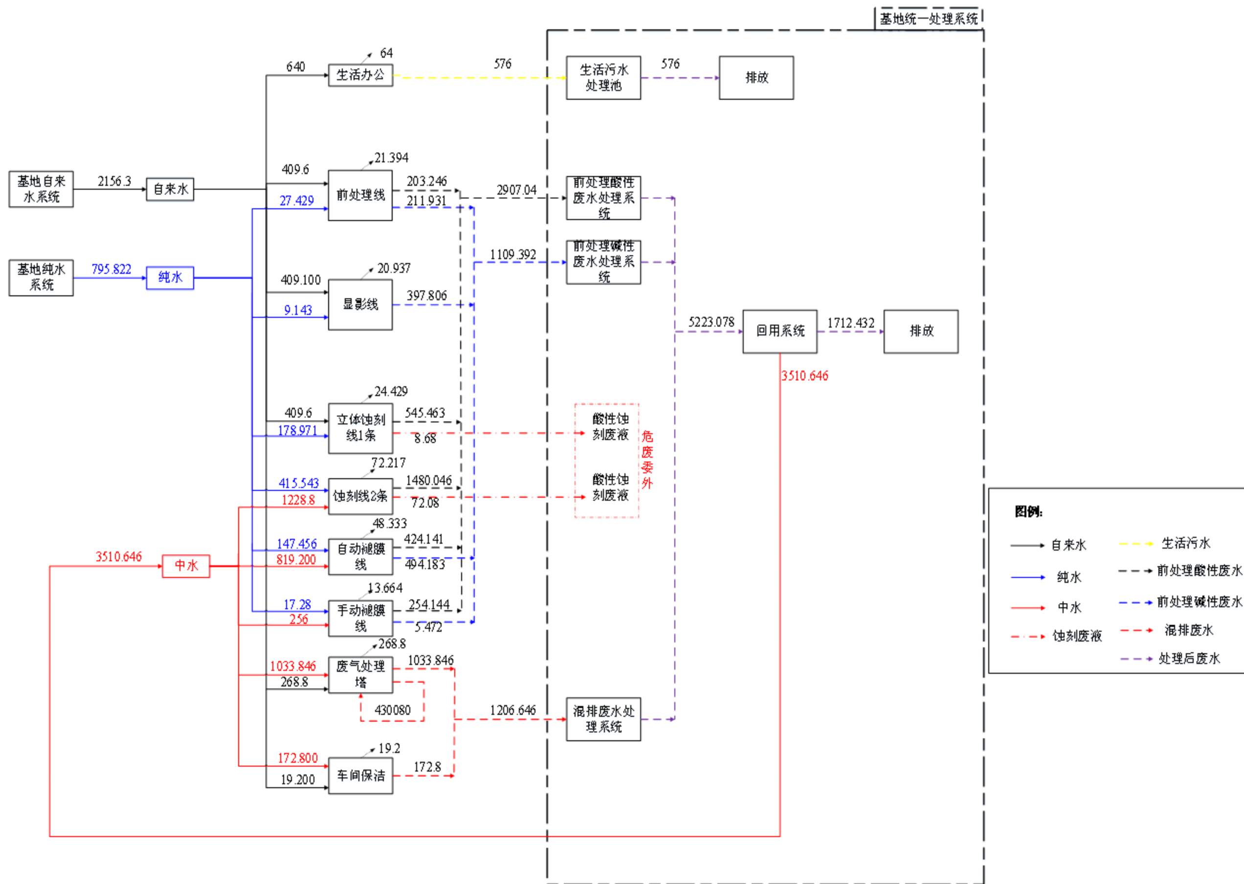
图 3.3-1 现有项目厂区用水平衡图 单位 m 3 /a
