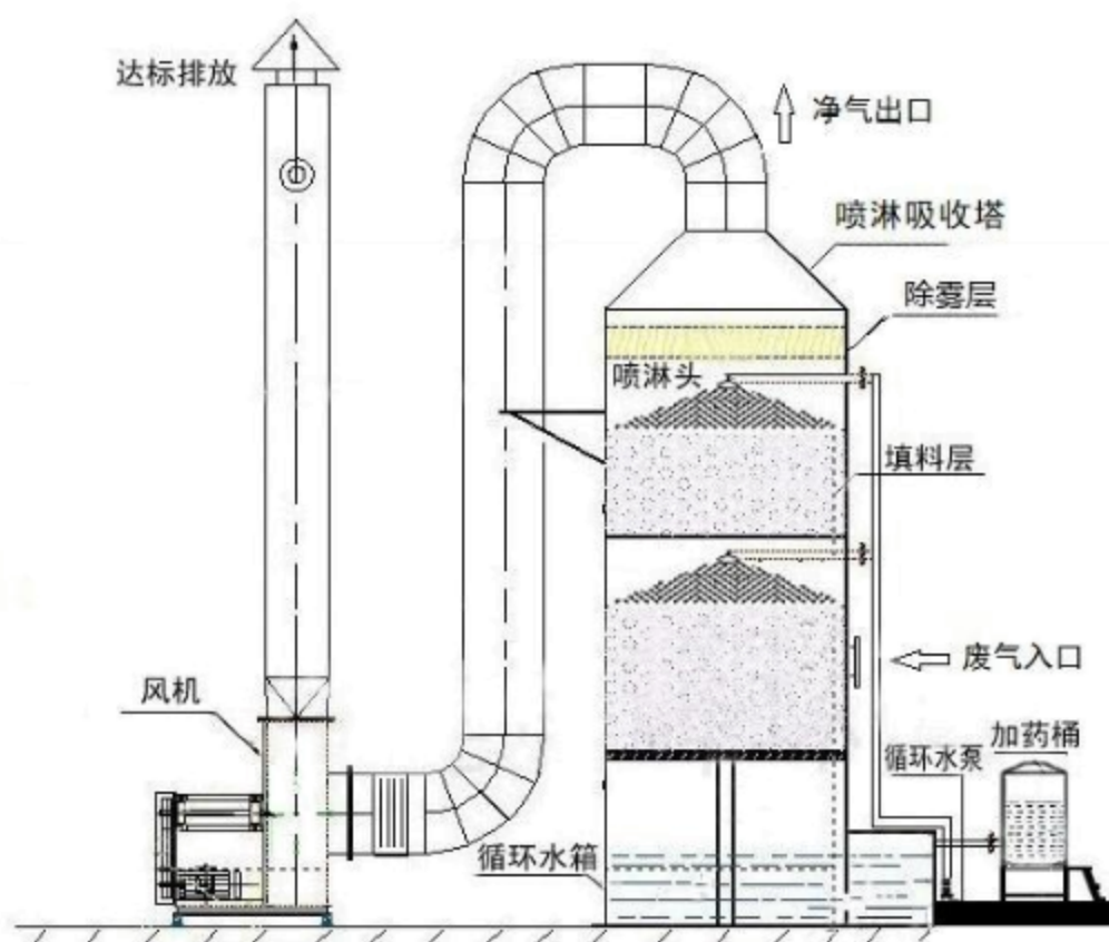
图 9.1-3 喷淋塔简图
