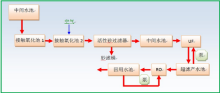
图 9.1-9 回用水系统处理工艺
