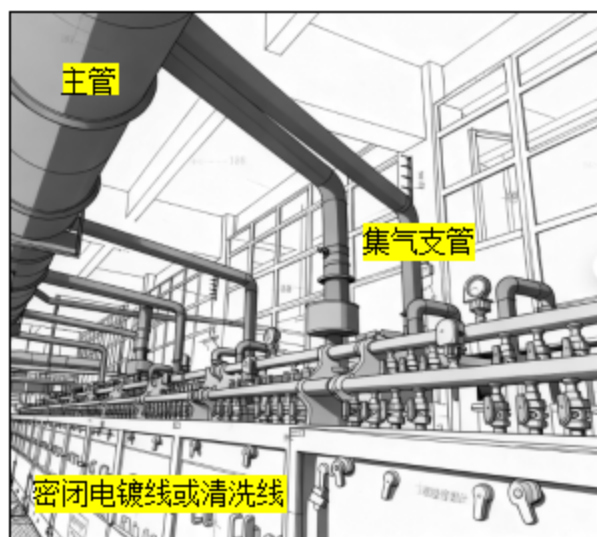
图 4.5-1 密闭式生产线废气收集示意图
