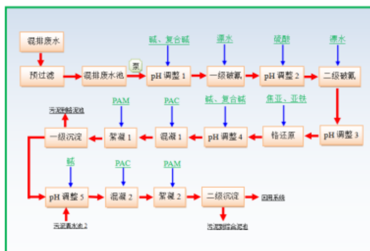
图 9.1-8 混排废水系统处理工艺
