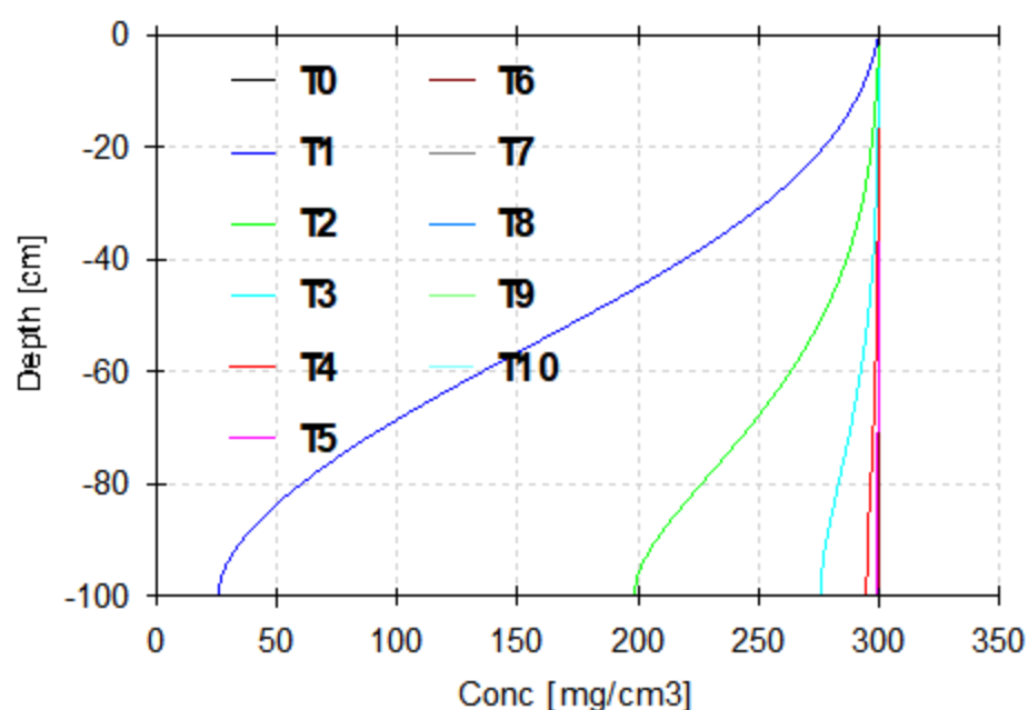
图 7.7-2 总镍在不同深度的浓度分布图 (T0~T10 为时间 0d、10d、20d、30d、40d、50d、60d、70d、80d、90d、100d)
