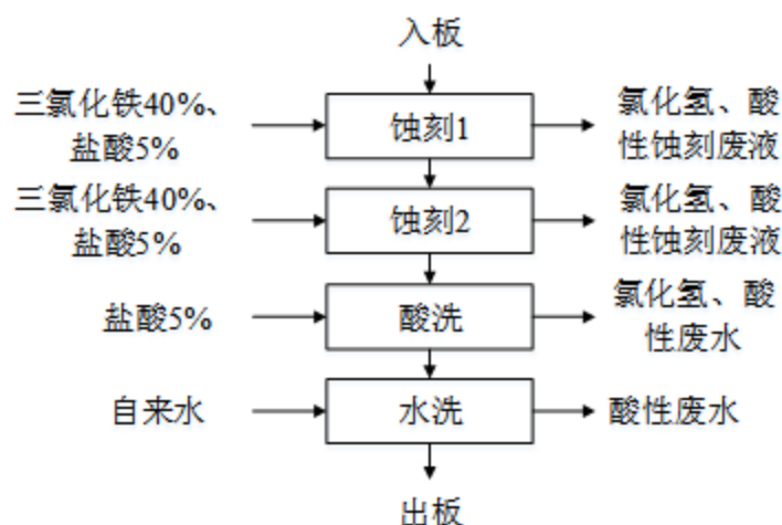
图 3.2-5 立体蚀刻线工艺流程及产污节点示意图
