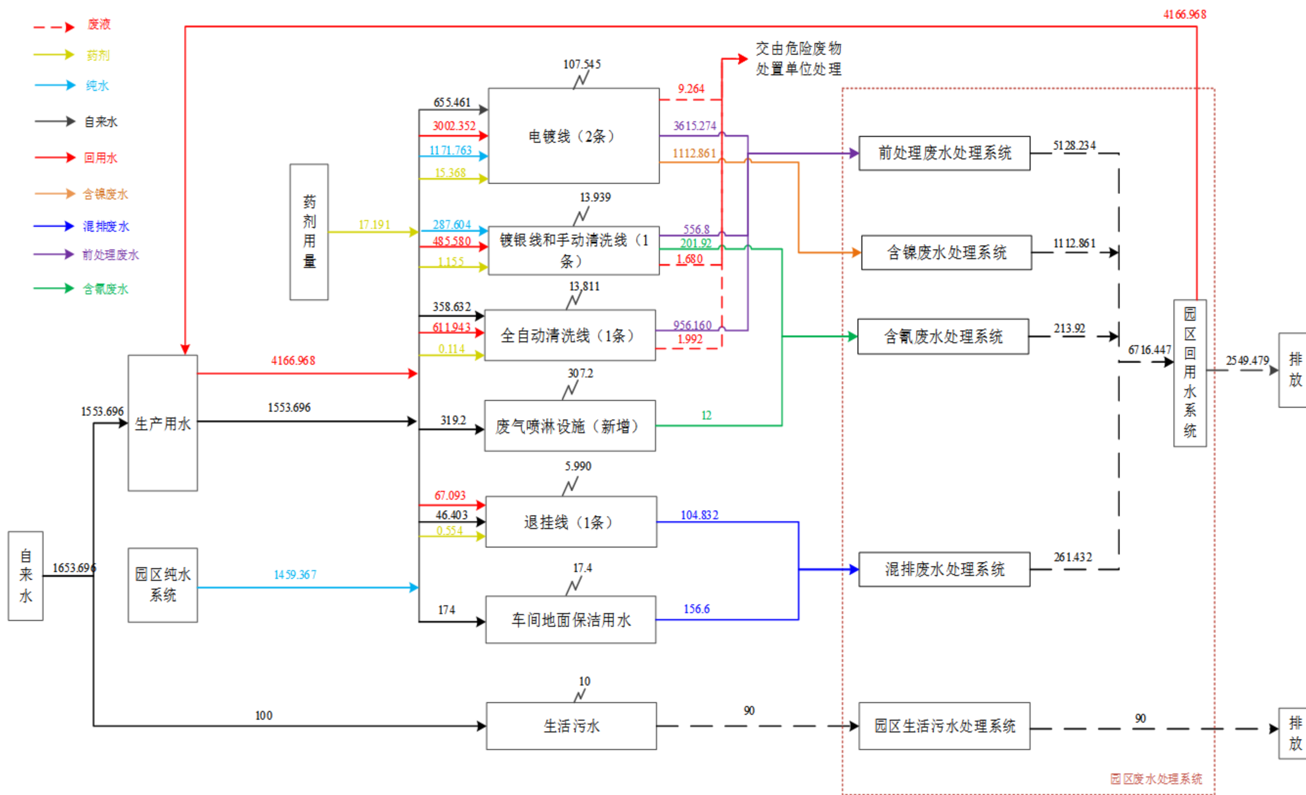
图 4.3-1 扩建项目水平衡图 (单位: \text{m}^3/\text{a} )
