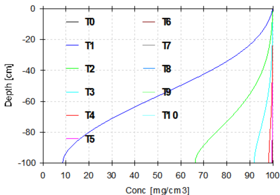
图 7.7-4 总铜在不同深度的浓度分布图 (T0~T10 为时间 0d、10d、20d、30d、40d、50d、60d、70d、80d、90d、100d)
