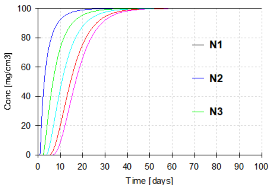
图 7.7-3 总铜在不同时间的浓度分布图 (N1~N6 为深度 0m、0.2m、0.4m、0.6m、0.8m、1.0m)
