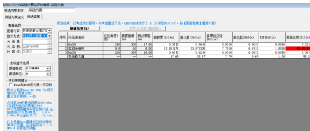
图 2.6-2 1 小时浓度占标率预测结果截图
