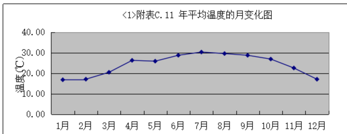
图 7.1-2 2024 年新会平均温度月变化曲线
