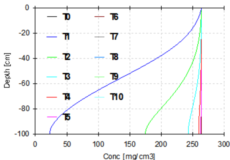
图 7.7-6 氰化物在不同深度的浓度分布图 (T0~T10 为时间 0d、10d、20d、30d、40d、50d、60d、70d、80d、90d、100d)
