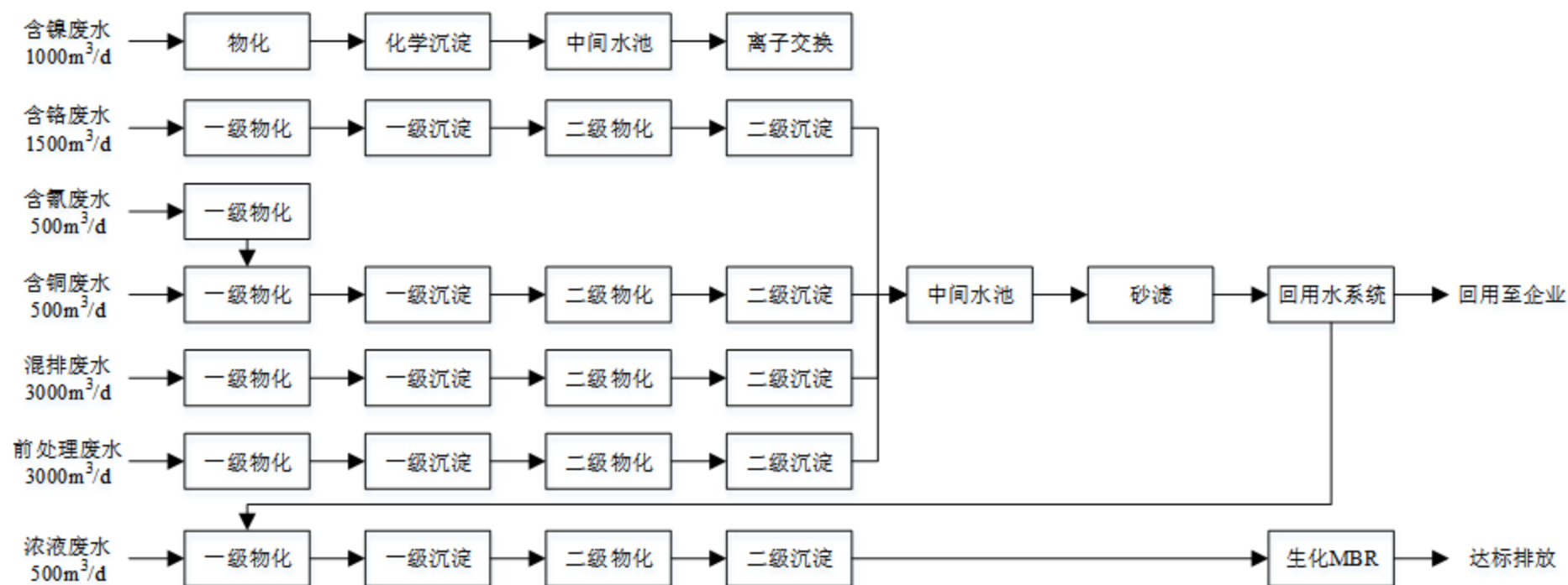
图 7.2-1 新财富环保产业园污水处理厂二期污水处理工艺流程图
