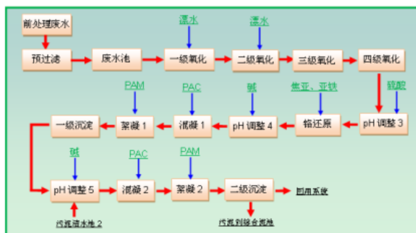
图9.1-5 前处理废水系统处理工艺
