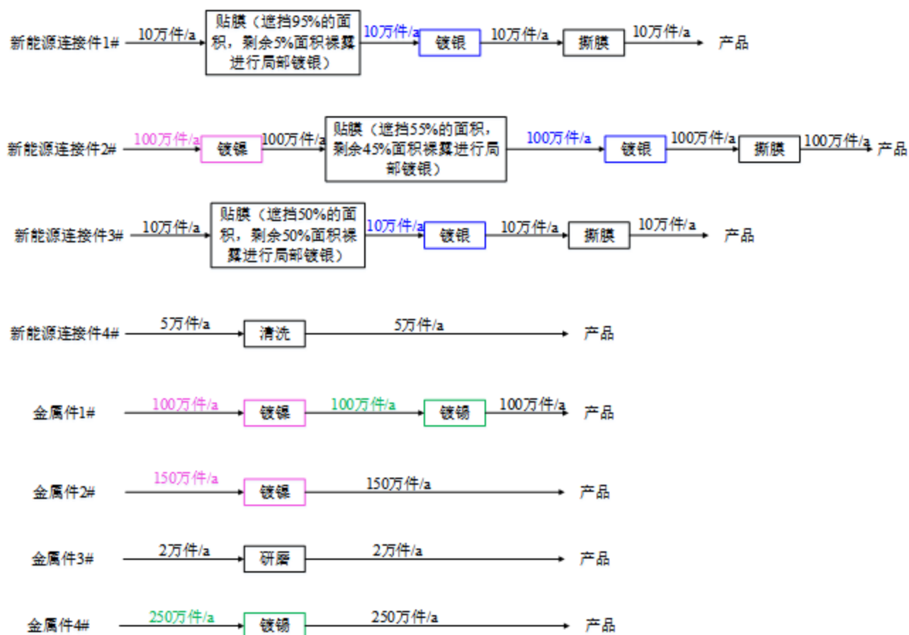
图 4.1-5 改扩建项目产品表面处理示意图
