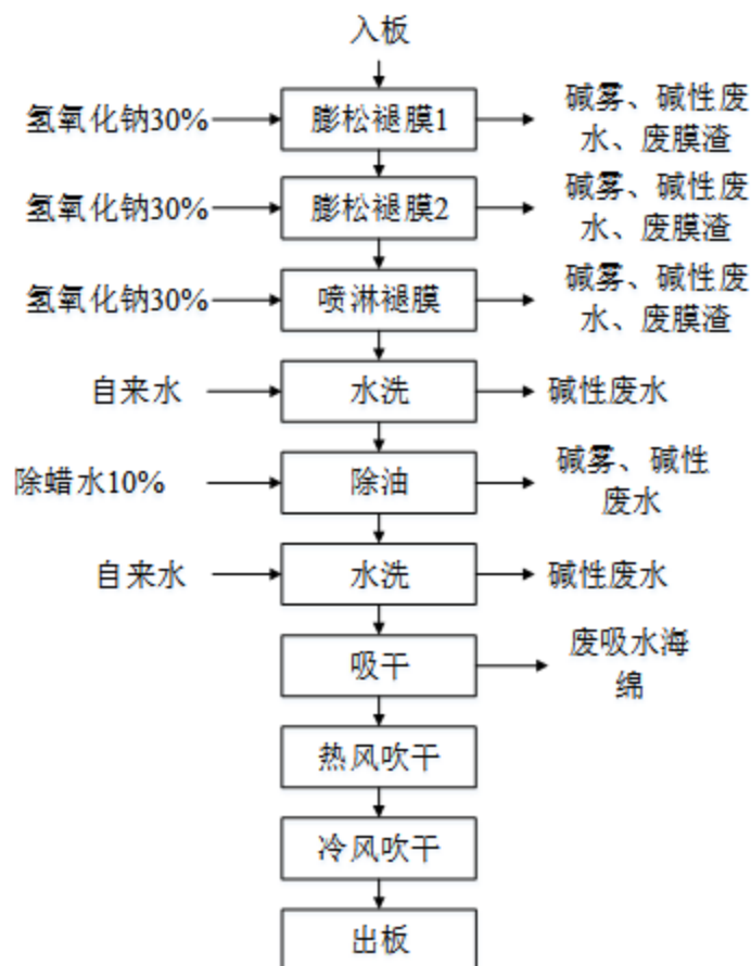
图 3.2-6 自动褪膜工段工艺流程及产污节点示意图
