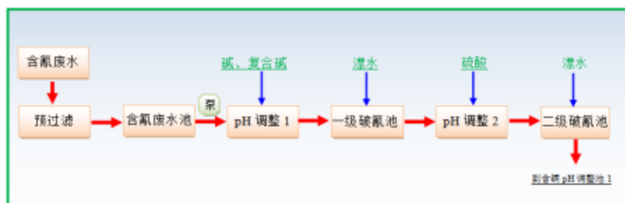
图 9.1-7 含氰废水处理工艺
