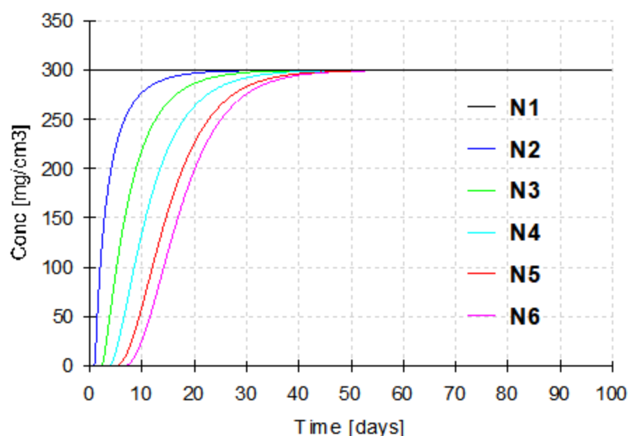
图 7.7-1 总镍在不同时间的浓度分布图 (N1~N6 为深度 0m、0.2m、0.4m、0.6m、0.8m、1.0m)
