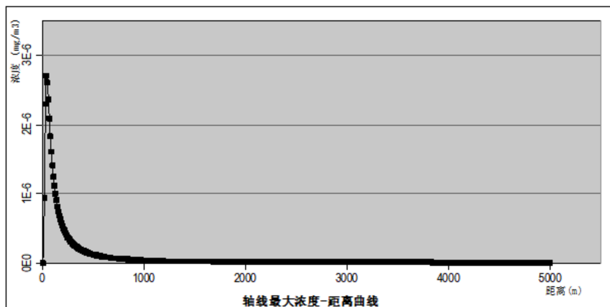
图 8.7-1 最不利气象条件下硫酸泄漏下风向不同距离处的最大浓度
