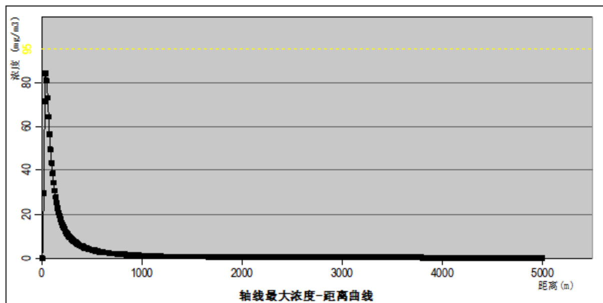
图 8.7-7 最不利气象条件下燃烧产生 CO 下风向不同距离处的最大浓度
