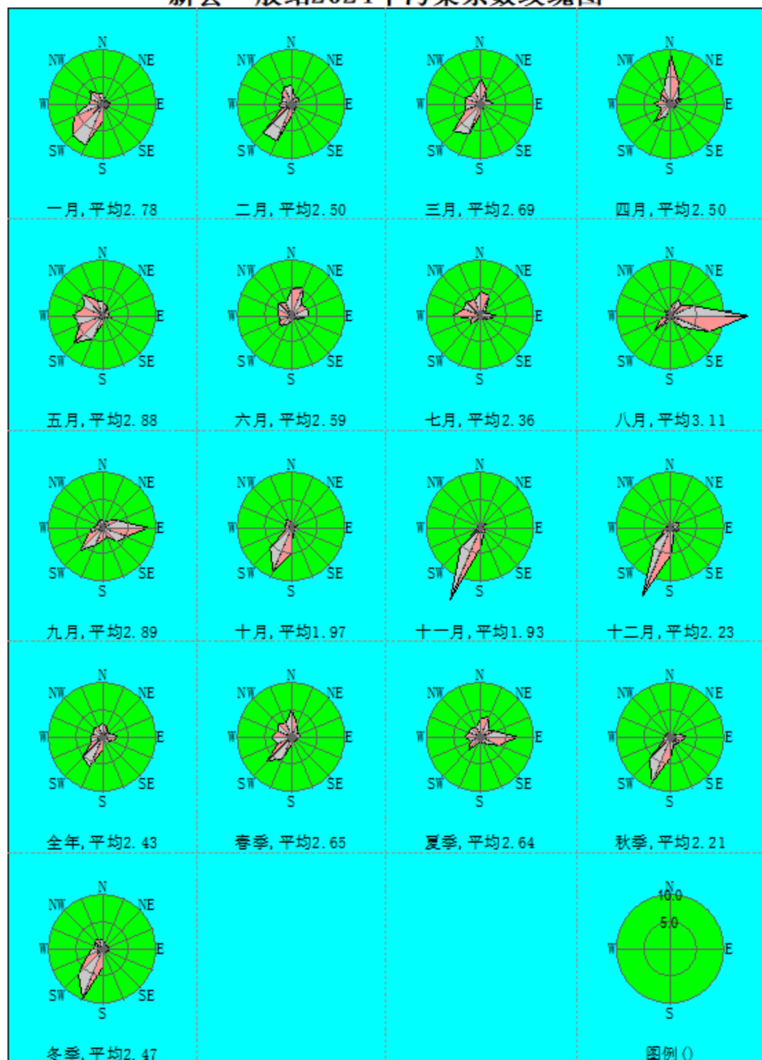
图 7.1-7 2024 年新会污染系数玫瑰图
