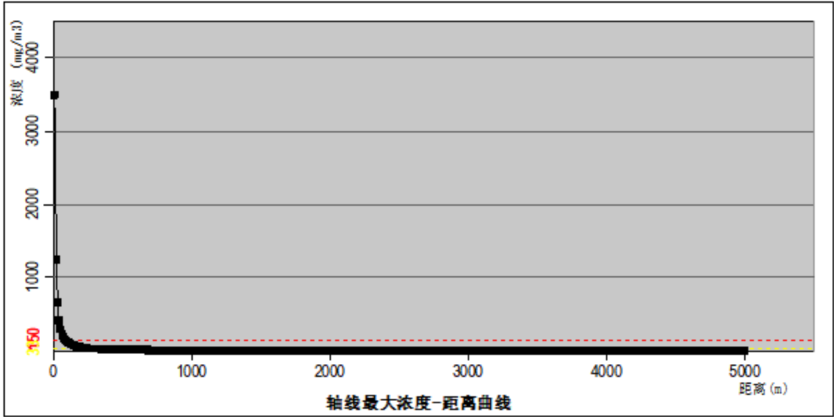
图 8.7-3 最不利气象条件下泄漏产生氯化氢下风向不同距离处的最大浓度
