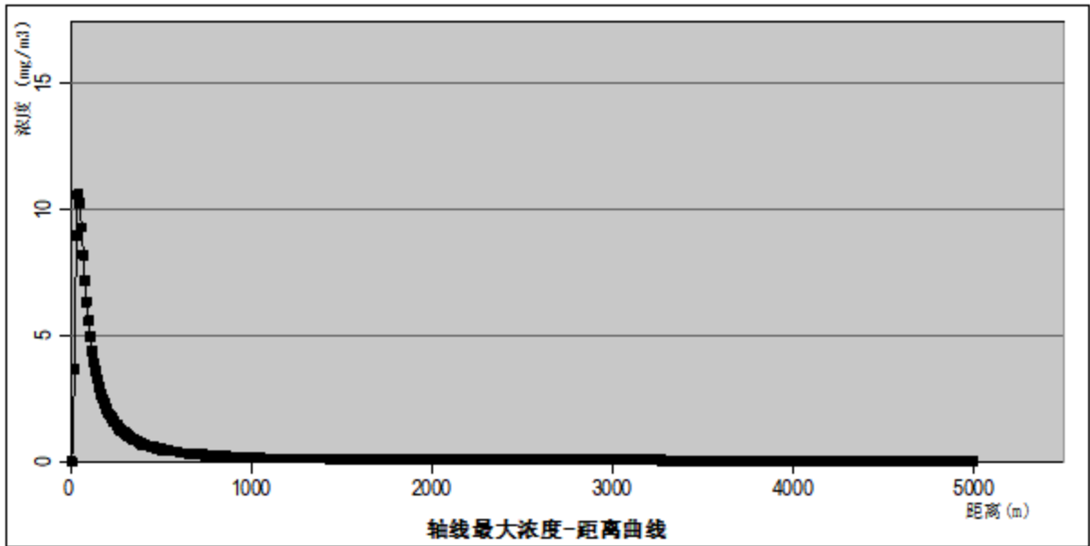
图 8.7-2 最不利气象条件下硝酸泄漏下风向不同距离处的最大浓度
