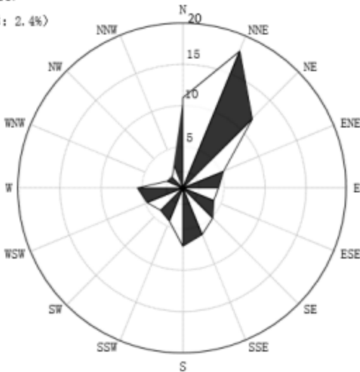
图 7.1-1 新会气象站累年各风向玫瑰图（统计年限：2005-2024 年）
