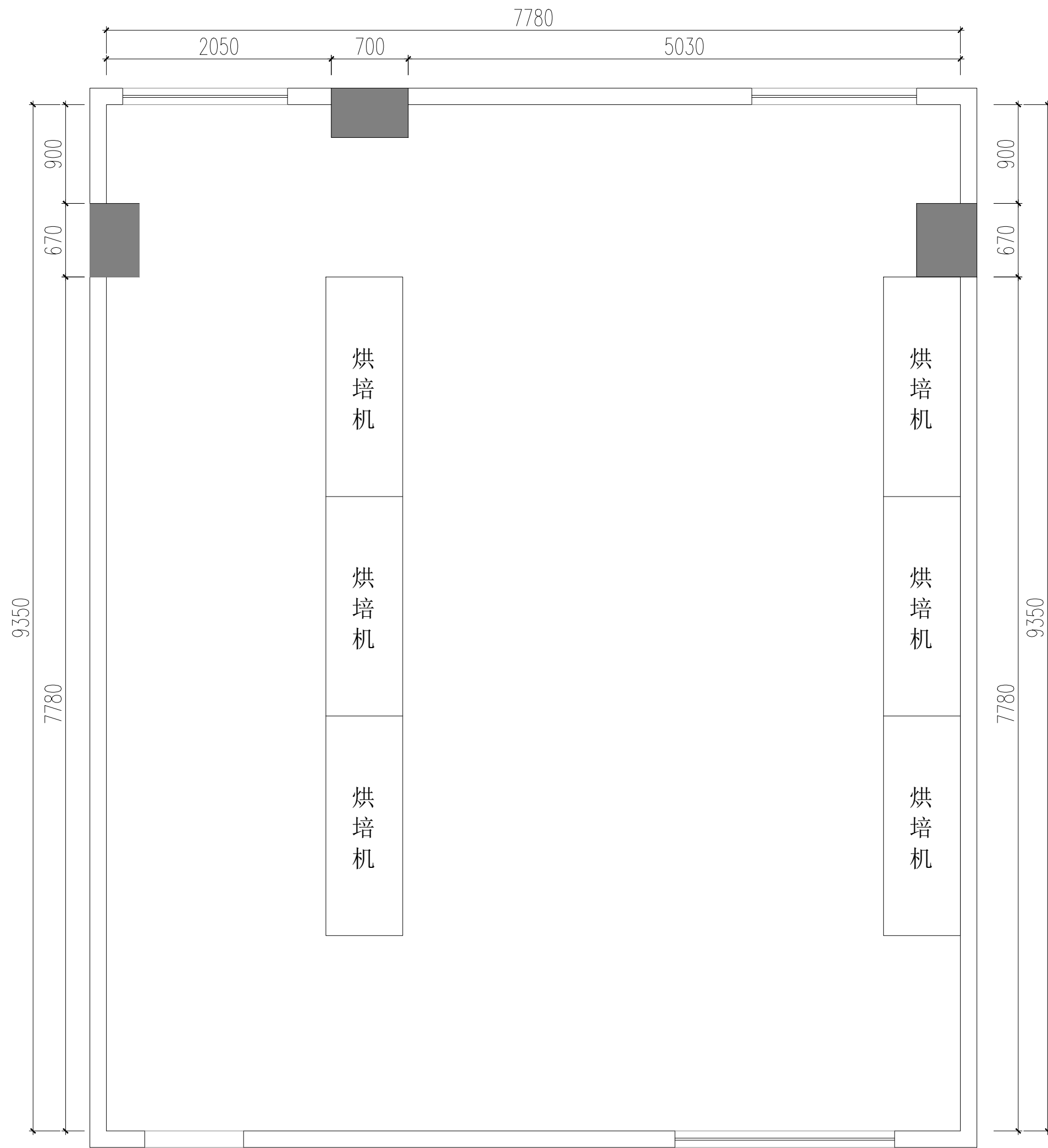
平面布置图
