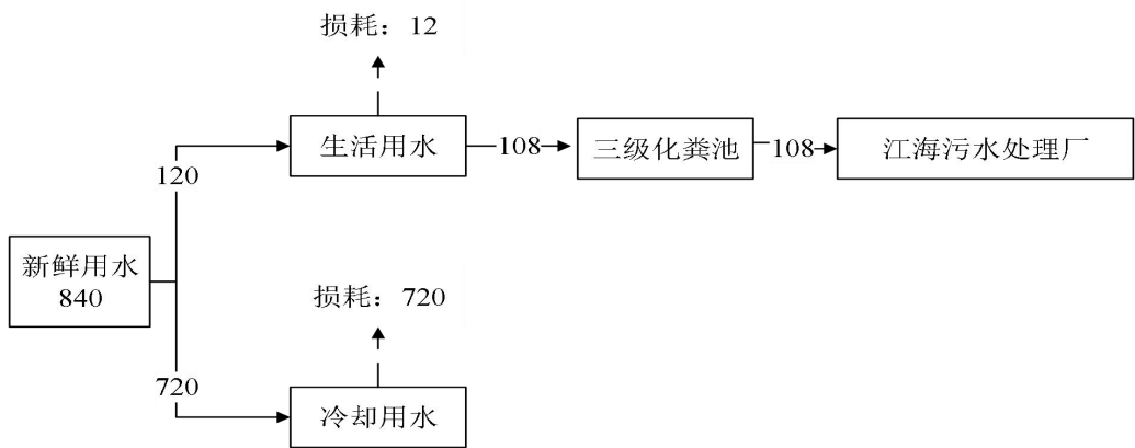
图 2-1 项目水平衡图（ \text{m}^3/\text{a} ）
