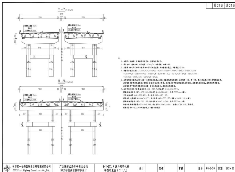
图 2.3.3-4 桥型布置结构图
