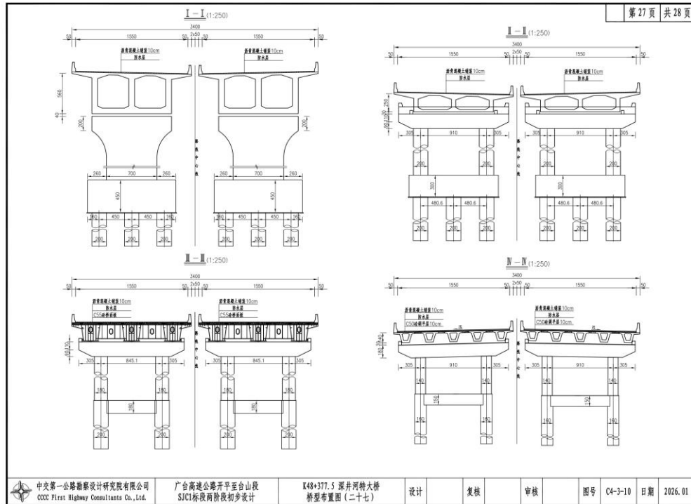
图 2.3.3-3 桥型布置结构图
