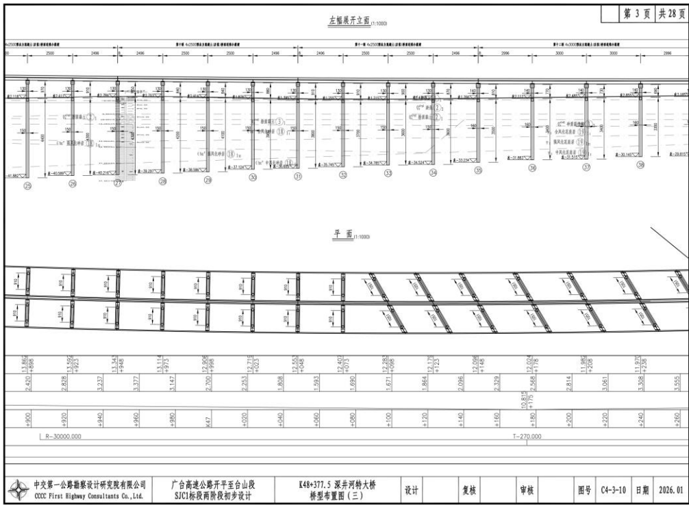
图 2.3.3-1c 桥型布置图
