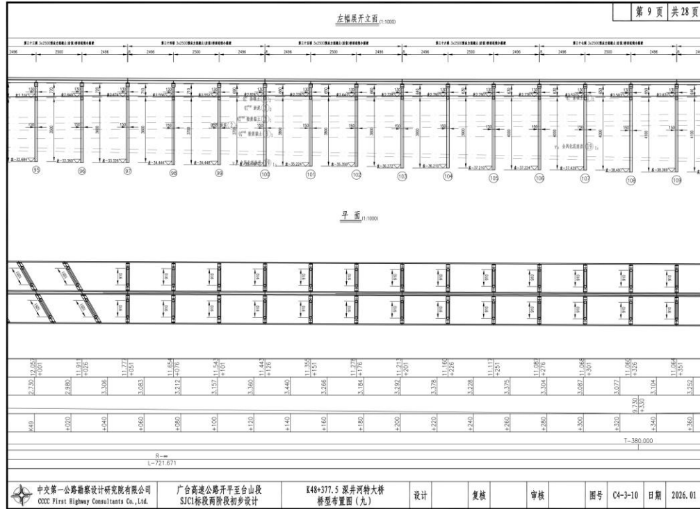
图 2.3.3-1i 桥型布置图
