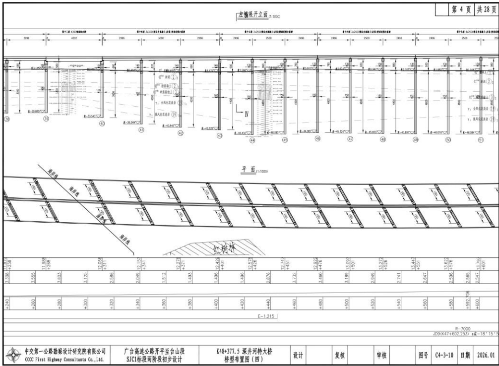
图 2.3.3-1d 桥型布置图
