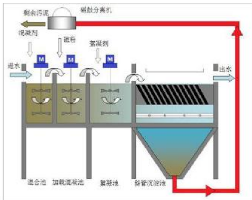
图 3.4-5 磁混凝沉淀池原理简图
