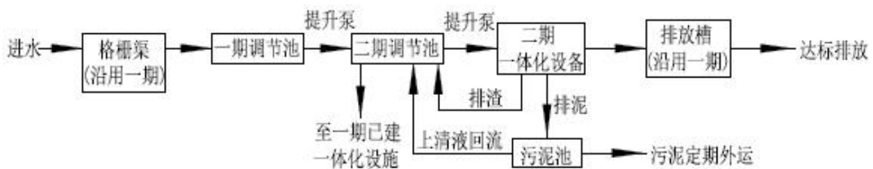
图 4.2-8 赤水镇污水处理厂污水处理工艺流程图
