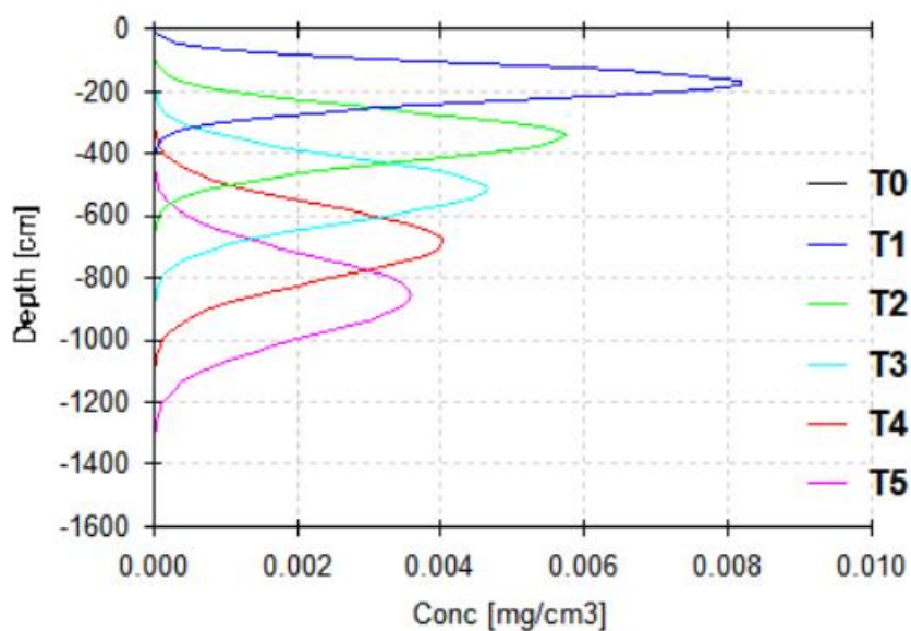
图 6.6-1 不同时间 COD Cr 浓度与垂向深度变化曲线图
