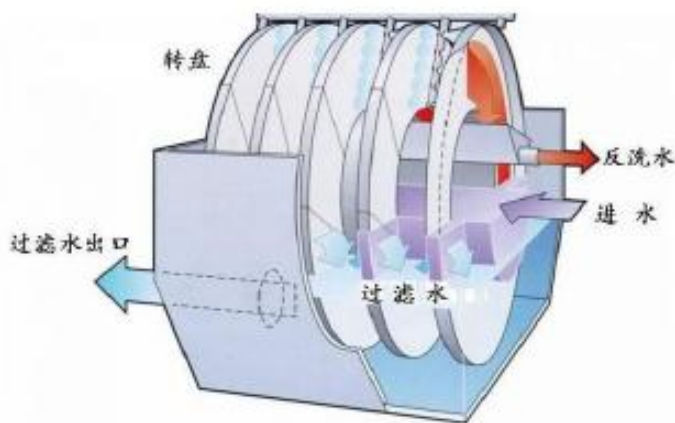
图 3.4-6 转盘过滤工作原理图
