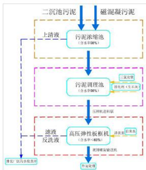
图 3.4-7 污泥脱水工艺流程图
