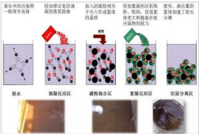
图 3.4-4 磁混凝沉淀池工艺原理
