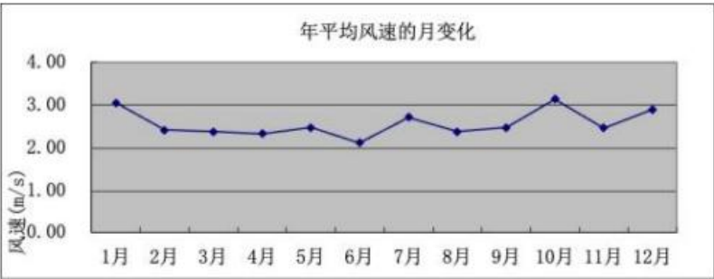
图 5.2-16 新会 2022 年平均风速月变化曲线图
