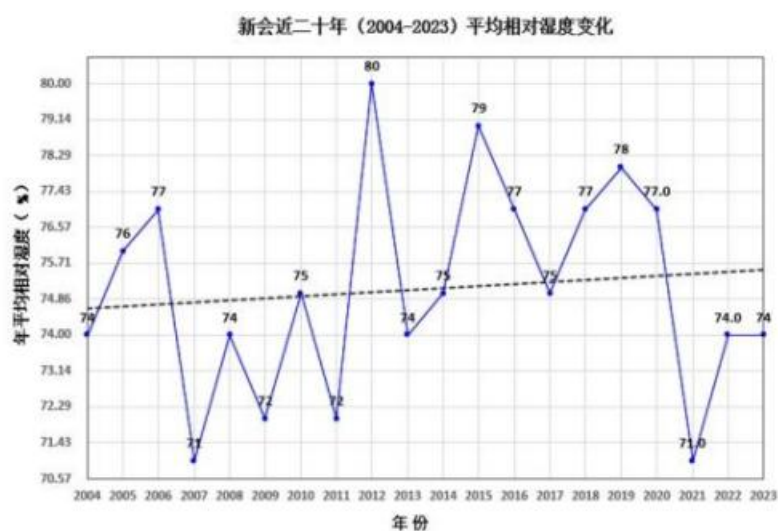
图 5.2-14 新会（2004-2023）年平均相对湿度（纵轴为百分比，虚线为趋势线）
