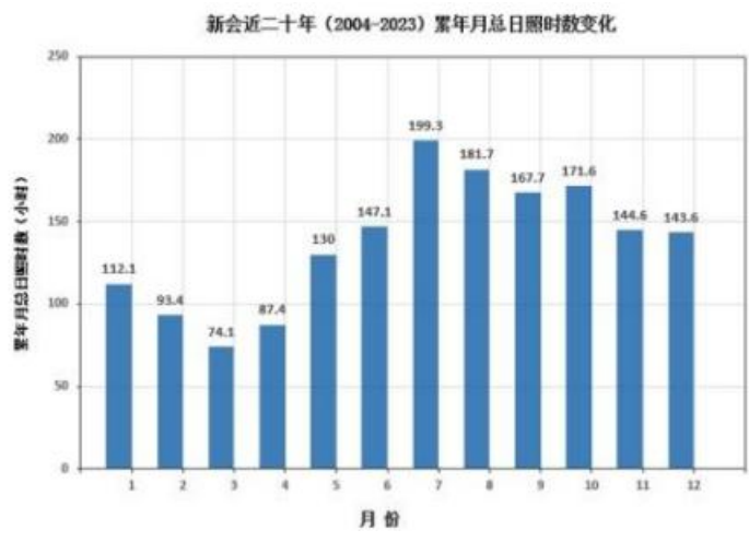
图 5.2-11新会月日照时数统计图（单位：小时）
