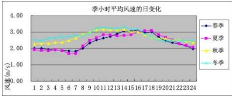
图 5.2-17 新会 2022 年各季小时平均风速日变化曲线图
