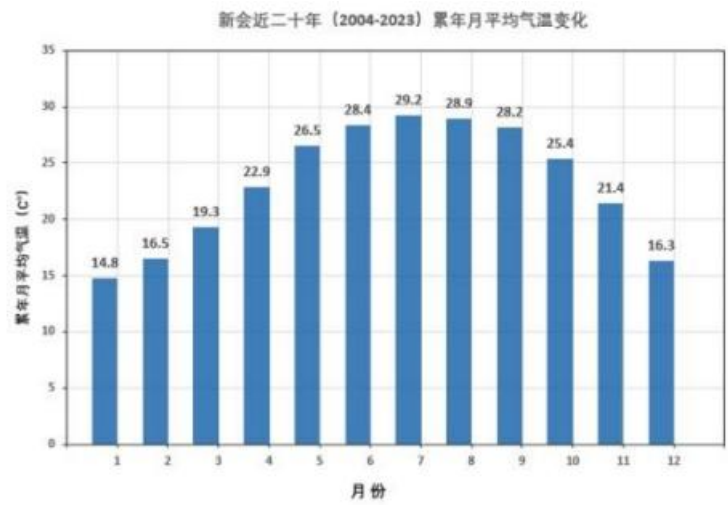
图 5.2-7 新会近 20 年月平均气温统计情况 （单位：℃）
