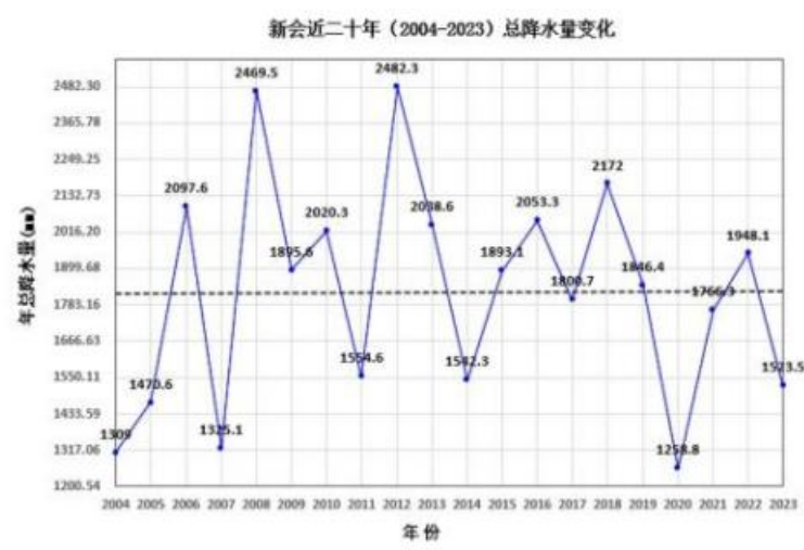
图 5.2-10新会（1999-2019）年总降水量（单位：毫米，虚线为趋势线）
