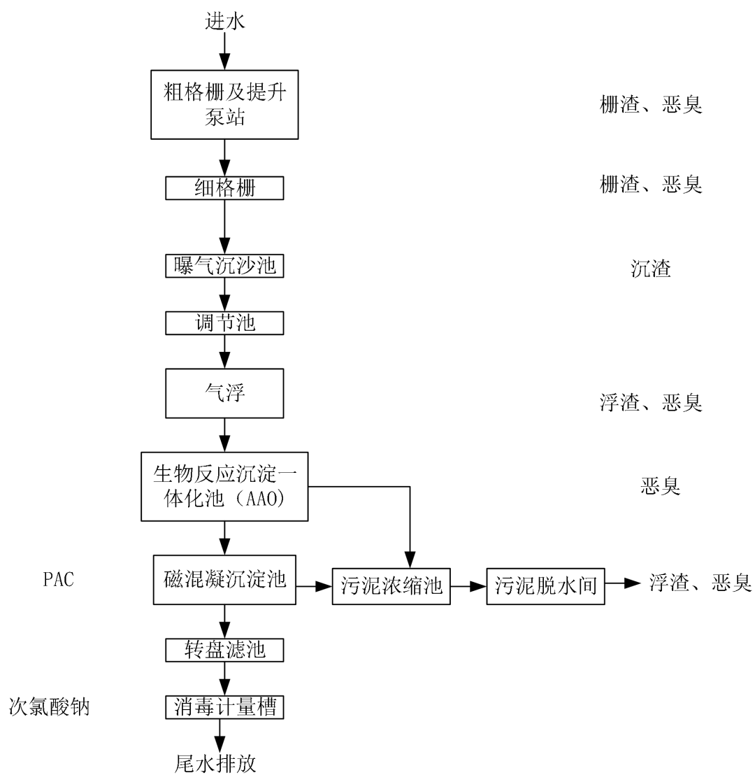
图 3.4-1 工艺流程图
