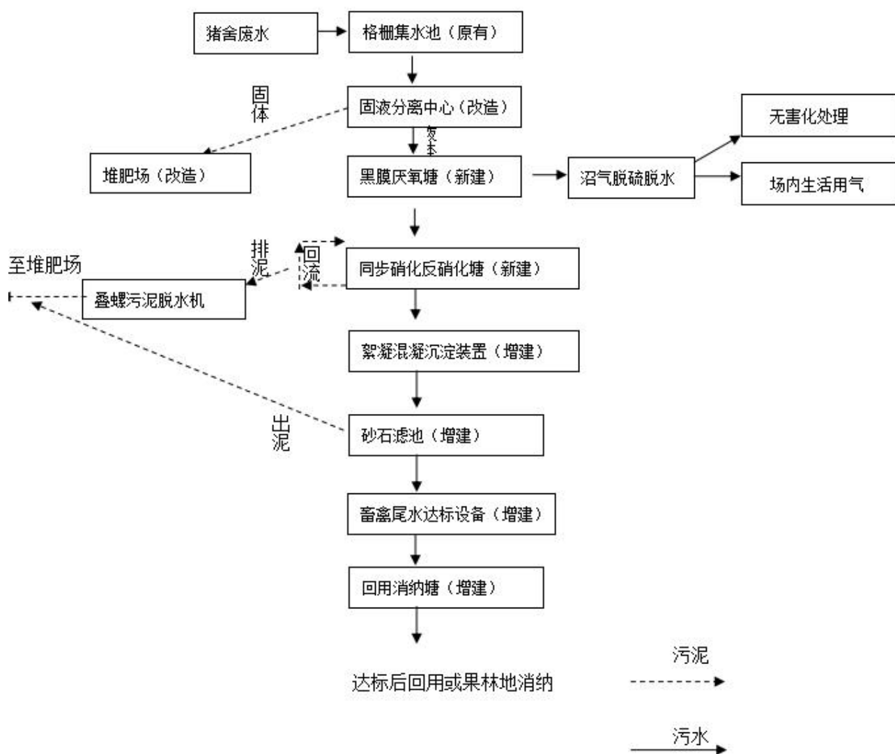
总体工艺流程图
