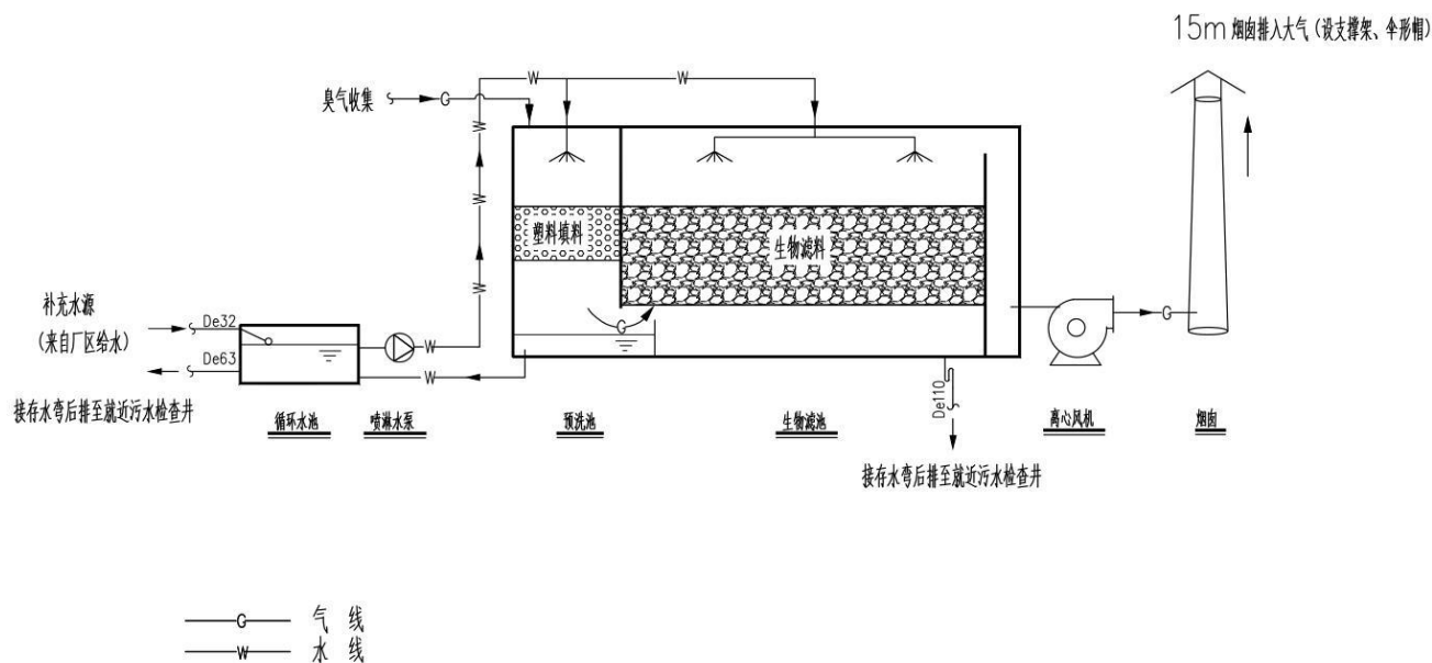
图 7.3-1 植物提取液喷淋+生物过滤除臭设施工艺流程图
