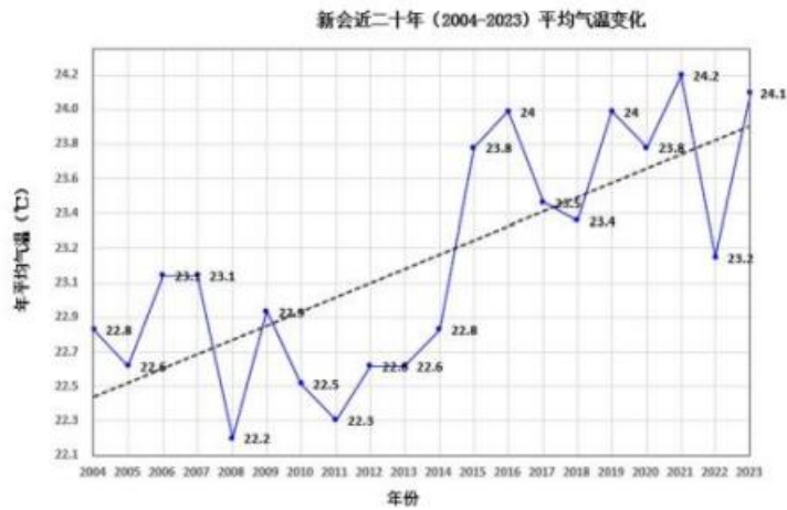
图 5.2-8 新会（2004-2023）年平均气温 （单位：℃，虚线为趋势线）
