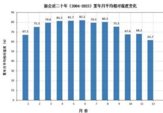
图 5.2-13新会近 20 年月平均相对湿度统计结果（纵轴为百分比）
