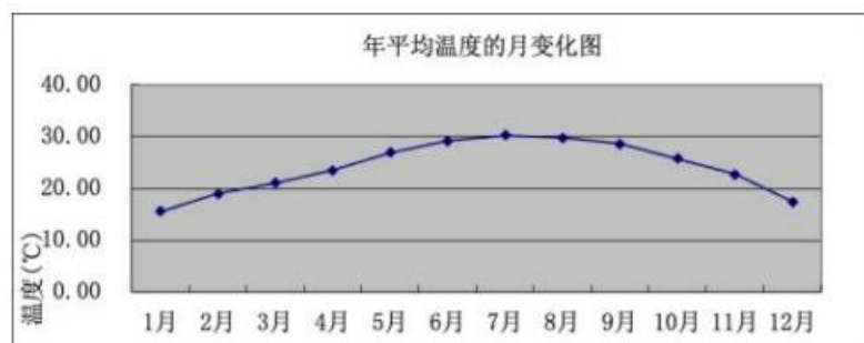
图 5.2-15 新会 2023 年平均温度月变化曲线图
