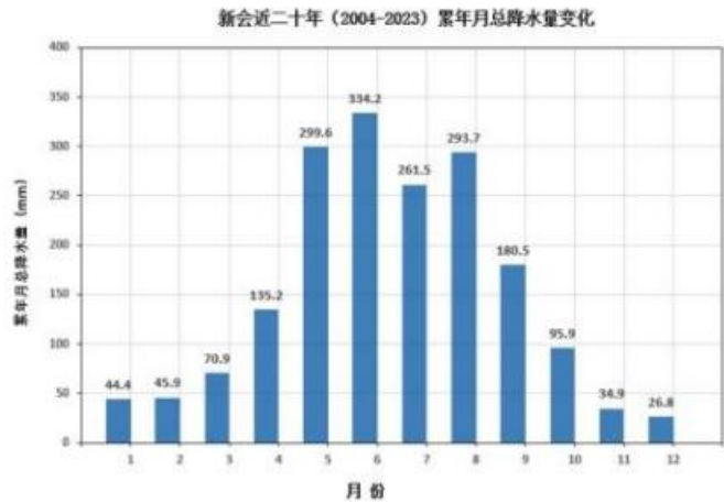
图 5.2-9新会近 20 年月平均降水量（单位：毫米）
