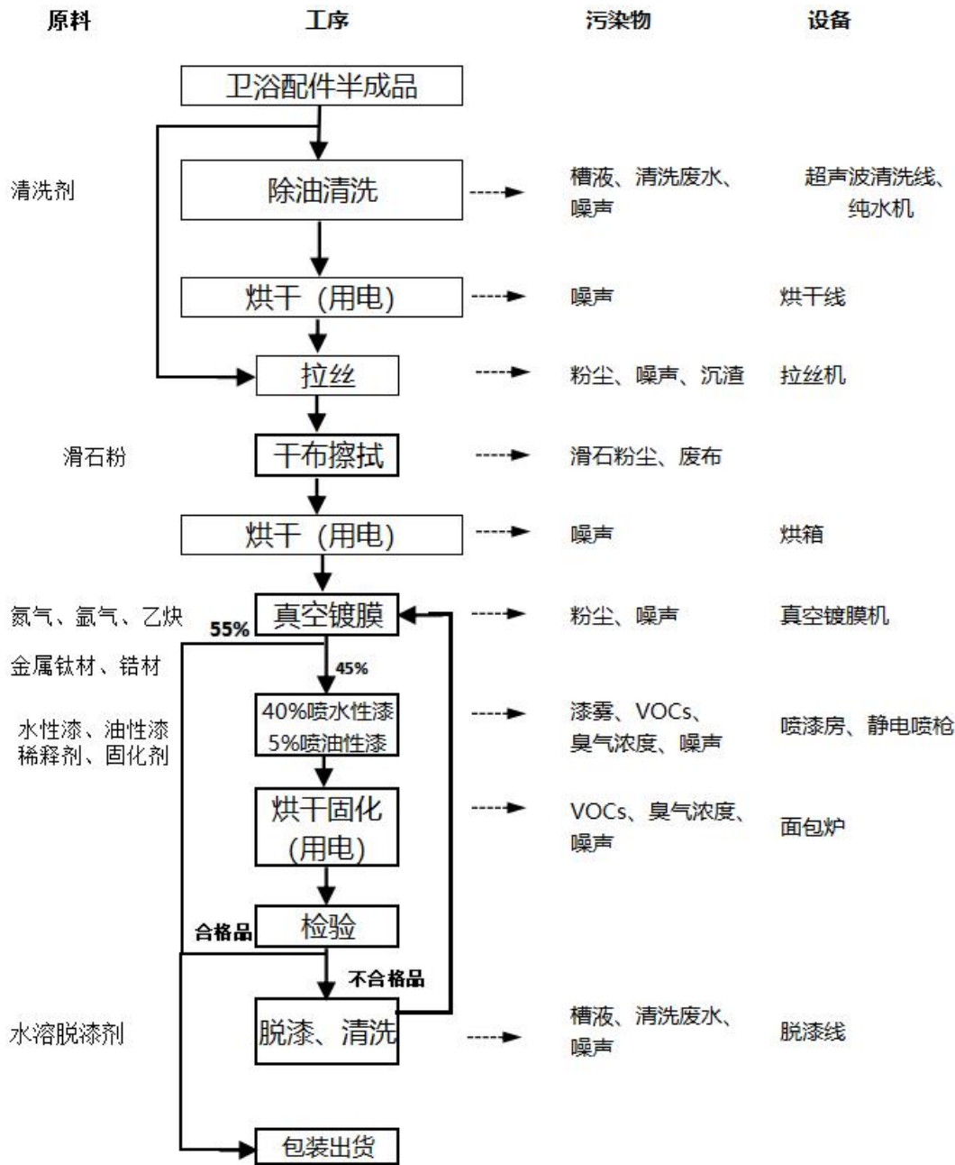
图 2-2 项目工艺流程及产污环节图
