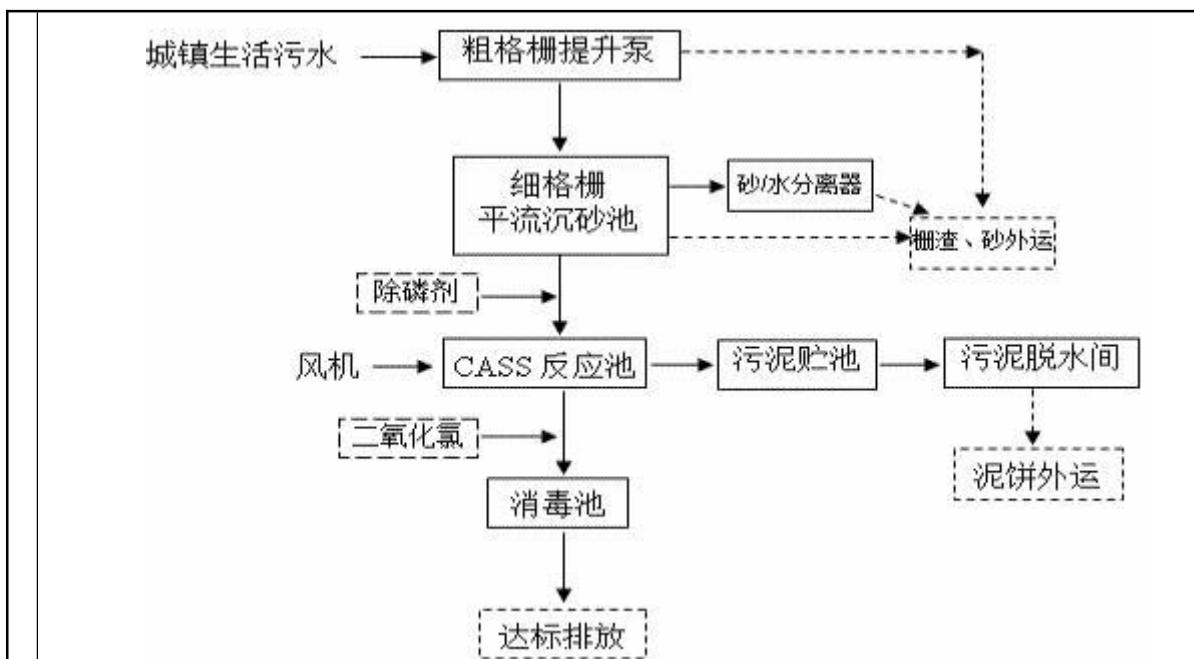
图 4-1 污水处理厂的处理工艺流程图
