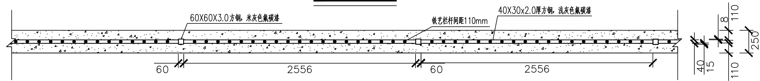
围墙改造标准平面图
