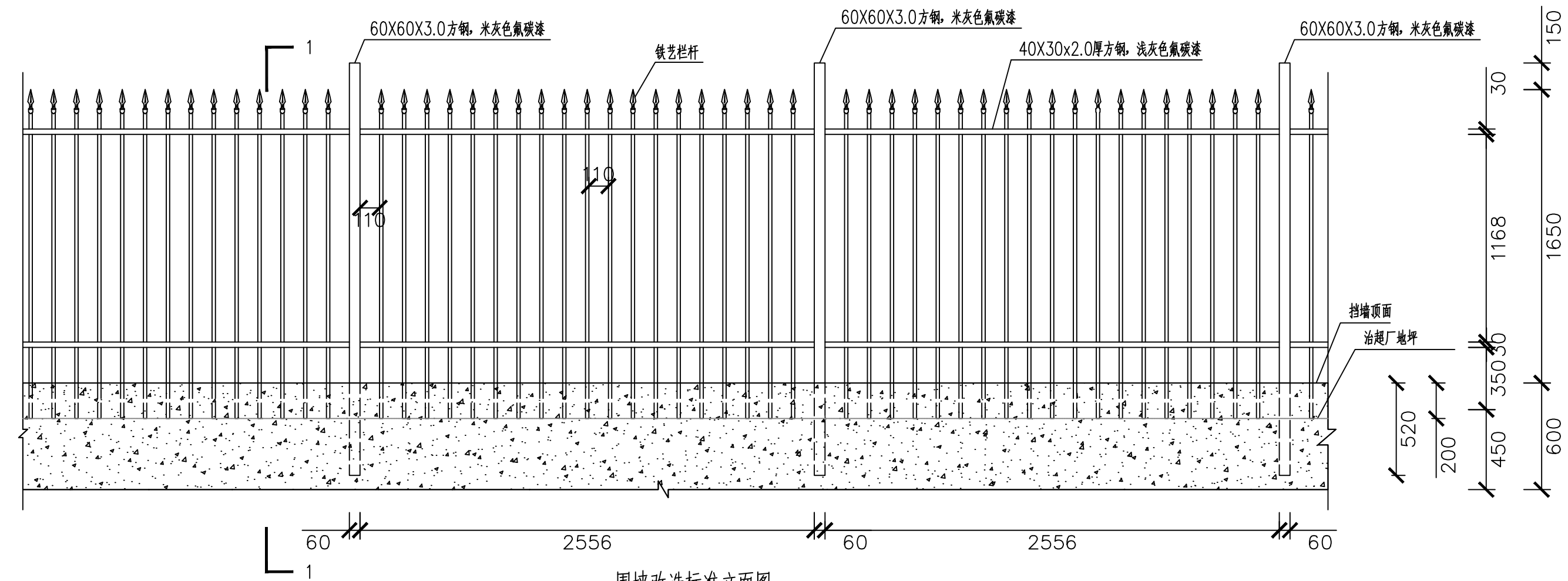
围墙改造标准立面图
