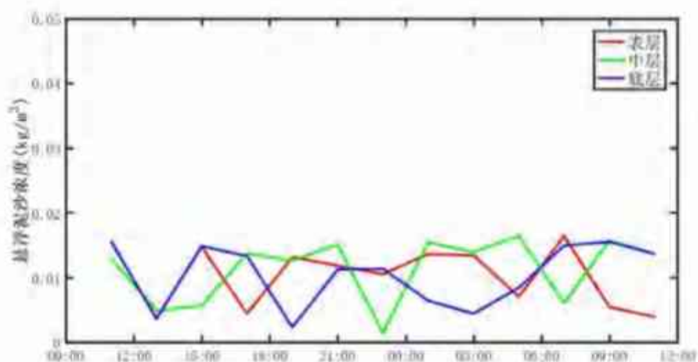
图 5.1.3-9f V6 站悬浮泥沙浓度曲线
