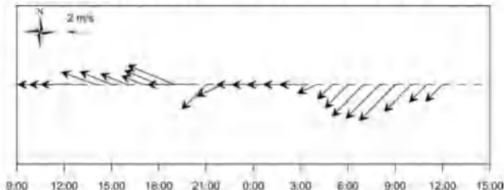
图 5.1.2-1 调查海域大潮期 V6 站实测风速风向图
