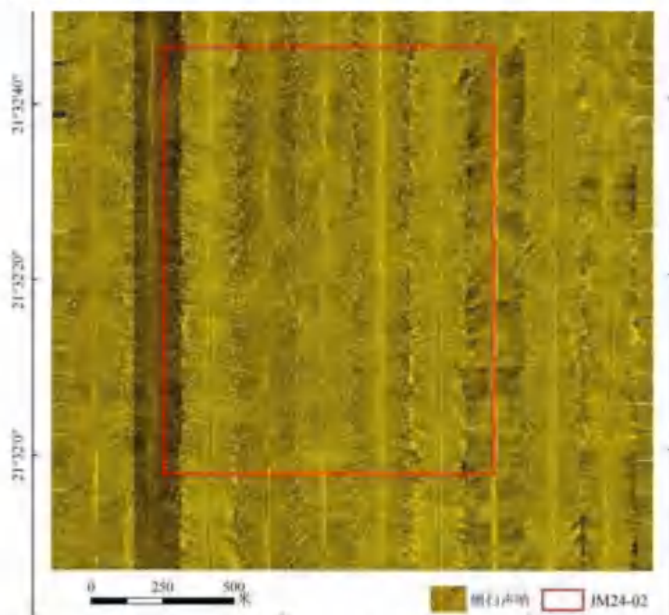
图 5.2.2-1 矿区海底侧扫声呐图
