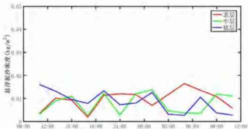
图 5.1.3—9d V4 站悬浮泥沙浓度曲线
