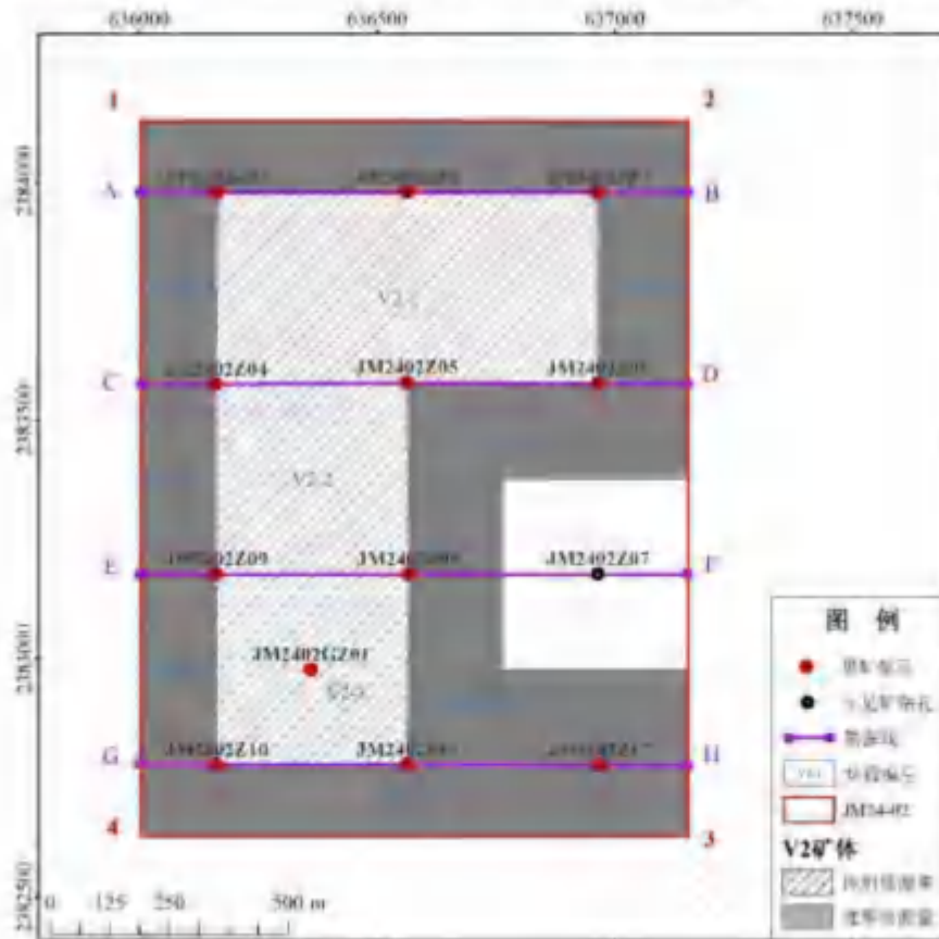
图 3.1.3-2 V2 矿体平面分布图
