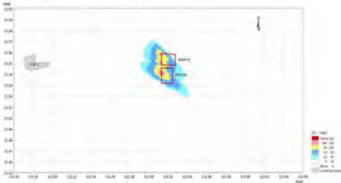
图6.3.4-13两个采砂区块同时施工增量悬浮泥沙最大浓度平面分布（底层）
