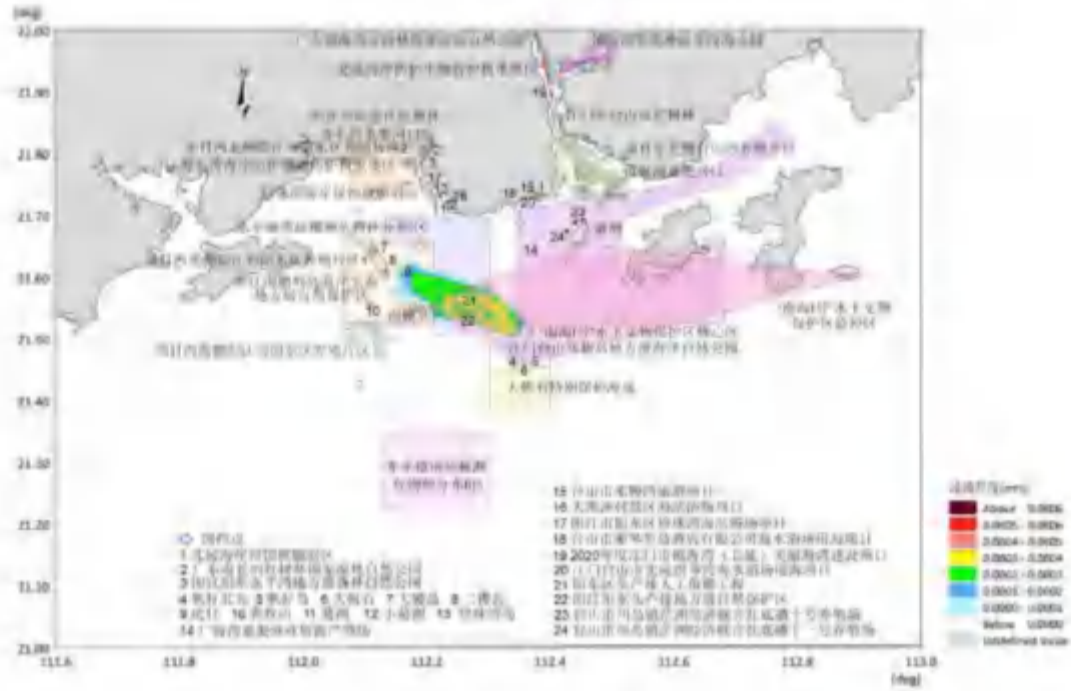
图 7.3.3-1 冬季 E 风向、13.8m/s 大潮涨初发生溢油 48 小时油膜扫海范围图
