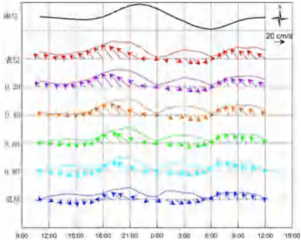
图 5.1.3-2a 调查海域大潮期 V1 站实测海流矢量图
