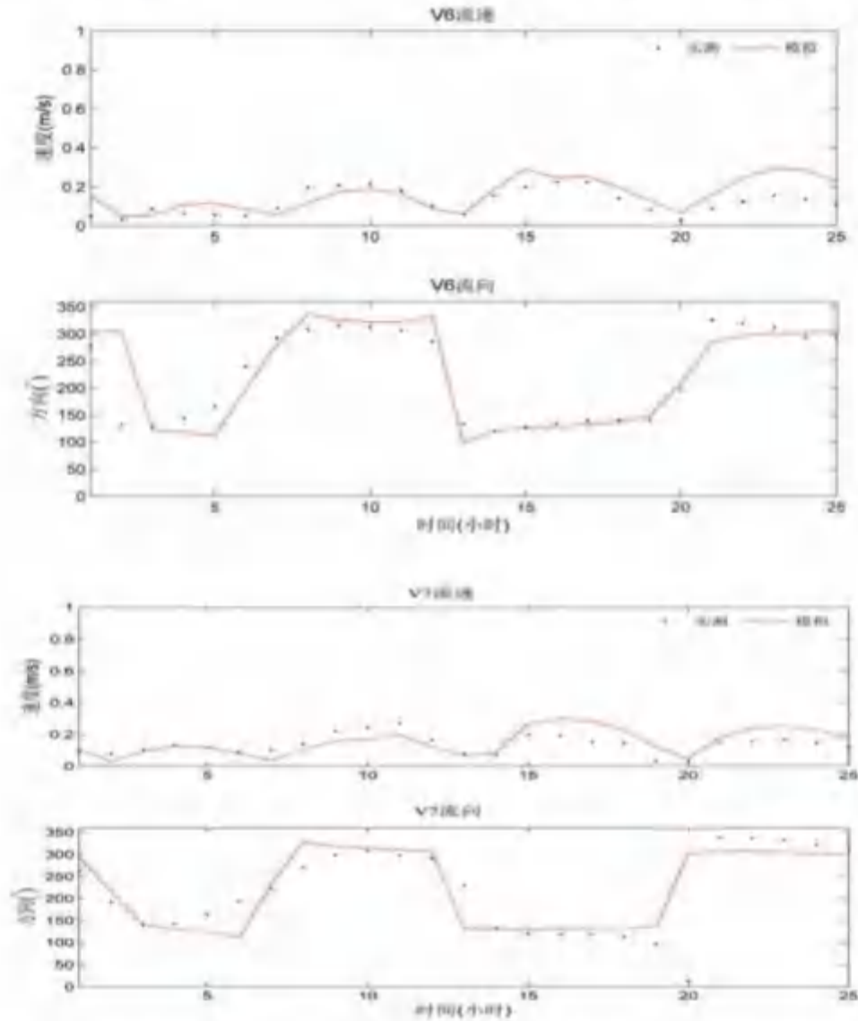
图 6.1.2-3c 2024 年 12 月底层流速流向验证图（·表示实测值，—表示模拟值）
