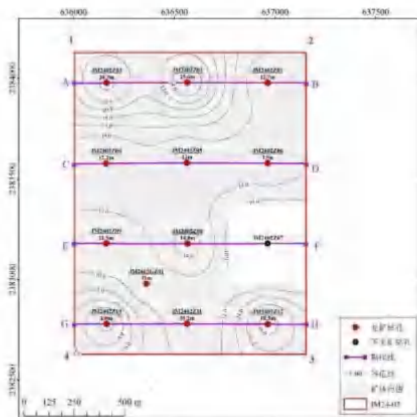
图 3.1.3-4 江门市大帆石北面海域 JM24-02 矿区 V2 矿体海砂等厚度图
