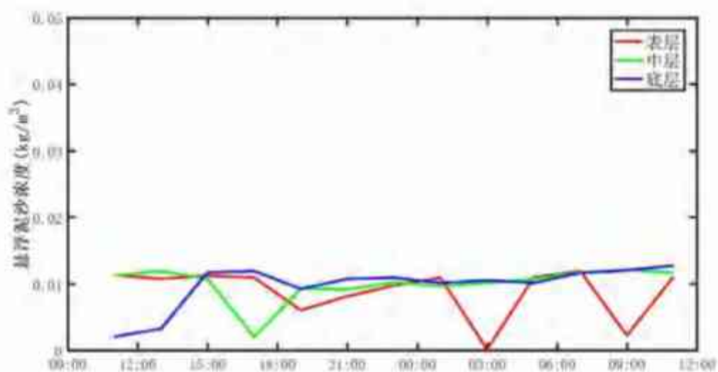
图 5.1.3-9c V3 站悬浮泥沙浓度曲线
