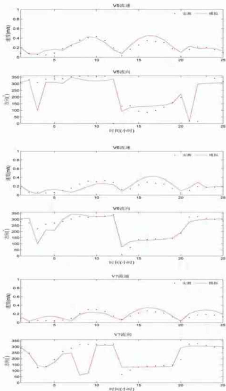
图 6.1.2-3a 2024 年 12 月表层流速流向验证图 (·表示实测值, —表示模拟值)
