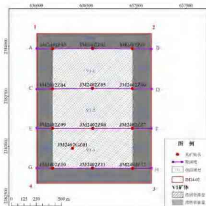
图 3.1.3-1 V1 矿体平面分布图
