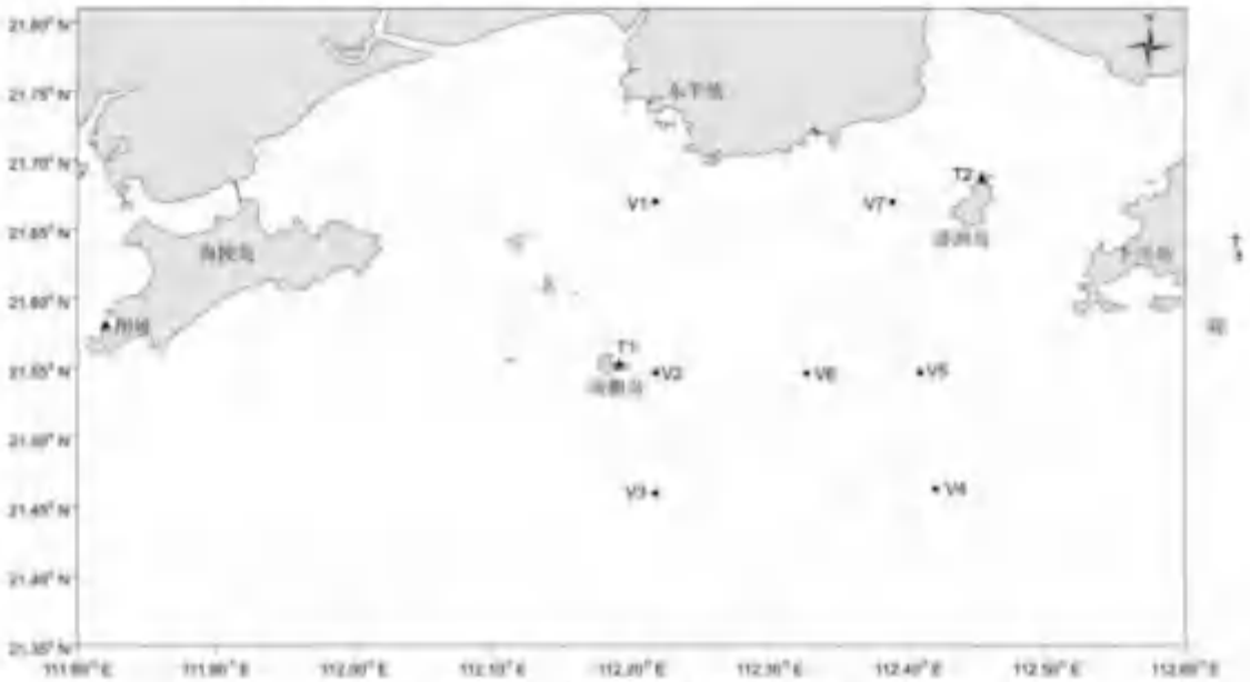
5.1.1-1 水文调查站位布设图
