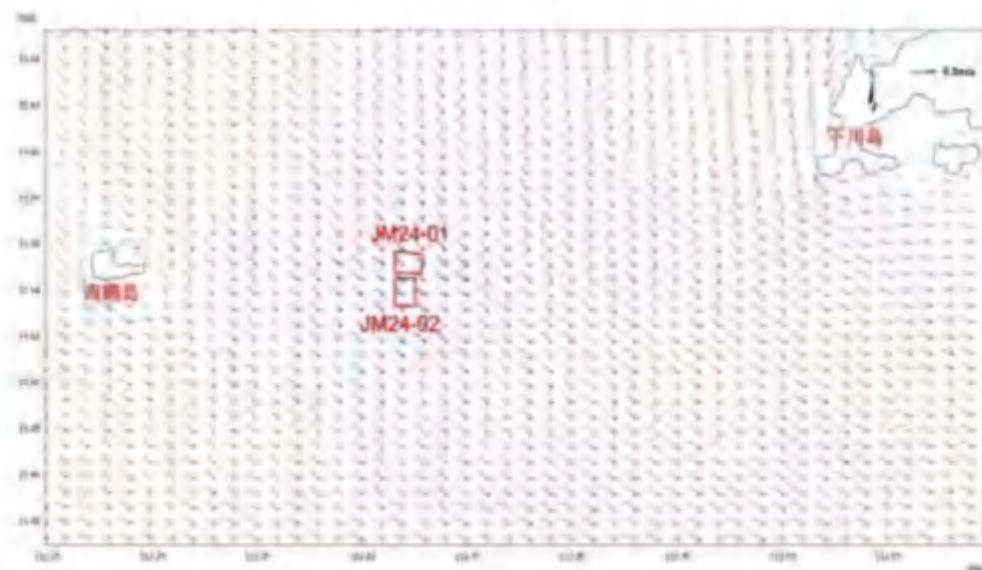
图6.1.3-5b工程海域落急流场对比（中层）
