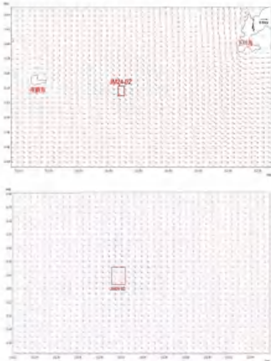
图 6.1.3-3c 工程海域落急流场对比（底层）
