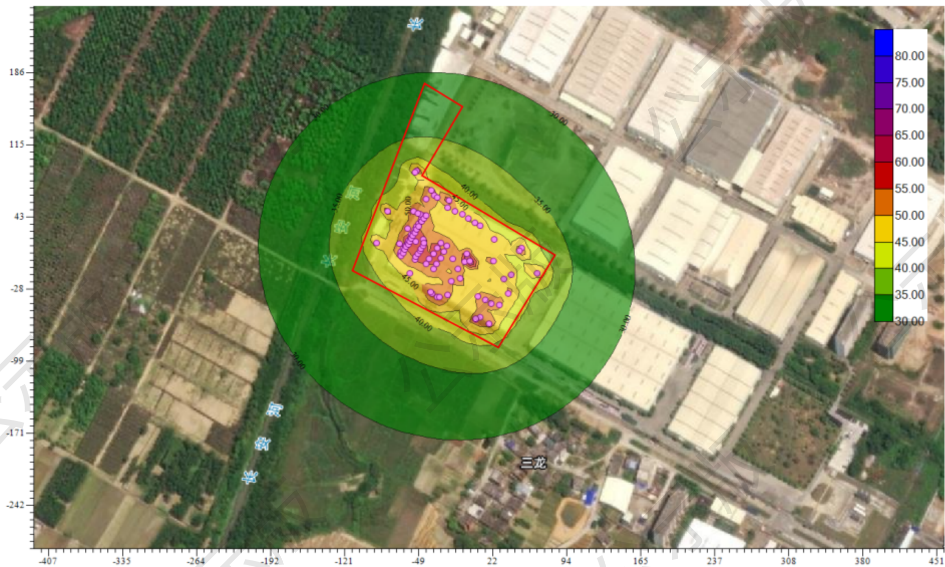
图 4.5-2 噪声等声线图
