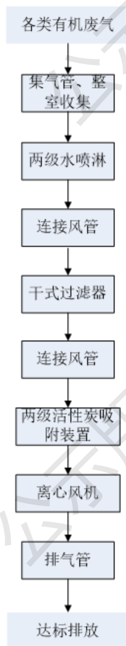
图 6.2-2 有机废气处理工艺流程图
