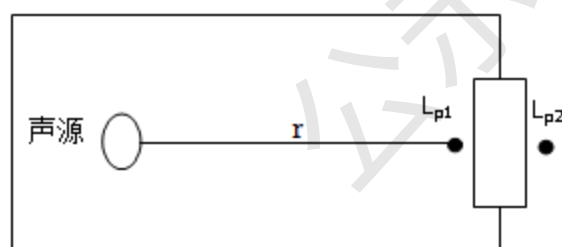
图 4.5-1 室内声源等效为室外声源图例
