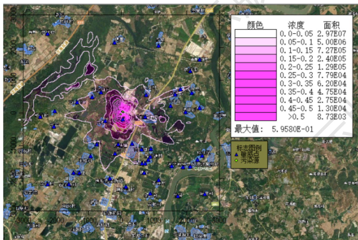
图 4.2-13 PM_{2.5} 日平均浓度贡献值网格浓度分布图(正常排放) 单位: \mu g/m^3
