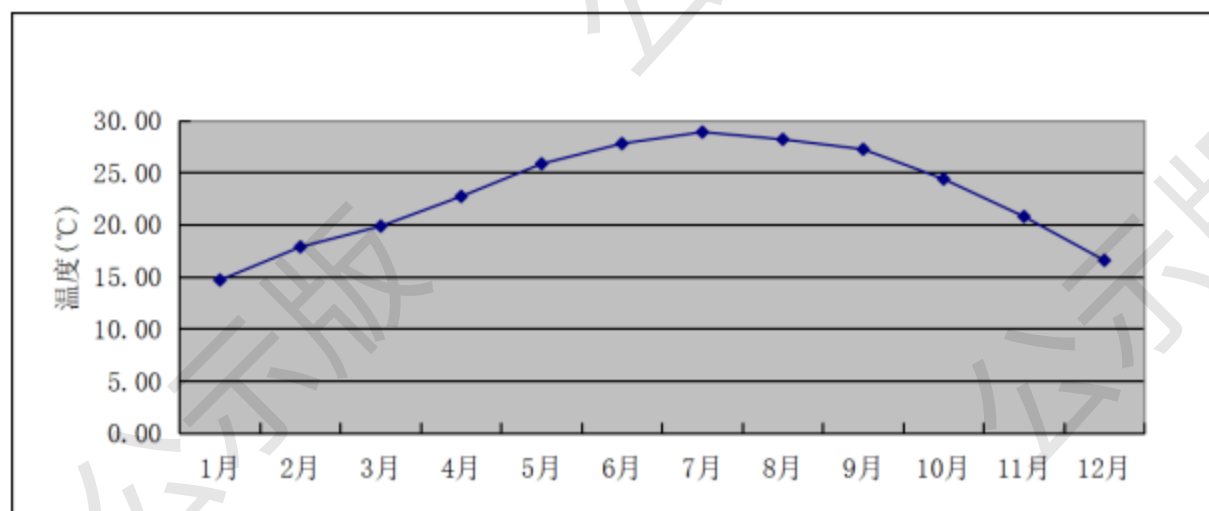
图 4.2-6 恩平气象站 2023 年年平均温度的月变化图
