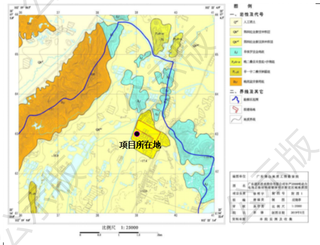
图 4.4-1 区域地质构造图
