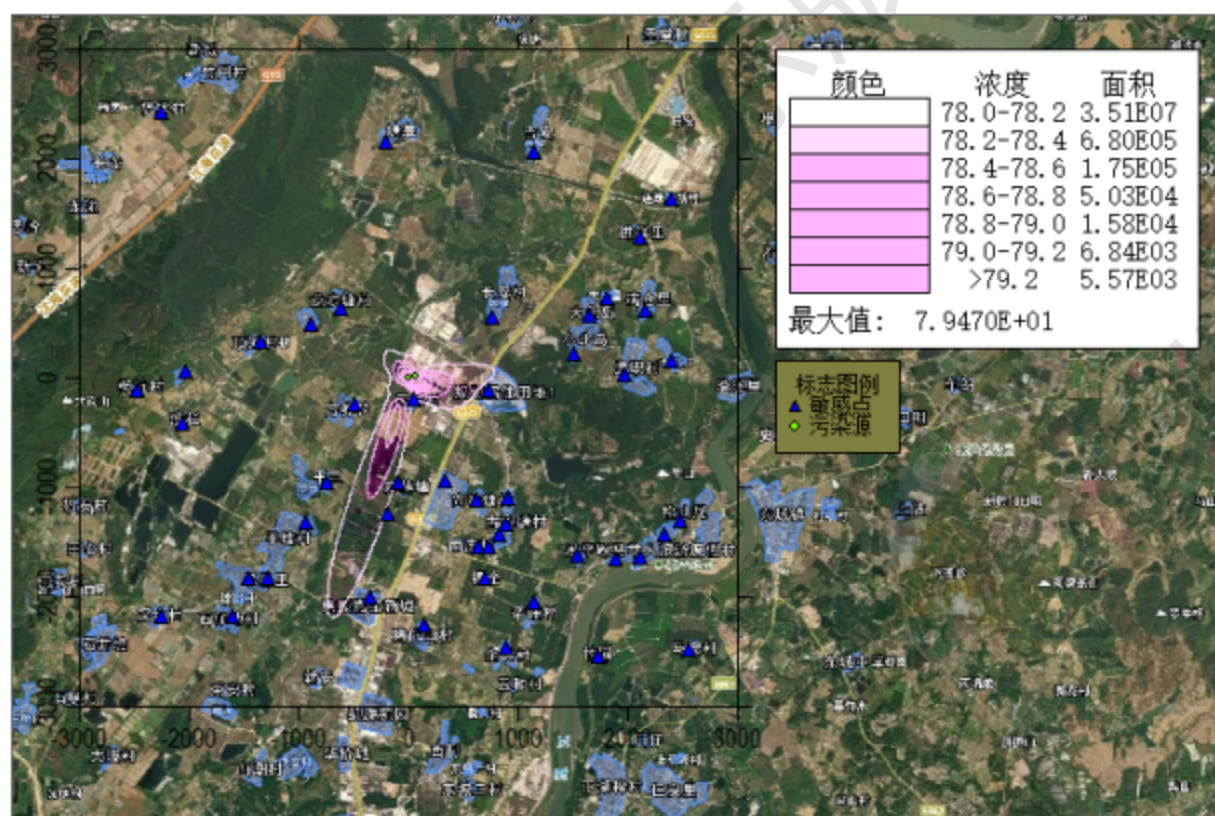
图 4.2-13 叠加后 PM 10 95%日均值浓度分布图(正常排放) 单位: \mu\text{g}/\text{m}^3
