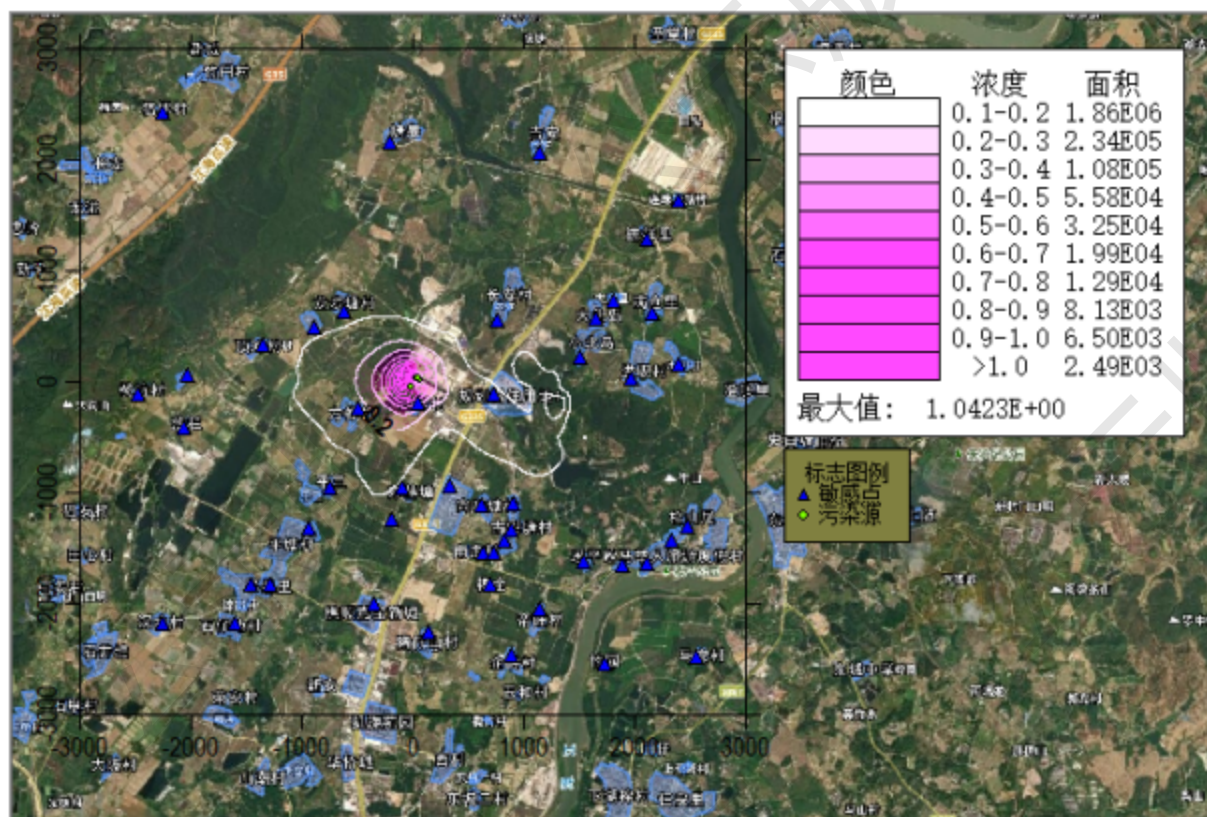
续图 4.2-12 NO 2 年平均浓度贡献值网格浓度分布图(正常排放) 单位: \mu\text{g}/\text{m}^3
