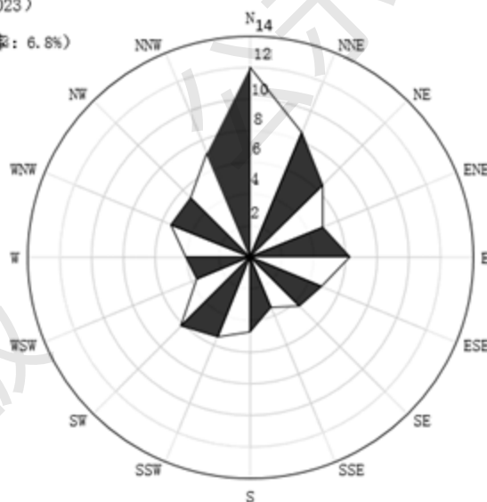
图 4.2-1 风向玫瑰图(静风频率 6.8%)
