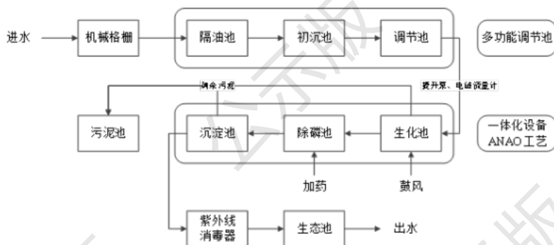
图 4.3-1 圣堂镇污水处理厂工艺流程图
