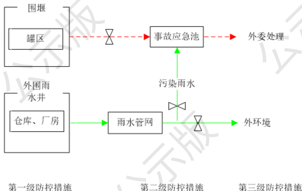
图 5.8-2 项目事故废水分区防控图
