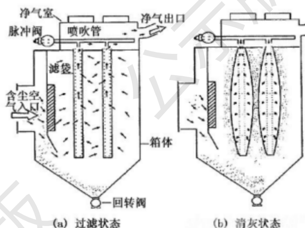
图 6.2-3 脉冲布袋除尘器处理工艺流程图
