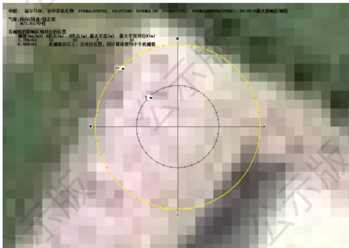
图 5.7-3 最常见气象条件下，甲醛最大影响区域图
