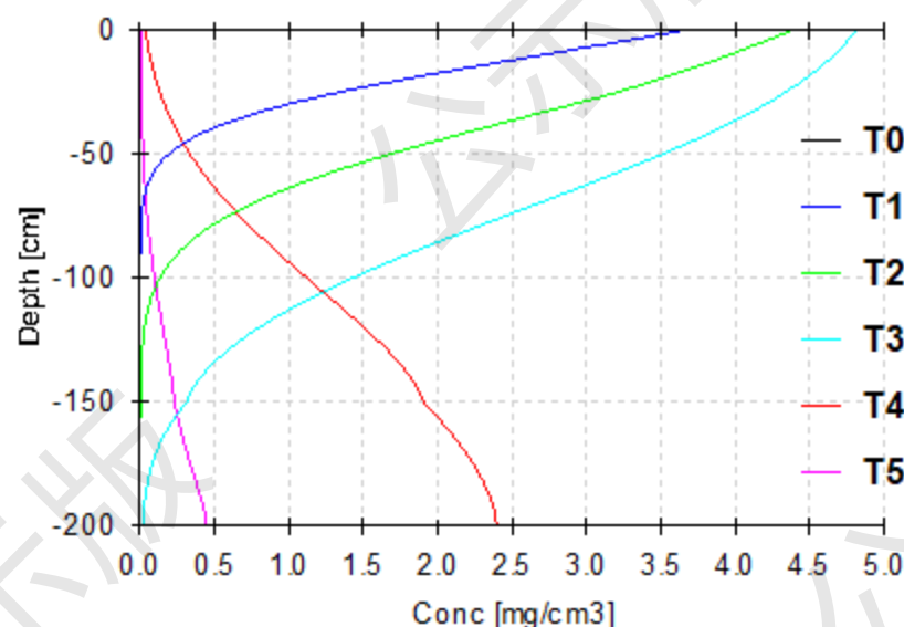
图 4.7-3 剖面上不同时间甲醛浓度随深度变化情况
