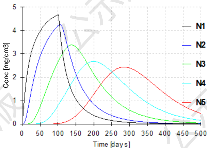
图 4.7-2 土壤各观测点甲醛浓度-时间曲线图
