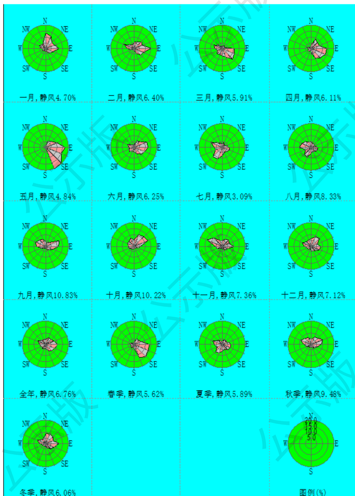
图4.2-9 恩平气象站2023年风向玫瑰图
