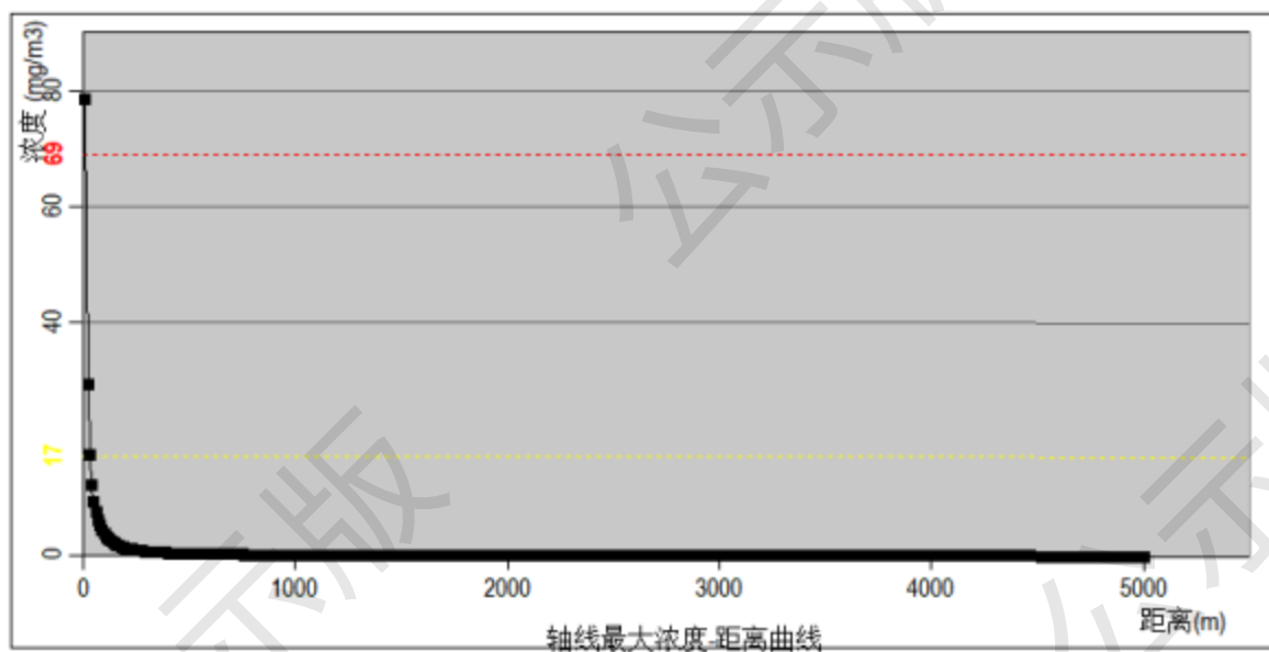
图 5.7-2 最不利气象条件下，甲醛轴线最大浓度图
