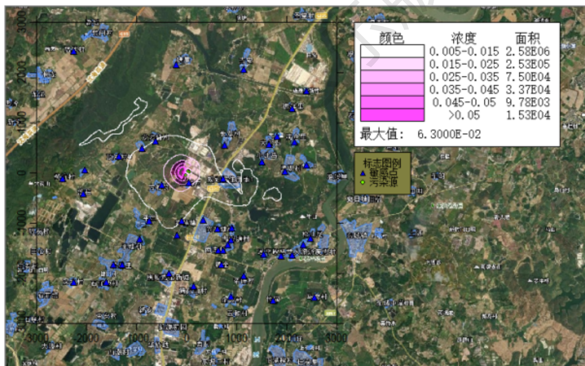
续图 4.2-11 SO 2 年平均浓度贡献值网格浓度分布图(正常排放) 单位: \mu\text{g}/\text{m}^3
