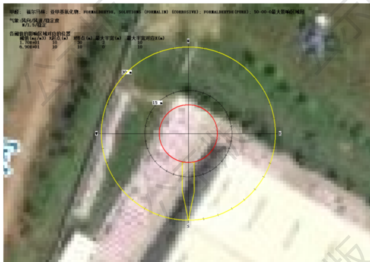
图 5.7-1 最不利气象条件下，甲醛最大影响区域图
