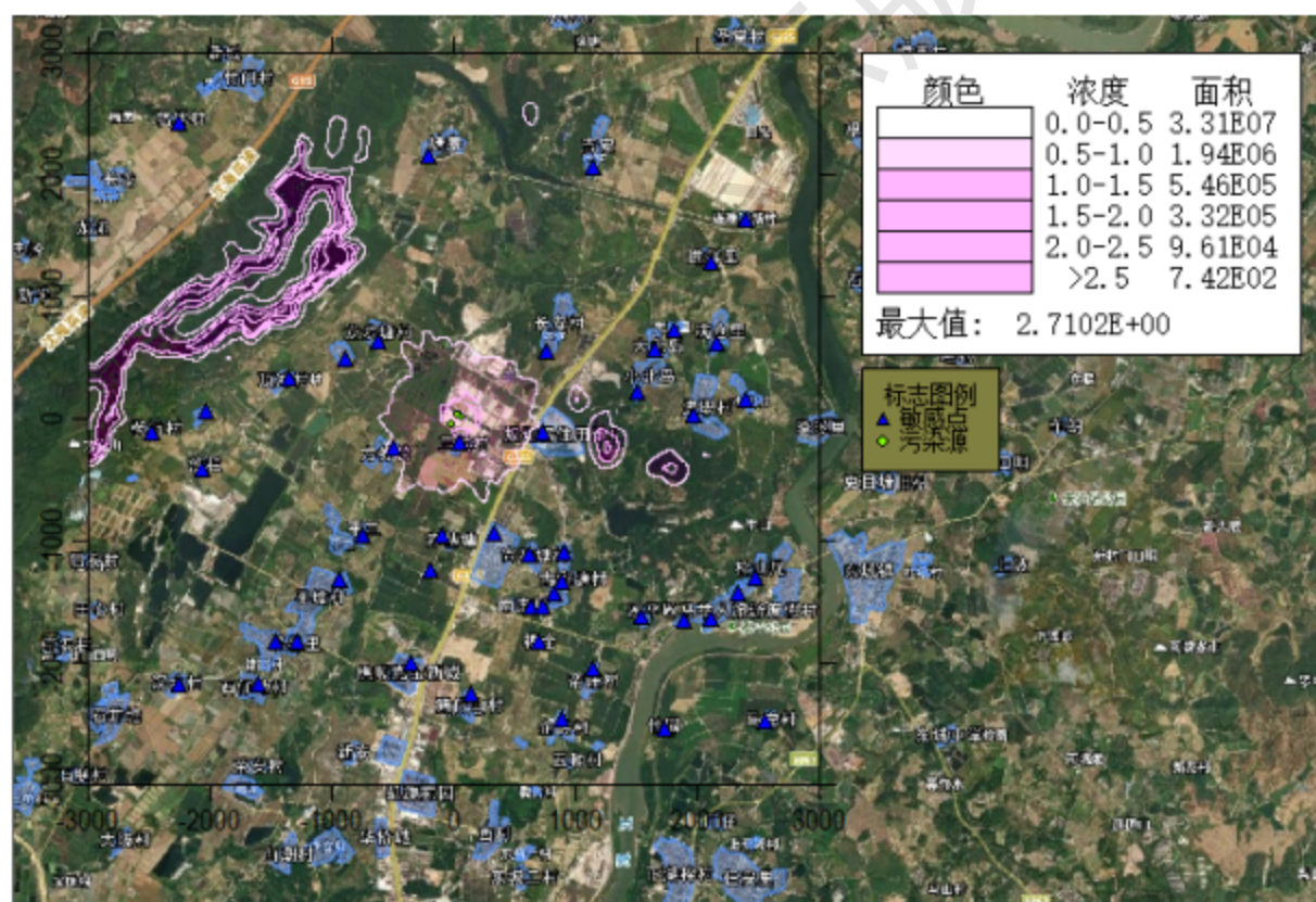
图 4.2-19 苯系物小时浓度贡献值网格浓度分布图(正常排放) 单位: \mu\text{g}/\text{m}^3
