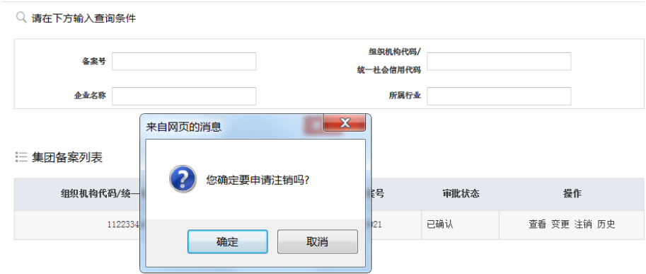
图 2.14 注销页面
