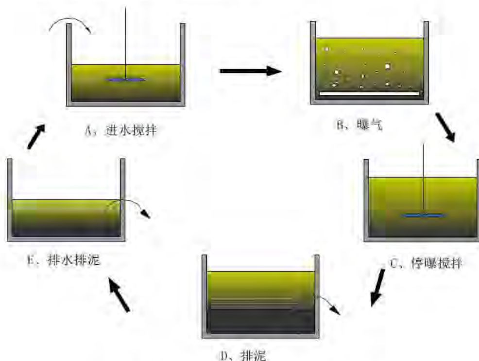
图 3.4-6 传统 SBR 工艺除磷脱氮运行图
