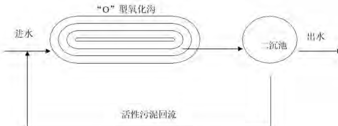
图 3.4-5 “O”型氧化沟流程简图
