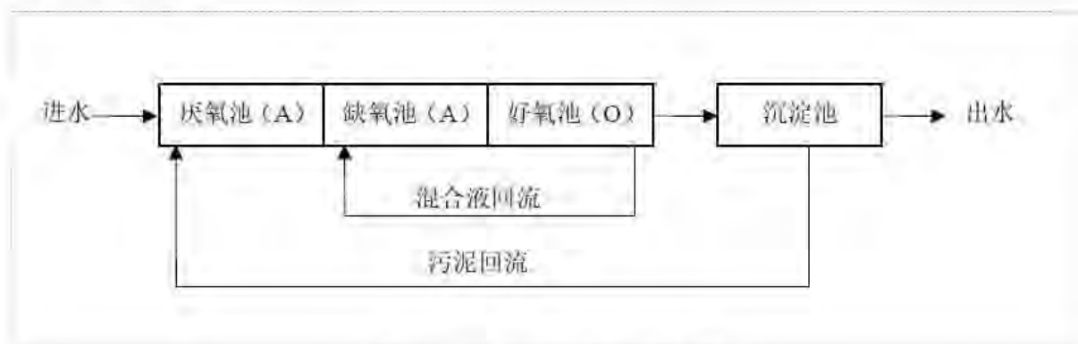
图 3.4.1 A 2 /O 工艺流程框图
