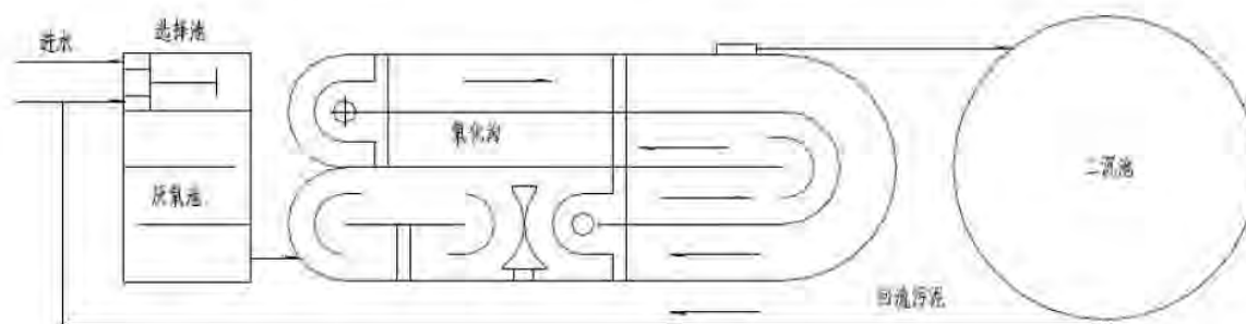
图 3.4-3 Carrousel 2000 氧化沟流程简图
