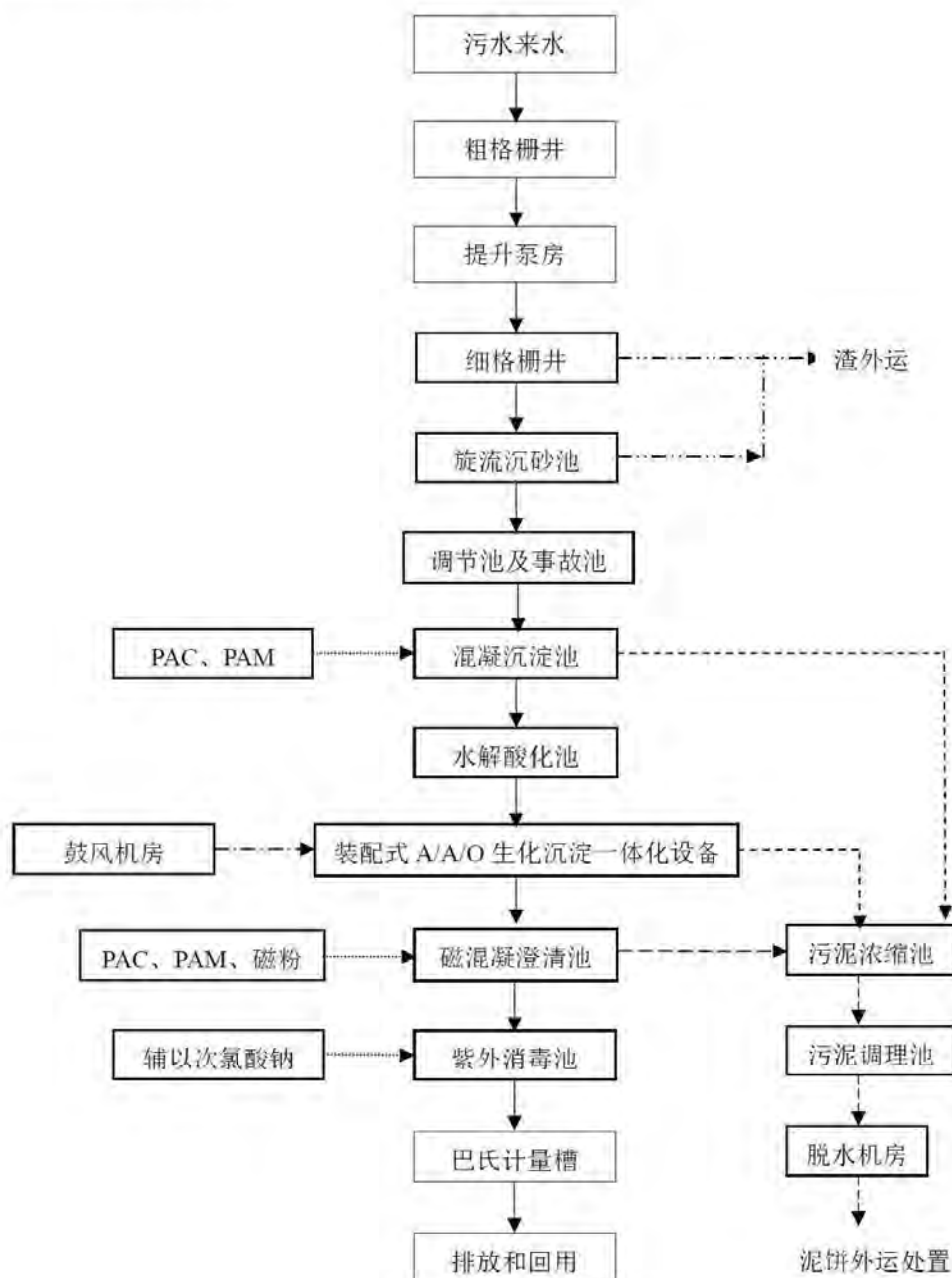
图 3.4-13 污水处理工程工艺流程图
