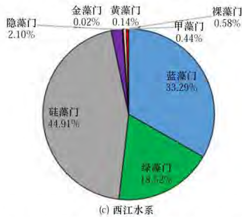
图 4.8-3 西江水系浮游植物密度占比（门水平）图
