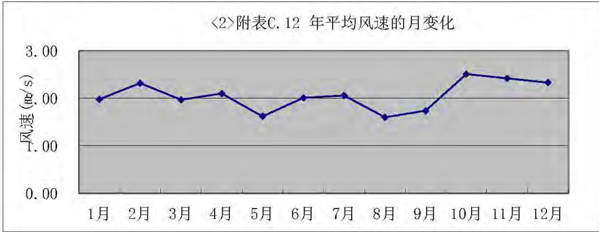
图 5.2-9 鹤山市 2024 年平均风速的月变化曲线图
