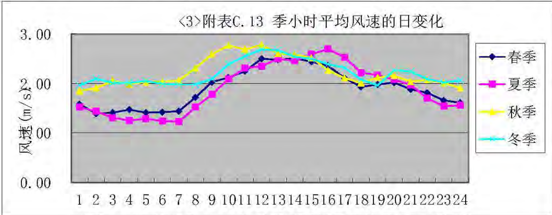
图 5.2-10 鹤山市 2024 年季小时平均风速的日变化曲线图
