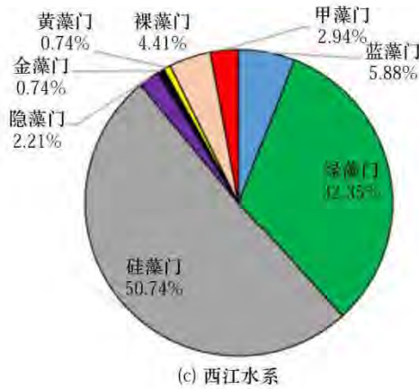
图 4.8-2 西江水系浮游植物群落组成及其占比图
