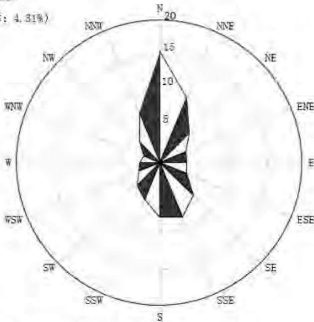
图 5.2-7 鹤山风向玫瑰图 (2005-2024)
