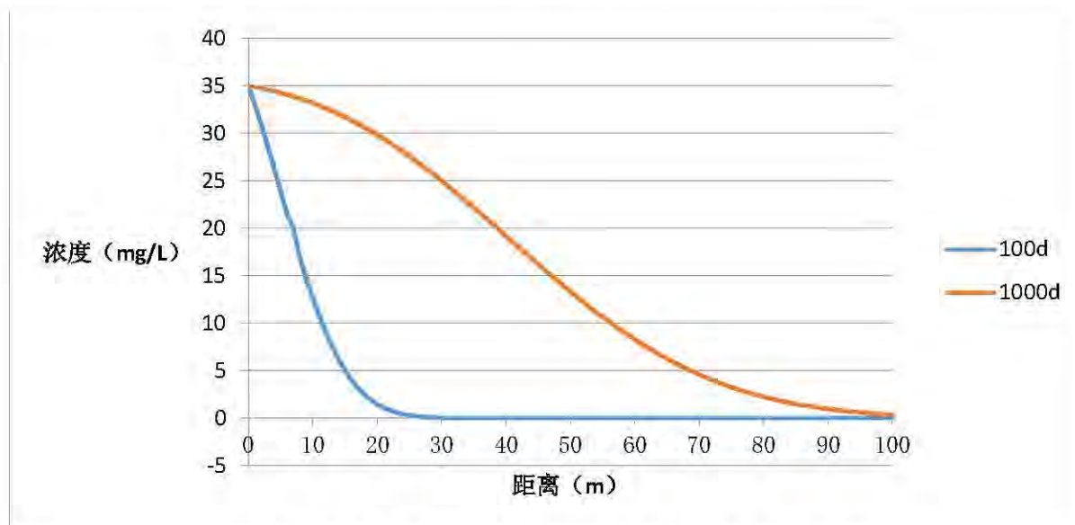
图 5.2-6 污染物 NH 3 -N 连续渗漏情况预测统计图
