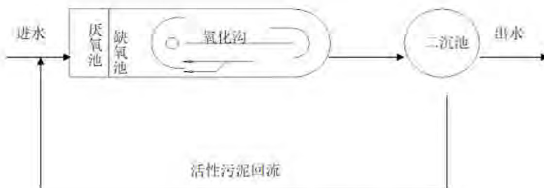
图 3.4-2 A 2 /C 氧化沟流程简图
