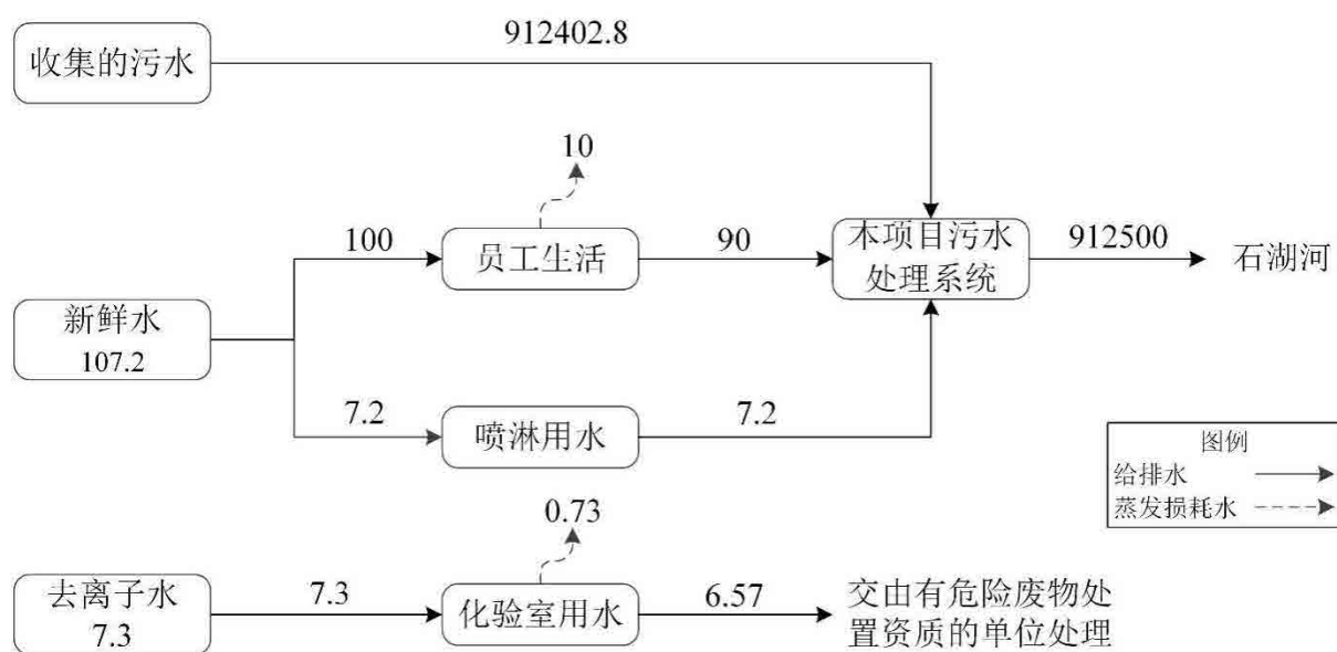
图 3.3-1 项目水平衡图 (单位: \text{m}^3/\text{a} )
