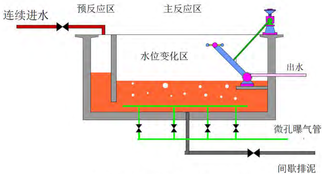
图 3.4-7 ICEAS 反应器基本构造图
