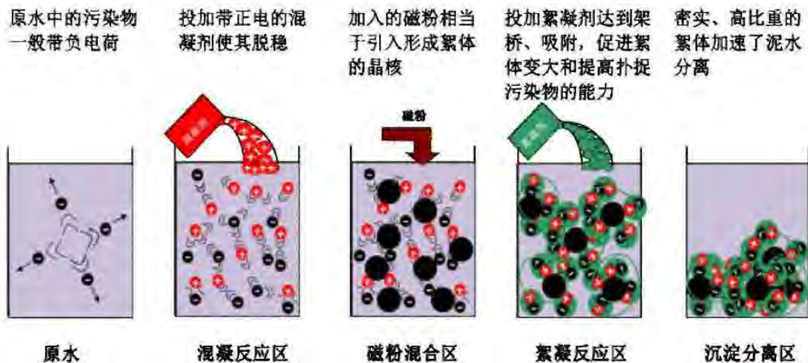
图 3.4-11 磁混凝澄清技术工艺原理图
