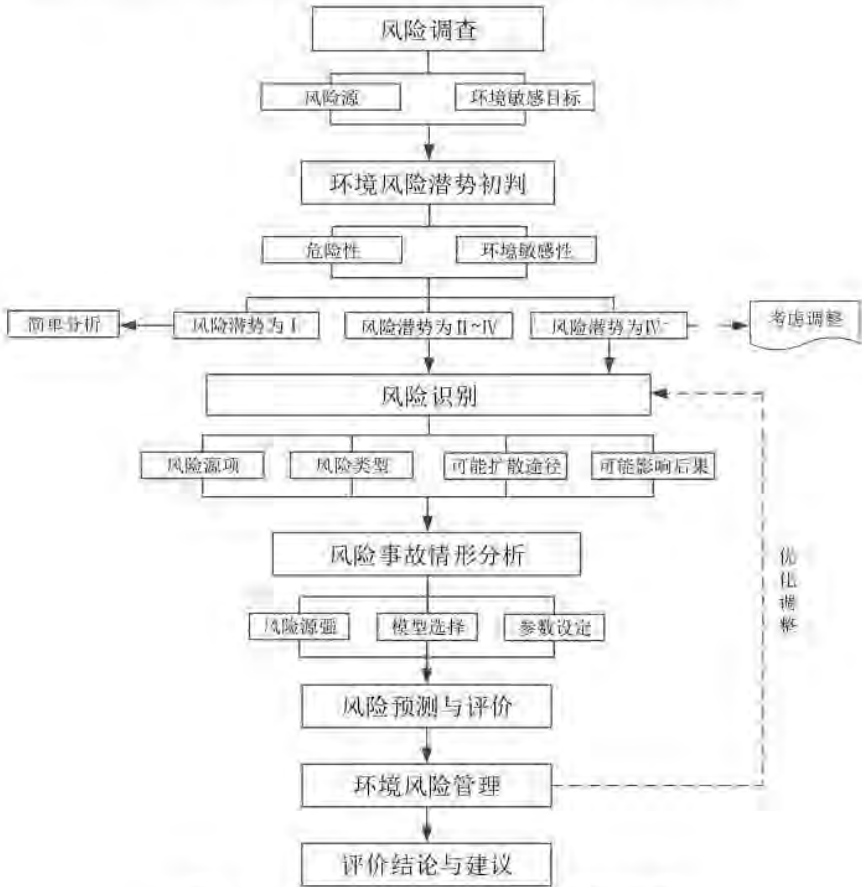
图 5.2-27 环境风险评价工作程序图
