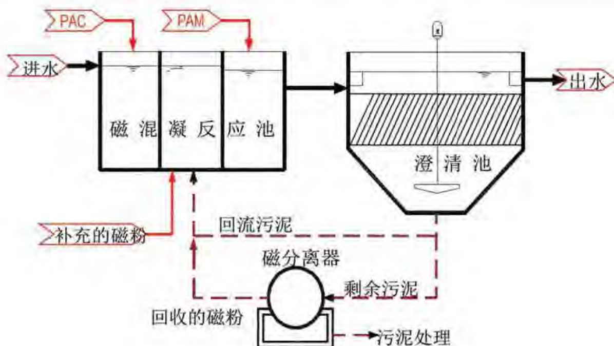
图 3.4-12 磁混凝澄清的系统构成图
