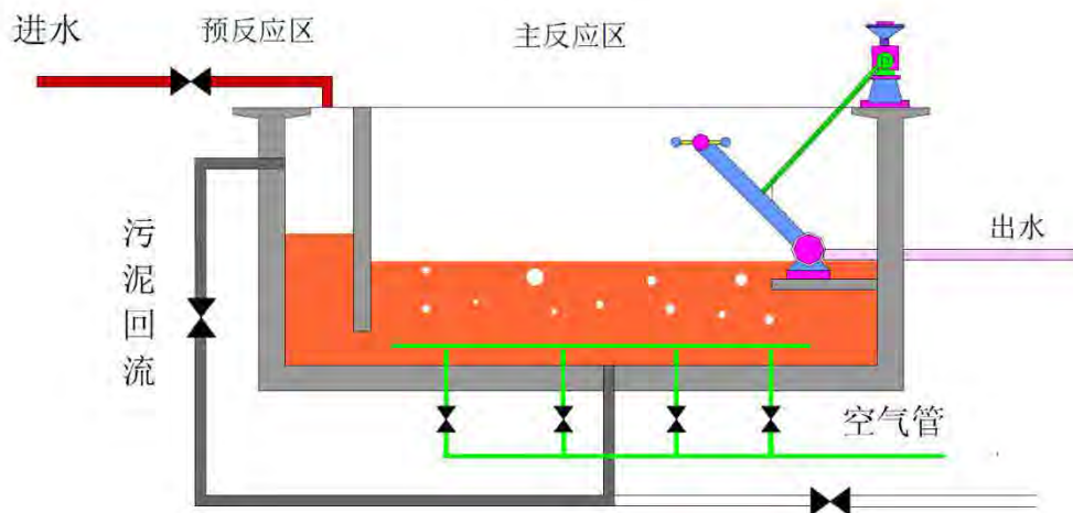
图 3.4-8 CASS 反应器基本构造图
