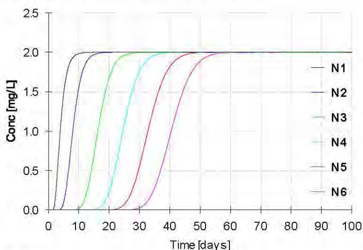
图 5.2-25 锌在不同时间的浓度分布图（N1~N6 为深度 0.1m、0.2m、0.4m、0.6m、0.8m、1.0m）
