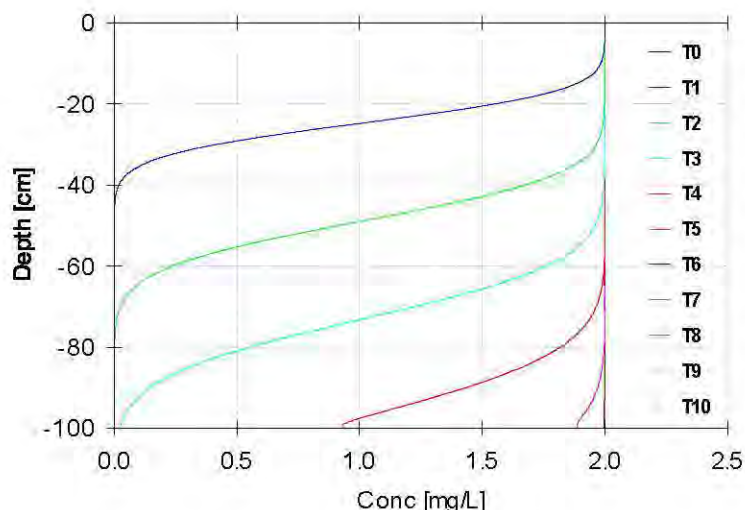
图 5.2-26 锌在不同深度的浓度分布图 (T0~T10 为时间 0d、10d、20d、30d、40d、50d、60d、70d、80d、90d、100d)
