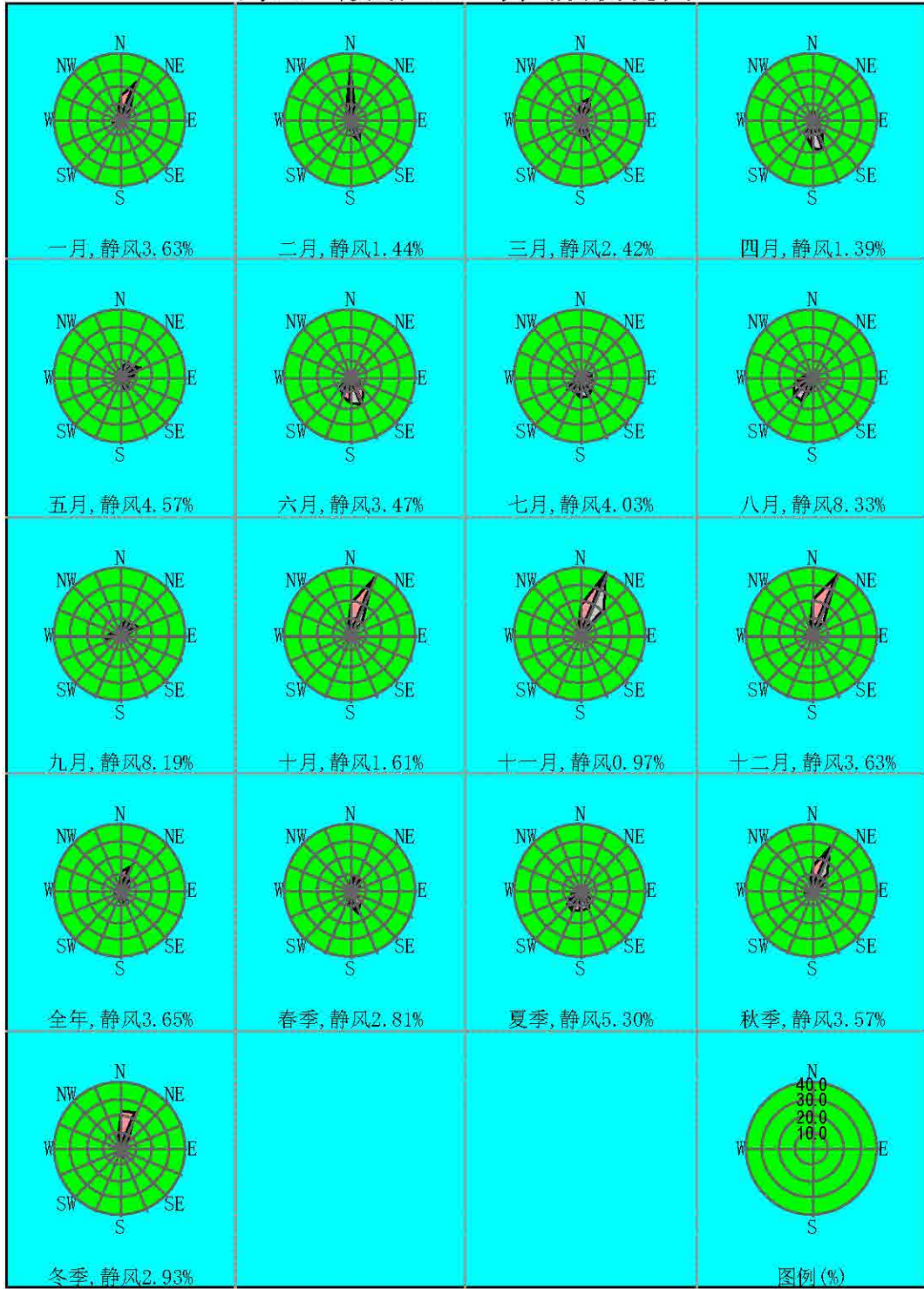
图 5.2-11 鹤山市 2024 年风频玫瑰图
