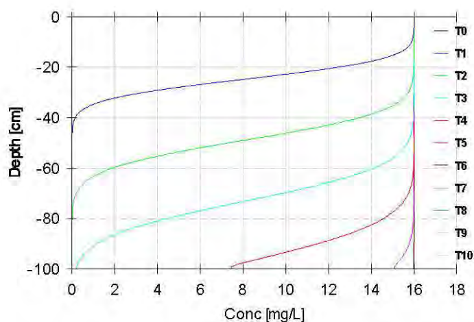
图 5.2-24 石油烃在不同深度的浓度分布图（T0~T10 为时间 0d、10d、20d、30d、40d、50d、60d、70d、80d、90d、100d）
