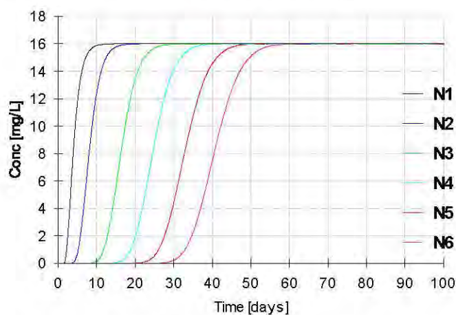
图 5.2-23 石油烃在不同时间的浓度分布图（N1~N6 为深度 0.1m、0.2m、0.4m、0.6m、0.8m、1.0m）
