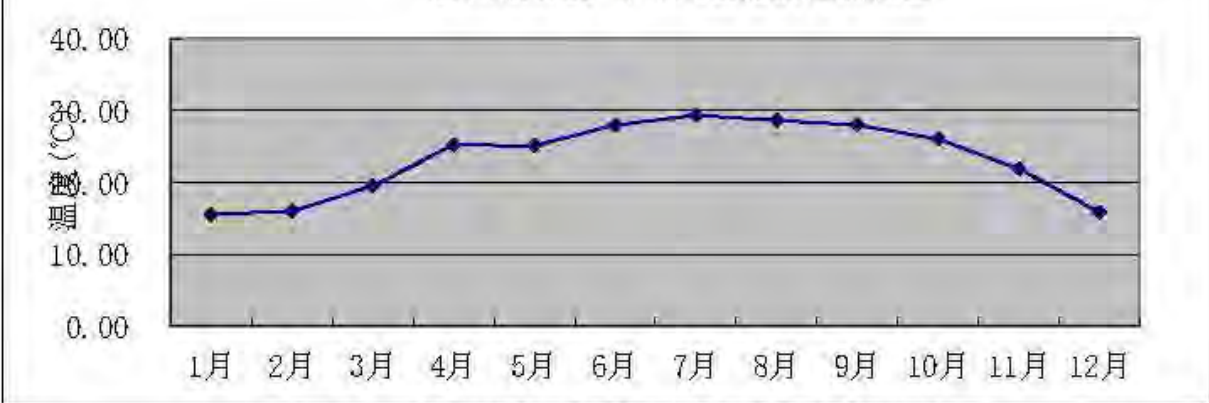
图 5.2-8 鹤山市 2024 年平均温度的月变化曲线图
