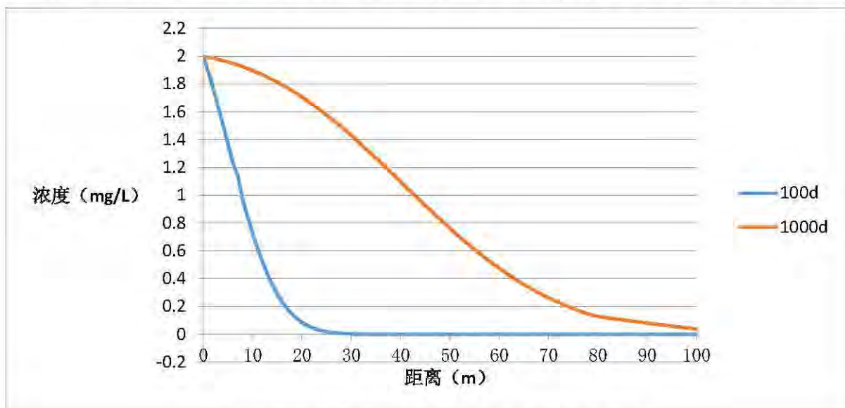
图 5.2-5 污染物铝连续渗漏情况预测统计图
