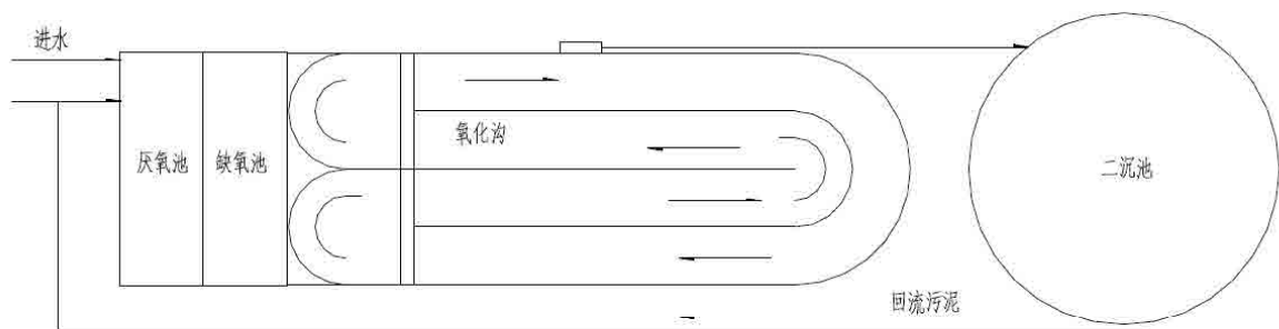
图 3.4-4 曝气氧化沟示意图
