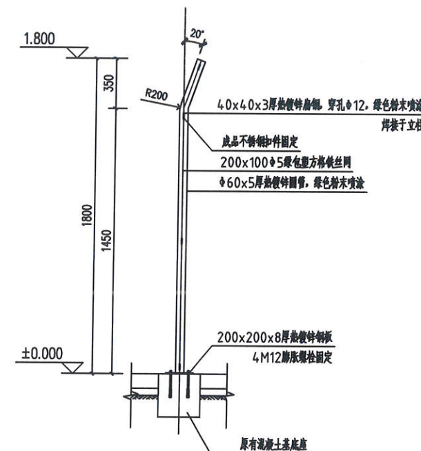
围栏详图
