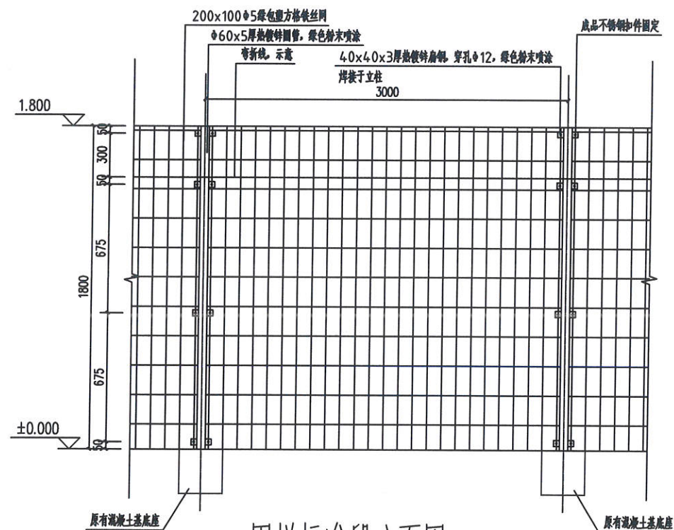
围栏标准段立面图
