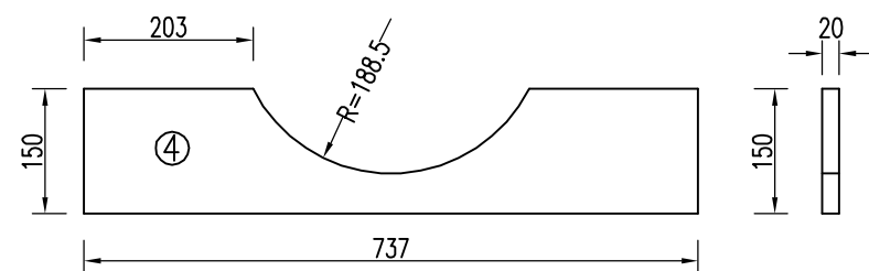
横梁加劲肋大样图 1:10
