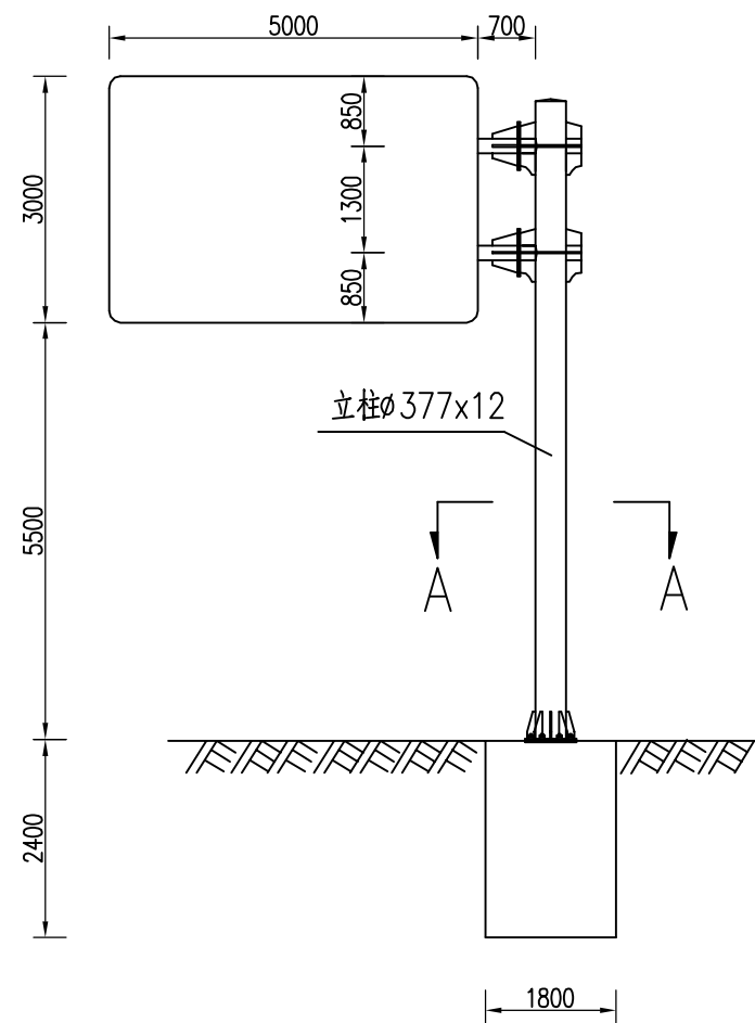
标志立面图 1:100
