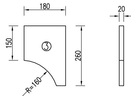
横梁加劲肋大样图 1:10
