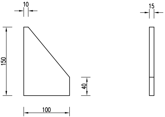
底座加劲肋
