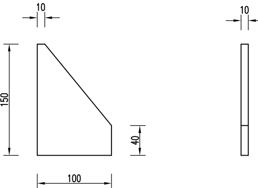
底座加劲肋
