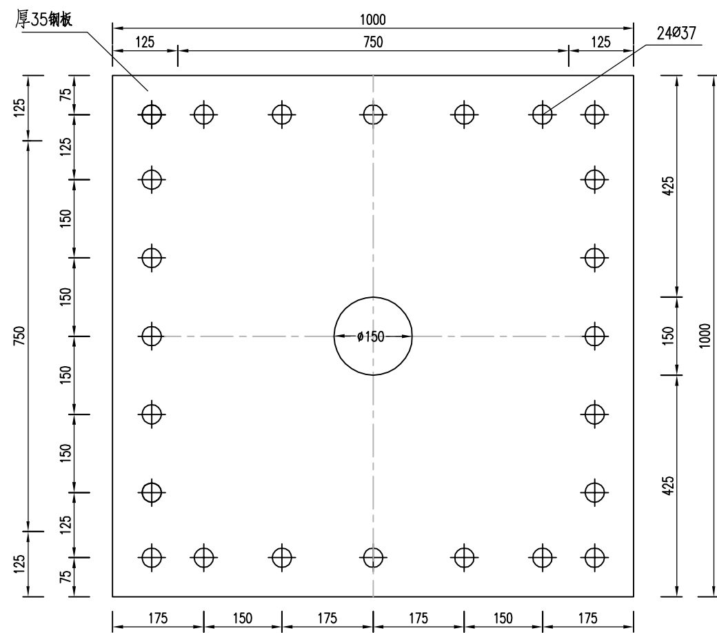
立柱底座法兰板 (右旋90°) 1:10
