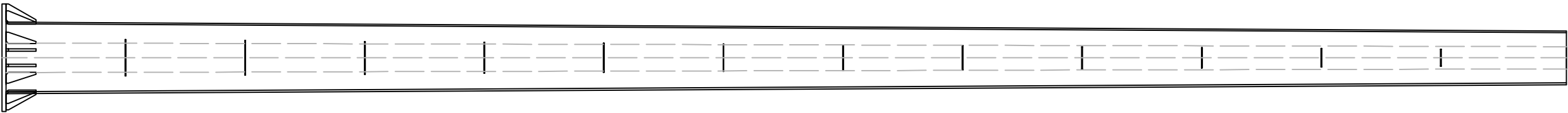
横梁加强肋平面布置图 1:40
