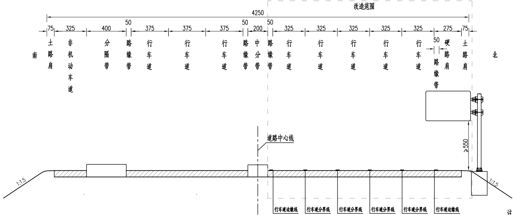
改造后交通工程横断面布置图 旧S274 1:200
