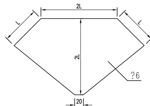
加强肋大样图 1:5
