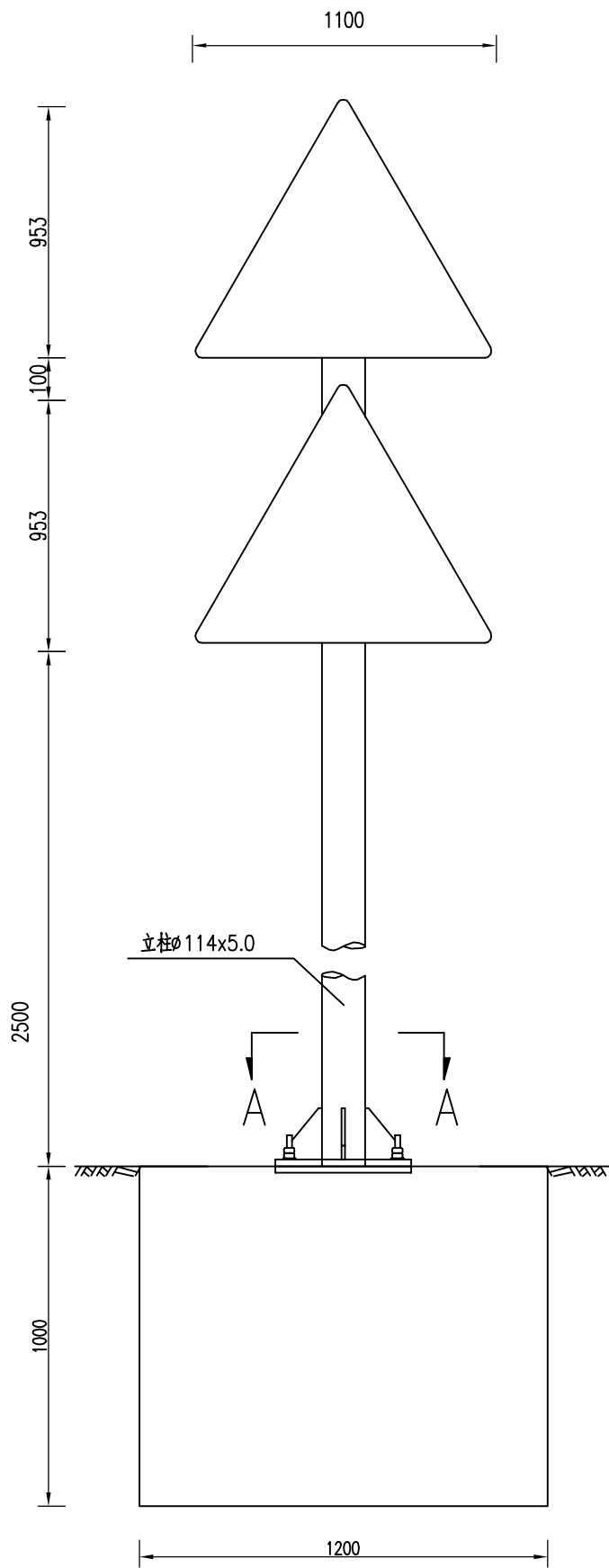
标志立面图
