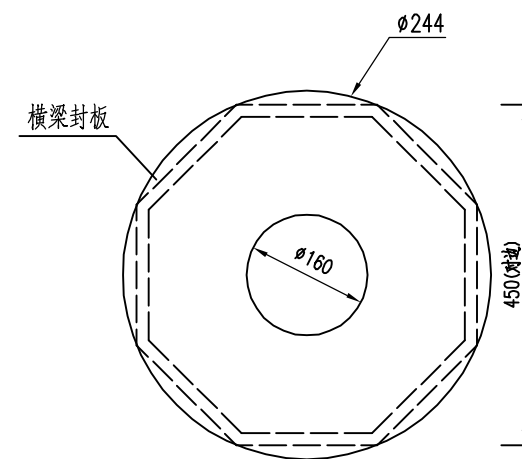
A向 1:10
