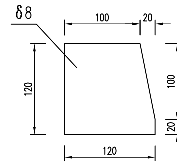
加劲肋2大样 1:5
