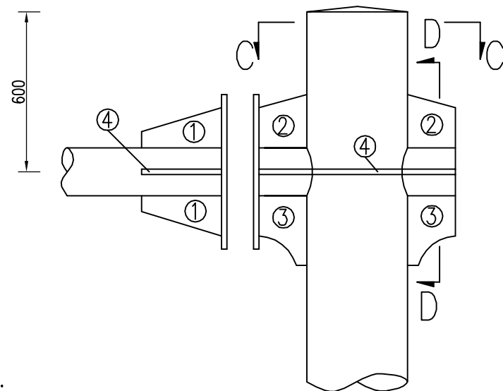
立柱与横梁连接部大样图 1:20
