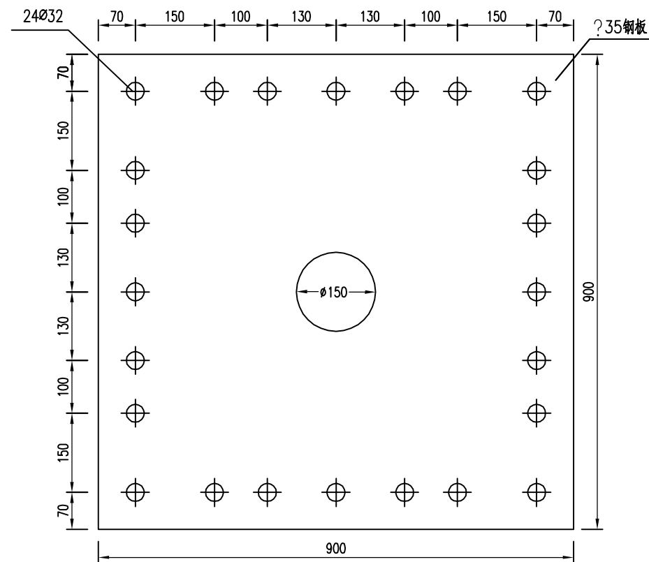
横梁法兰板2 1:10
