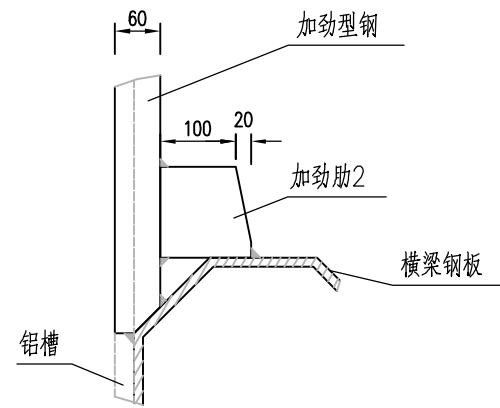
节点1侧面 1:10
