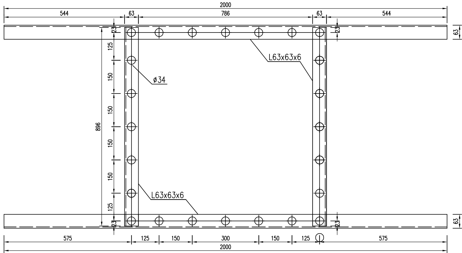
角钢框架平面图 1:10
