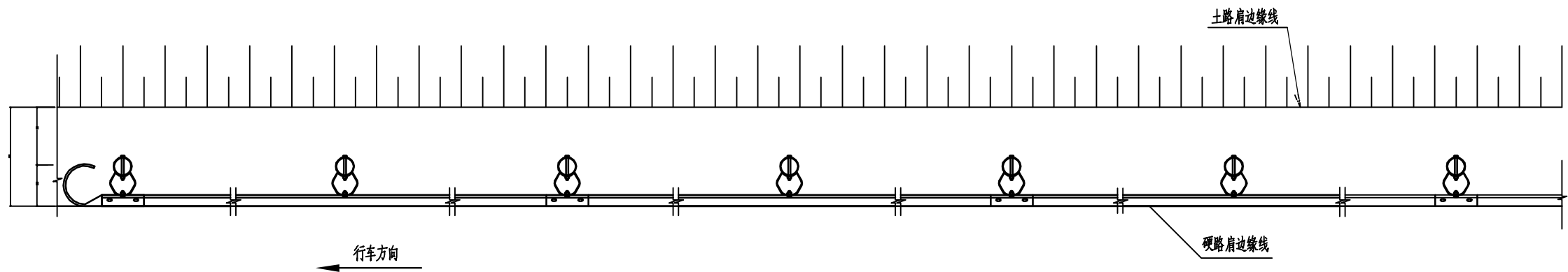
下游端头连接平面图(A级AT2-1) 1:40
