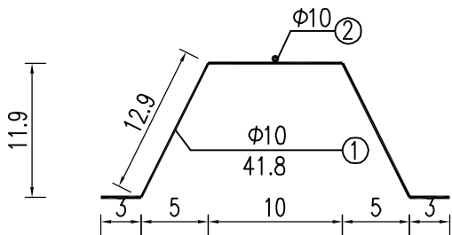
传力杆支架大样图
