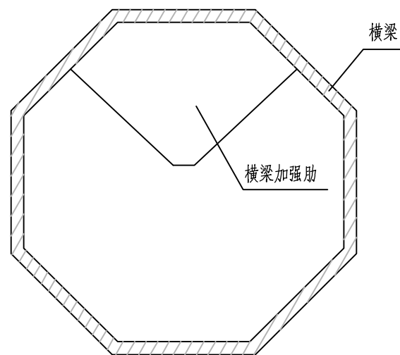
C-C 1:5
