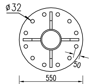
D-D剖面图 1:20
