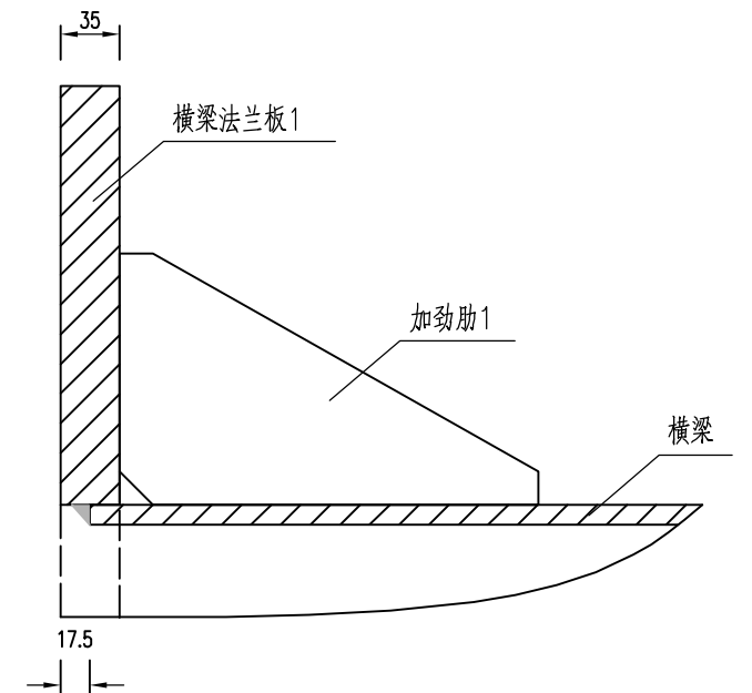
节点2大样 1:5
