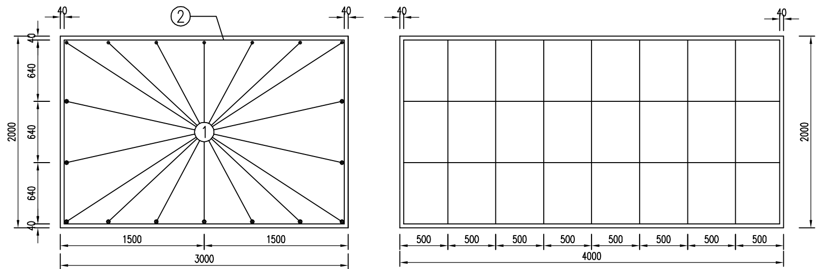
基础配筋图 1:40
