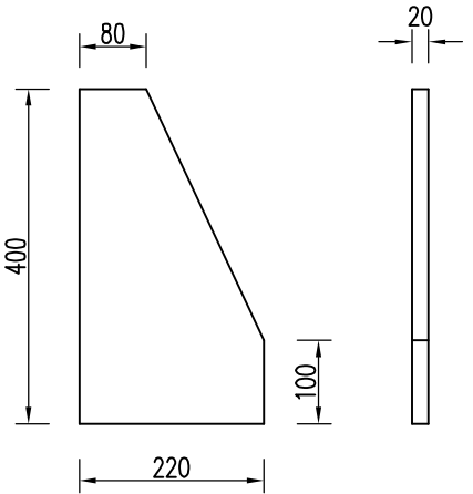
底座加劲肋 1:5
