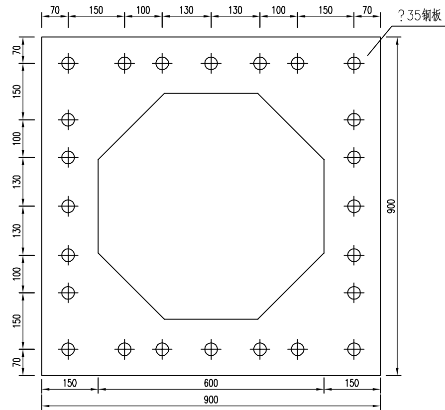
横梁法兰板1 1:10
