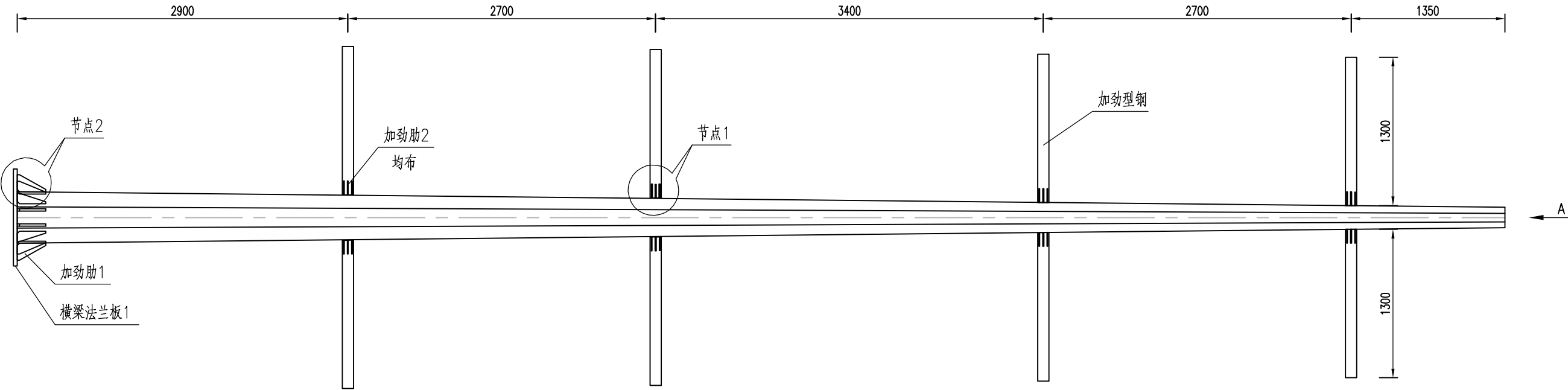
横梁大样图 1:40
