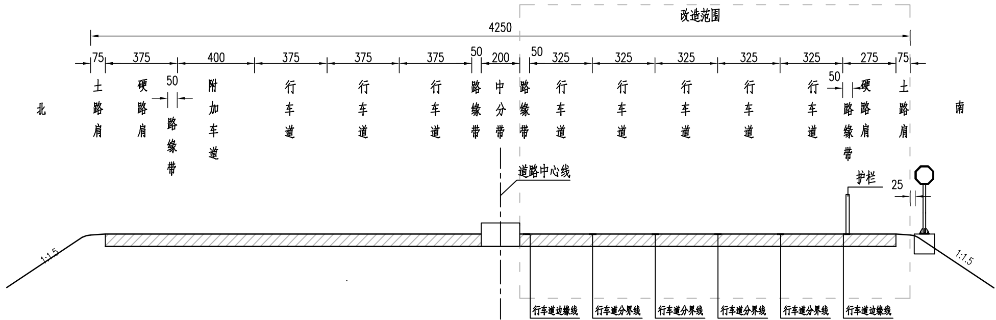
改造后交通工程横断面布置图 S533 1:200
