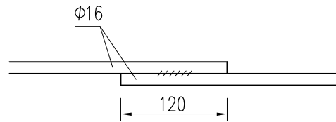
地板搭接焊大样图
