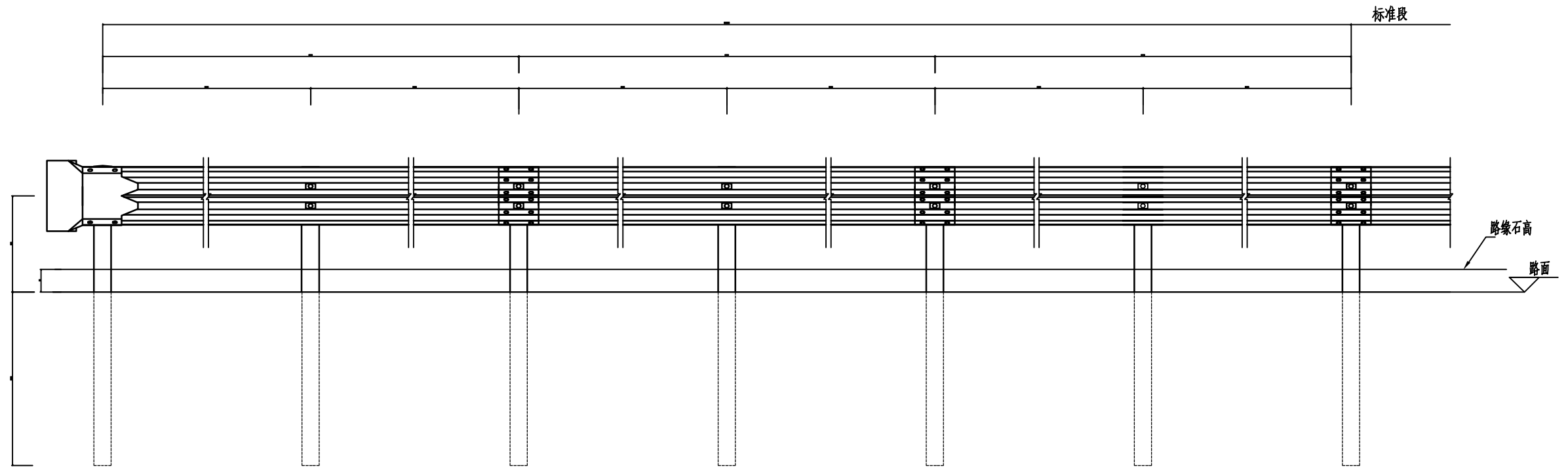
下游端头连接立面图(A级AT2-1) 1:40
