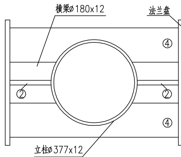
C-C剖面图 1:10
