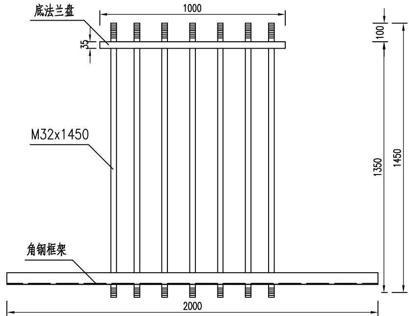
角钢框架立面图 1:20
