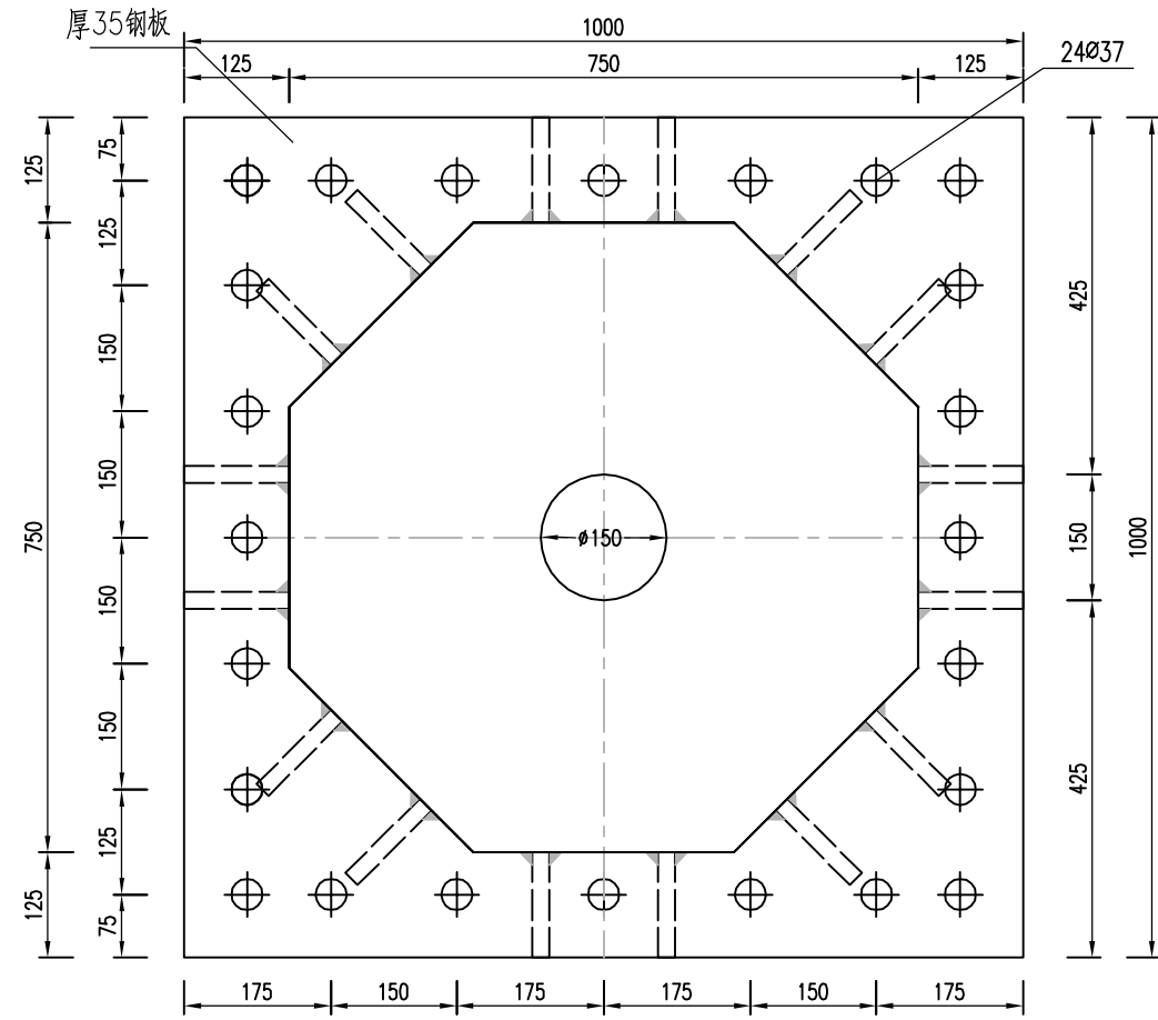
C向 1:10
