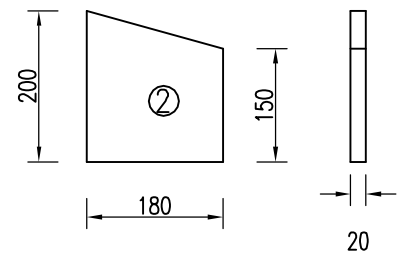
横梁加劲肋大样图 1:10
