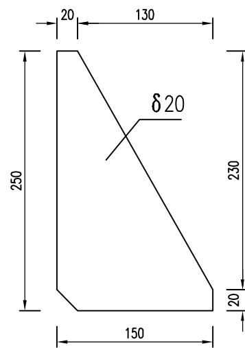
加劲肋1大样 1:5
