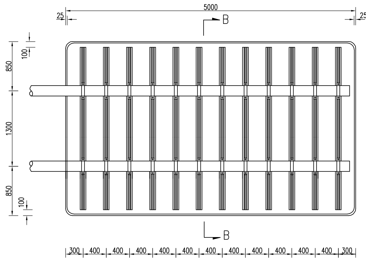
标志板与横梁连接图 1:40
