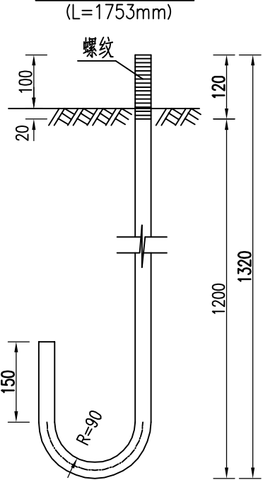
M30地脚大样图 1:20
