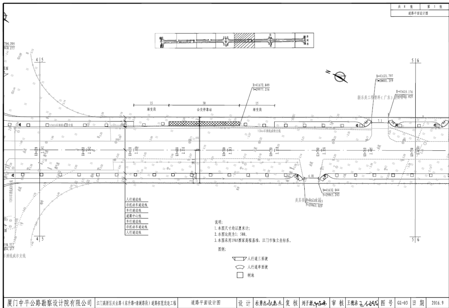
附图 11 道路平面设计图 (五)
