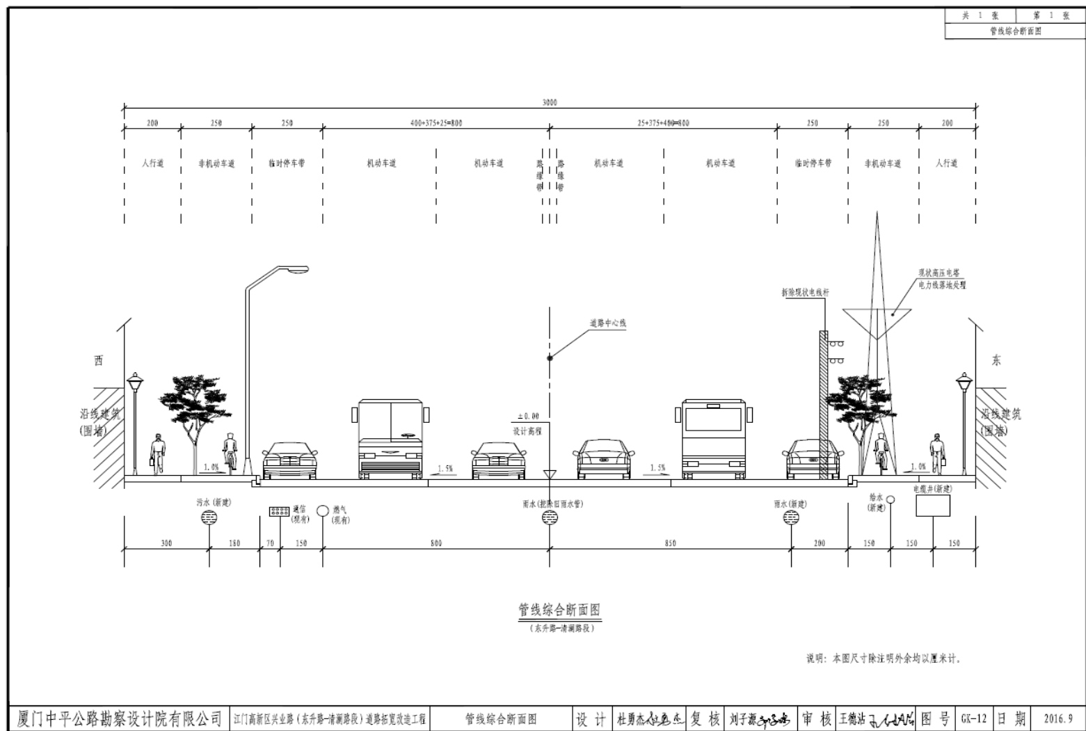
附图 6 管线综合断面图
