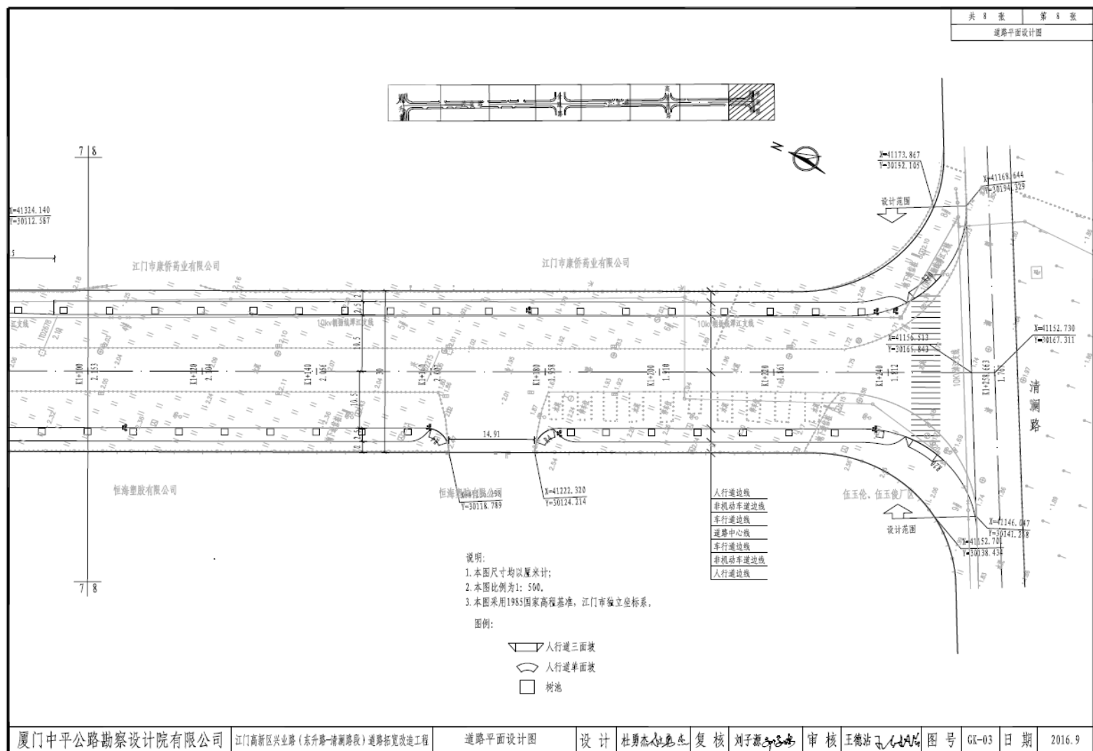
附图 13 道路平面设计图 (七)
